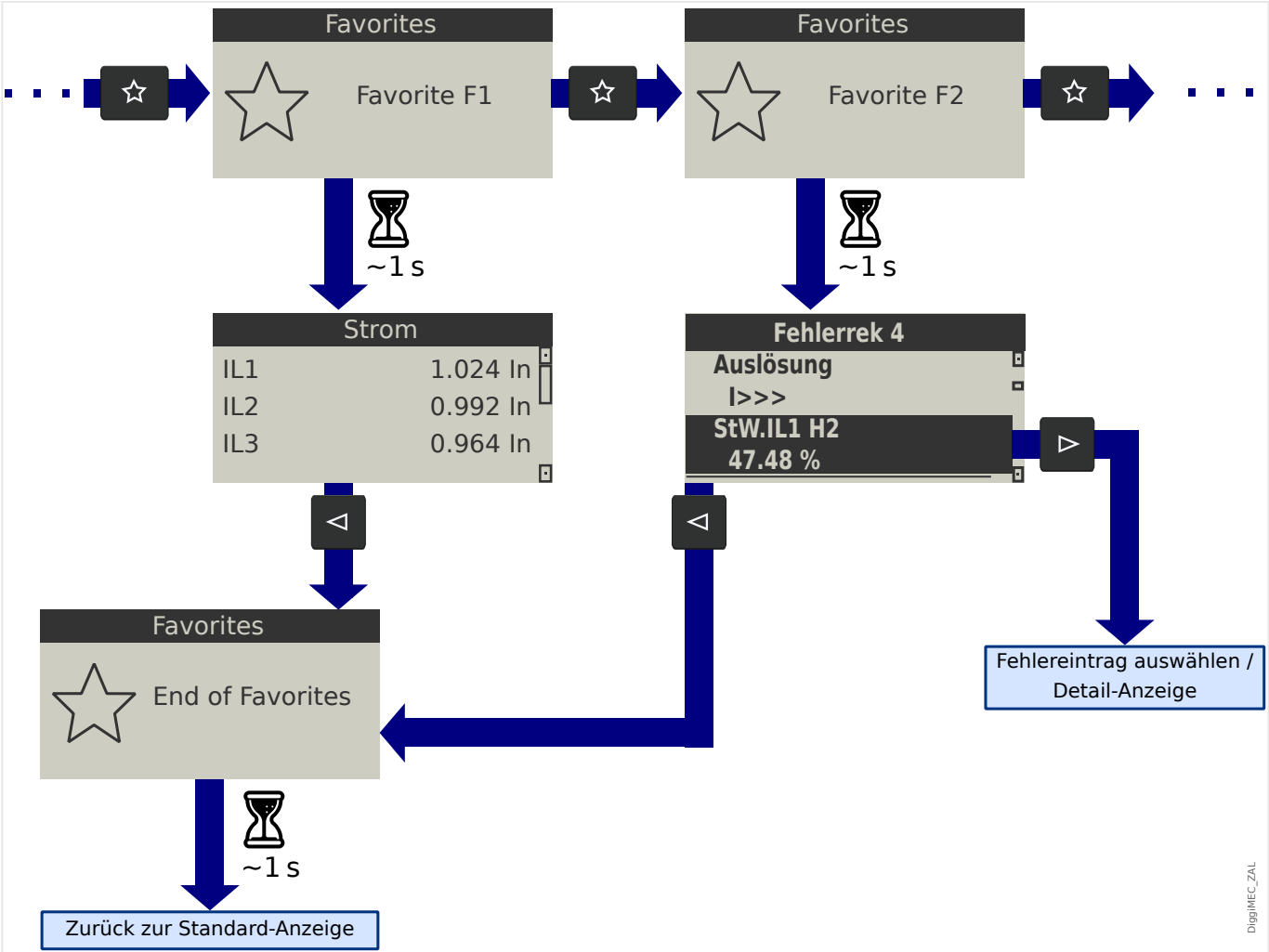
Abb. 8: Prinzip der Favoriten-Taste.
