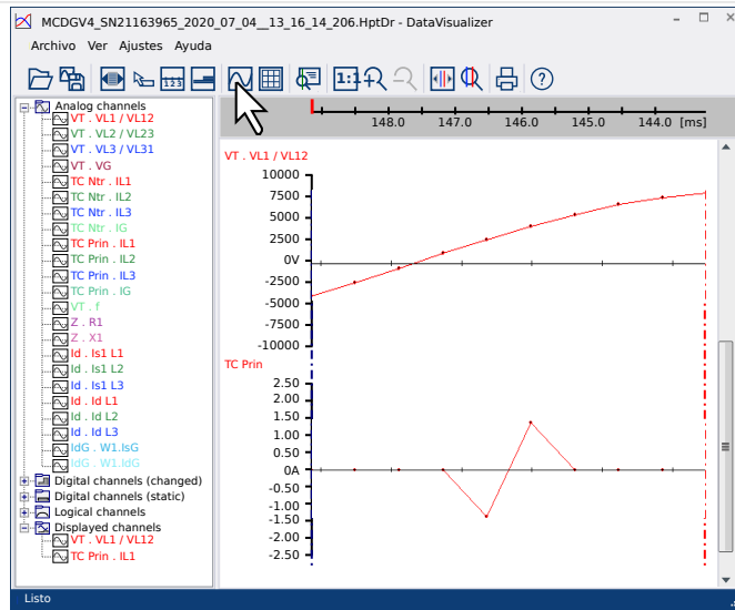
Fig. 9: Marcado de puntos de muestra.
