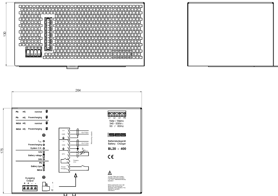
Figura 4.1: Dimensiones
