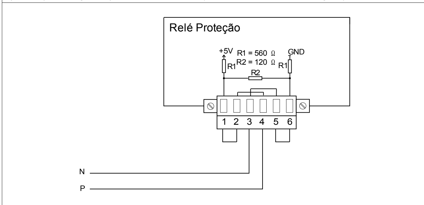
Tipo Exemplo de Fiação, Dispositivo no Final do BUS (usando o Resistor Terminal integrado)
