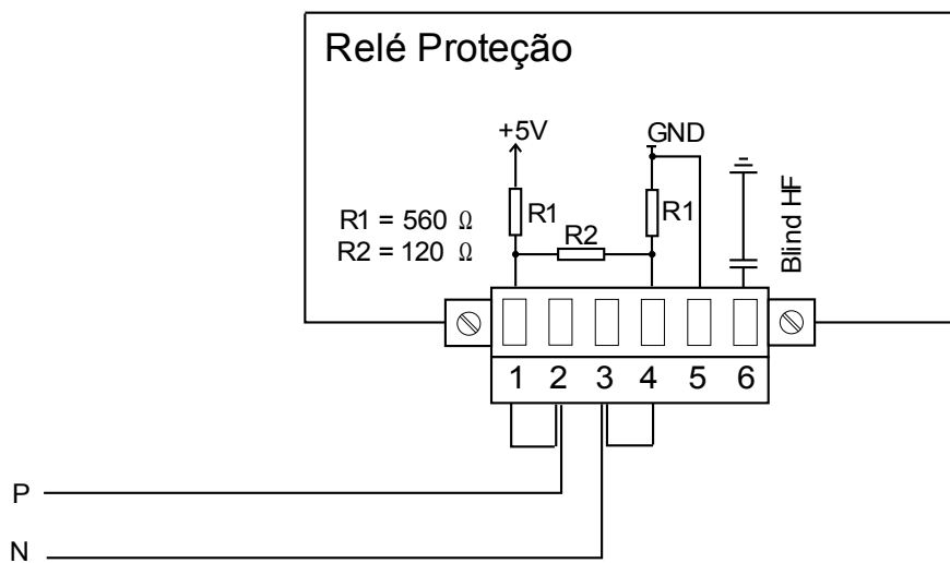
Tipo 2 Exemplo de Fiação, Dispositivo no Final do BUS (usando o Resistor Terminal integrado)
