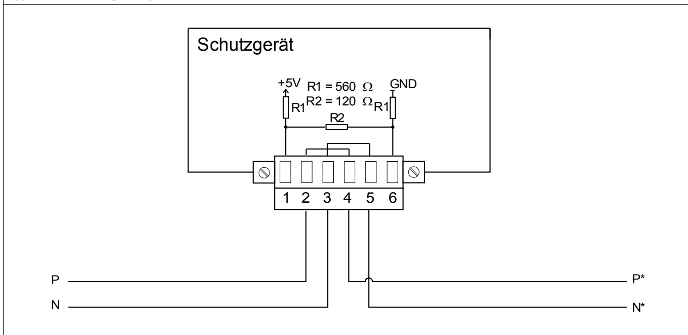
Typ 1 Verdrahtungsbeispiel, Gerät in der Mitte des Busses
