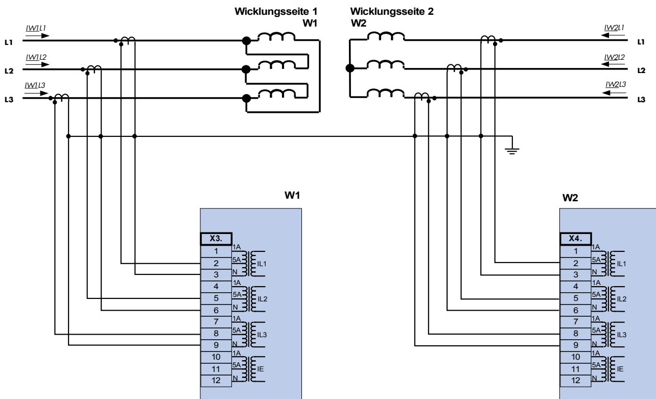
Dreiphasiger Stromwandleranschluss ; In sekundär = 5 A.
