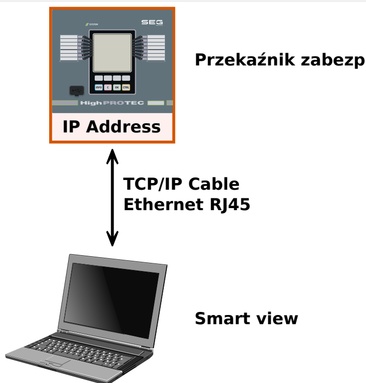
Rys. 2: Parametryzacja i odczyt danych przez TCP/IP.
