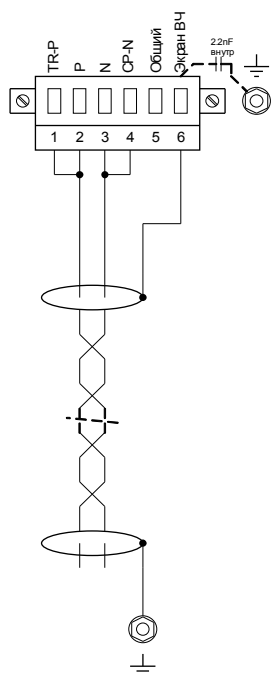
Экранированная оплетка на ведущей стороне шины подключена к согласованному резистору тока на землю
