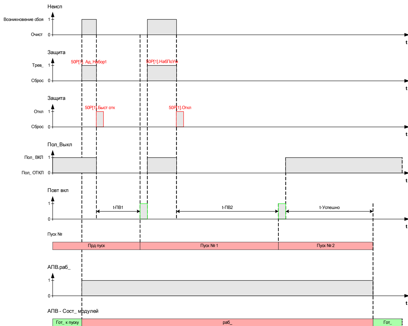
Временная диаграмма автоматического повторного включения для успешной схемы автоматического повторного включения с 2 срабатываниями и ускорением во время предварительного срабатывания
