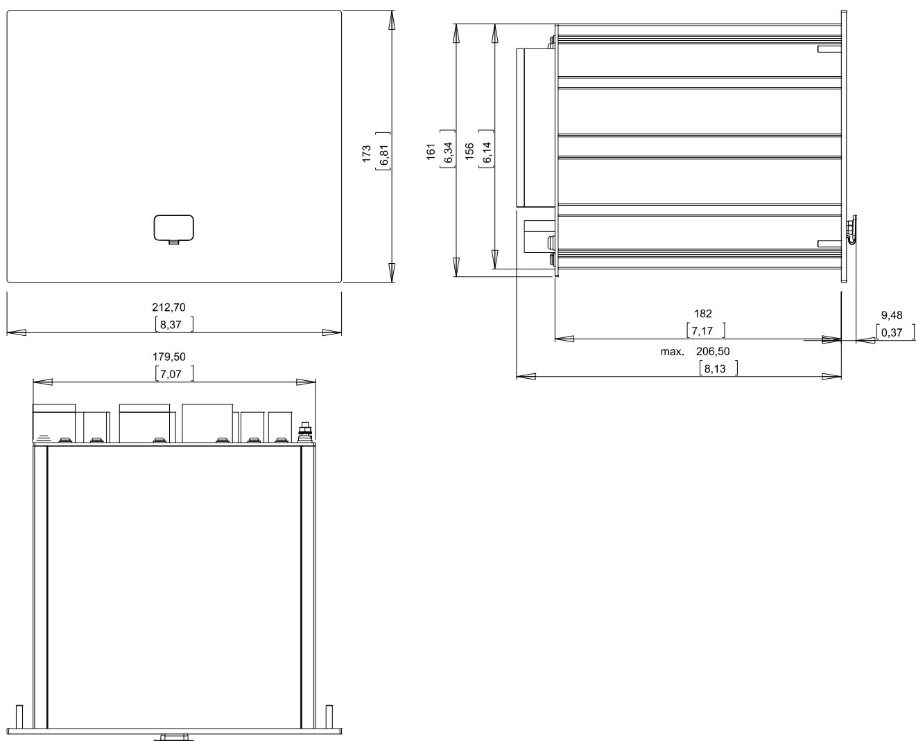
Корпус В2: внешний вид (устройства с 7 кнопками)
