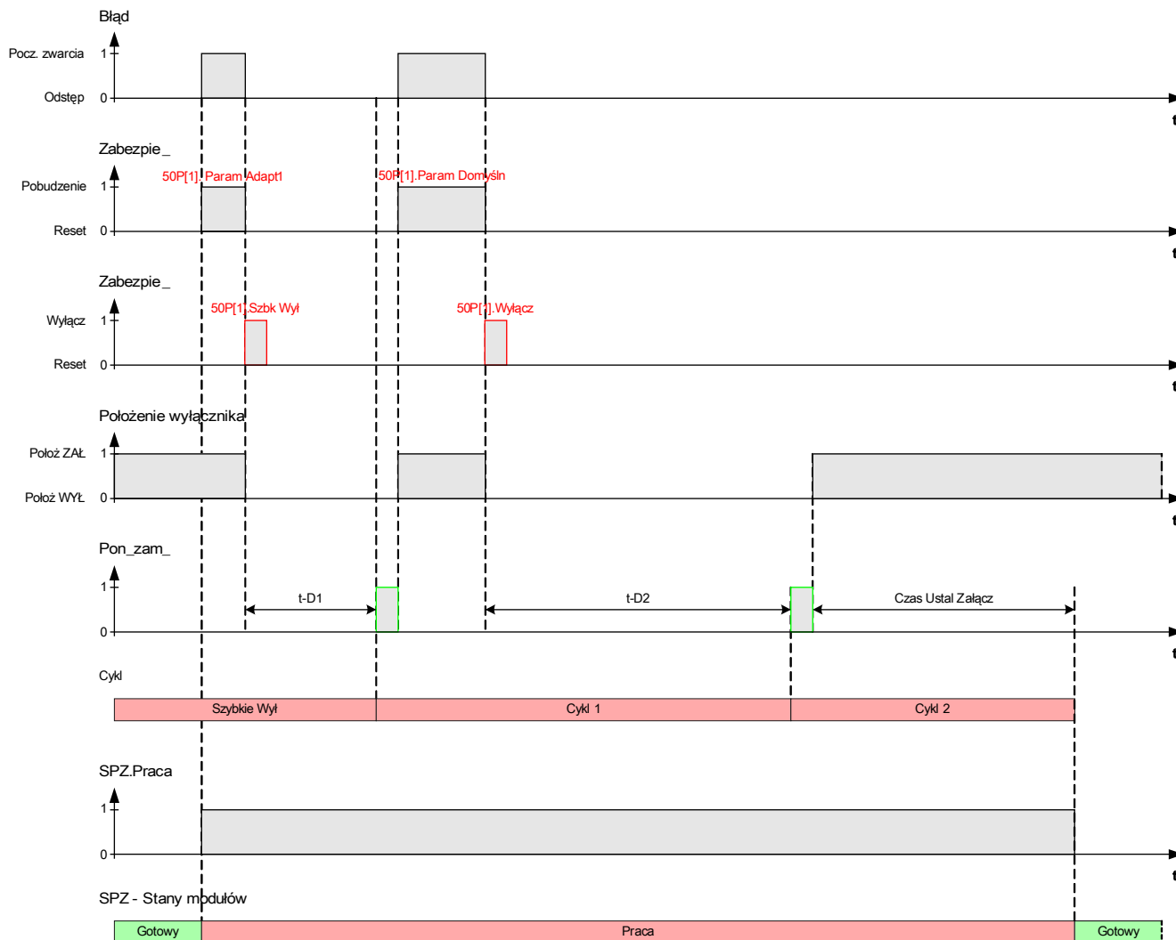
Schemat czasów SPZ dla udanego planu SPZ z 2 próbami i przyspieszeniem przy próbie wstępnej
