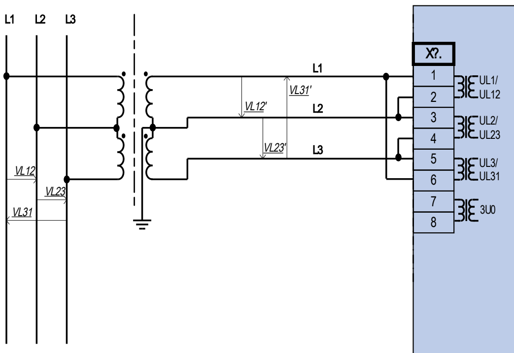
Pomiar napięcia dla dwóch faz w układzie otwartego trójkąta
