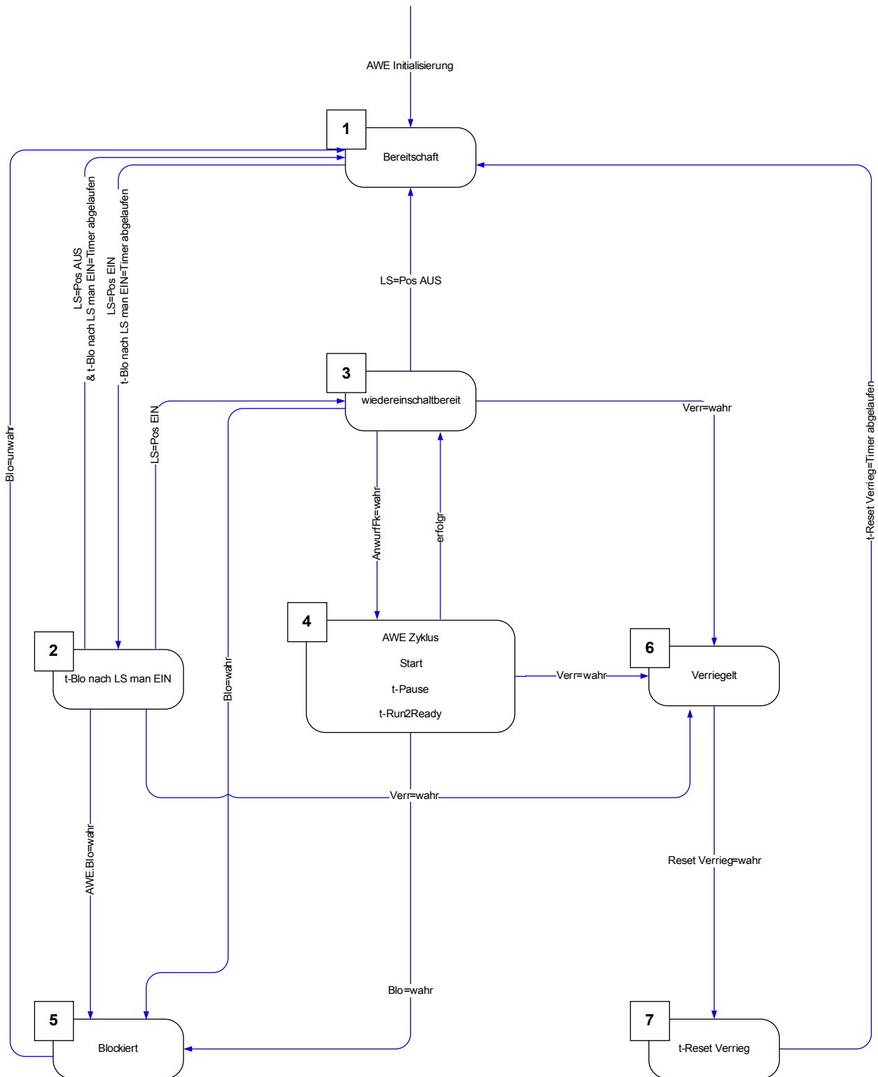
Zustandsdiagramm
