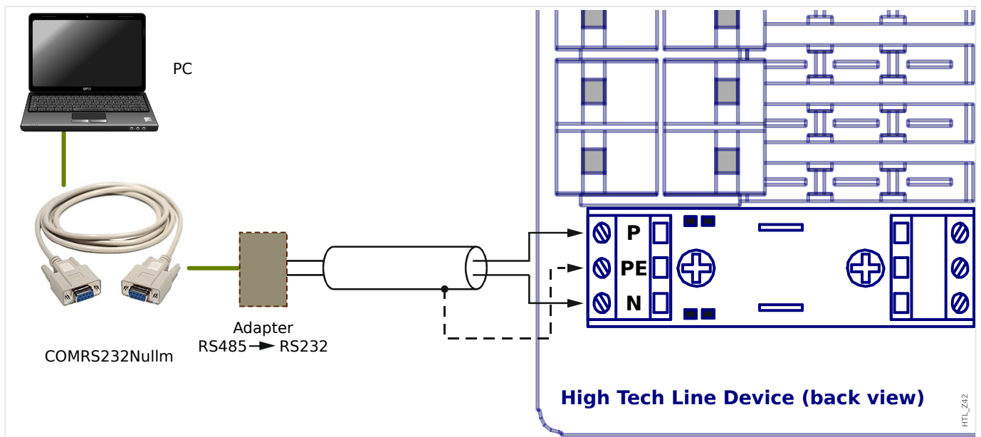
Fig. 3: Conexión de un dispositivo de protección High Tech Line con un PC.
