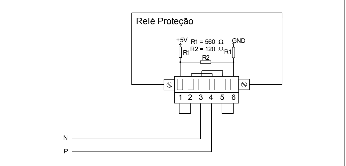
Tipo 1 Exemplo de Fiação, Dispositivo no Final do BUS (usando o Resistor Terminal integrado)
