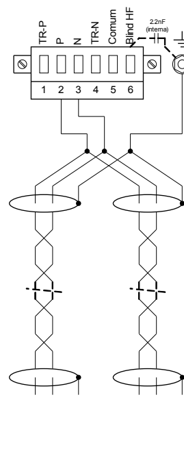
Blindag no lado disposit de barram conectado a resist term terra não usada
