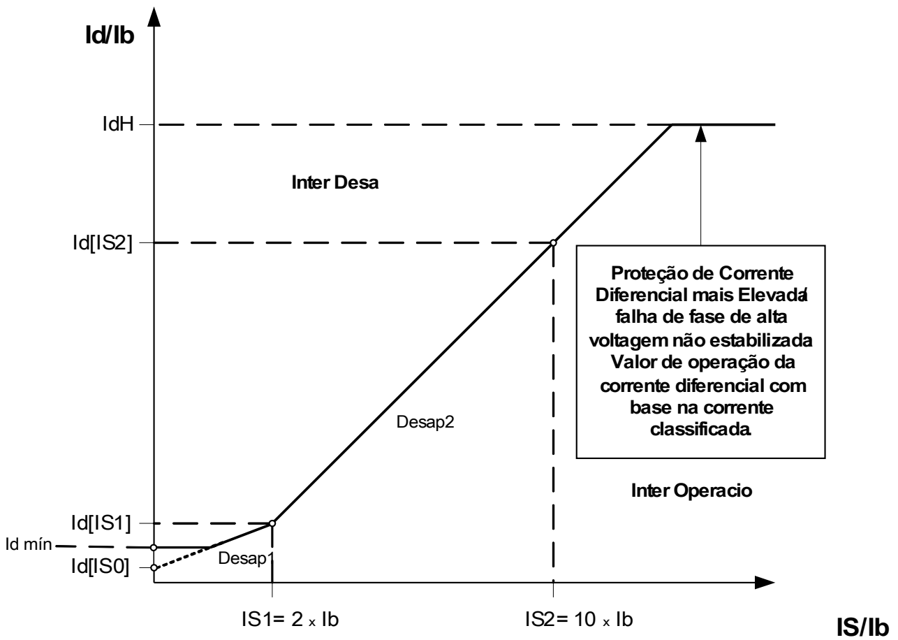
Passo IsH de Proteção Diferencial de Distância Irrestrita
