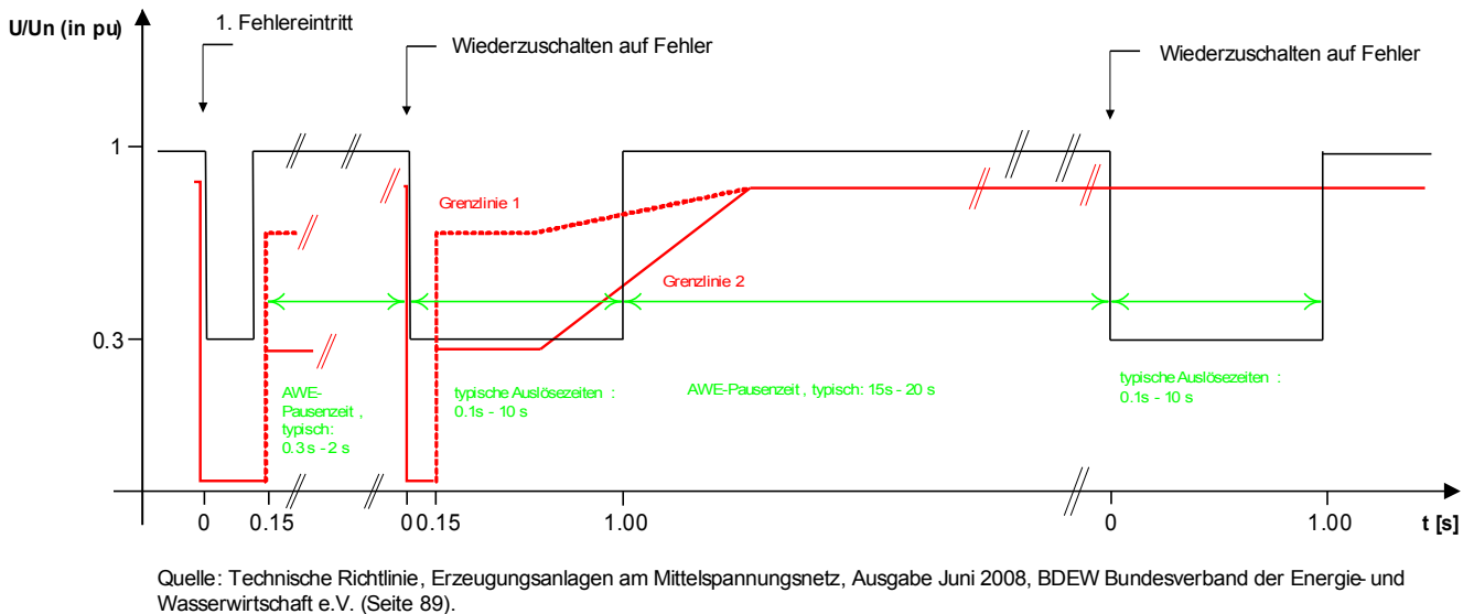
Abbildung: Spannungsverlauf während einer zweischüssigen, nicht erfolgreichen AWE
