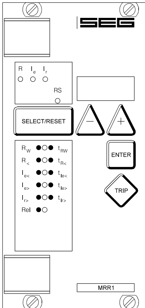
Figura 3.2: Placa frontal
