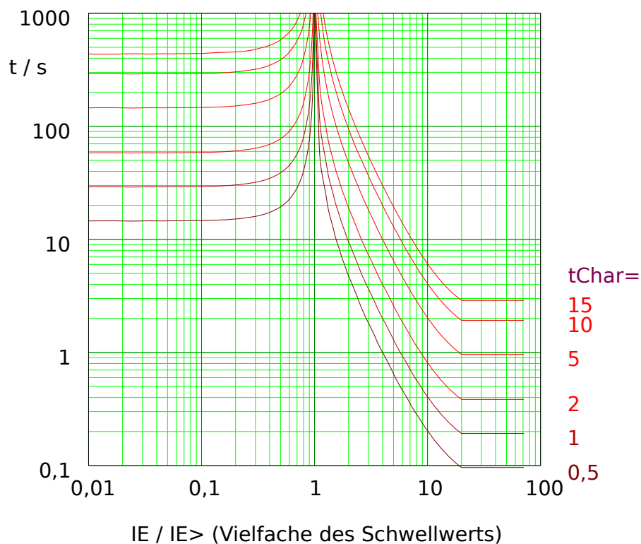
Abb. 71: EINV: Rückfallverzögerung (linke Hälfte, IE < IE_{>} ) und Auslöseverzögerung (rechte Hälfte, IE > IE_{>} ), Beispieldiagramm für I_{max} = 20 \cdot IE_{>} .
