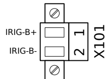
Abb. 29: IRIG-B00X - Elektromechanische Zuordnung.
