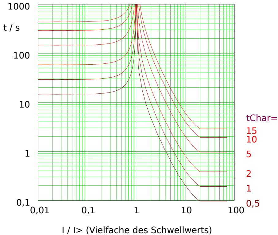
Abb. 59: EINV: Rückfallverzögerung (linke Hälfte, I < I_{>} ) und Auslöseverzögerung (rechte Hälfte, I > I_{>} ), Beispieldiagramm für I_{max} = 20 \cdot I_{>} .
