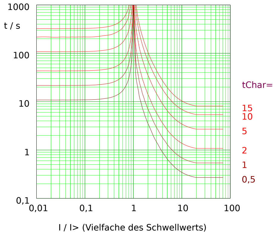
Abb. 58: VINV: Rückfallverzögerung (linke Hälfte, I < I_{>} ) und Auslöseverzögerung (rechte Hälfte, I > I_{>} ), Beispieldiagramm für I_{max} = 20 \cdot I_{>} .
