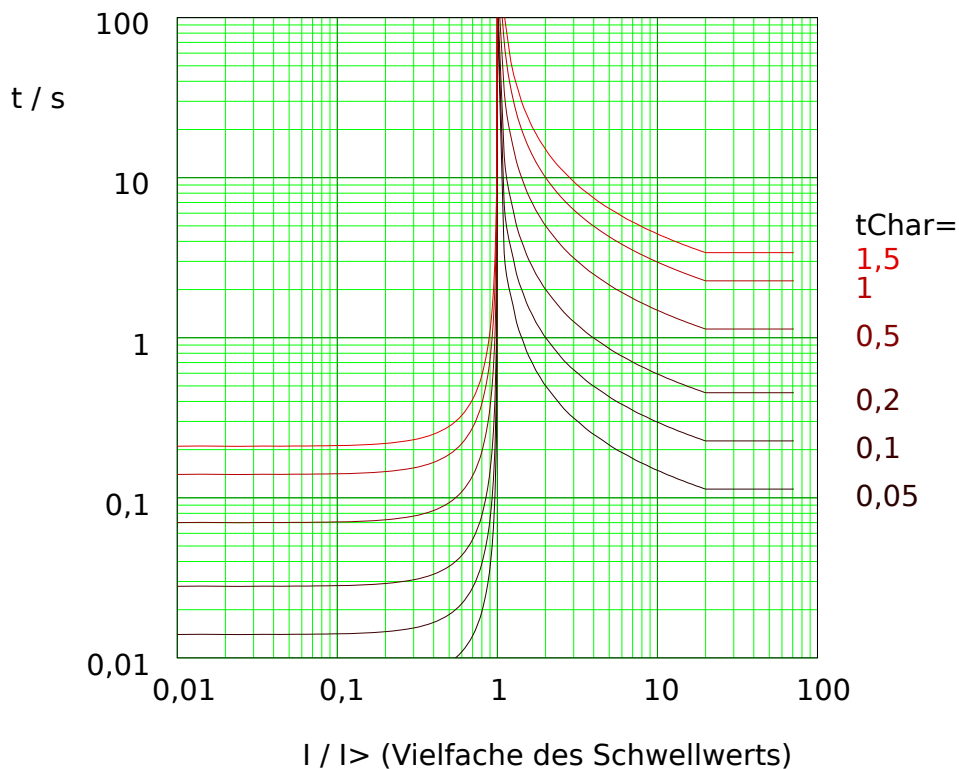
Abb. 52: NINV: Rückfallverzögerung (linke Hälfte, I < I_{>} ) und Auslöseverzögerung (rechte Hälfte, I > I_{>} ), Beispieldiagramm für I_{max} = 20 \cdot I_{>} .
