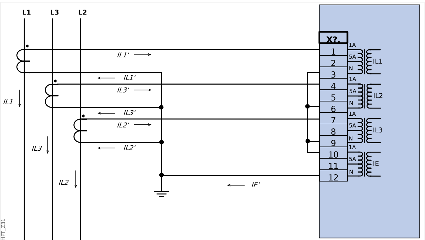
Abb. 25: Dreiphasiger Stromwandleranschluss; In sekundär = 1 A. Erdstromerfassung über Holmgrenschtaltung IEn sekundär = 1 A.
