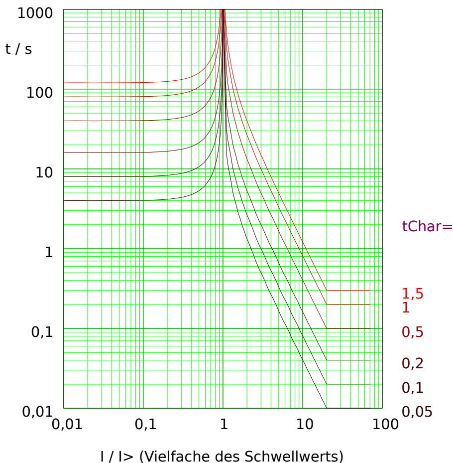
Abb. 54: EINV: Rückfallverzögerung (linke Hälfte, I < I_{>} ) und Auslöseverzögerung (rechte Hälfte, I > I_{>} ), Beispieldiagramm für I_{max} = 20 \cdot I_{>} .
