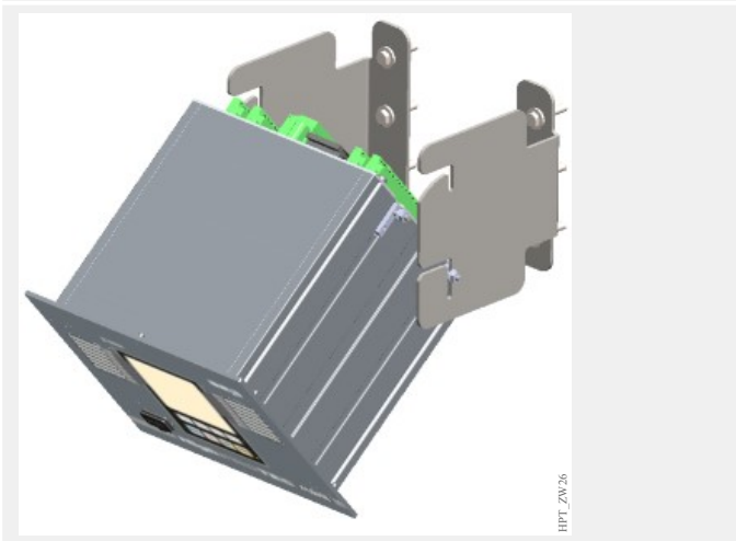
Abkippen des HighPROTEC zur Montageposition
