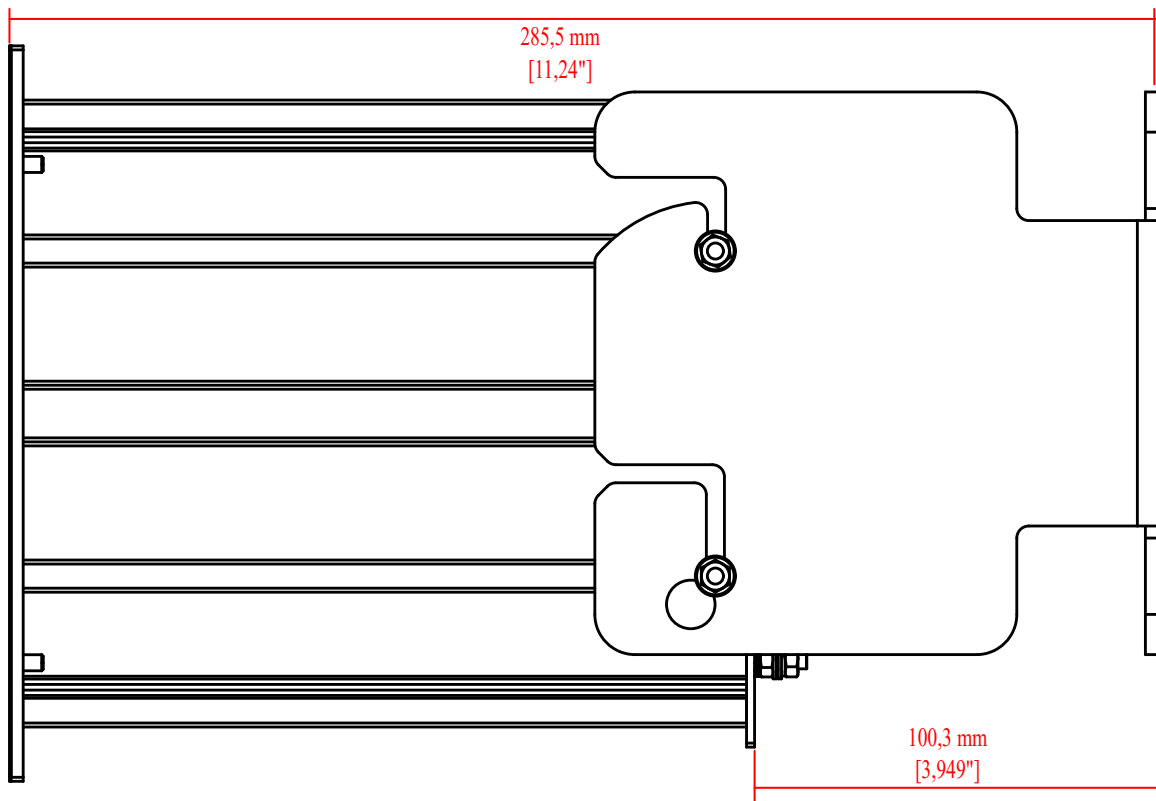
Abb. 8: Ansichten mit Abmessungen für Gehäusegröße B1 (Hinter- und Seitenansicht).
