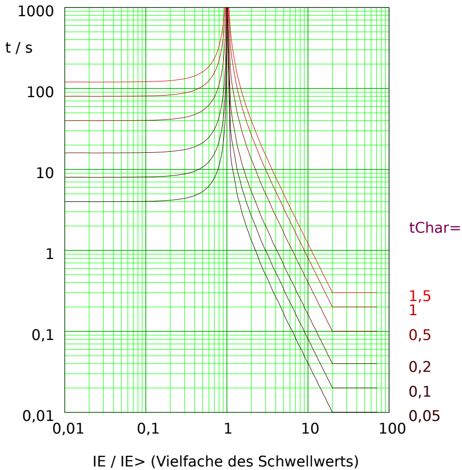
Abb. 66: EINV: Rückfallverzögerung (linke Hälfte, IE < I_{E>} ) und Auslöseverzögerung (rechte Hälfte, IE > I_{E>} ), Beispieldiagramm für I_{max} = 20 \cdot I_{E>} .
