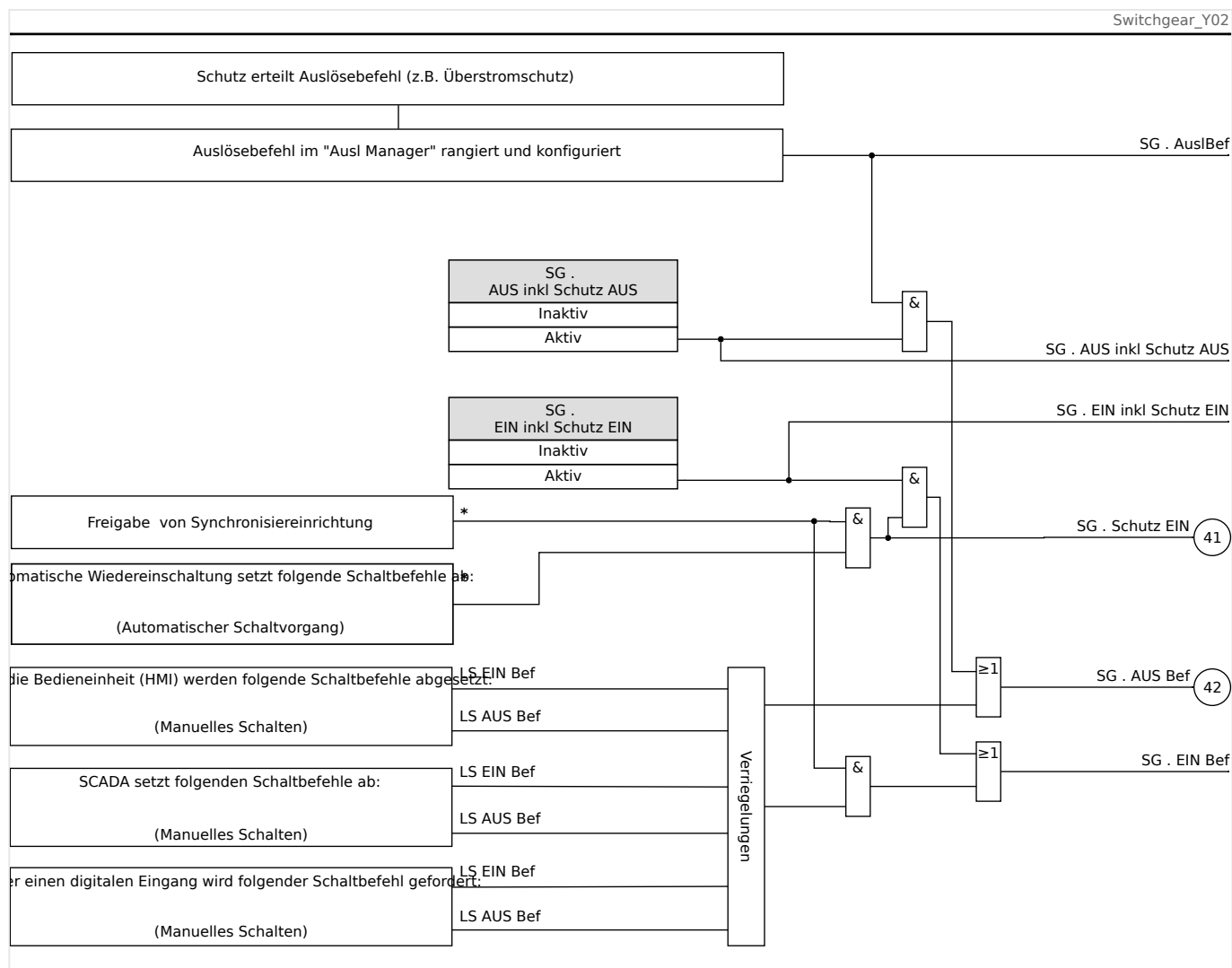
Abb. 97: Verriegelungen. (Für die mit „*“ markierten Teile gilt: Verfügbarkeit hängt von der bestellten Gerätevariante ab.)
