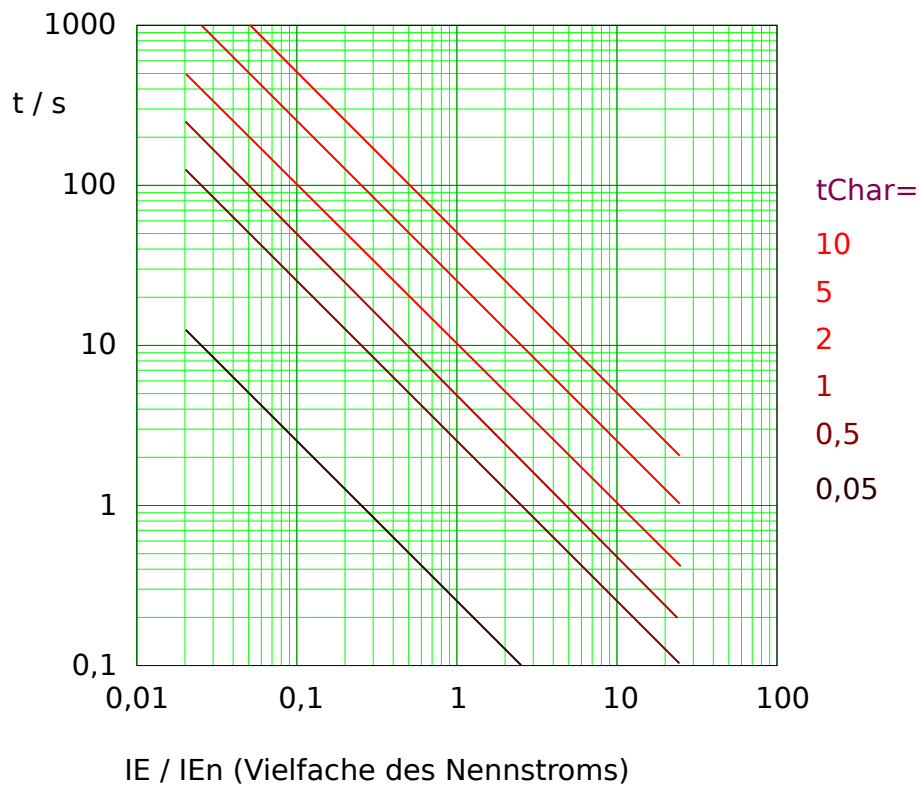
Abb. 74: Auslösekurve „IT“, wobei nur der Bereich IE > I_{E>} jeweils anwendbar ist. Beispieldiagramm für gemessenen (nicht empfindlichen) Erdstrom.
