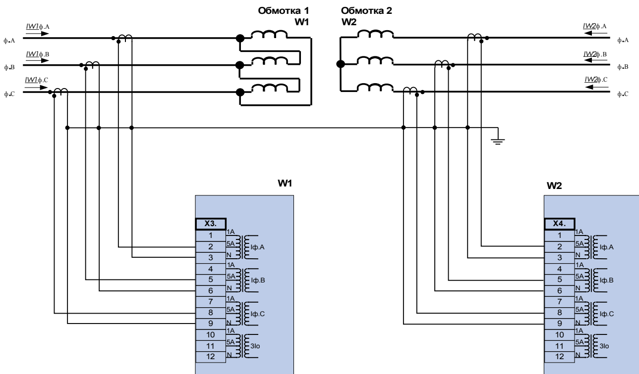
Измерение фазных токов по схеме «полной» звезды; In вторичн. = 5 А.
