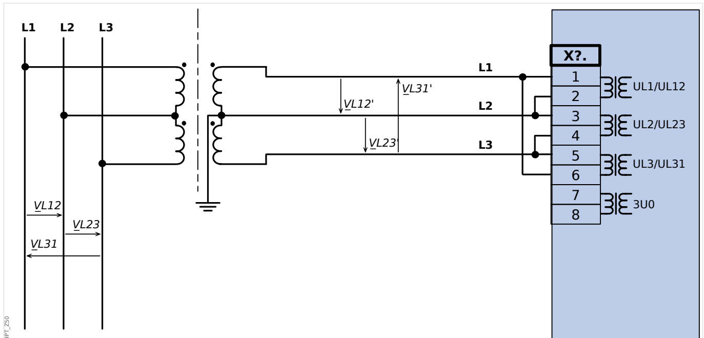
Rys. 21: Pomiar napięcia dla dwóch faz w układzie otwartego trójkąta
