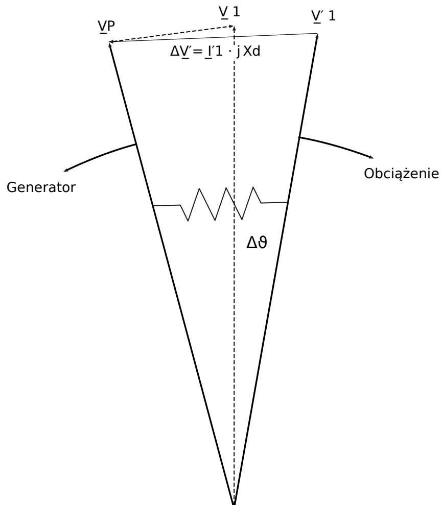
Rys. 48: Wektory napięcia przy awarii sieci.
