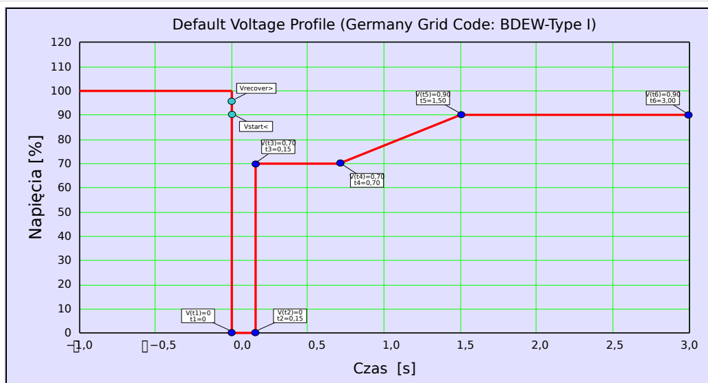
Rys. 58: Profil domyślny LVRT (BDEW typ I).
