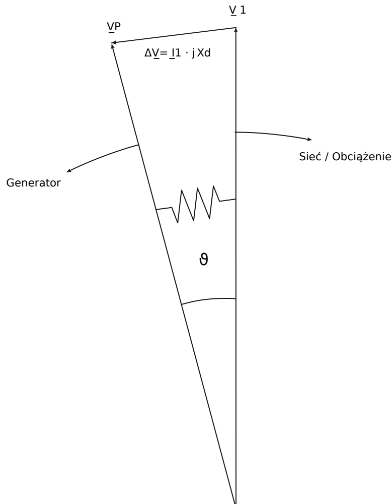
Rys. 46: Wektory napięcia przy pracy równoległej z siecią.
