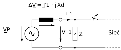
Rys. 47: Schemat zastępczy przy awarii sieci.
