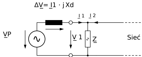
Rys. 45: Schemat zastępczy dla prądnicy synchronicznej pracującej równolegle z siecią.
