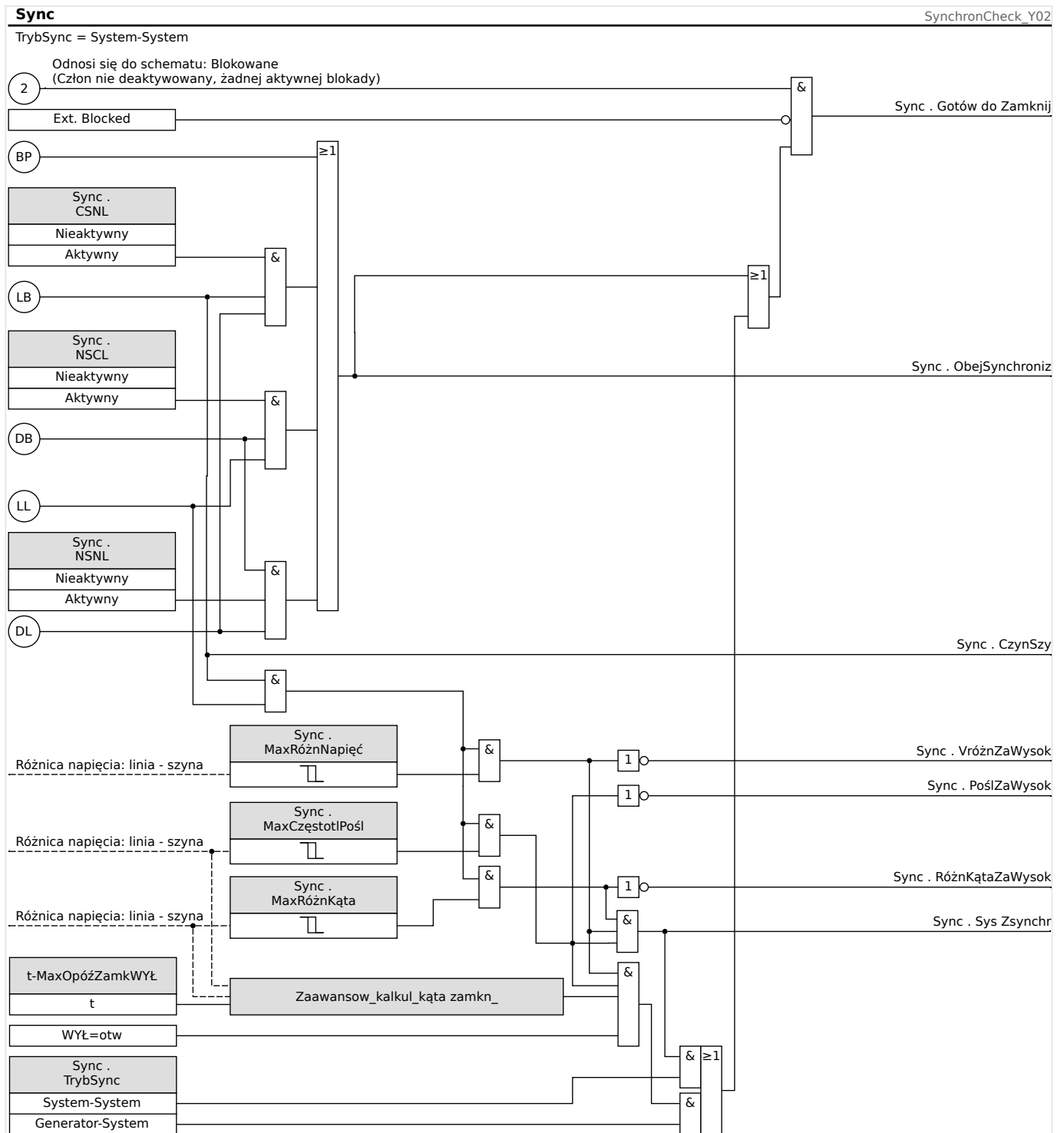
Rys. 54: Działanie modułu „Sync”, „System-System”.
