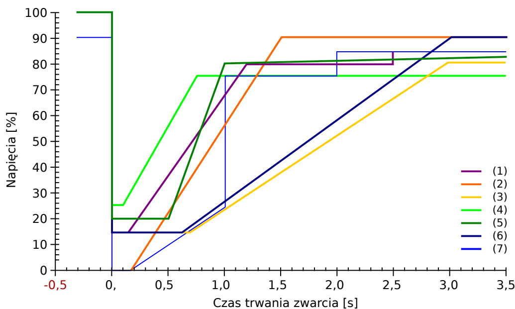
Rys. 55: Normy LVRT; źródło: eBWK Bd. 60 (2008) Nr 4. Autorzy: Dipl.-Ing. Thomas Smolka, Dr.-Ing. Karl-Heinz Weck, Zertifizierungstelle der FGH e.V., Mannheim, sowie Dipl.-Ing. (FH) Matthias Bartsch, Enercon GmbH, Aurich.
