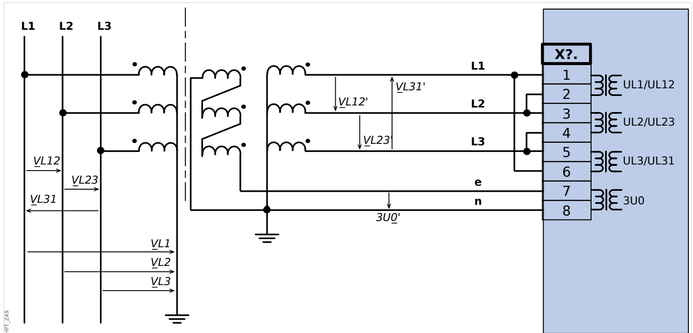
Rys. 20: Trójfazowy pomiar napięcia w układzie trójkąta: połączenie przewodów wejść pomiarowych: "połączenie w trójkąt" Pomiar 3U_0 napięcia szczytkowego poprzez dodatkowe uzwojenia (e-n) w układzie otwartego trójkąta
