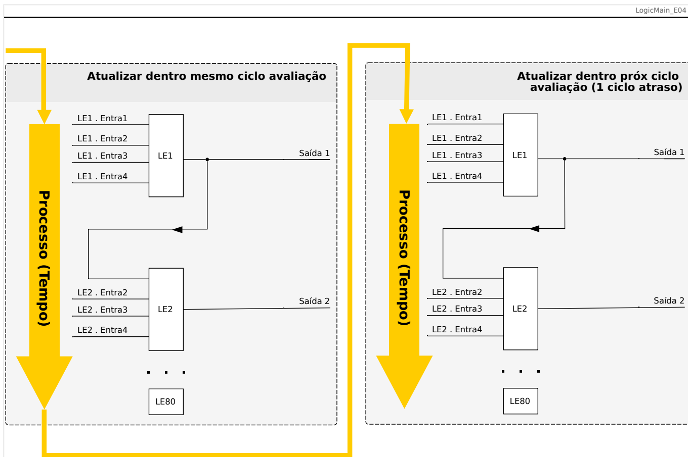
Fig. 76: Em cascata crescente.
