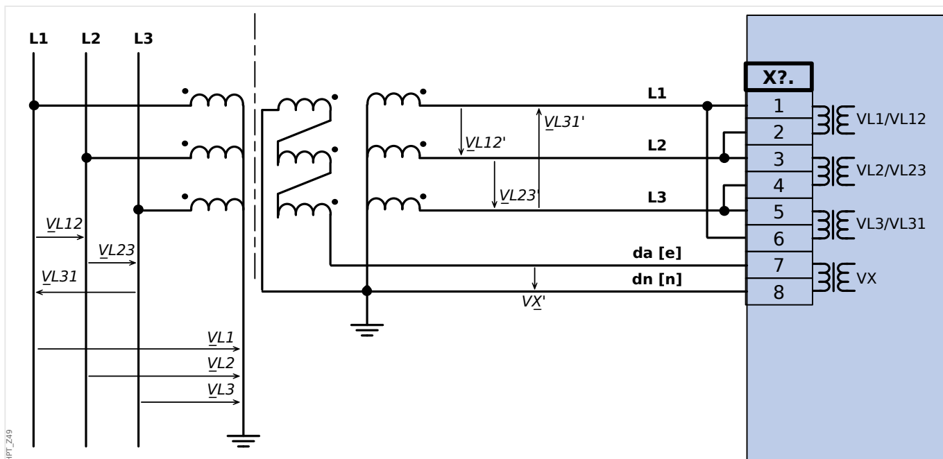
Fig. 20: Medição VG tensão residual por meio de "delta aberto" (e-n) de circuito auxiliar
