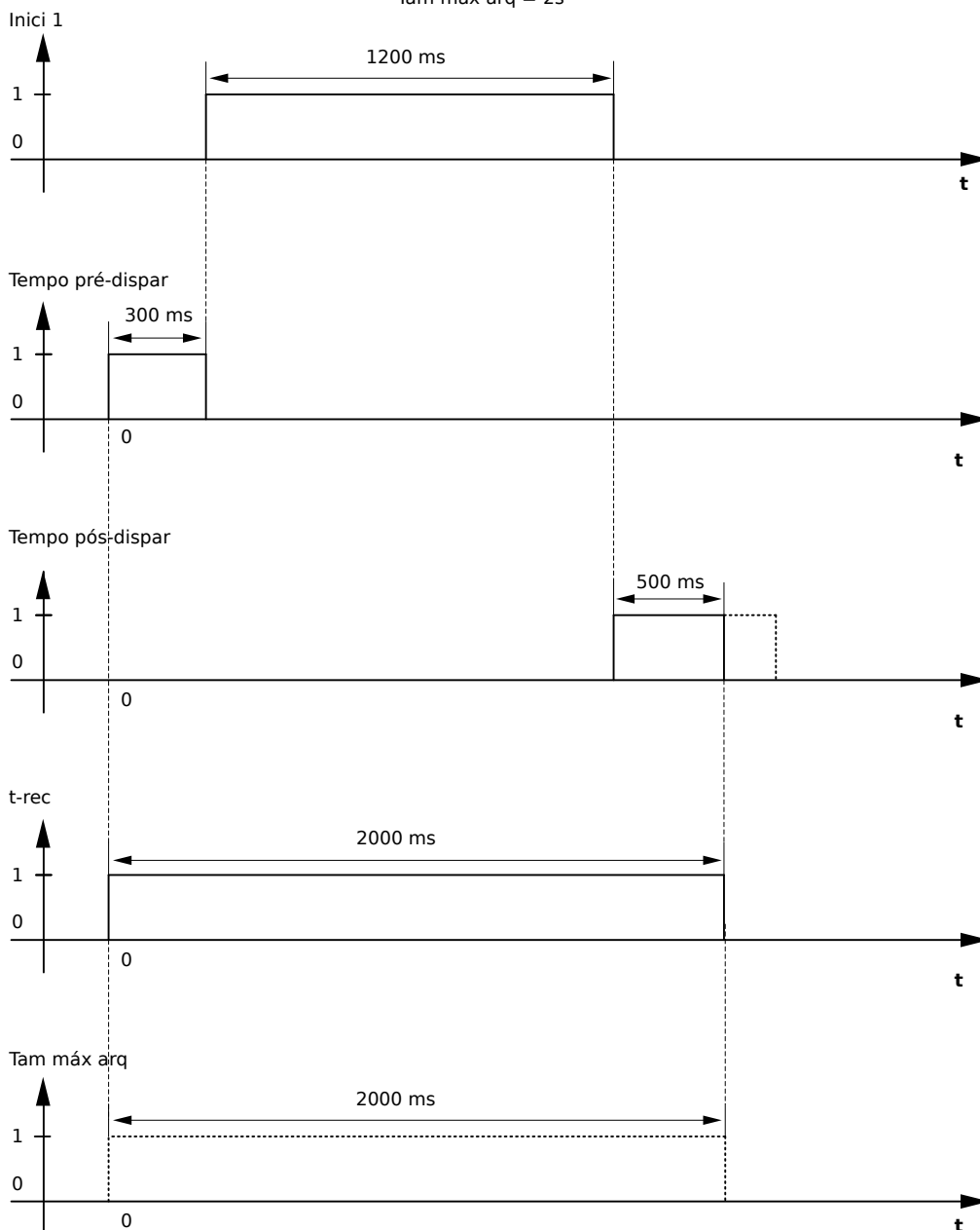
Fig. 70: Exemplo de Gráfico de Prazo do Gravador de Perturbação I
