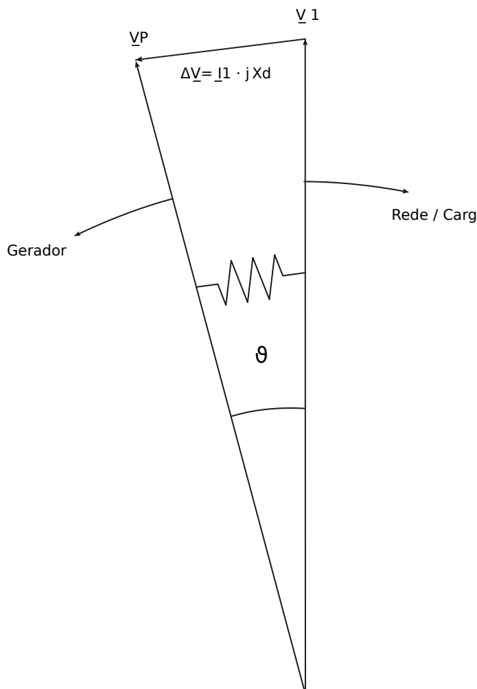
Fig. 47: Vetores de voltagem em operação paralela.
