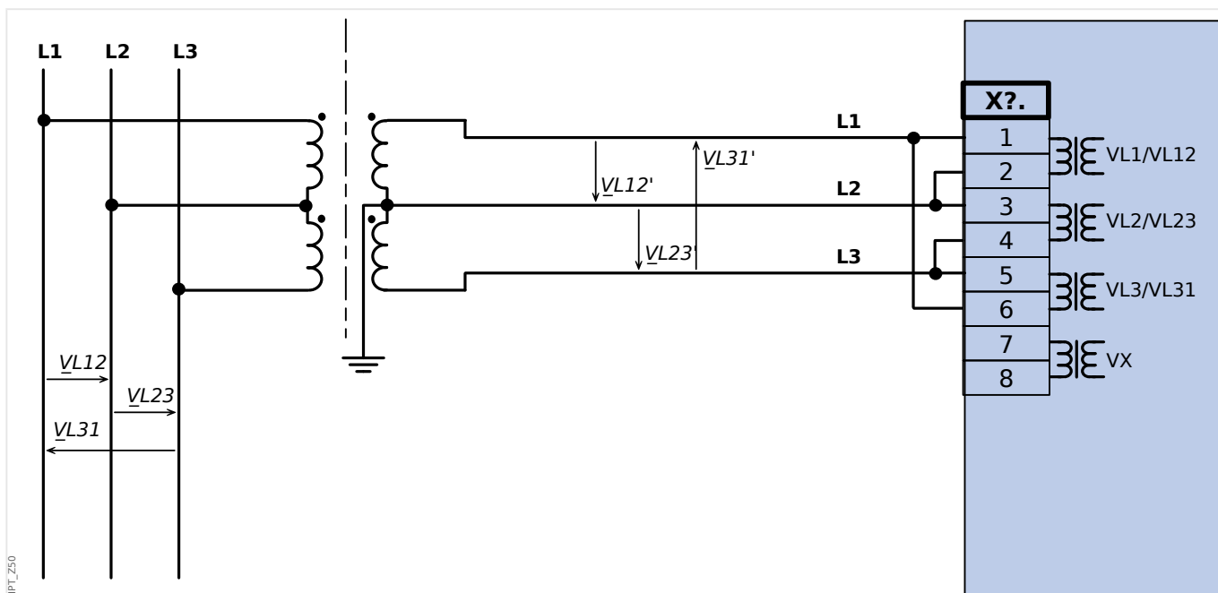
Fig. 21: Medição de tensão bifásica - fiação das entradas de medição: "Delta Aber"
