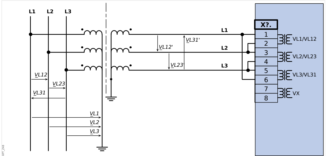
Fig. 19: Medição de tensão trifásica - fiação das entradas de medição: "conexão-delta"
