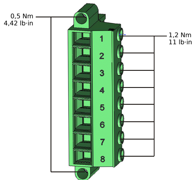
Fig. 80: Terminais de medição de tensão da placa de medição “TU” (↳ “3.5.1 TU - Entradas de Medição de Tensão”).
