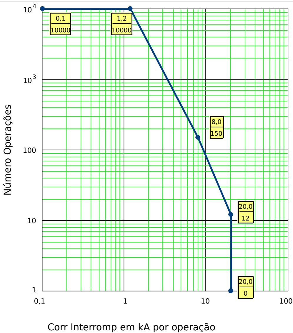
Fig. 69: Curva Manutenção de Disjuntor para Disjuntor normal 25kV
