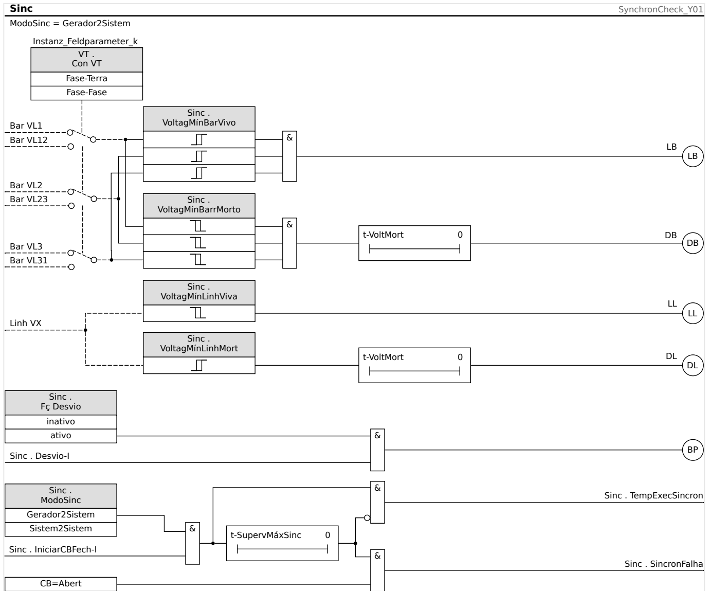
Fig. 54: Funcionalidade do módulo »Sinc«, “Gerador2Sistem”.
