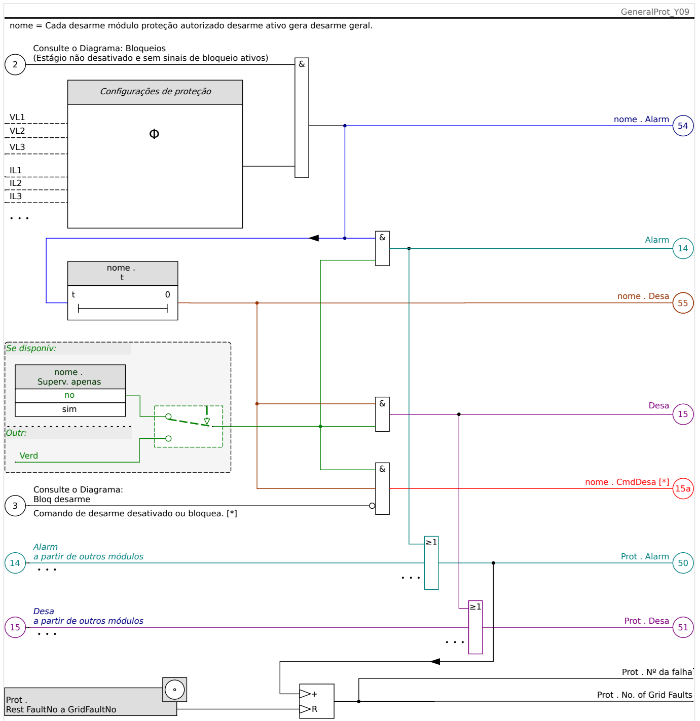
Fig. 40: Esboço rápido da funcionalidade de qualquer HighPROTEC elemento de proteção.
