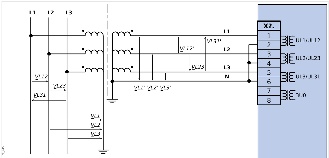
Rys. 17: Przekładnik napięciowy połączony w gwiazdę: Trójfazowy pomiar napięcia w układzie gwiazdy
