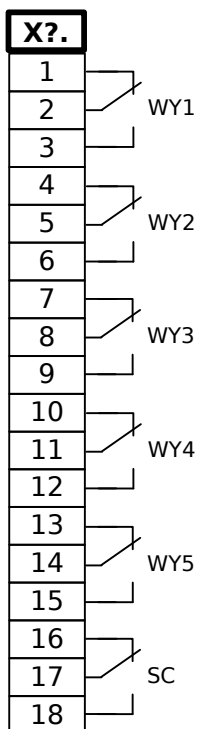
Rys. 12: RO-5 — oznaczenie zacisków
