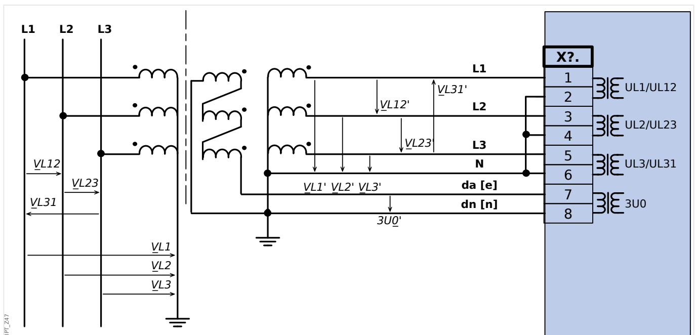
Rys. 18: Przekładnik napięciowy połączony w gwiazdę z otwartym trójkątem.
