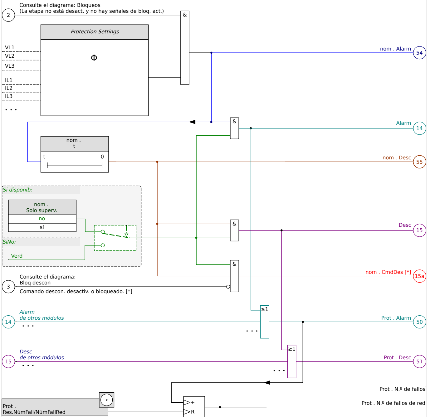
Fig. 40: Descripción a grandes rasgos de la funcionalidad de cualquier elemento de protección de HighPROTEC.
