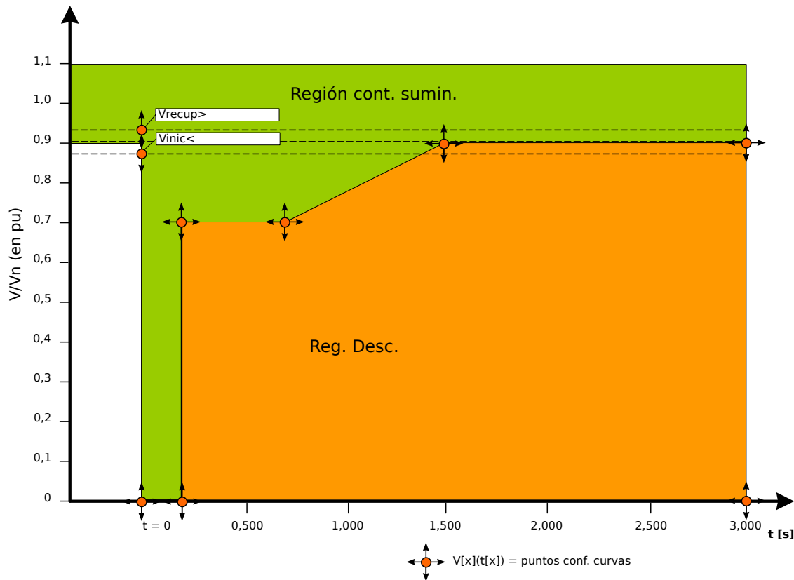
Fig. 58: Regiones de continuidad y desconexión.
