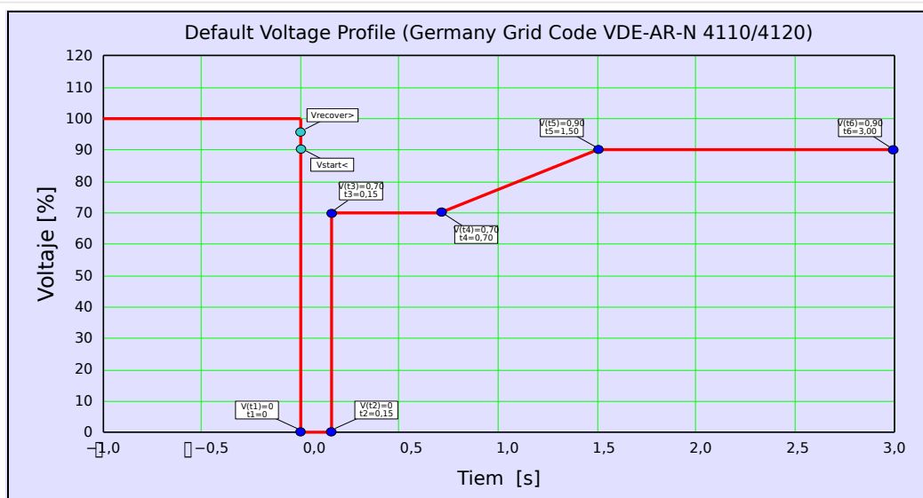
Fig. 59: Perfil de LVRT predeterminado (Tipo I).
