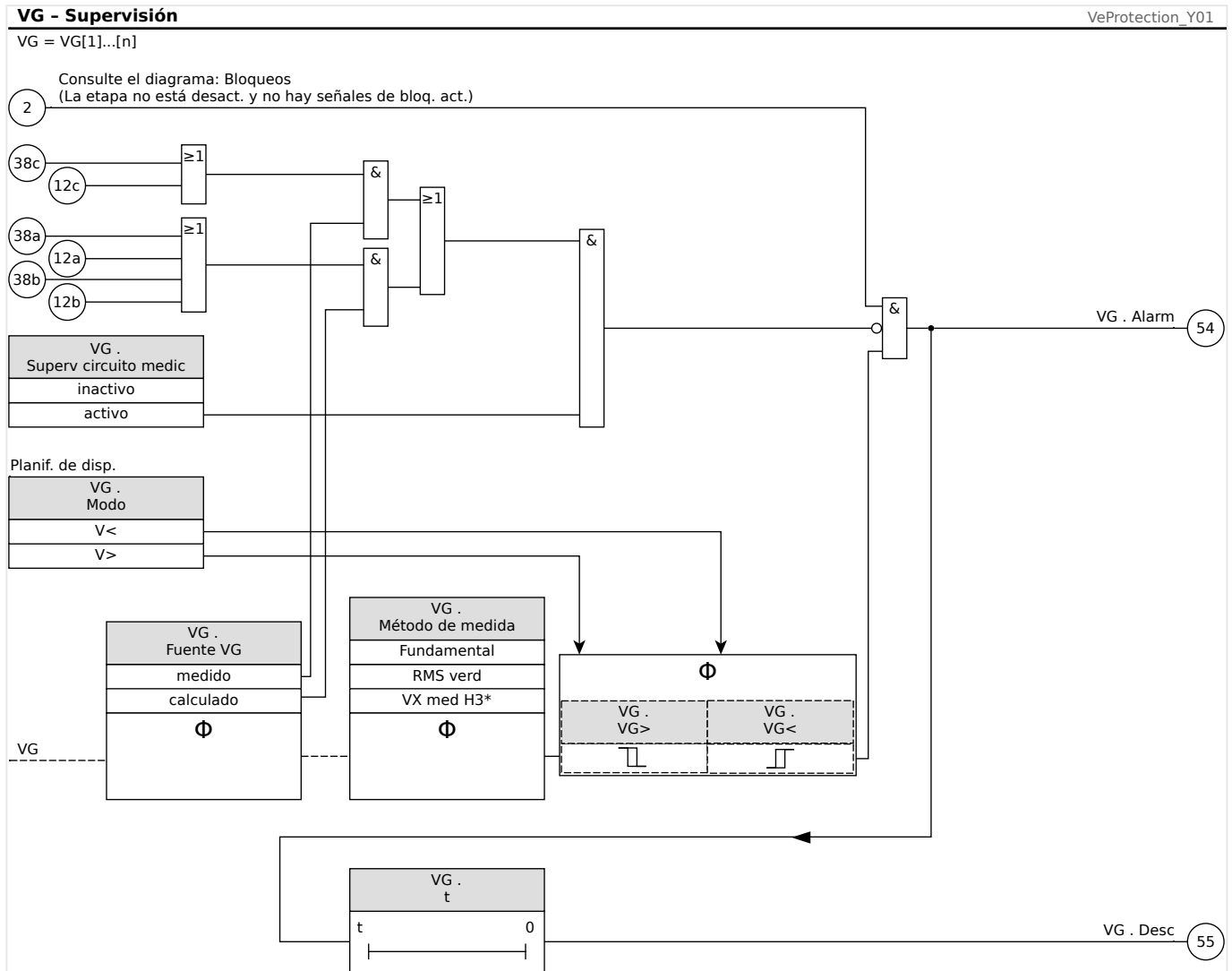
Fig. 44: VG, VX Supervisión de tensión, parte 1 (función de supervisión, decisión de desconexión).
