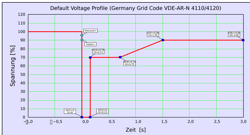
Abb. 60: LVRT-Werkseinstellung (Typ I).
