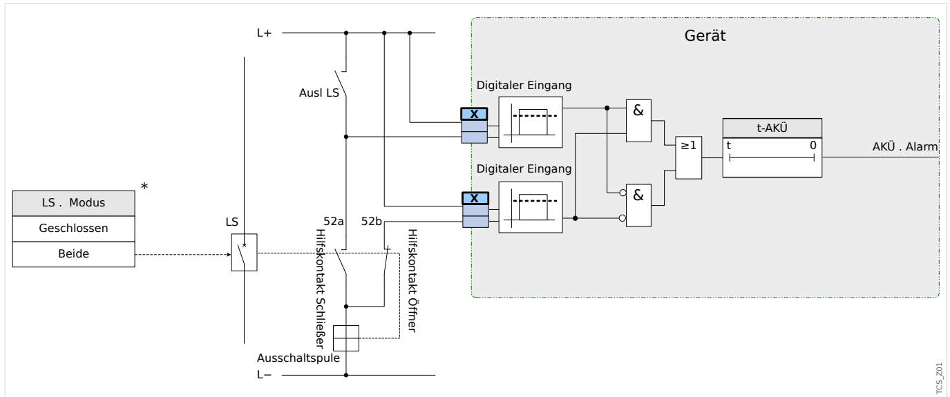
Abb. 62: Anschlussbeispiel (Empfehlung): Auslösekreisüberwachung mit zwei Hilfskontakten »Hiko EIN« (52a) und »Hiko AUS« (52b).
