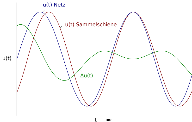
Abb. 53: Spannungsverlauf der Schwebespannung \Delta u(t) , vergrößert.
