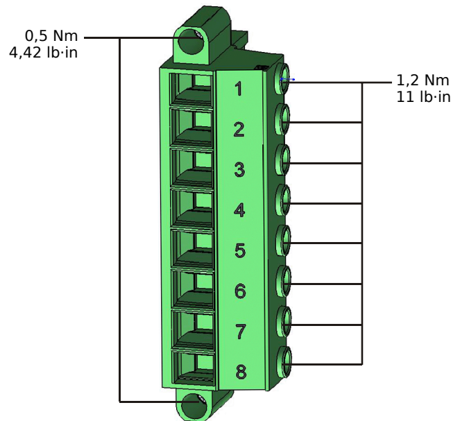
Abb. 82: Spannungsmessstecker der Spannungsmesskarte „TU“ (↳ „3.5.1 TU - Spannungsmesseingänge“).
