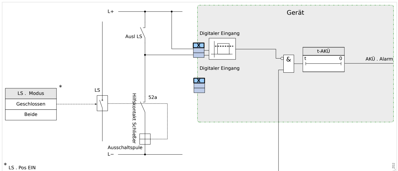
Abb. 63: Anschlussbeispiel: Auslösekreisüberwachung mit einem Hilfskontakt »Hiko EIN« (52a).
