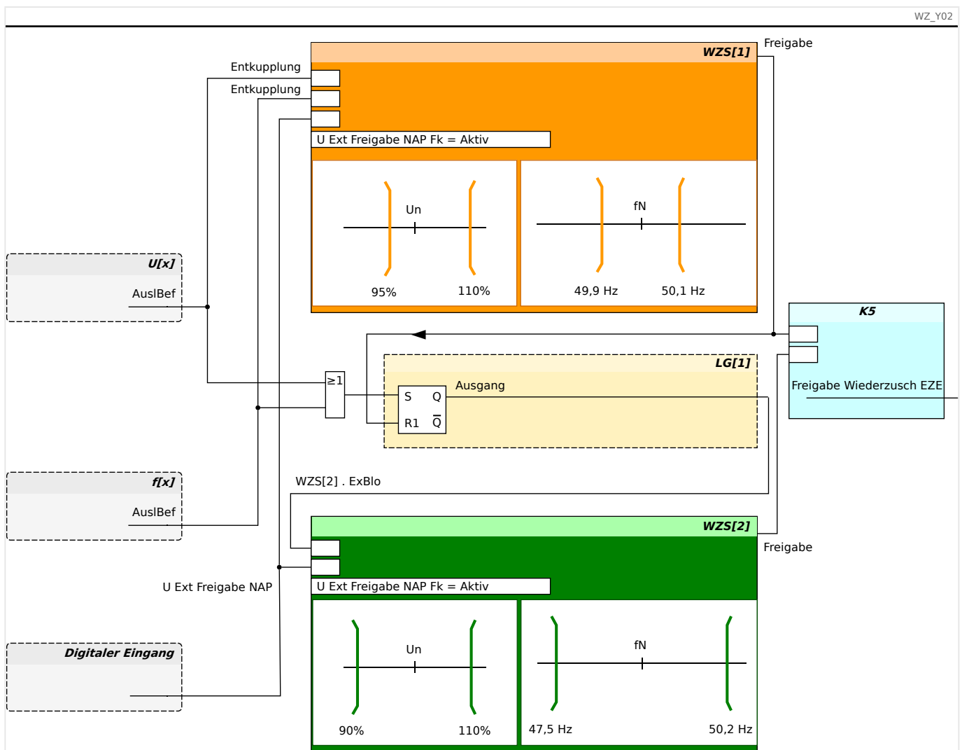
Abb. 56: Applikationsbeispiel für ein Zuschalten in Abhängigkeit von einer vorherigen Schutzauslösung.
