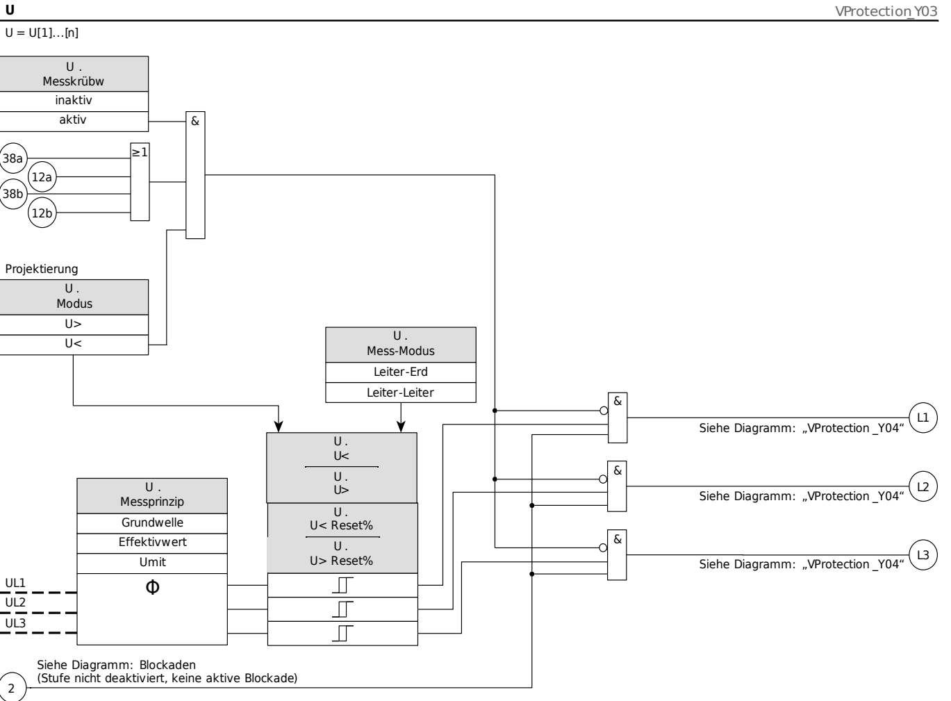
Funktionalität des Spannungsschutzmoduls, Teil 1.
