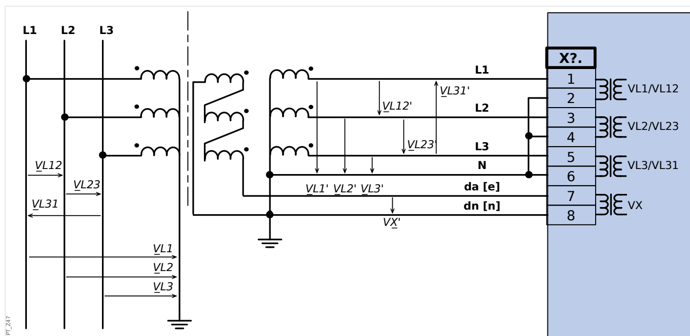
Fig. 18: VT Wye com conexão Broken Delt.
