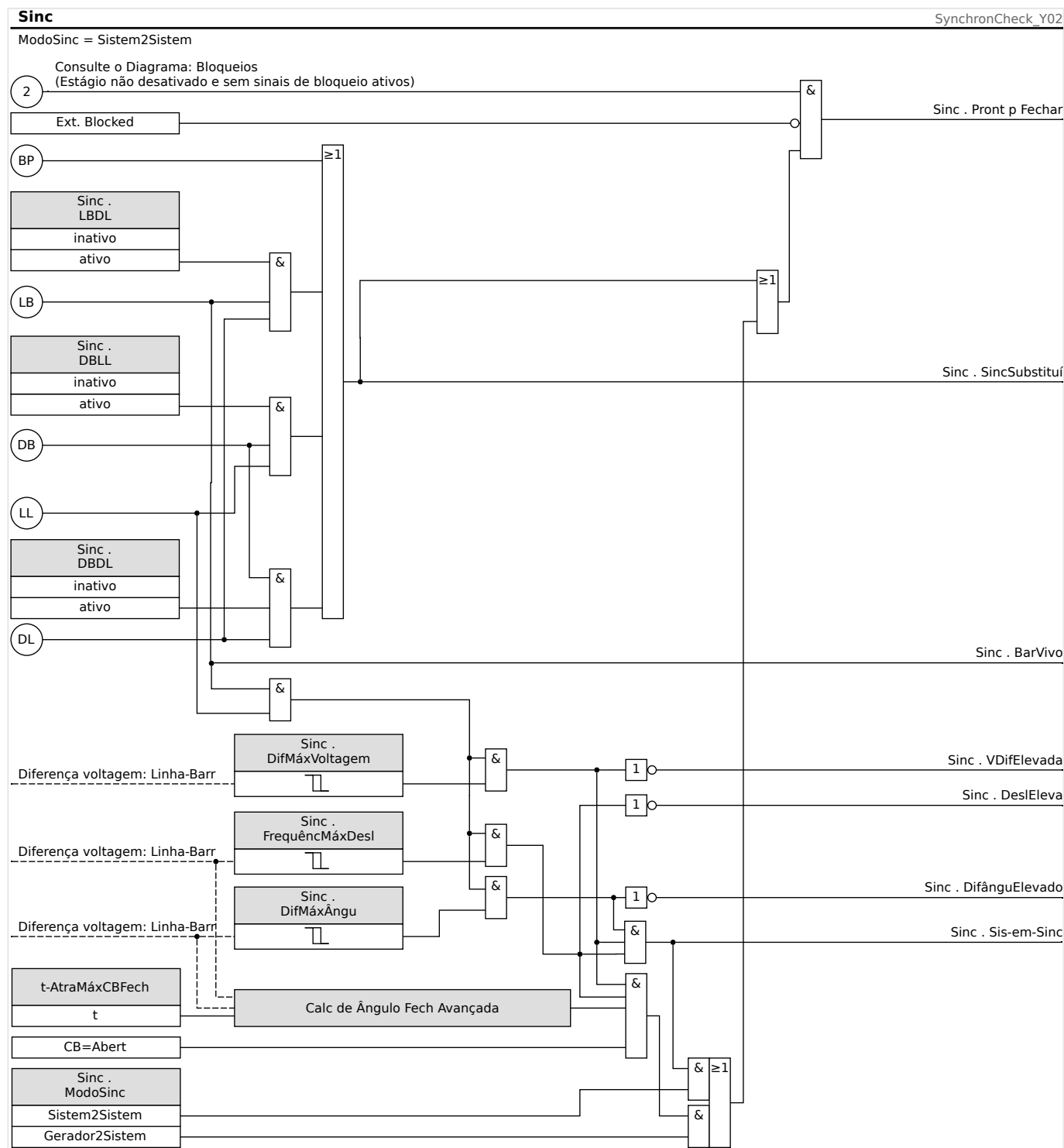
Fig. 55: Funcionalidade do módulo »Sinc«, "Sistem2Sistem".
