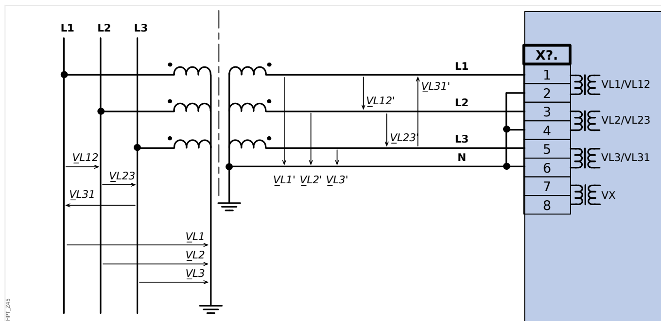
Fig. 17: VT Wye: Medição de voltagem trifásica - fiação das entradas de medição: "conexão estrela"
