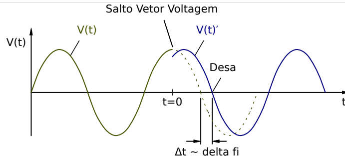
Fig. 50: Aumento de vetor de tensão.
