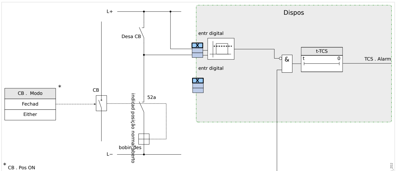
Fig. 62: Exemplo de conexão: Supervisão do circuito de disparo com apenas um contato CB auxiliar »Aux ON« (52a).
