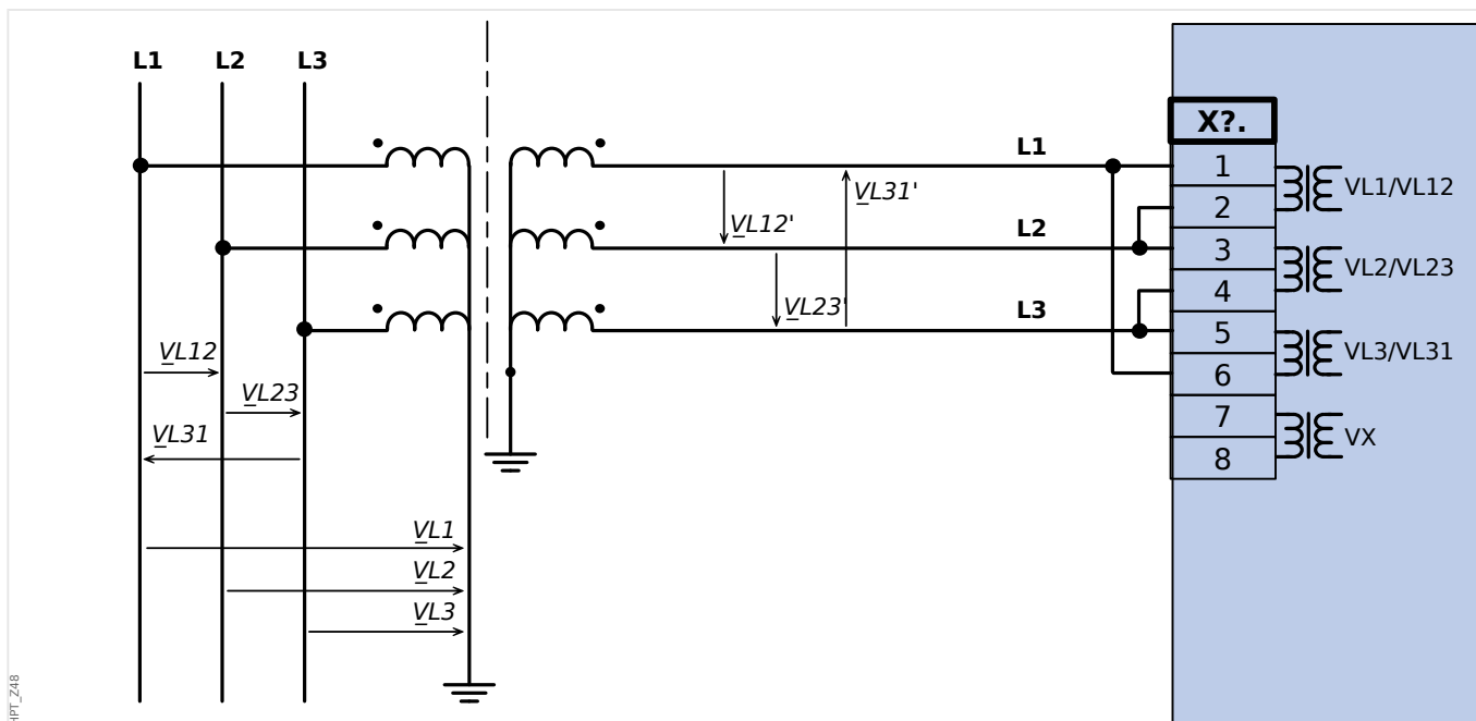
Fig. 19: Medição de tensão trifásica - fiação das entradas de medição: "conexão-delta"
