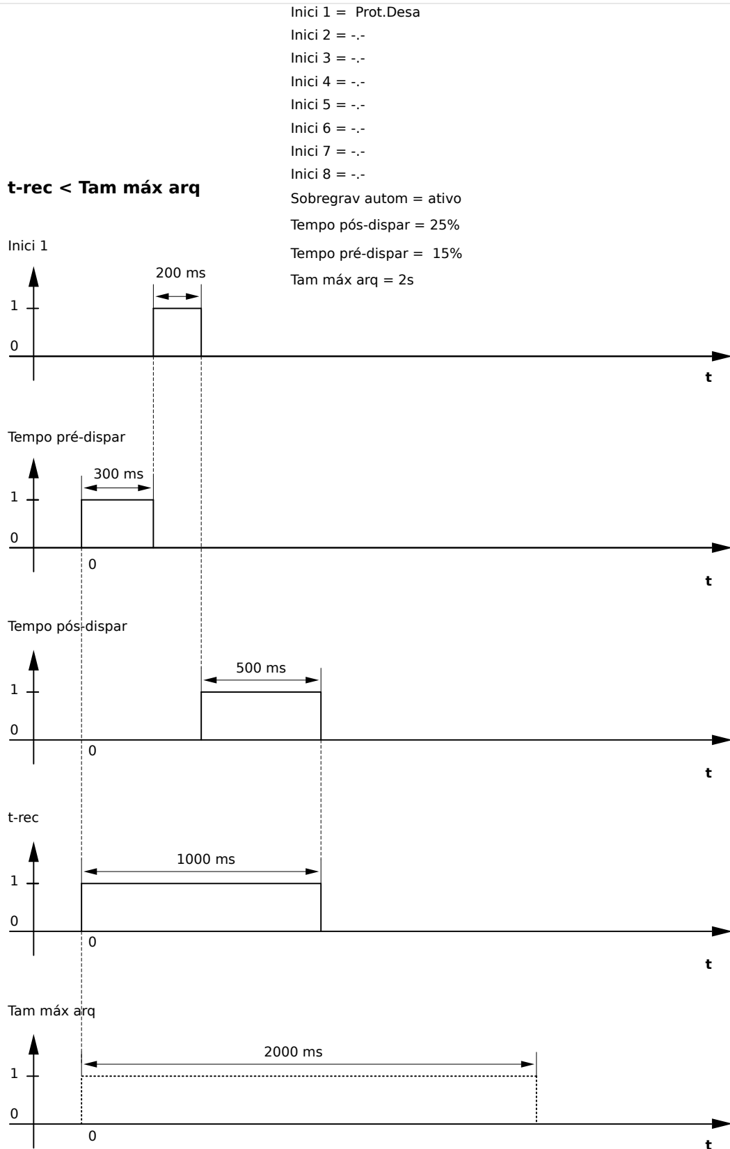
Fig. 71: Exemplo de Gráfico de Prazo do Gravador de Perturbação II
