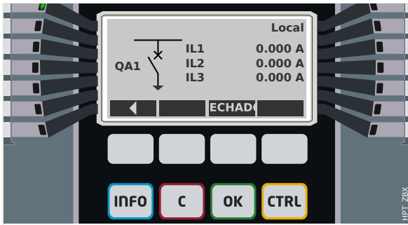
Fig. 66: Exemplo de página de controle, com o "Disjuntor" na posição aberta.
