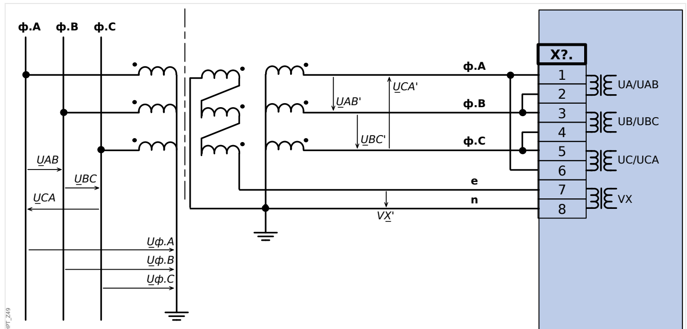
Рис. 20: Измерение трехфазного напряжения - схема измерительных входов: "соединение треугольником" Измерение напряжения нулевой последовательности V_G через вспомогательные обмотки (e-n) («открытый треугольник»)
