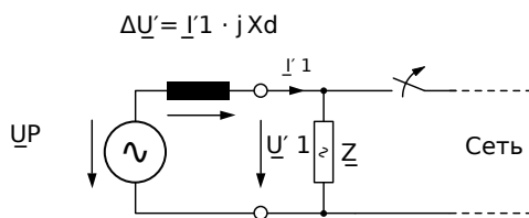
Рис. 47: Эквивалентная цепь при сбое электросети.
