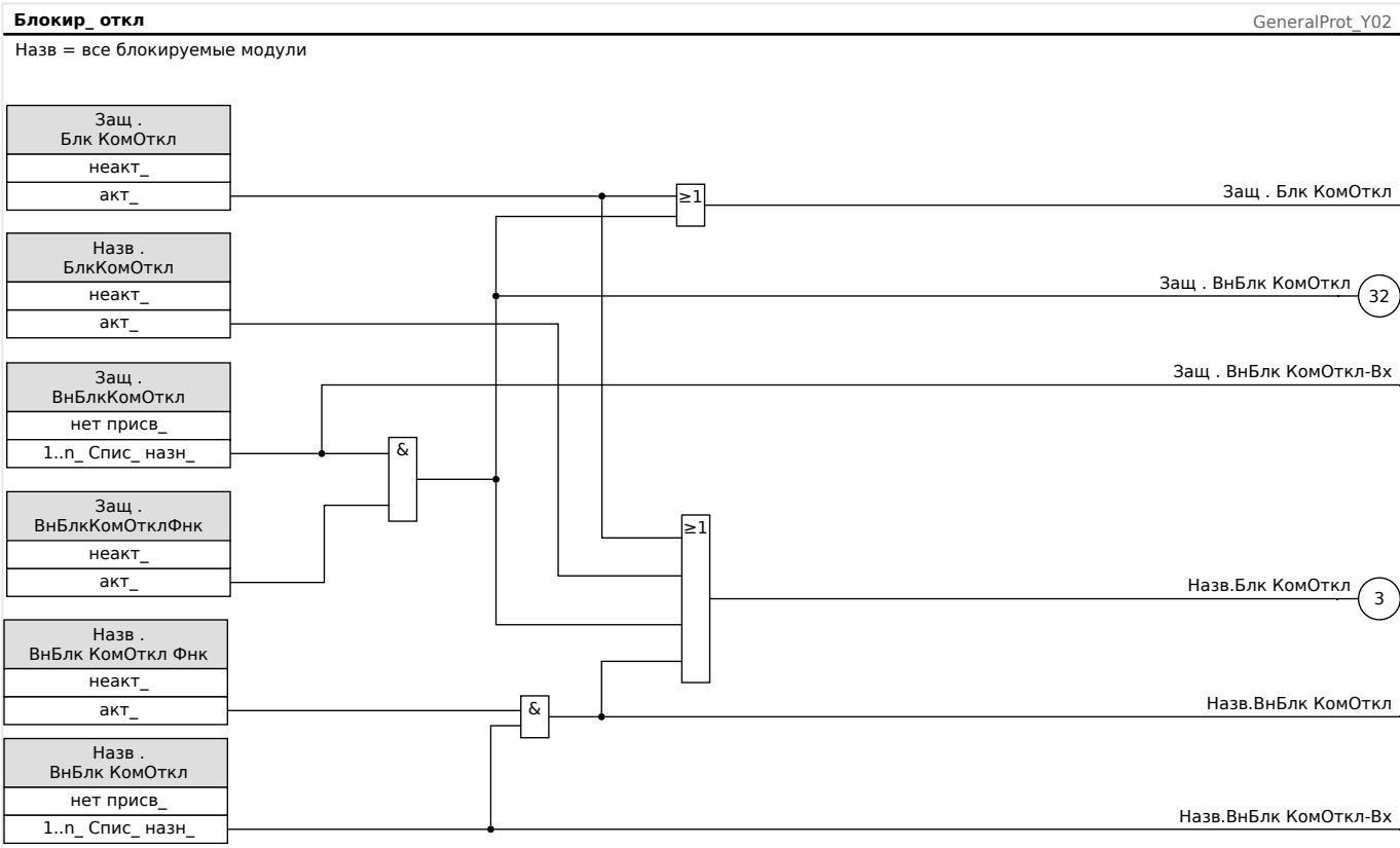
Рис. 40: Активация и деактивация команды отключения модуля защиты
