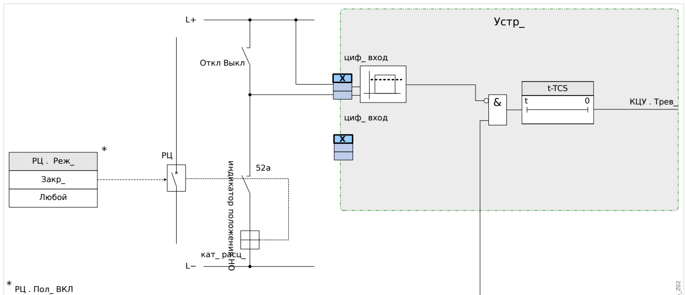
Рис. 61: Пример соединения: контроль цепи отключения только с одним вспомогательным контактом выключателя «Всп Вкл» (52a).
