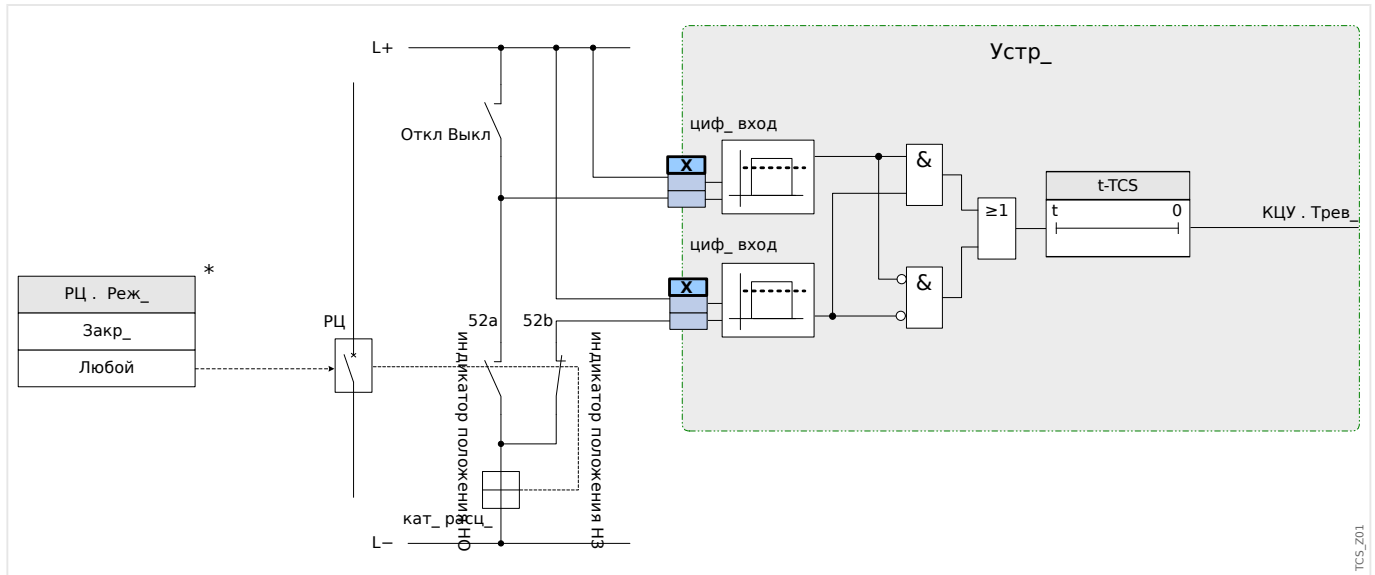
Рис. 60: Пример соединения: контроль цепи отключения с двумя вспомогательными контактами выключателя «Всп Вкл» (52a) и «Всп Выкл» (52b).
