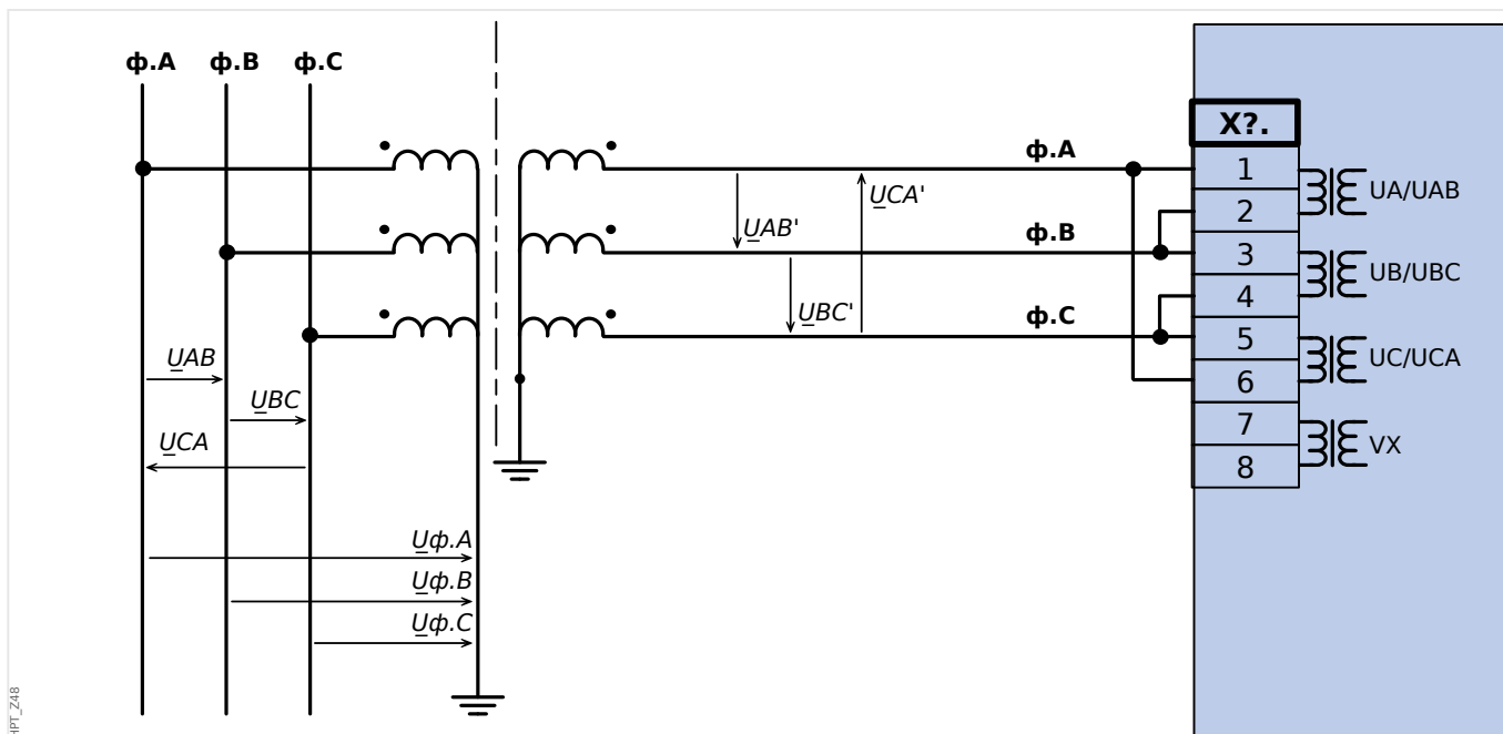
Рис. 19: Измерение трехфазного напряжения - схема измерительных входов: "соединение треугольником"
