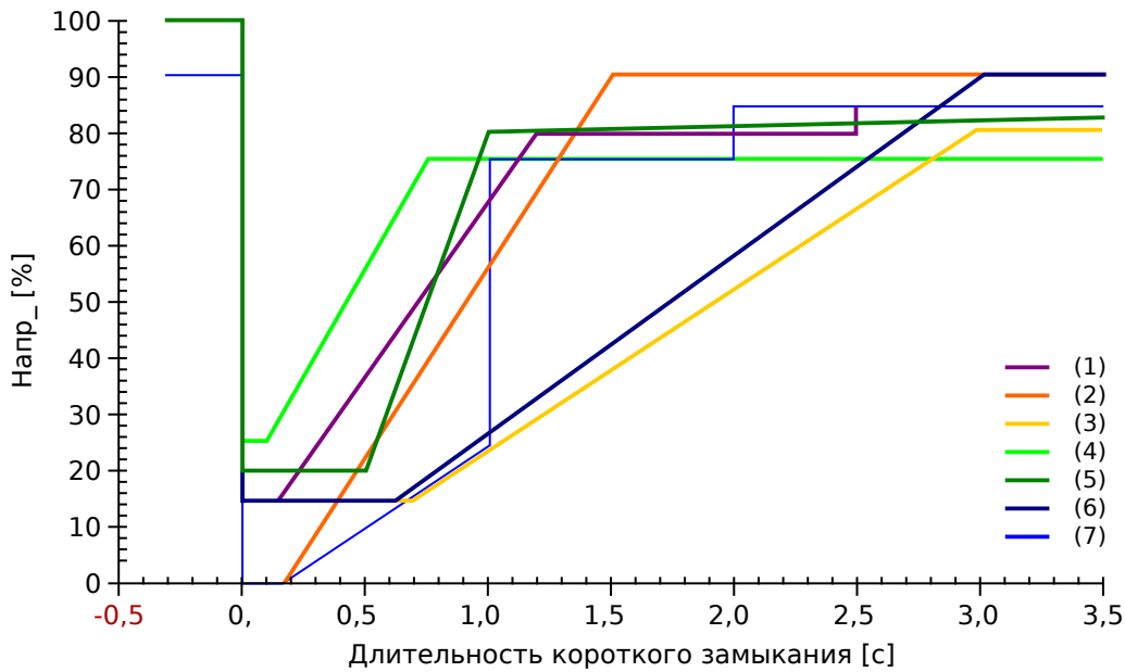
Рис. 55: Стандарты РПН; источник: eBWK Bd. 60 (2008 г.), № 4. Авторы: дипломированный инженер Томас Смолка, д. т. н. Карл-Хайнц Век, центр сертификации FGH e.V., Мангейм, а также дипломированный инженер (FH) Матиас Барч, Enercon GmbH, Аурих.
