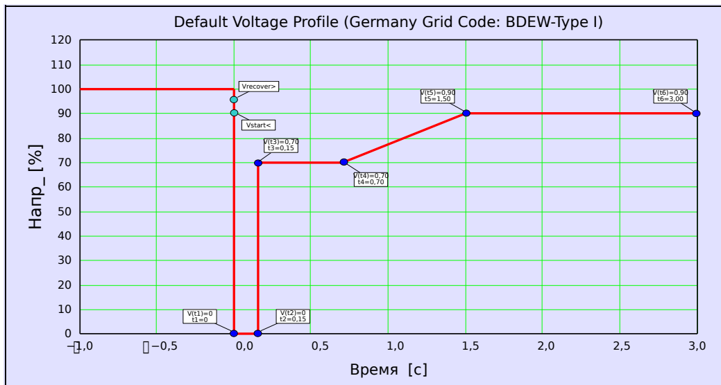
Рис. 58: Профиль LVRT по умолчанию (BDEW, тип I).
