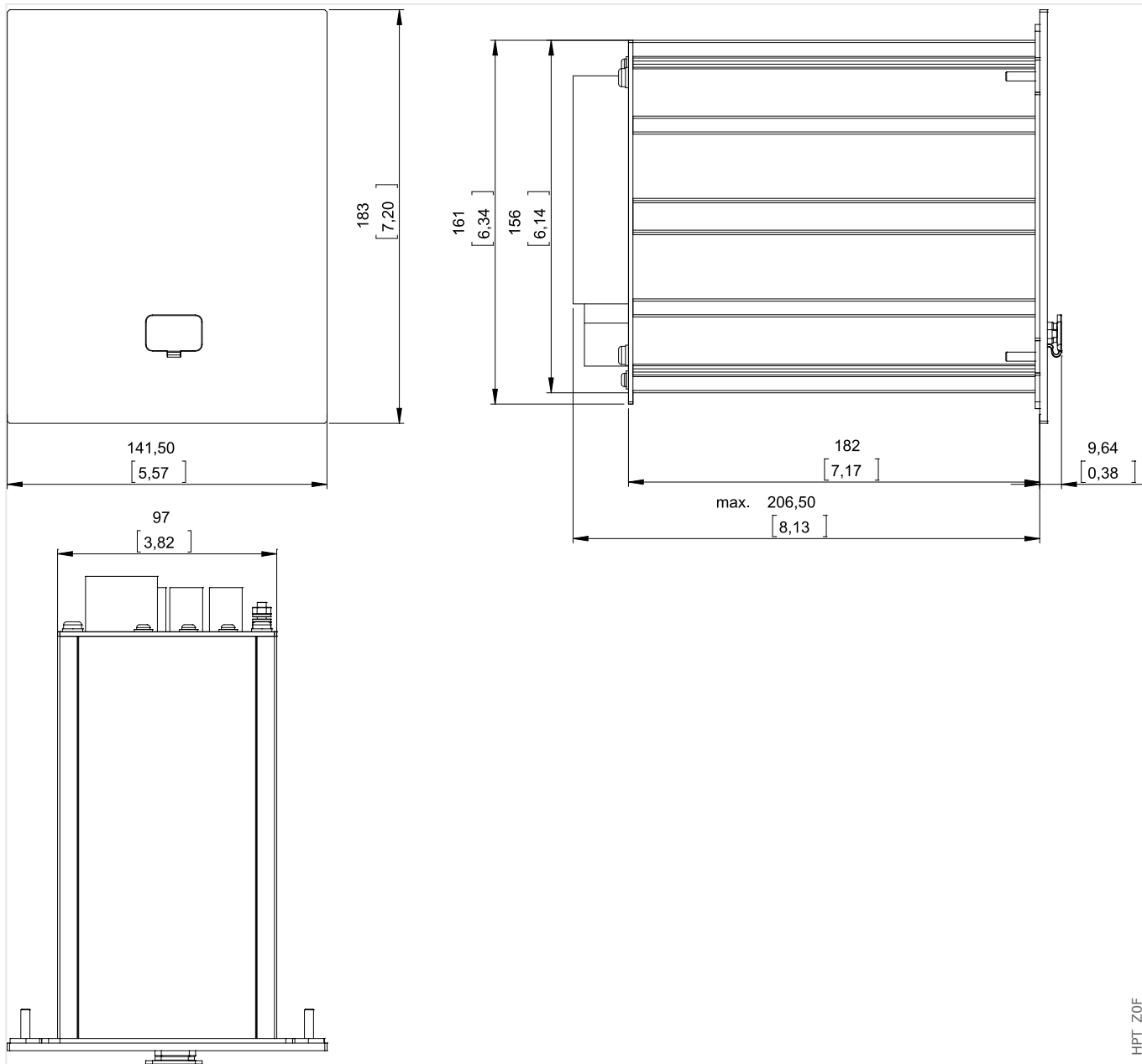
Рис. 5: Корпус V1: внешний вид (устройства с 8 кнопками). (Все размеры указаны в миллиметрах, за исключением размеров в квадратных скобках — [дюймы].)
