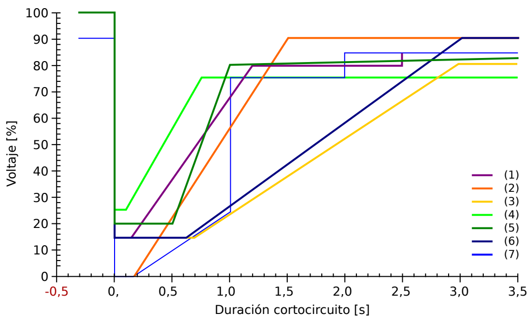
Fig. 55: Estándares de LVRT; fuente: eBWK Bd. 60 (2008) N.º 4. Autores: Dipl.-Ing. Thomas Smolka, Dr.-Ing. Karl-Heinz Weck, Zertifizierungstelle der FGH e.V., Mannheim, sowie Dipl.-Ing. (FH) Matthias Bartsch, Enercon GmbH, Aurich.
