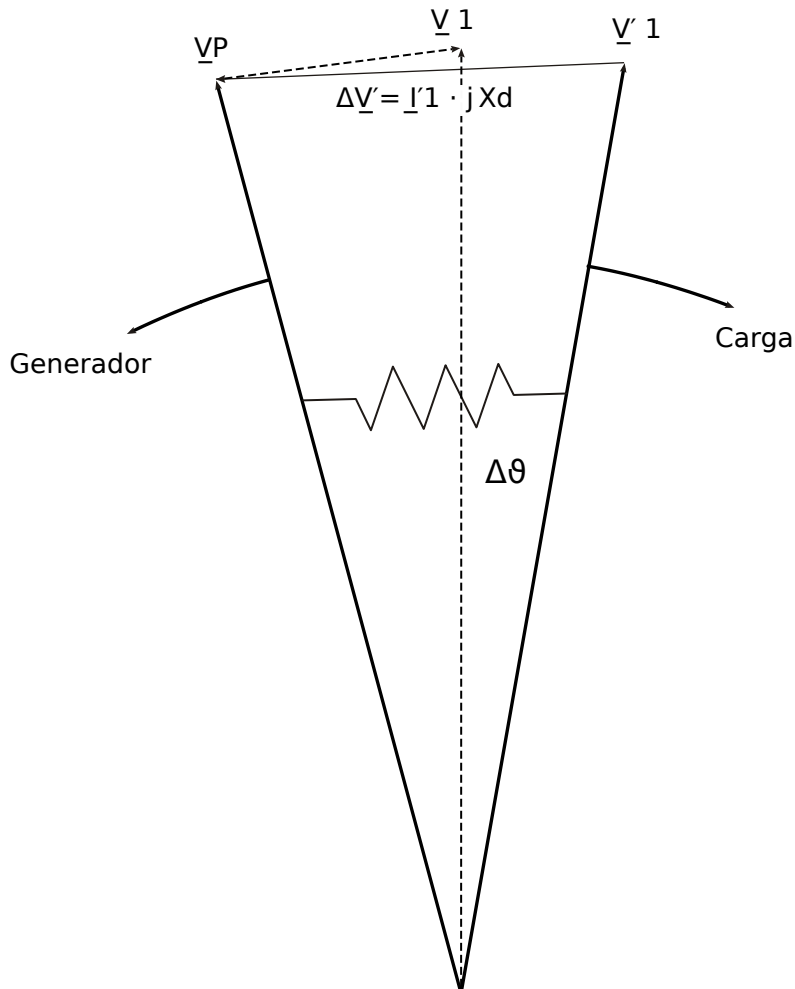
Fig. 48: Fallo de los vectores de tensión en la red.
