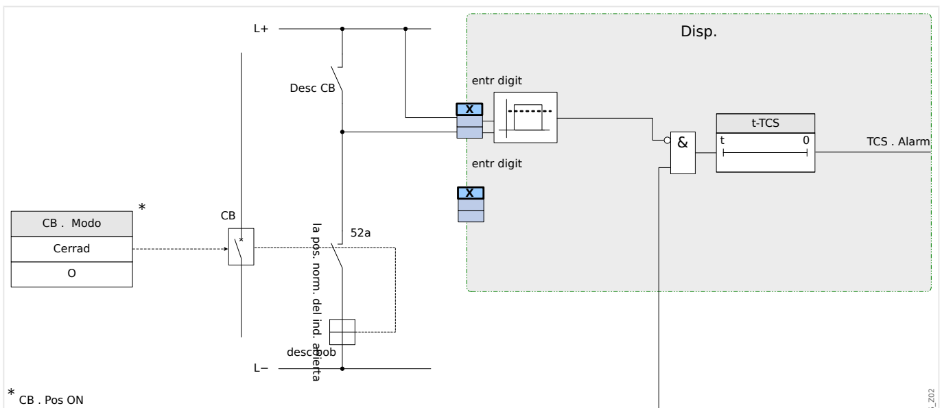
Fig. 61: Ejemplo de conexión: Supervisión del circuito de desconexión solo con un contacto auxiliar CB »Aux ON« (52a).
