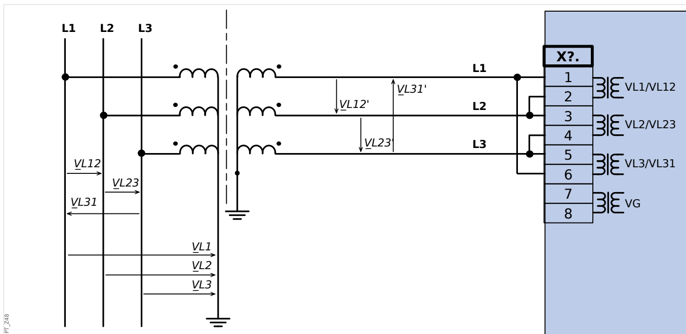
Fig. 19: Medida de tensión trifásica (cableado de las entradas de medición: "conexión delta")
