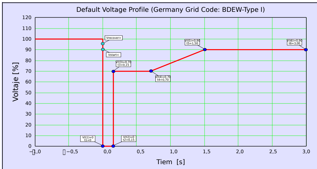
Fig. 58: Perfil de LVRT predeterminado (Tipo I de BDEW).
