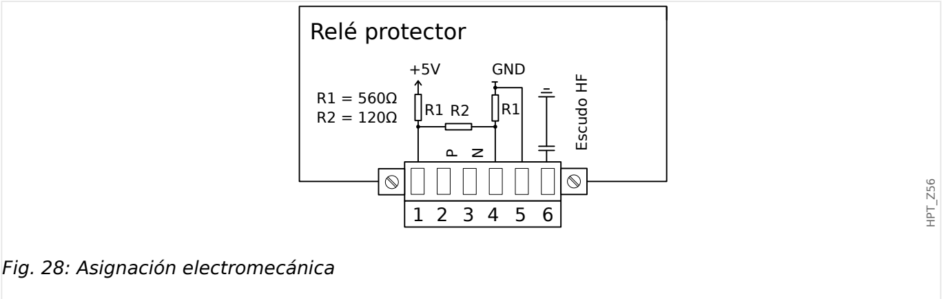
Fig. 27: Terminales
