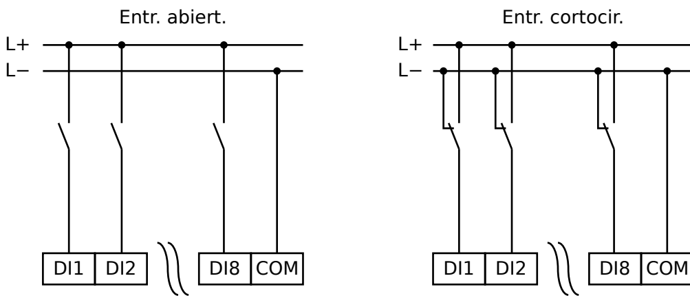
Fig. 82: Estado seguro de entradas digitales
