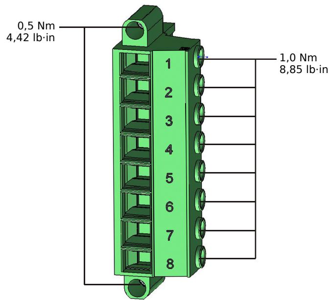
Fig. 81: Terminales de medición de tensión de la tarjeta de medición “TU” (↪ «TU - Entradas de medición de tensión»).
