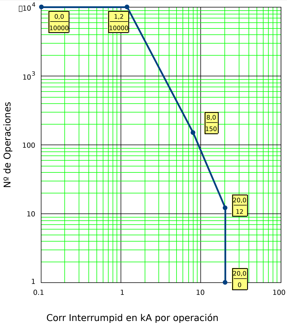
Fig. 68: Curva Mantenim Interruptor para Interrupt Circuito típico 25kV
