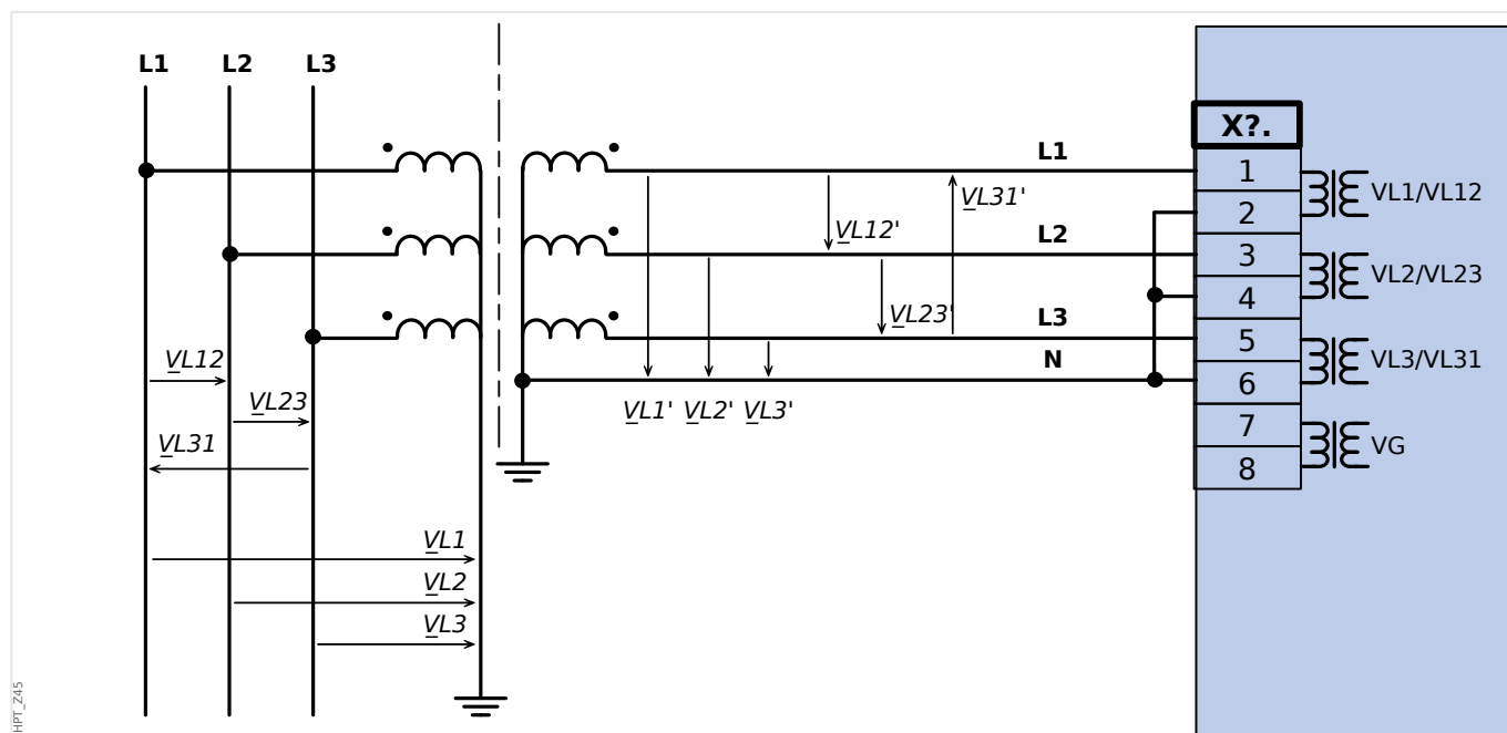
Fig. 17: VT Wye: Medida de voltaje trifásico: cableado de las entradas de medida: "conex. estrella"
