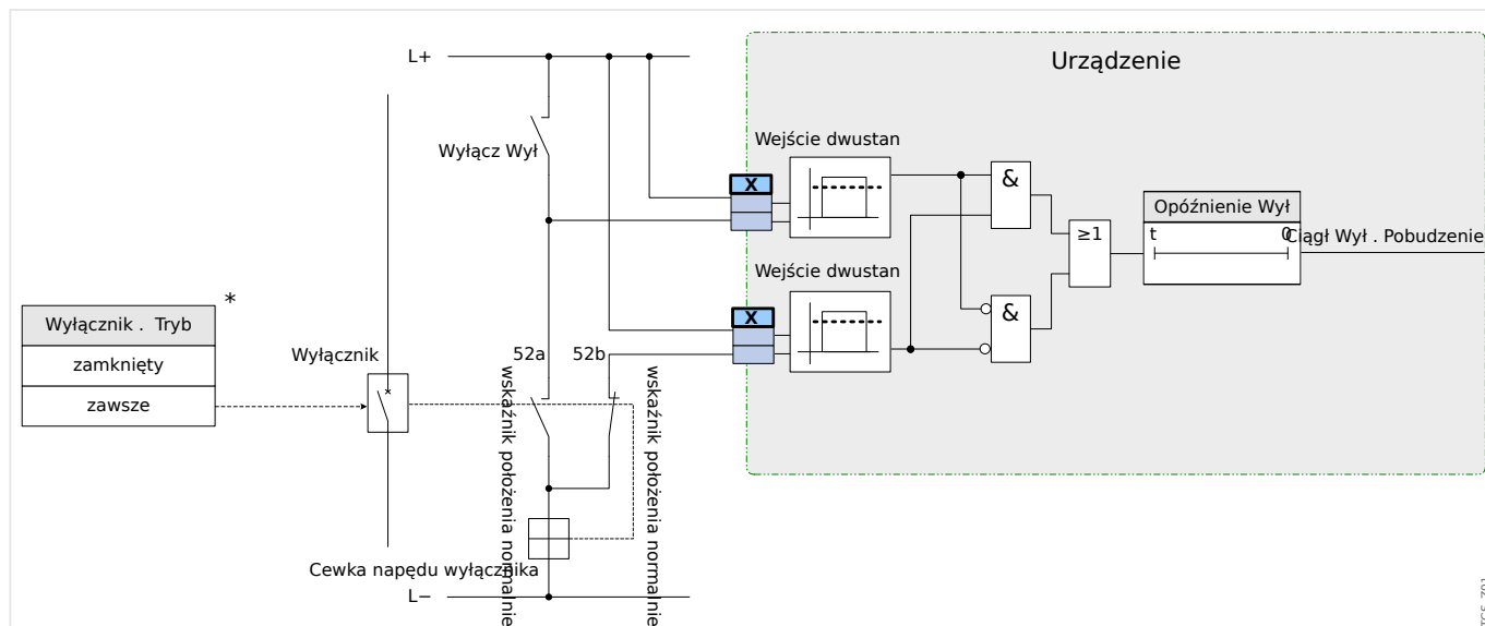
Rys. 84: Przykład okablowania: Układ kontroli ciągłości obwodów wyłącznika z dwoma stykami pomocniczymi wyłącznika „Położ ZAŁ” (52a) i „Położ WYŁ” (52b).
