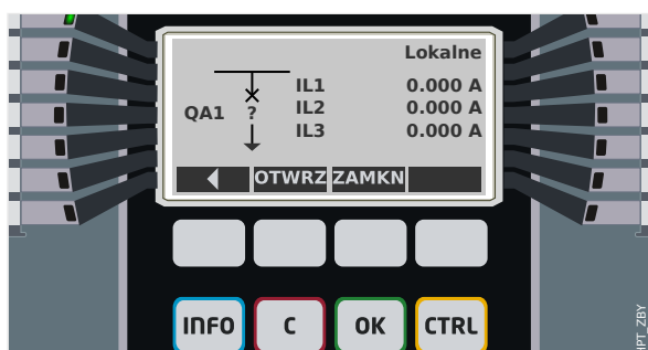
Rys. 89: Przykład strony sterowania z wyłącznikiem w pozycji zakłóconej (lub nieprawidłowej).
