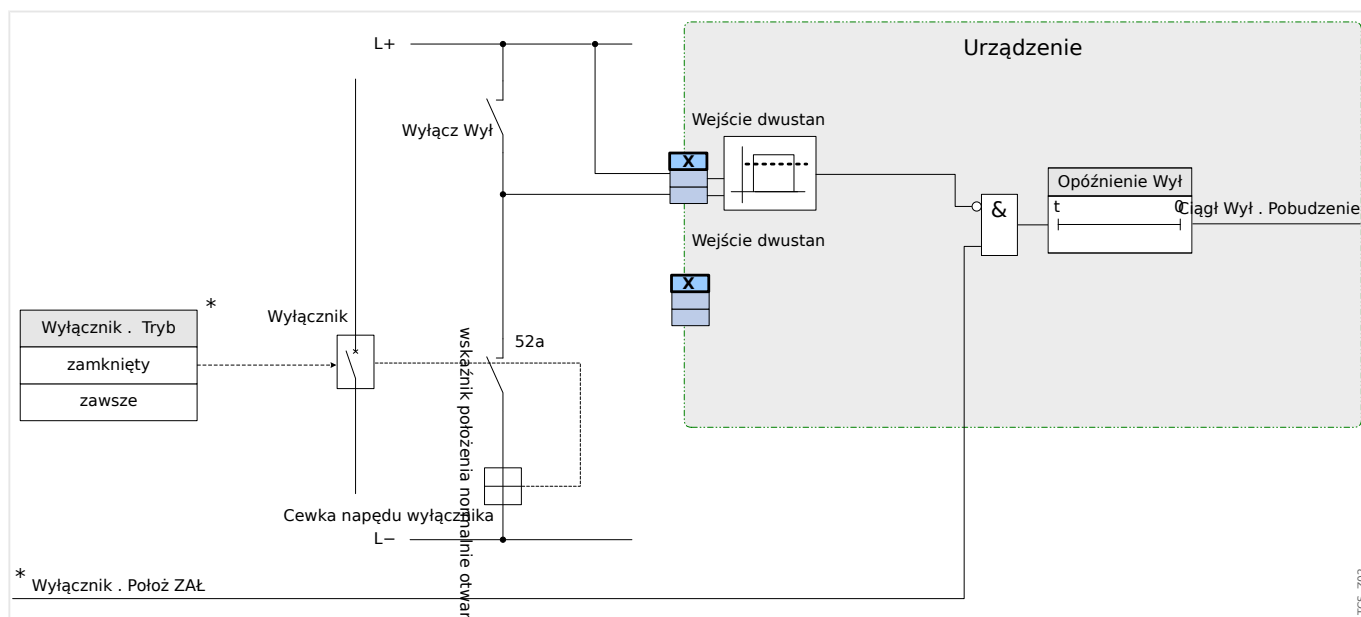
Rys. 85: Przykład okablowania: Układ kontroli ciągłości obwodów wyłącznika z tylko jednym stykiem pomocniczym wyłącznika „Położ ZAŁ” (52a).
