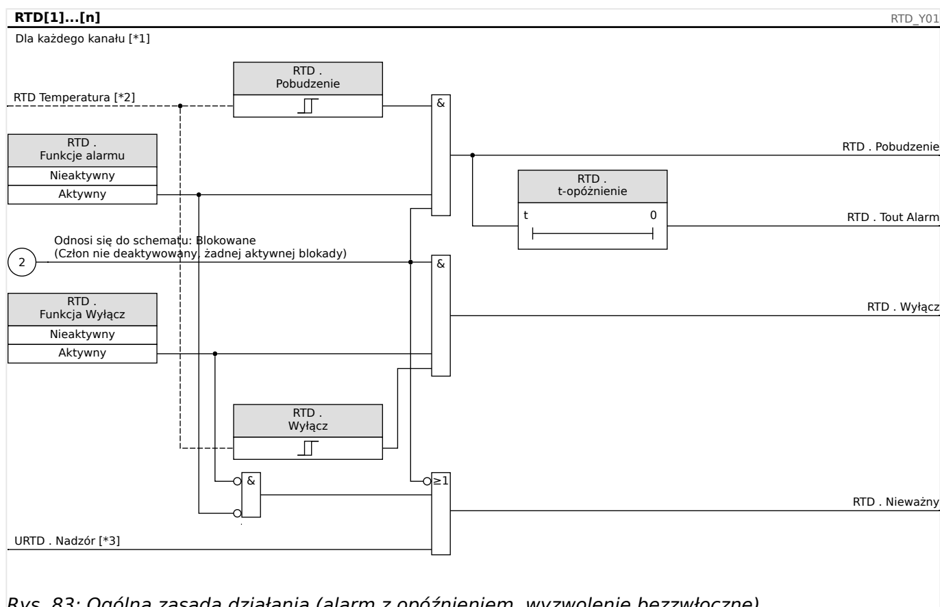
Rys. 83: Ogólna zasada działania (alarm z opóźnieniem, wyzwolenie bezzwłoczne).
