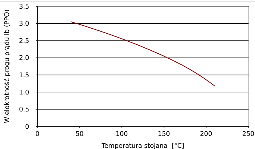
Rys. 61: Próg prądu skutecznego w stosunku do maksymalnej temperatury stojana.
