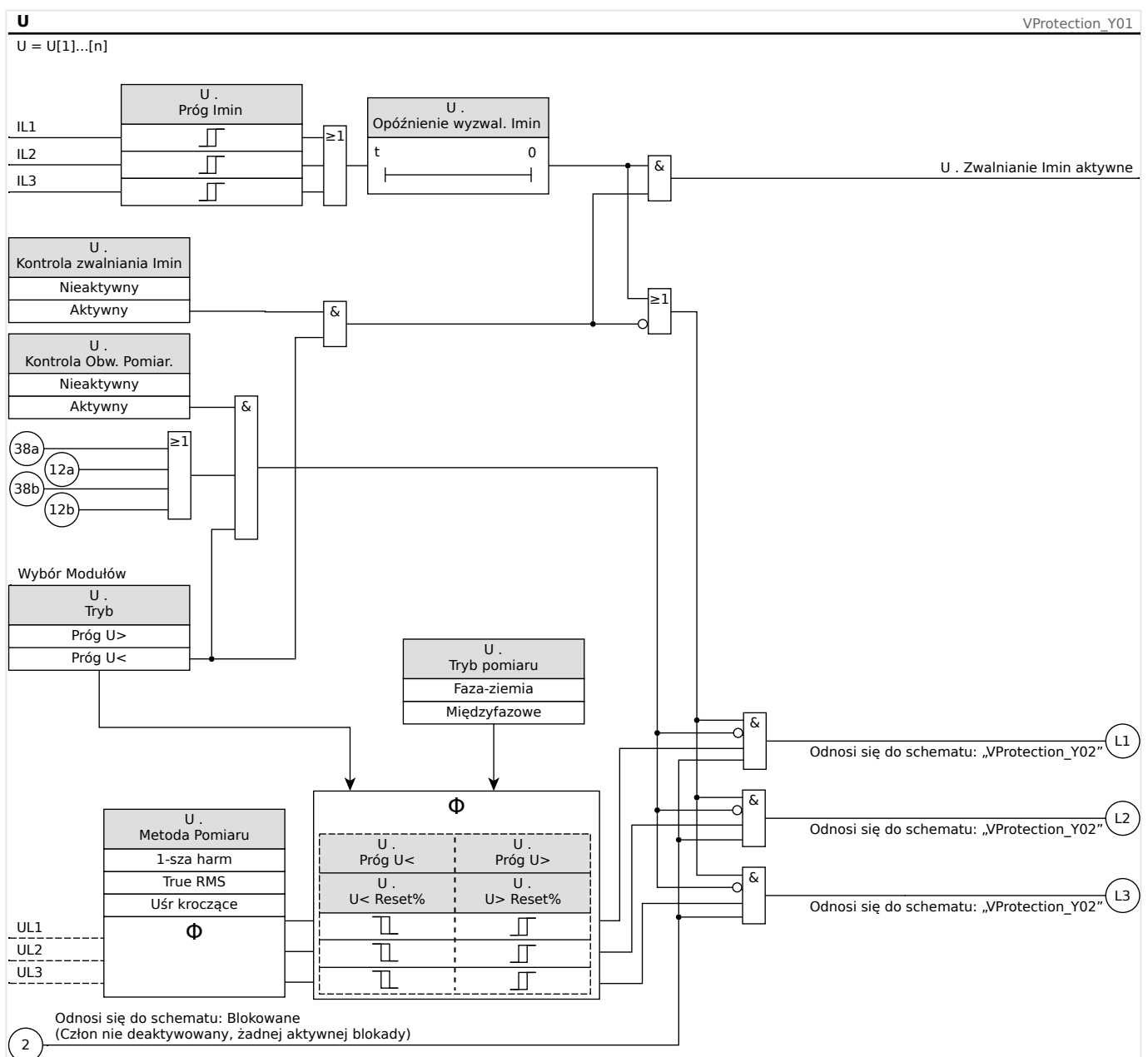
Rys. 71: Działanie modułu zabezpieczenia napięciowego, część 1.
