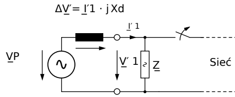
Rys. 77: Schemat zastępczy przy awarii sieci.
