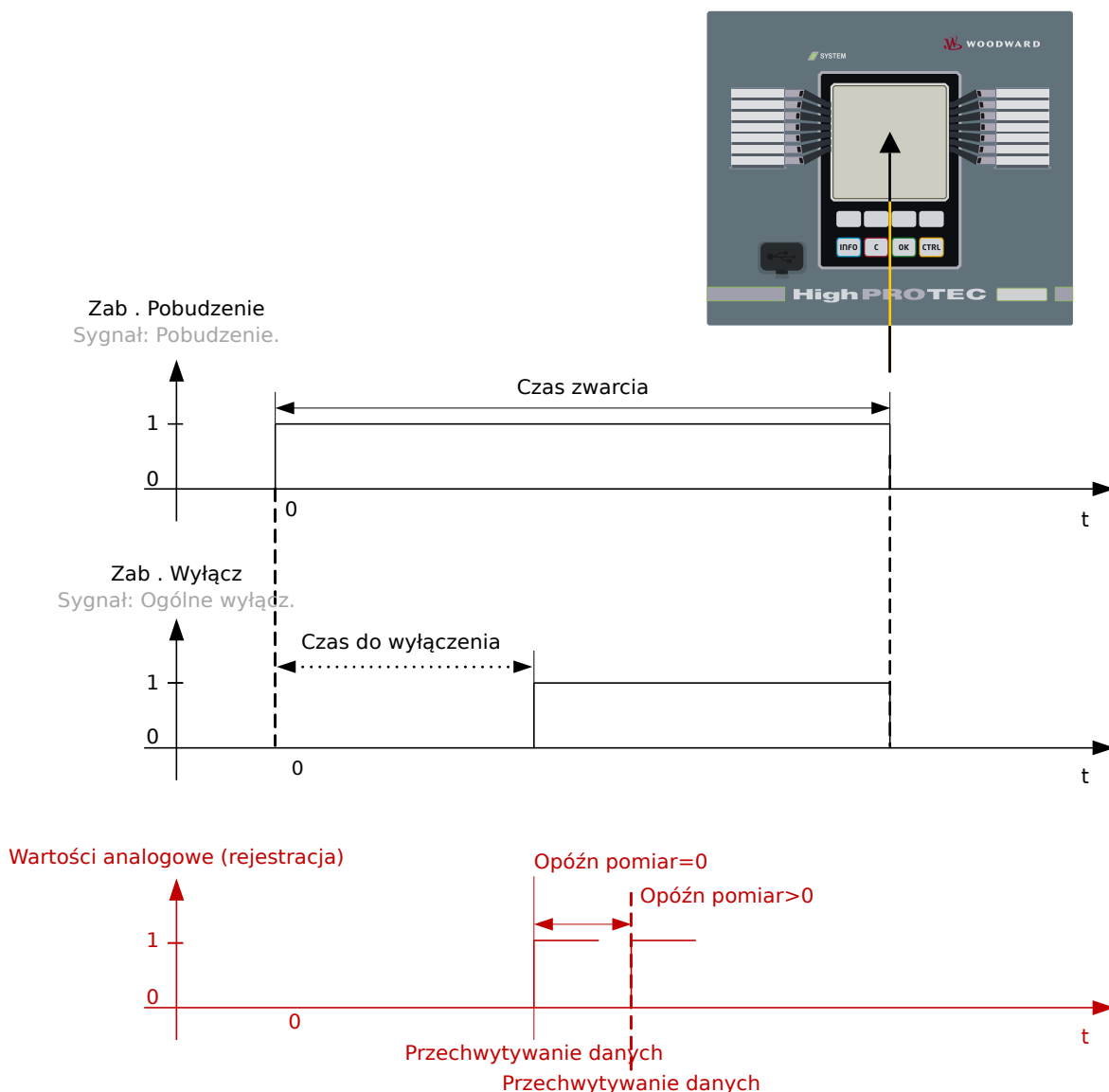
Rys. 98: Rejestrator zwarć: czasy (trwania).
