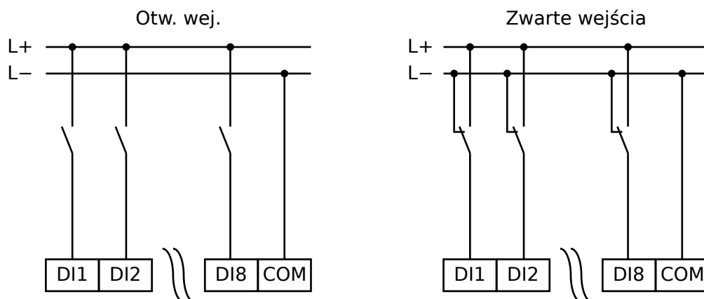
Rys. 110: Stan bezpieczny wejść dwustanowych
