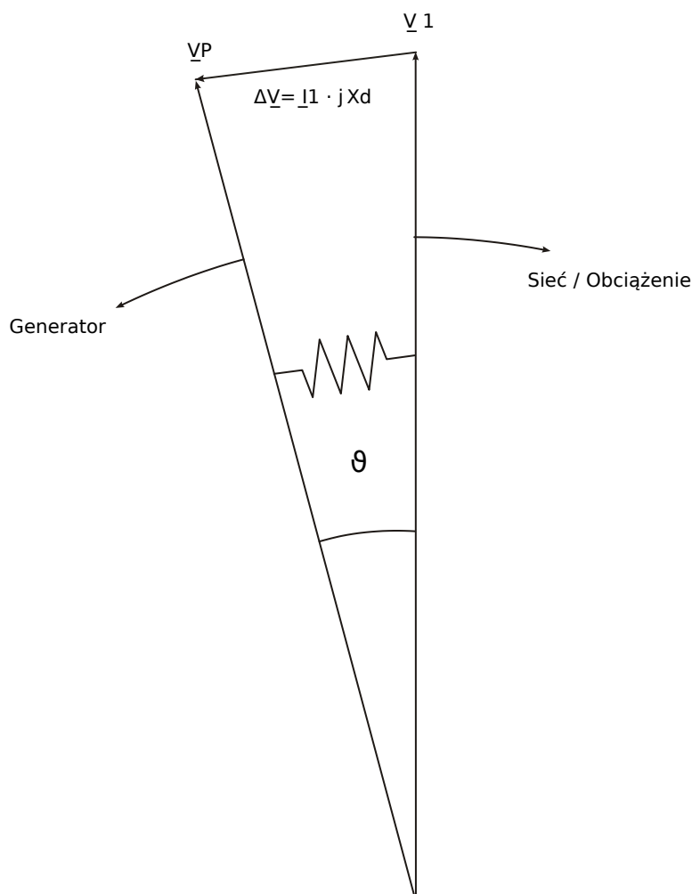
Rys. 76: Wektory napięcia przy pracy równoległej z siecią.
