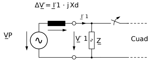
Fig. 77: Circuito equivalente en fallo de red eléctrica.
