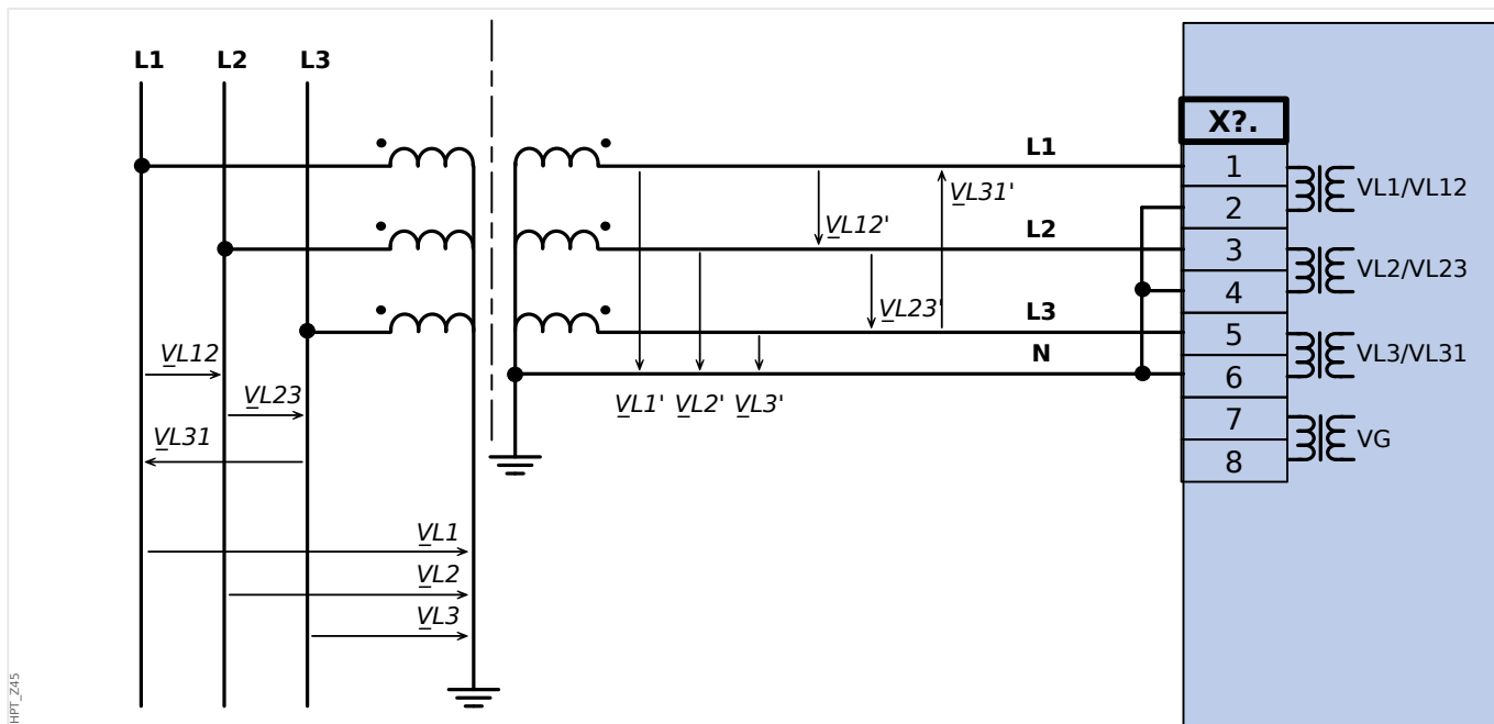
Fig. 28: VT Wye: Medida de voltaje trifásico: cableado de las entradas de medida: "conex. estrella"
