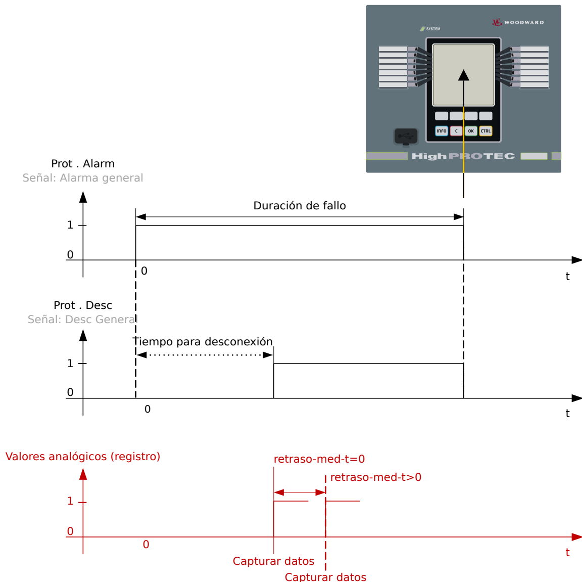
Fig. 98: Registrador de fallos: tiempos y duraciones.
