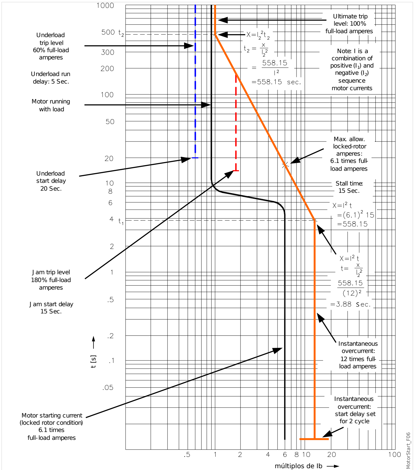
Fig. 65: Curva de protección de motor (ejemplo 2 sin RTD).
