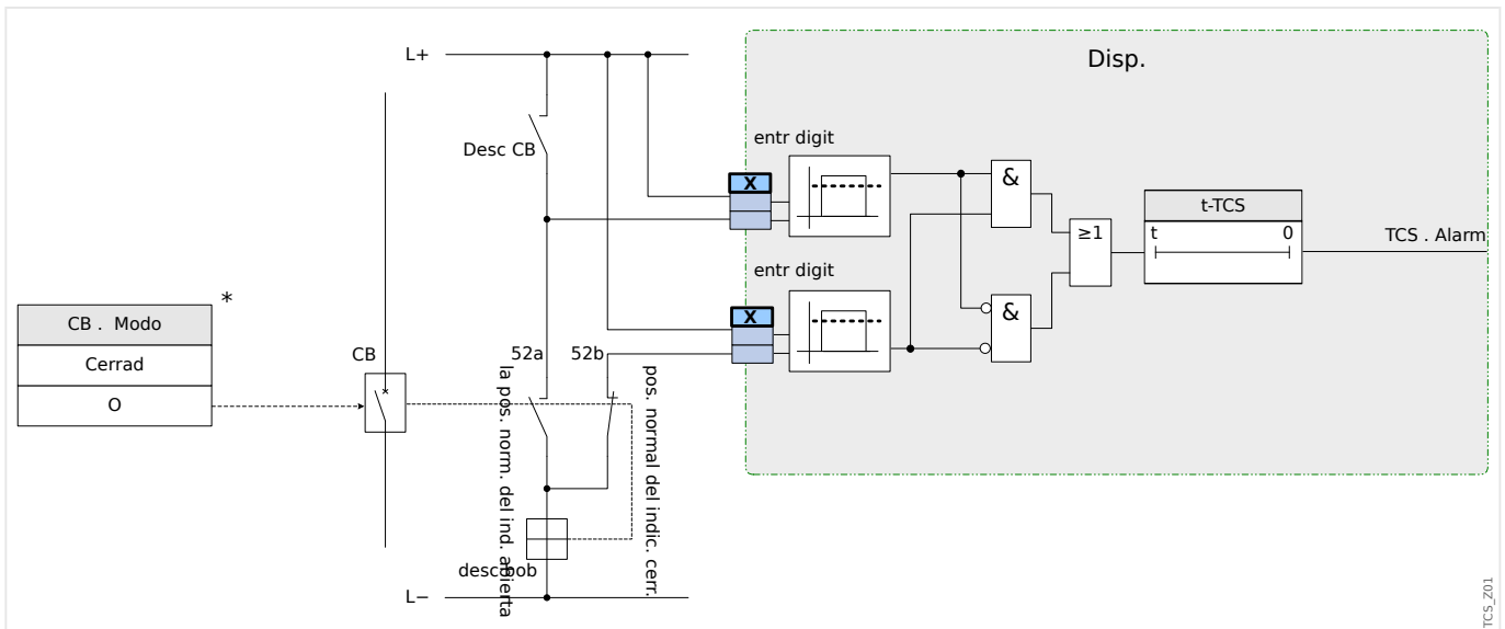
Fig. 84: Ejemplo de conexión: Supervisión del circuito de desconexión con dos contactos auxiliares CB »Aux ON« (52a) and »Aux OFF« (52b).
