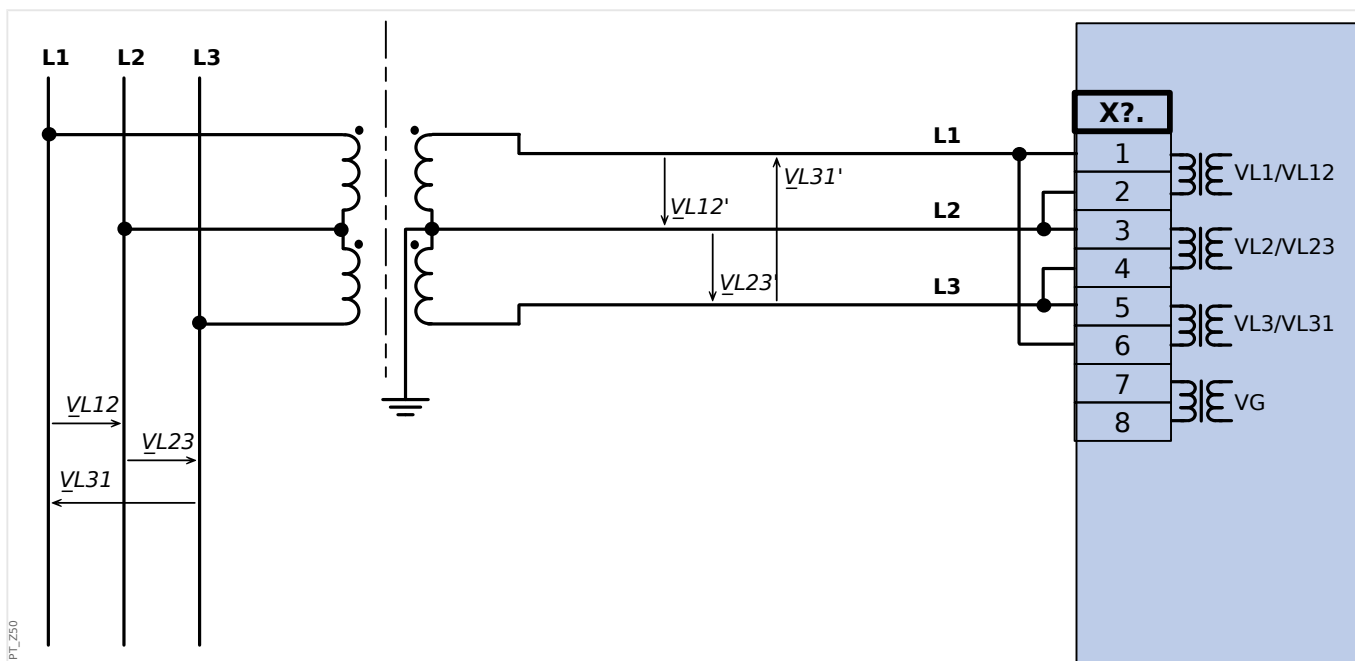
Fig. 32: Medida voltaje bifásico: cableado de las entradas de medida: "Abr. Delta"
