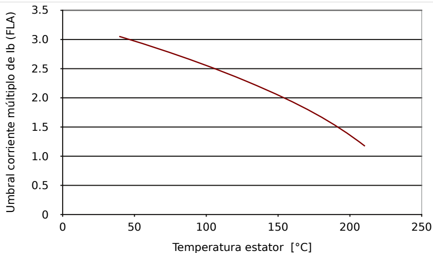
Fig. 61: Umbral corriente efectiva frente a temperatura máxima estator.
