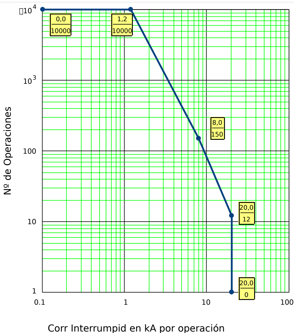
Fig. 93: Curva Mantenim Interruptor para Interrupt Circuito típico 25kV
