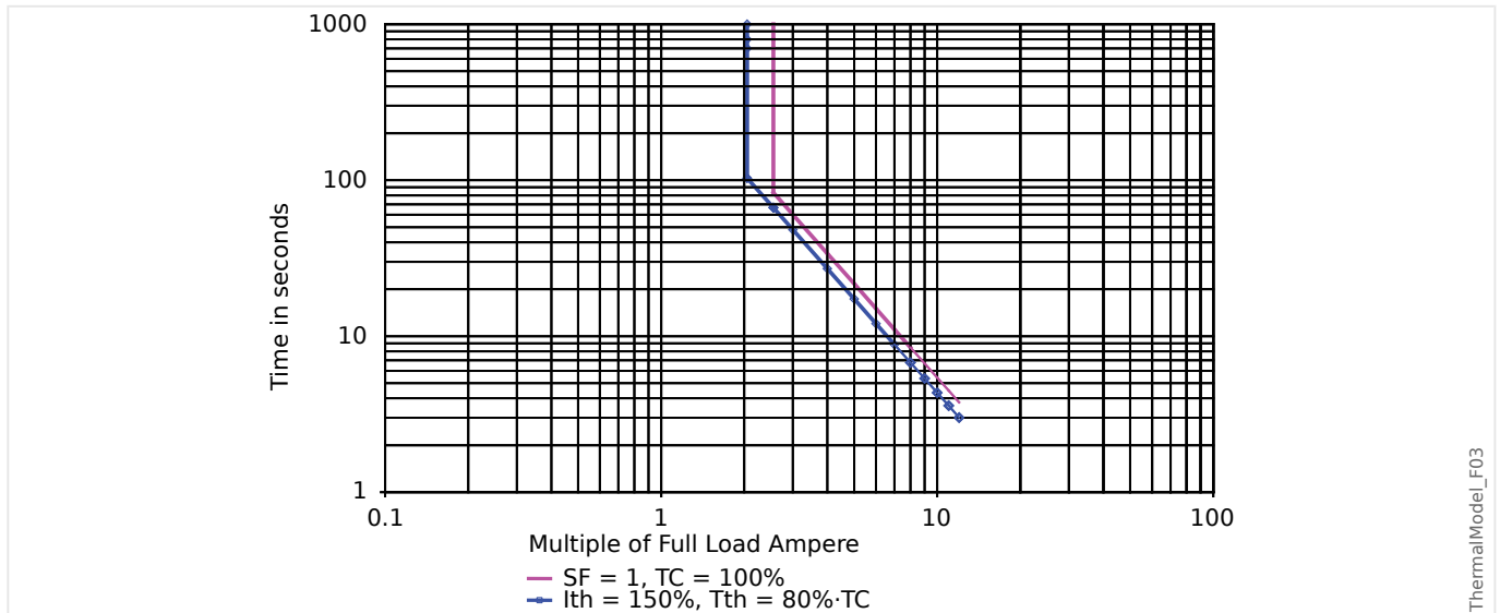
Fig. 63: Límite y curvas de desconexión del modelo de réplica térmica con RTD = 100°C.
