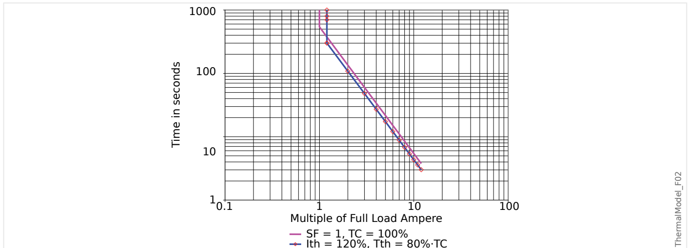
Fig. 62: Límite y curvas de desconexión del modelo de réplica térmica sin RTD.
