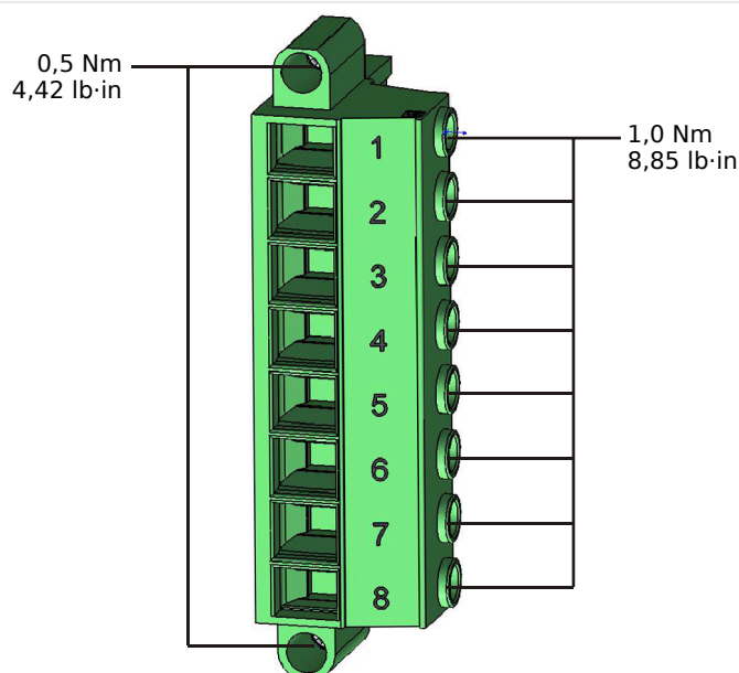
Fig. 109: Terminales de medición de tensión de la tarjeta de medición "TU" (↳ «TU - Entradas de medición de tensión»).
