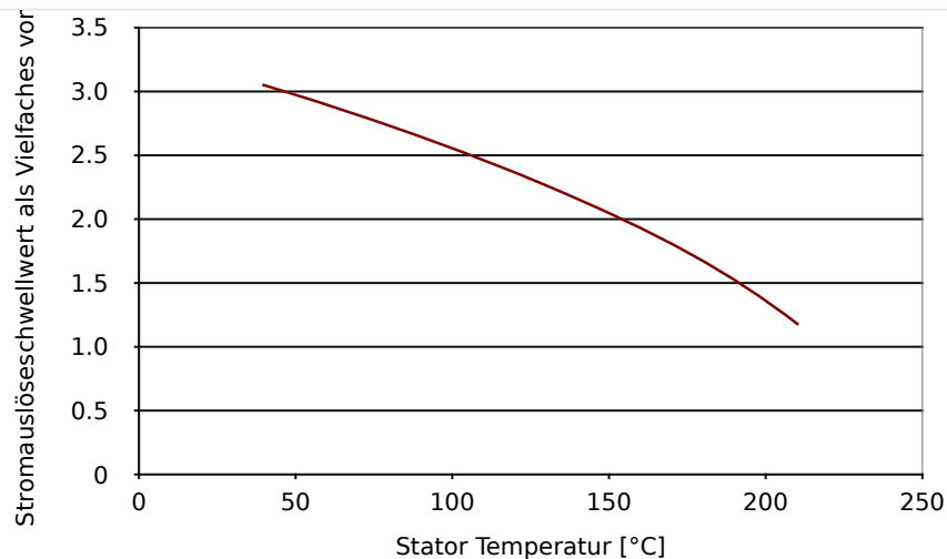
Abb. 63: Stromauslöseschwellwerte (Effektivwerte) über der maximalen Statortemperatur.
