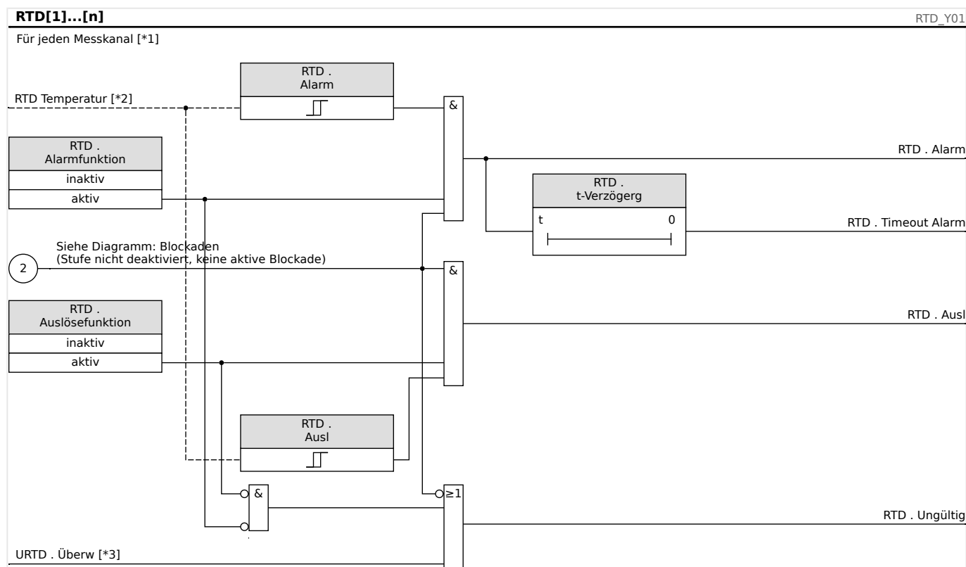
Abb. 85: Generelles RTD-Funktionsprinzip.
