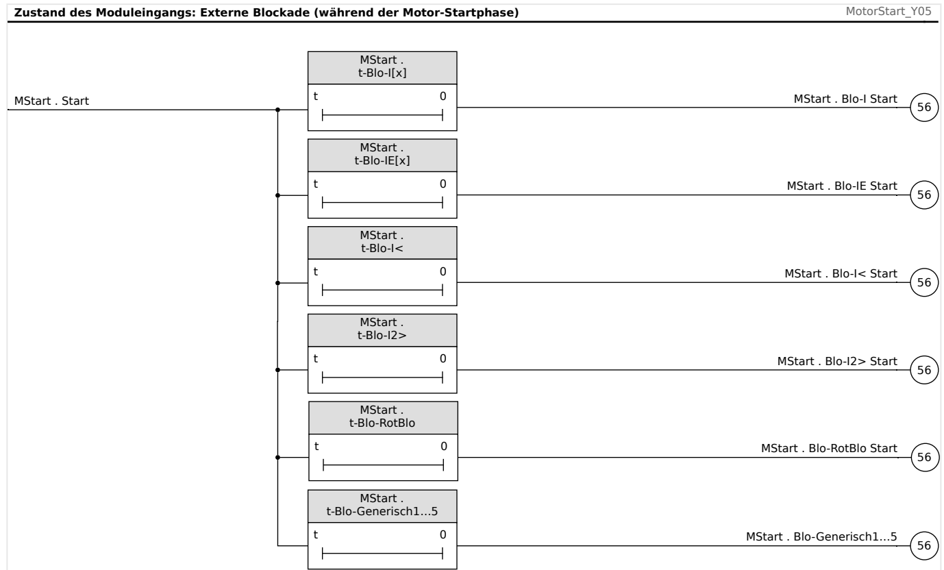
Abb. 59: Temporäre Blockade von Stromschutzfunktionen während Motorstarts.
