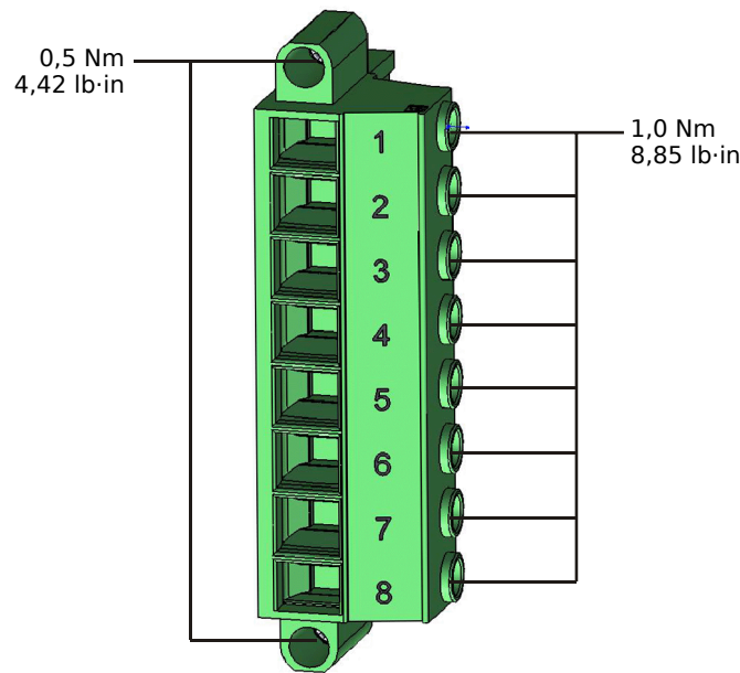
Abb. 111: Spannungsmessstecker der Spannungsmesskarte „TU“ (↳ „TU - Spannungsmesseingänge“).
