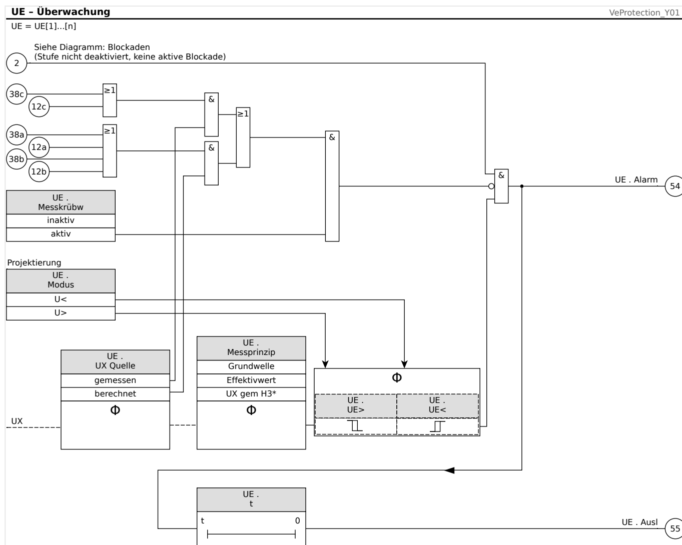
Abb. 75: UE/UX-Spannungsüberwachung, Teil 1 (Überwachungsfunktion, Auslöse-Entscheidung).
