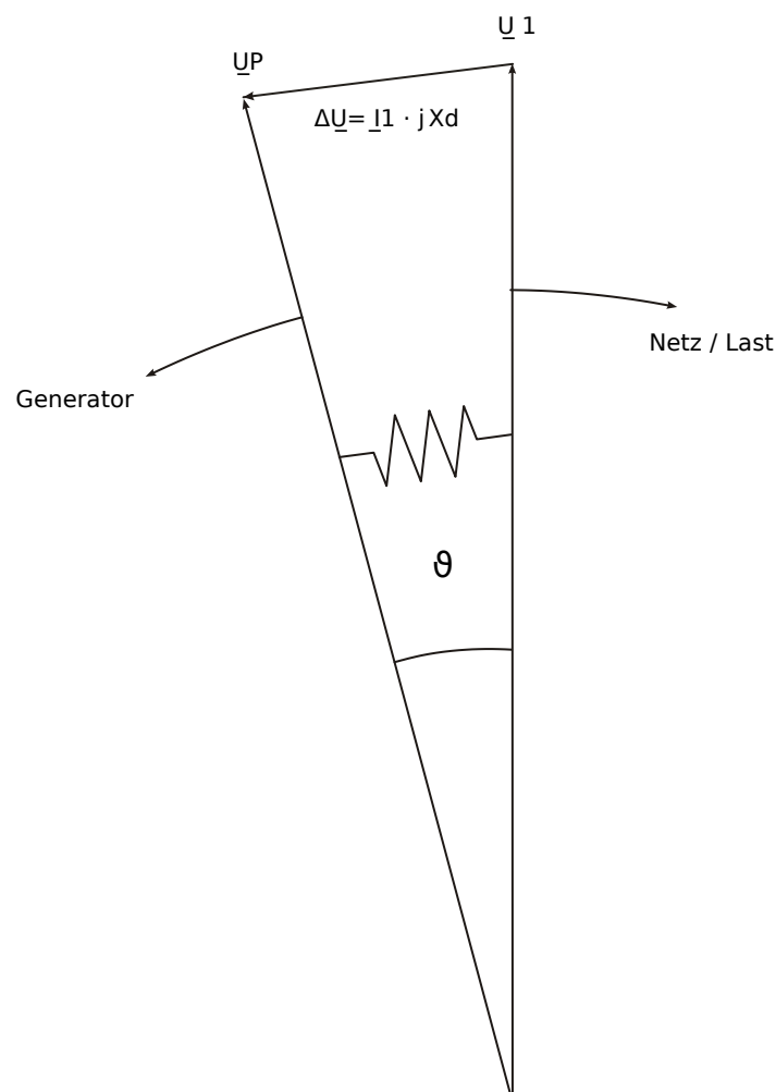
Abb. 78: Polradwinkel bei konstanter Belastung des Generators.
