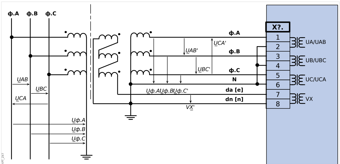
Рис. 29: VT Уюе с соединением разомкнутого треугольника.
