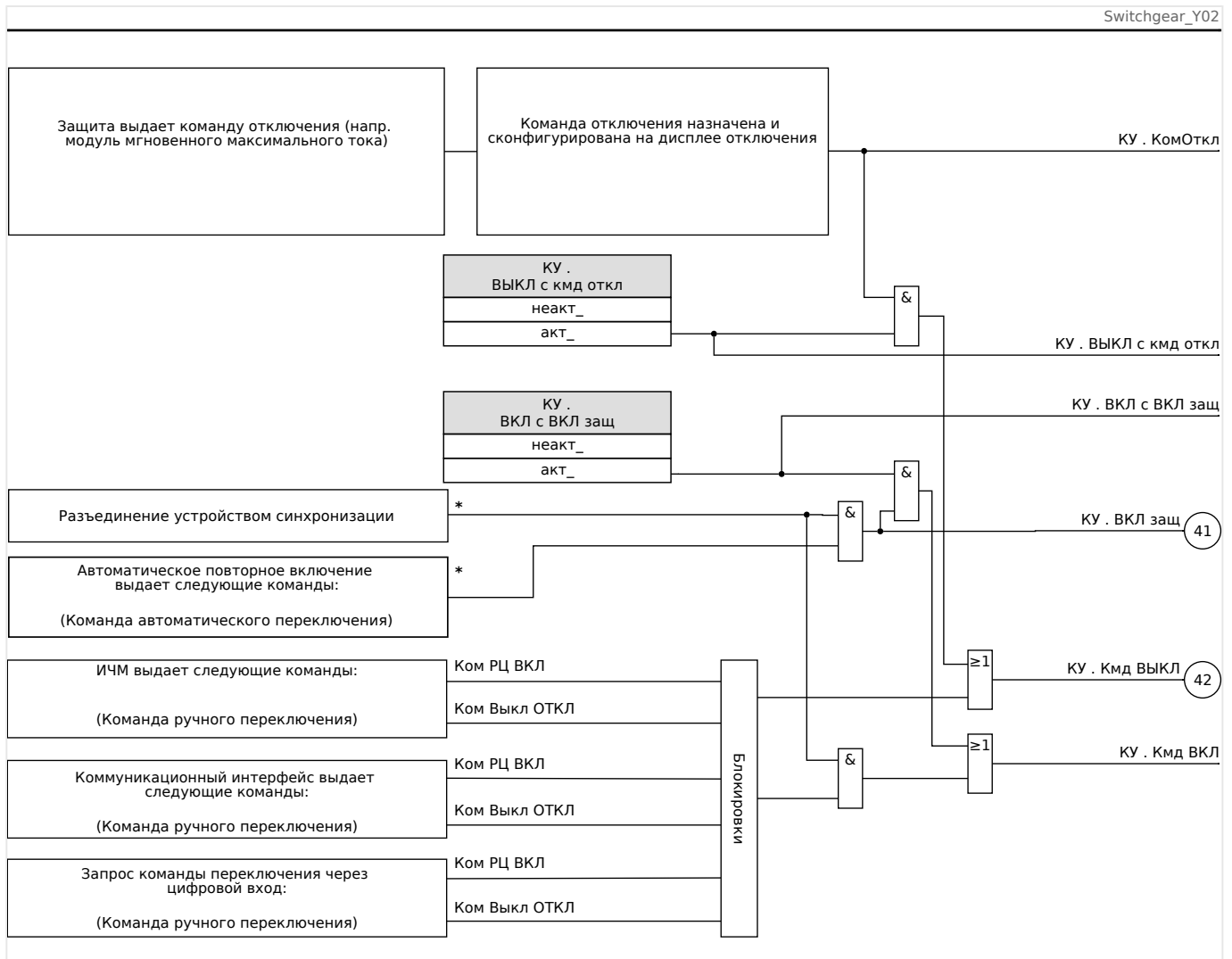
Рис. 102: Блокировки. (Детали, отмеченные «*»: наличие зависит от заказанного типа устройства.)
