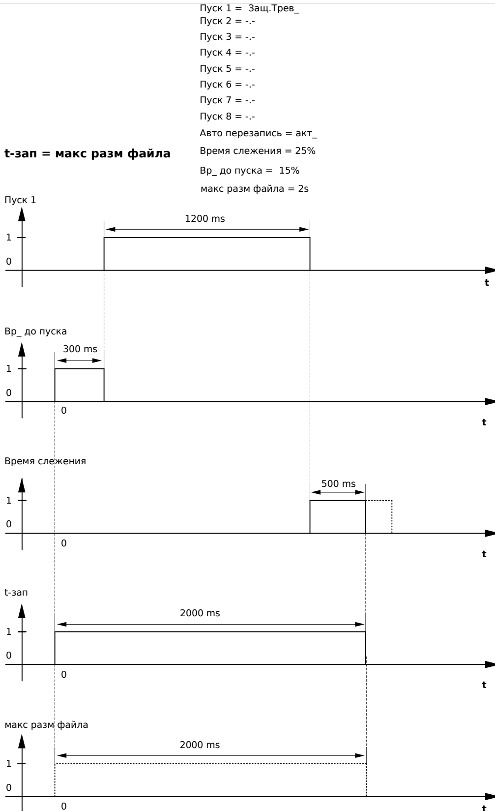
Рис. 107: Пример временной диаграммы регистратора аварийных нарушений I
