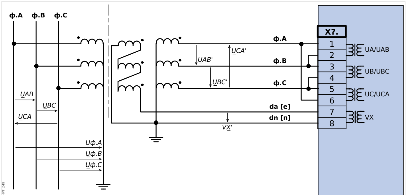
Рис. 31: Измерение трехфазного напряжения - схема измерительных входов: "соединение треугольником" Измерение напряжения нулевой последовательности VG через вспомогательные обмотки (e-n) («открытый треугольник»)
