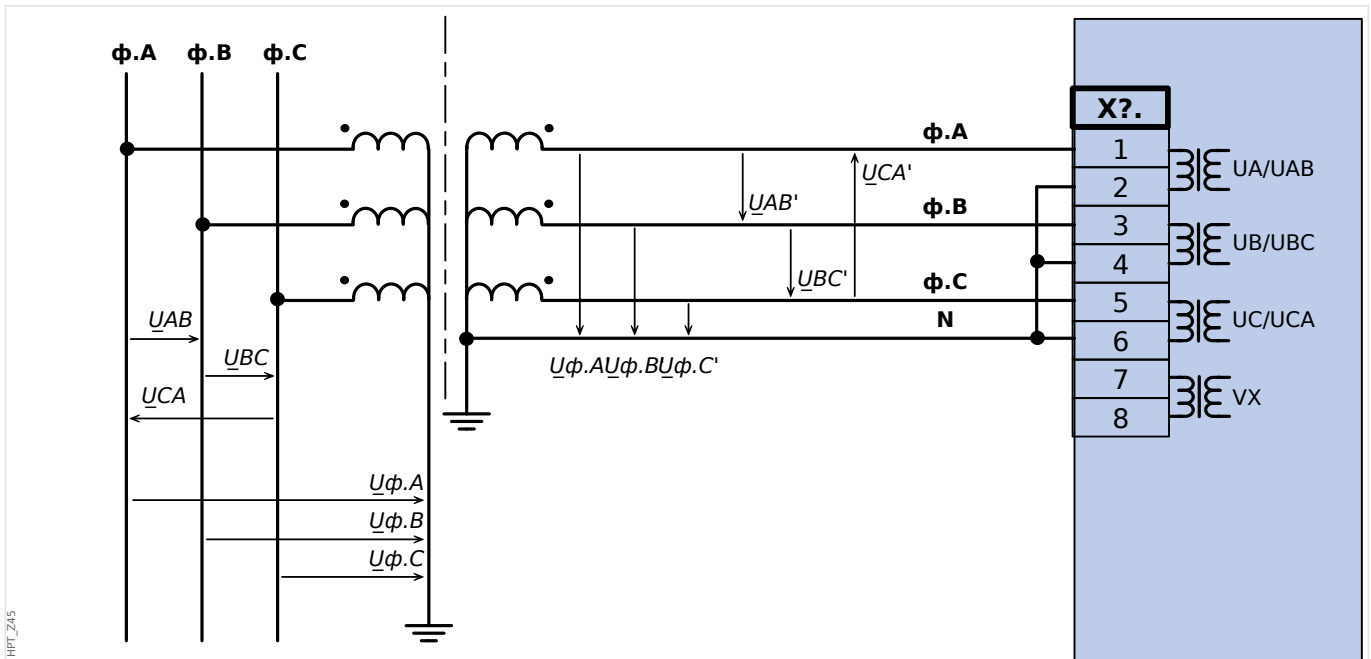
Рис. 28: VT Уюе: Измерение трехфазного напряжения по схеме «звезда»
