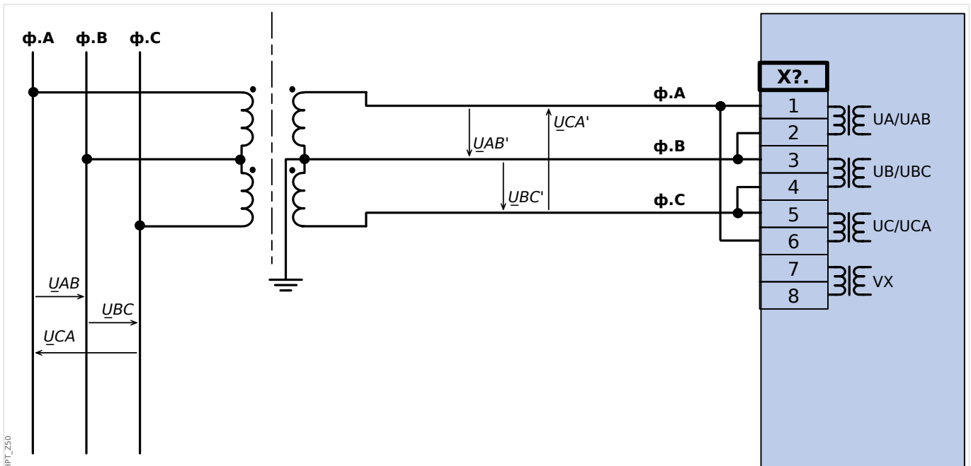
Рис. 32: Измерение двухфазного напряжения - электрическая схема измерительных входов: «соединение открытым треугольником»
