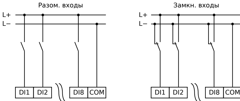
Рис. 119: Безопасное состояние цифровых входов
