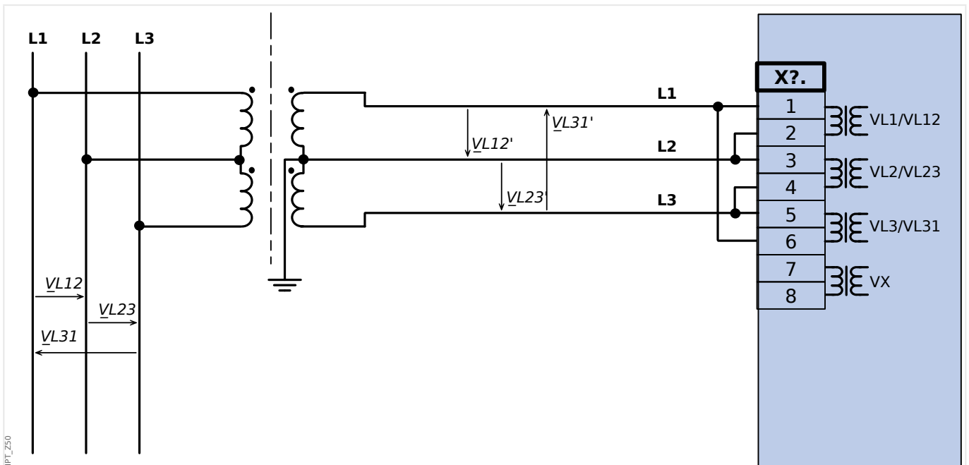
Fig. 32: Medição de voltagem bifásica - fiação das entradas de medição: "Delta Aber"
