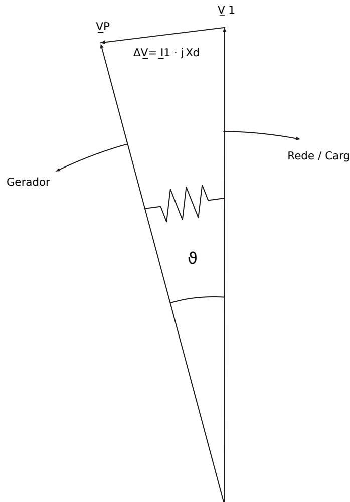
Fig. 87: Vetores de tensão em operação paralela.
