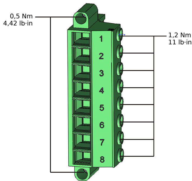
Fig. 118: Terminais de medição de tensão da placa de medição "TU" (↳ "3.6.1 TU - Entradas de Medição de Tensão").
