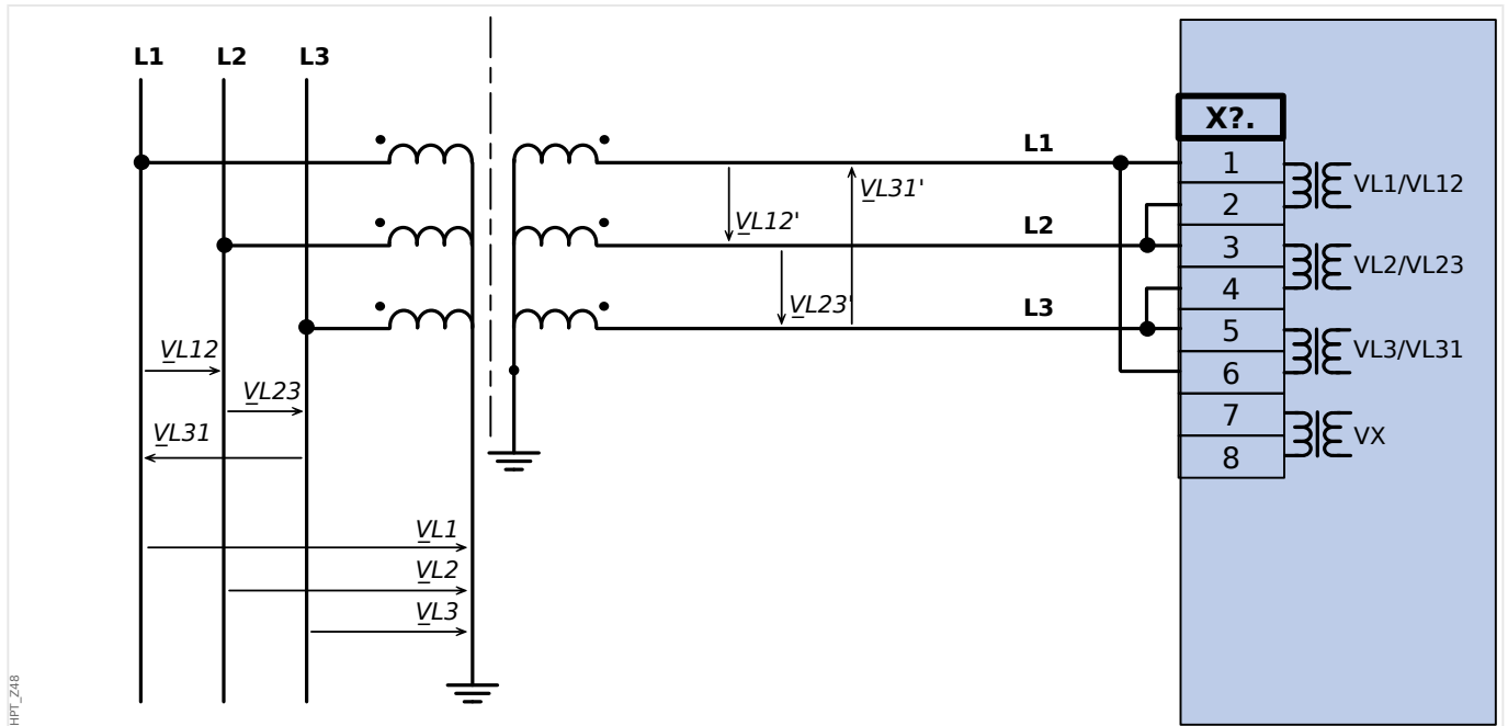
Fig. 30: Medição de tensão trifásica - fiação das entradas de medição: "conexão-delta"
