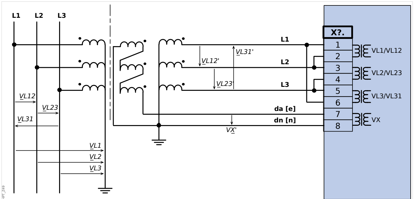
Fig. 31: Medição VG voltagem residual por meio de "delta aberto" (e-n) de circuito auxiliar
