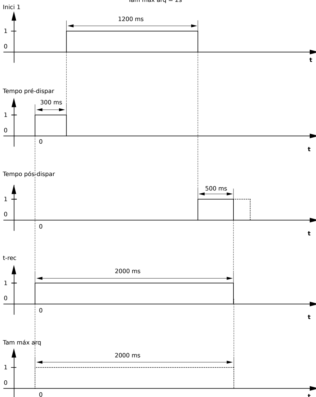
Fig. 107: Exemplo de Gráfico de Prazo do Gravador de Perturbação I
