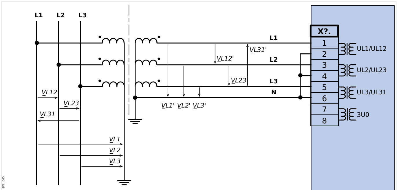
Rys. 28: Przekładnik napięciowy połączony w gwiazdę: Trójfazowy pomiar napięcia w układzie gwiazdy
