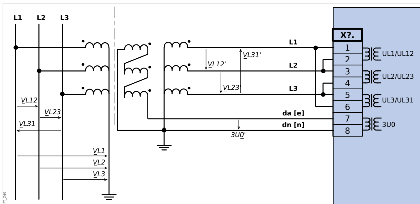
Rys. 31: Trójfazowy pomiar napięcia w układzie trójkąta: połączenie przewodów wejść pomiarowych: "połączenie w trójkąt" Pomiar 3U_0 napięcia szczytkowego poprzez dodatkowe uzwojenia (e-n) w układzie otwartego trójkąta
