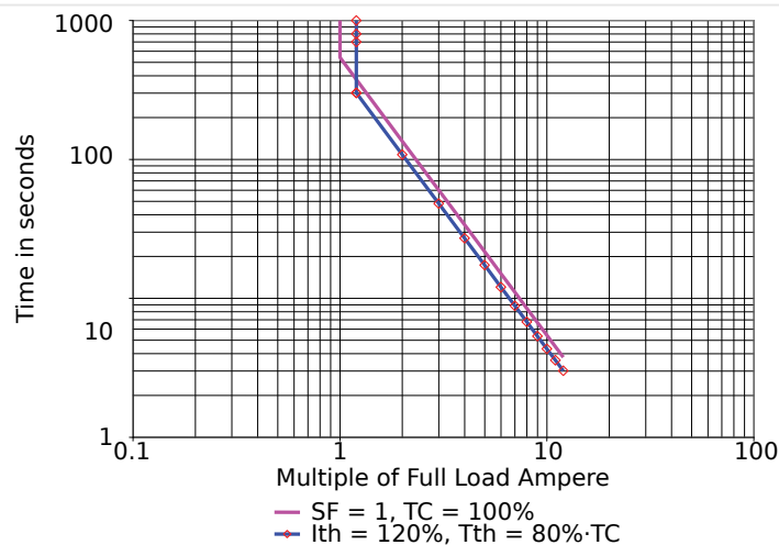
Rys. 65: Limit modelu cieplnego i krzywe wyzwalań bez RCT.
