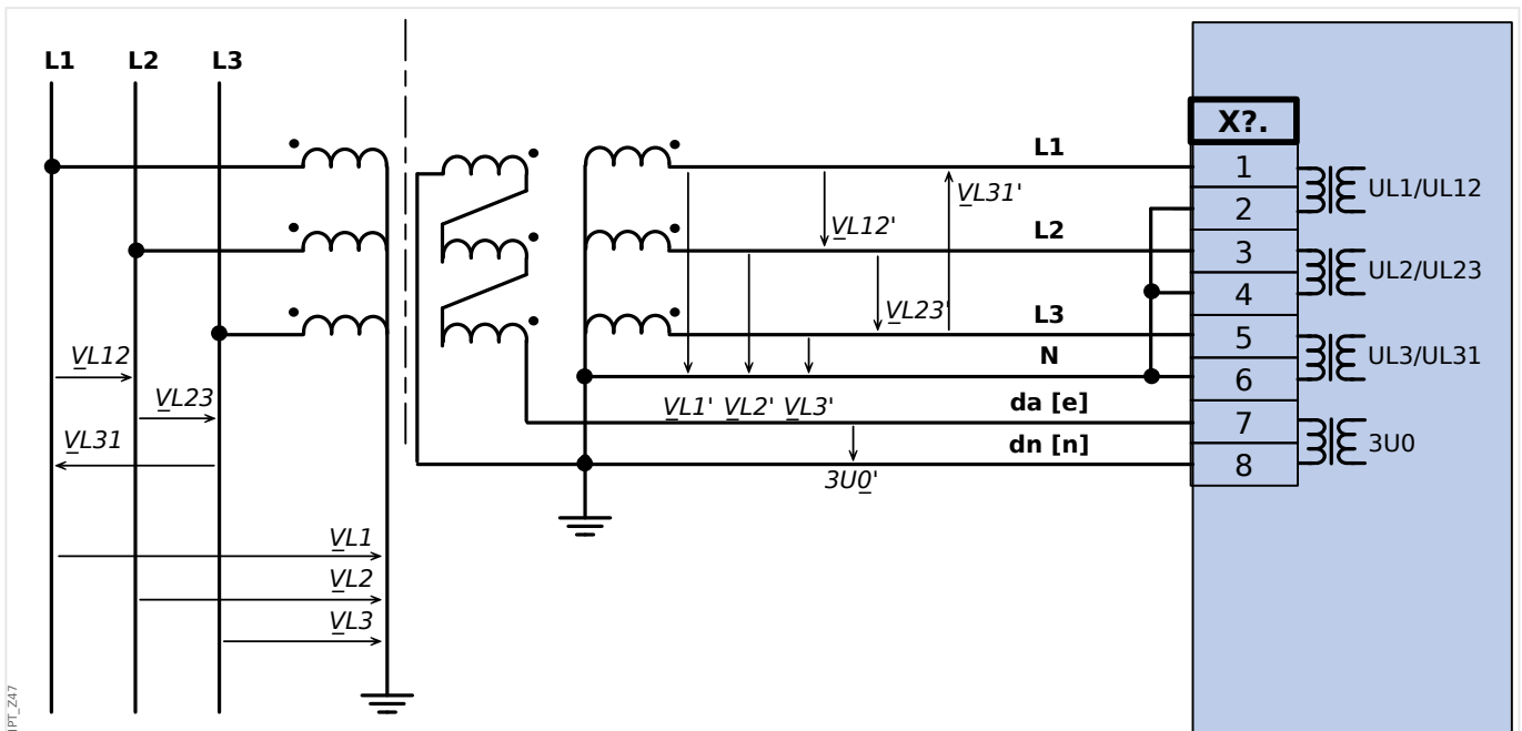
Rys. 29: Przekładnik napięciowy połączony w gwiazdę z otwartym trójkątem.
