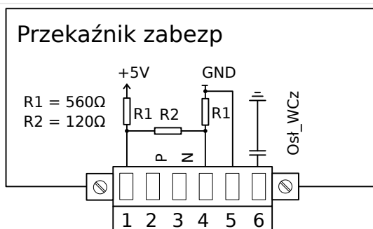
Rys. 43: Przypisanie elektromechaniczne
