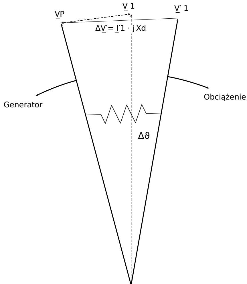
Rys. 89: Wektory napięcia przy awarii sieci.
