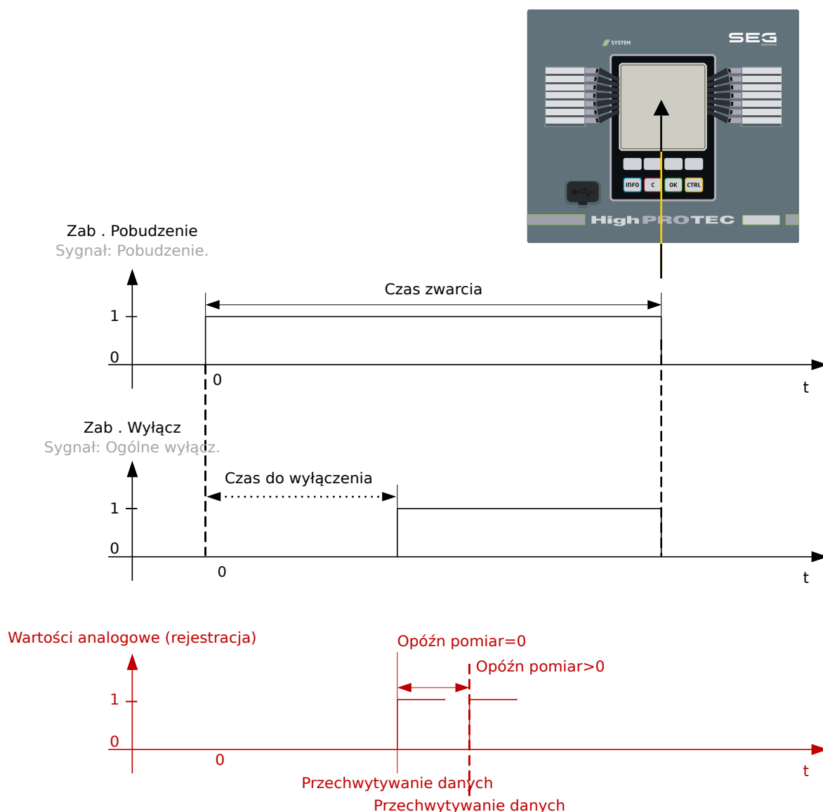
Rys. 109: Rejestrator zwarć: czasy (trwania).
