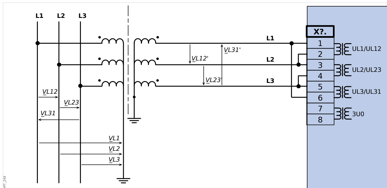
Rys. 30: Trójfazowy pomiar napięcia w układzie trójkąta: połączenie przewodów wejść pomiarowych: "połączenie w trójkąt"
