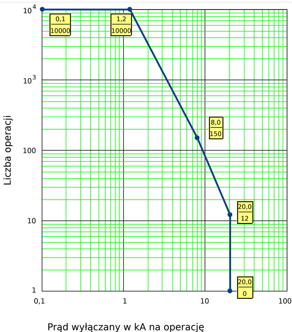
Rys. 104: Krzywa konserwacji wyłącznika typowego wyłącznika 25 kV
