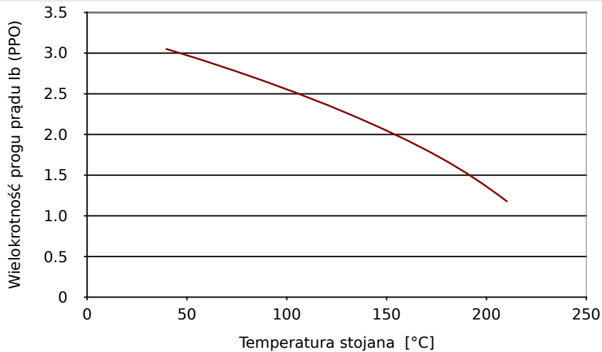
Rys. 64: Próg prądu skutecznego w stosunku do maksymalnej temperatury stojącej.
