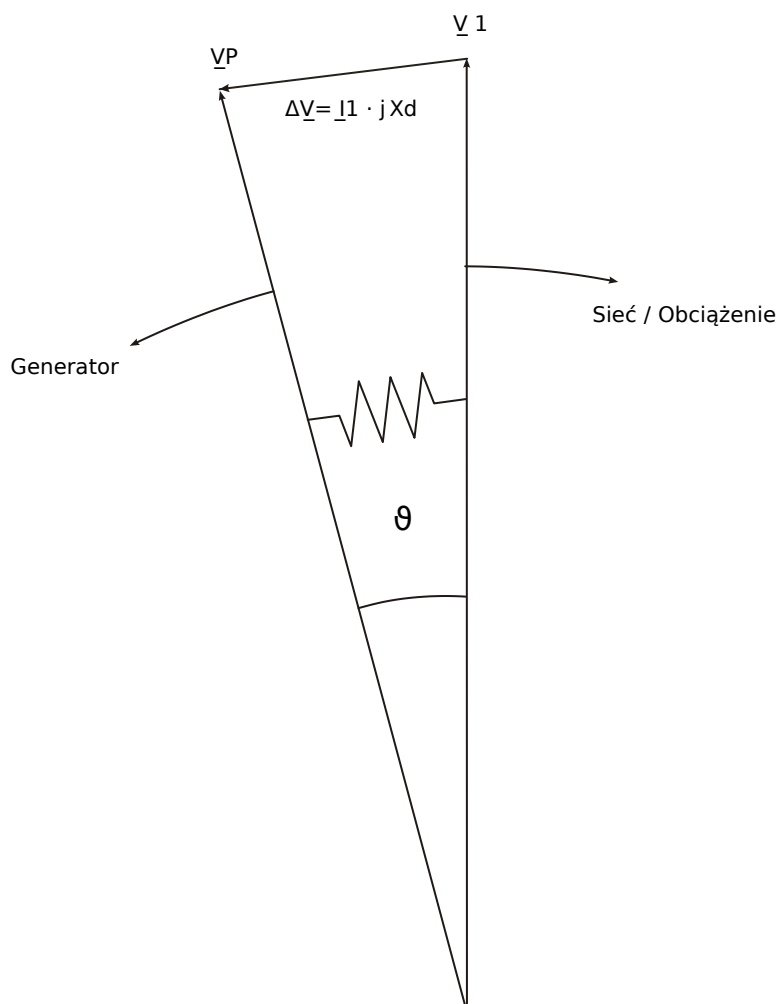
Rys. 87: Wektory napięcia przy pracy równoległej z siecią.
