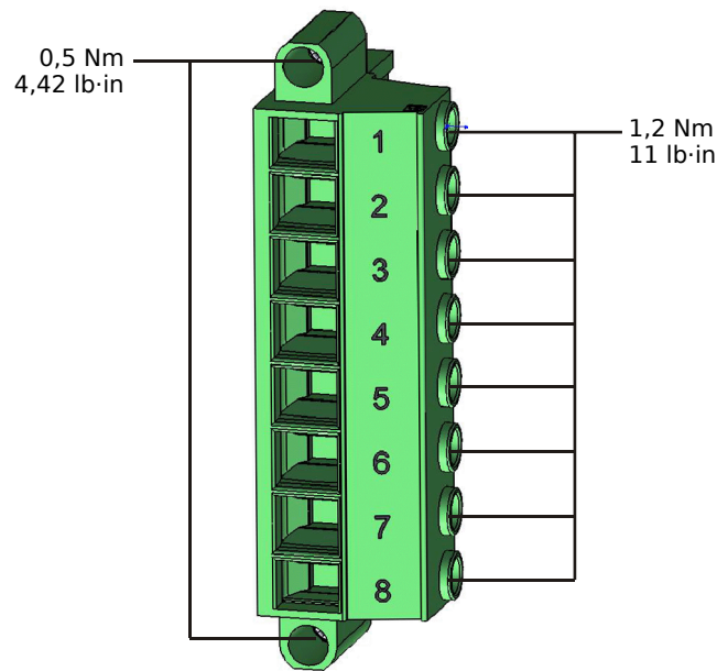
Fig. 118: Bornes de mesure de tension de la carte de mesure « TU » (↳ « 3.6.1 TU - Entrées de mesure de tension »).
