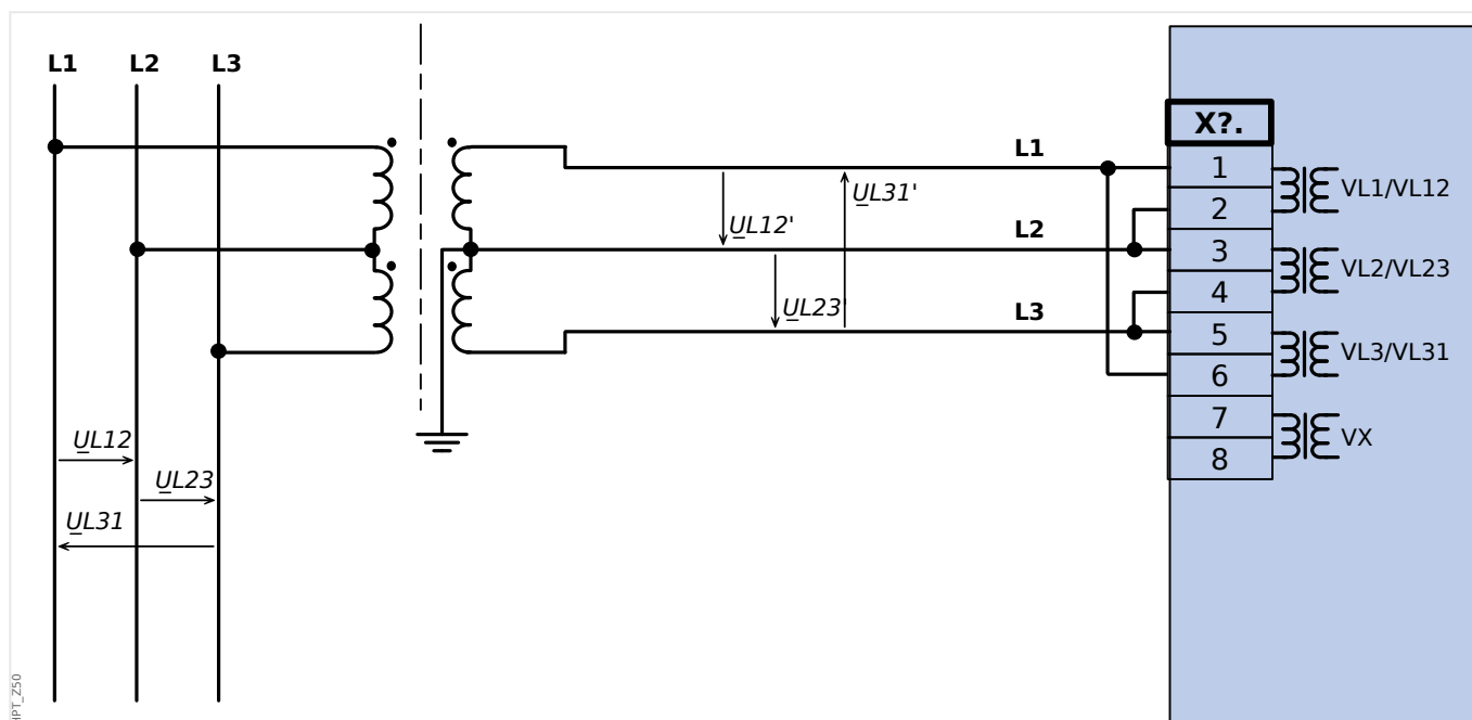
Fig. 32: Mesure de tension biphasée - câblage des entrées de mesure: "Triang ouv"
