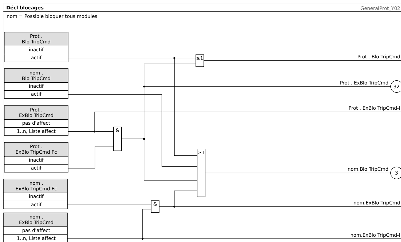
Fig. 59: Activation ou désactivation de la commande de déclenchement d'un module de protection
