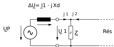
Fig. 86: Circuit équivalent au niveau du générateur synchrone en parallèle avec le réseau.
