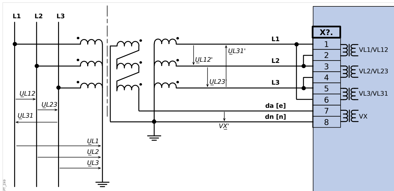
Fig. 31: Mesure de tension triphasée - câblage des entrées de mesure : "delta-connection" (Connexion en triangle). Mesure tension résid VG via enroults auxiliaires (e-n) "triangle fermé"
