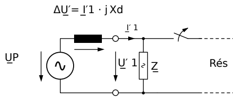
Fig. 88: Circuit équivalent en cas de coupure de réseau.
