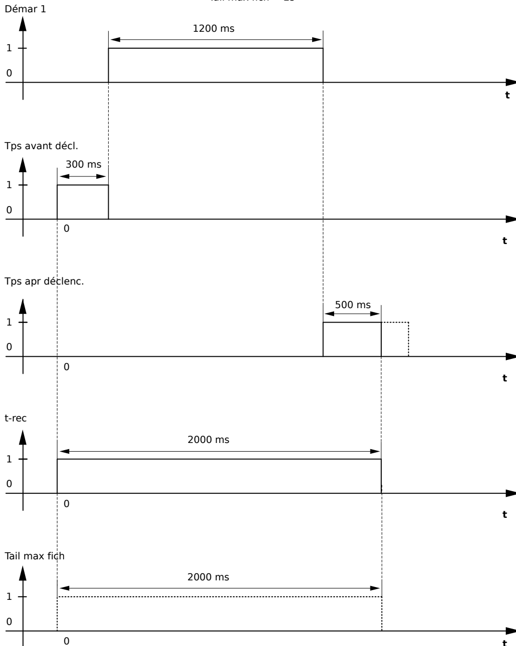
Fig. 107: Exemple de diagramme des temps de l'enregistreur de perturbations I
