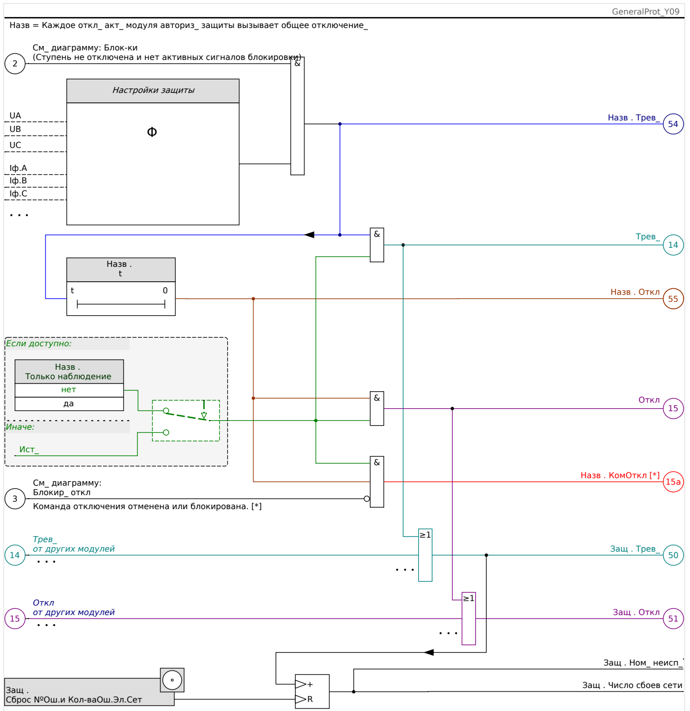
Рис. 57: Примерная схема функций любого элемента защиты HighPROTEC.
