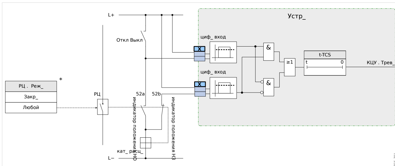
Рис. 84: Пример соединения: контроль цепи отключения с двумя вспомогательными контактами выключателя «Всп Вкл» (52a) и «Всп Выкл» (52b).
