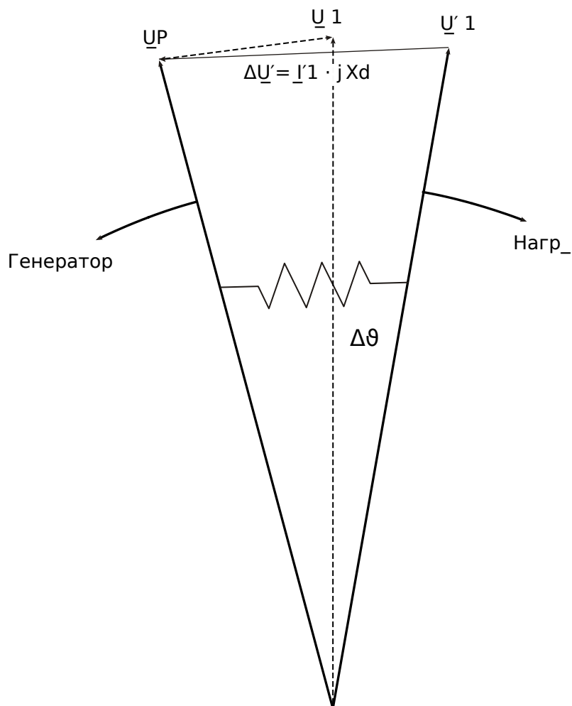
Рис. 78: Векторы напряжения при сбое электросети.
