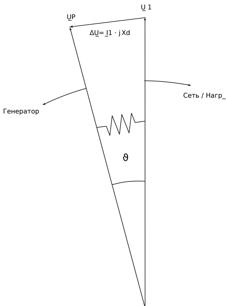
Рис. 76: Векторы напряжения в параллельной работе с электросетью.
