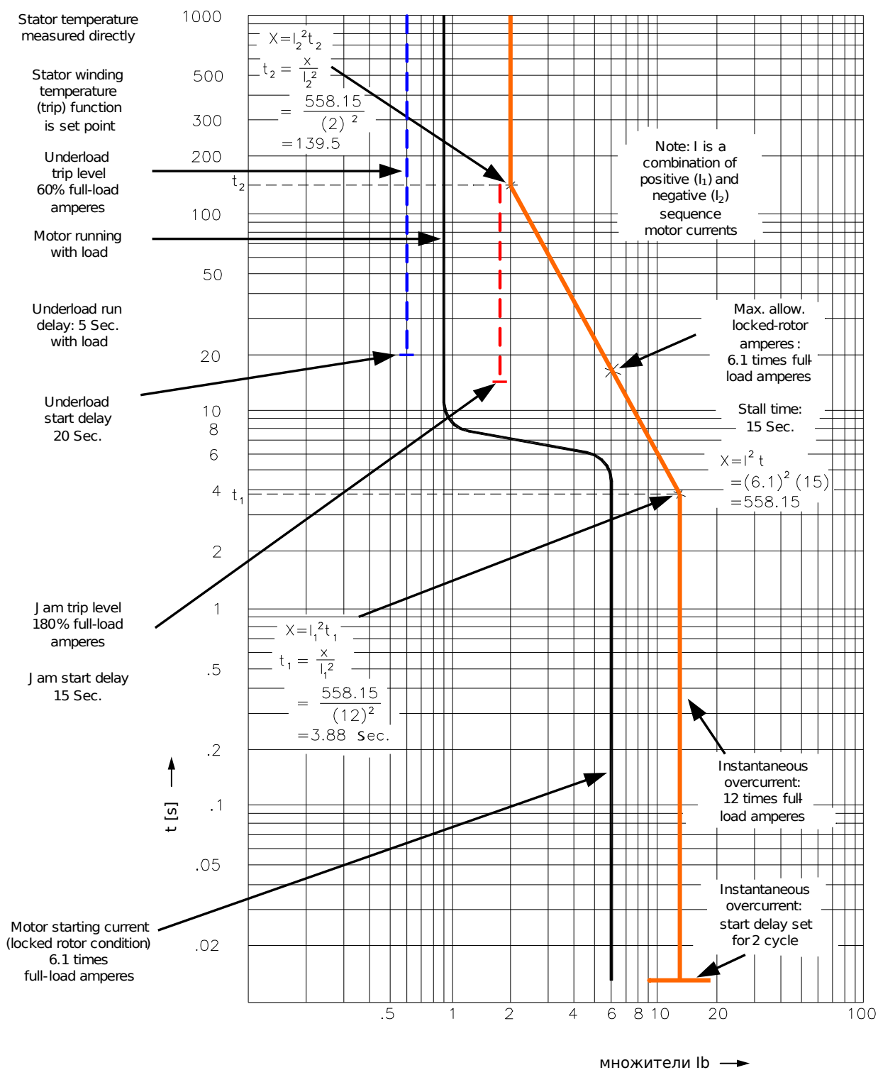
Рис. 6б: Кривая защиты двигателя (пример 3 — с ТДС).
