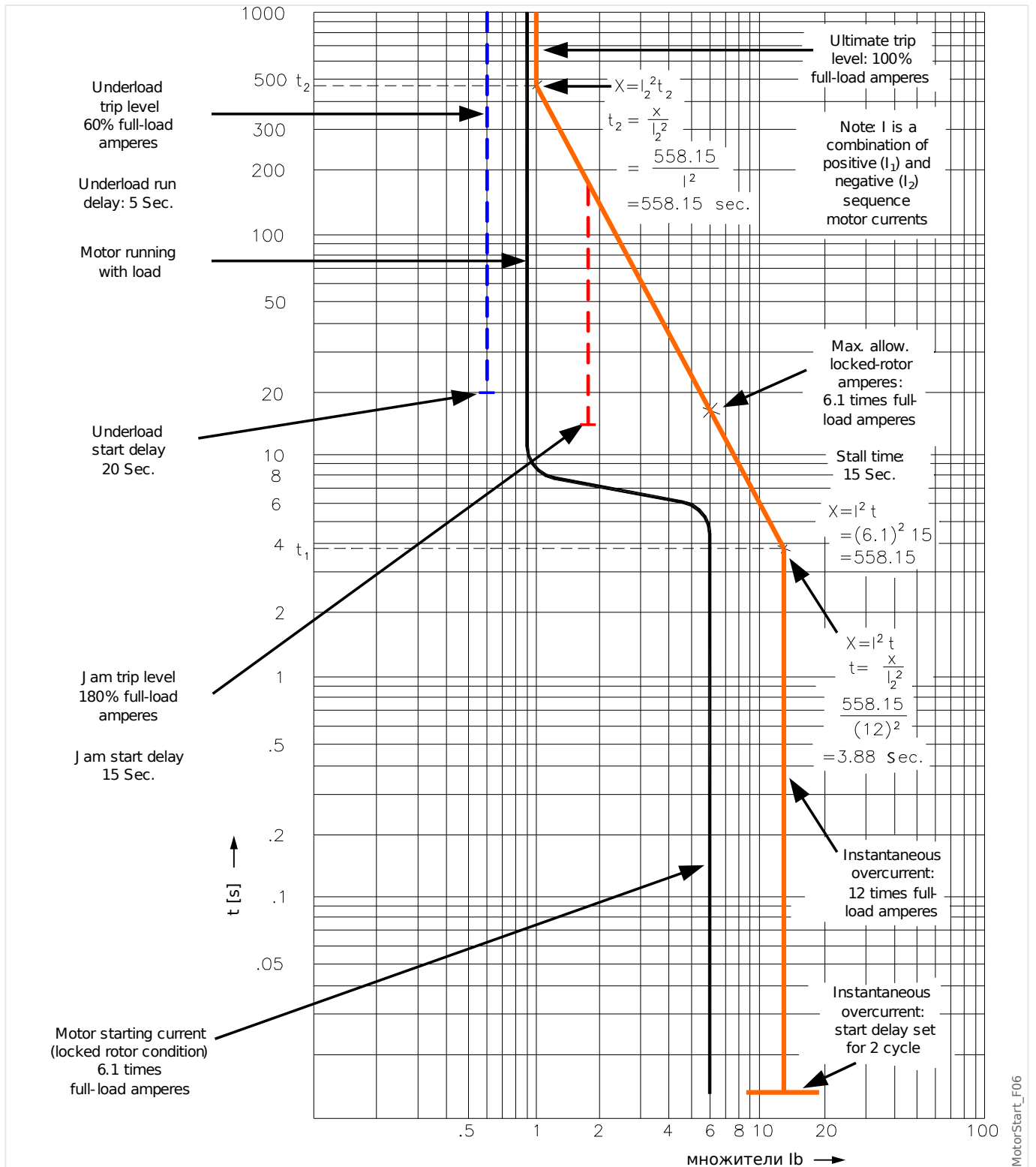
Рис. 65: Кривая защиты двигателя (пример 2 — без ТДС).
