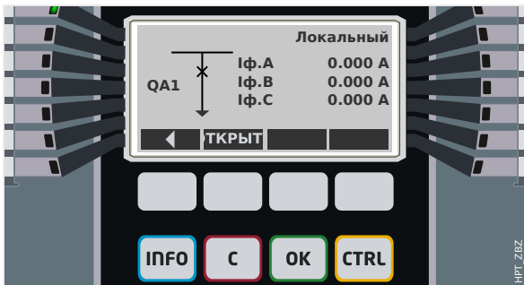
Рис. 88: Пример страницы управления, выключатель в замкнутом положении.
