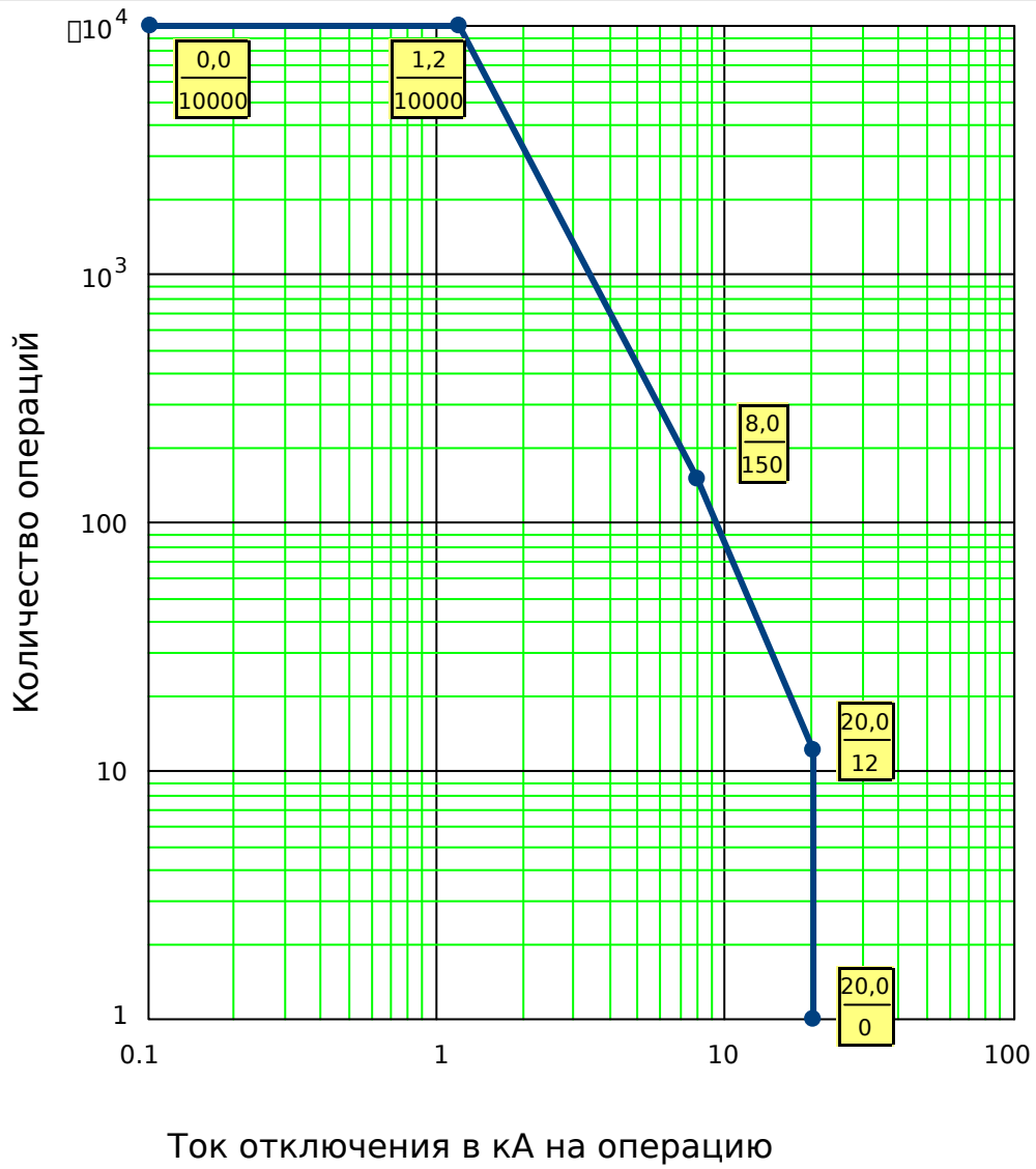
Рис. 93: Эксплуатационная кривая выключателя для типичного выключателя 25кВ
