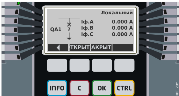
Рис. 89: Пример страницы управления, выключатель в аварийном (недопустимое состояние) положении.
