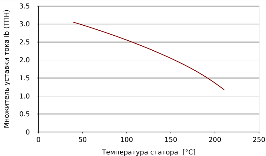
Рис. 61: Эффективная уставка тока по ср. с максимальной температурой статора.
