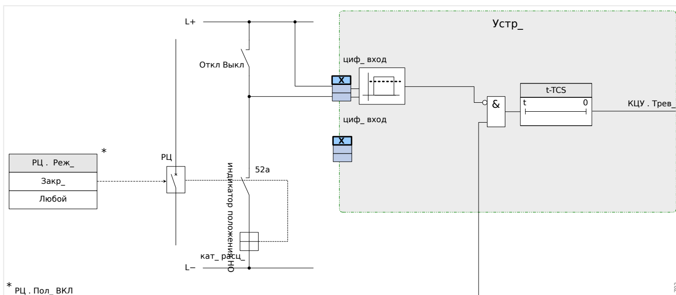
Рис. 85: Пример соединения: контроль цепи отключения только с одним вспомогательным контактом выключателя «Всп Вкл» (52a).
