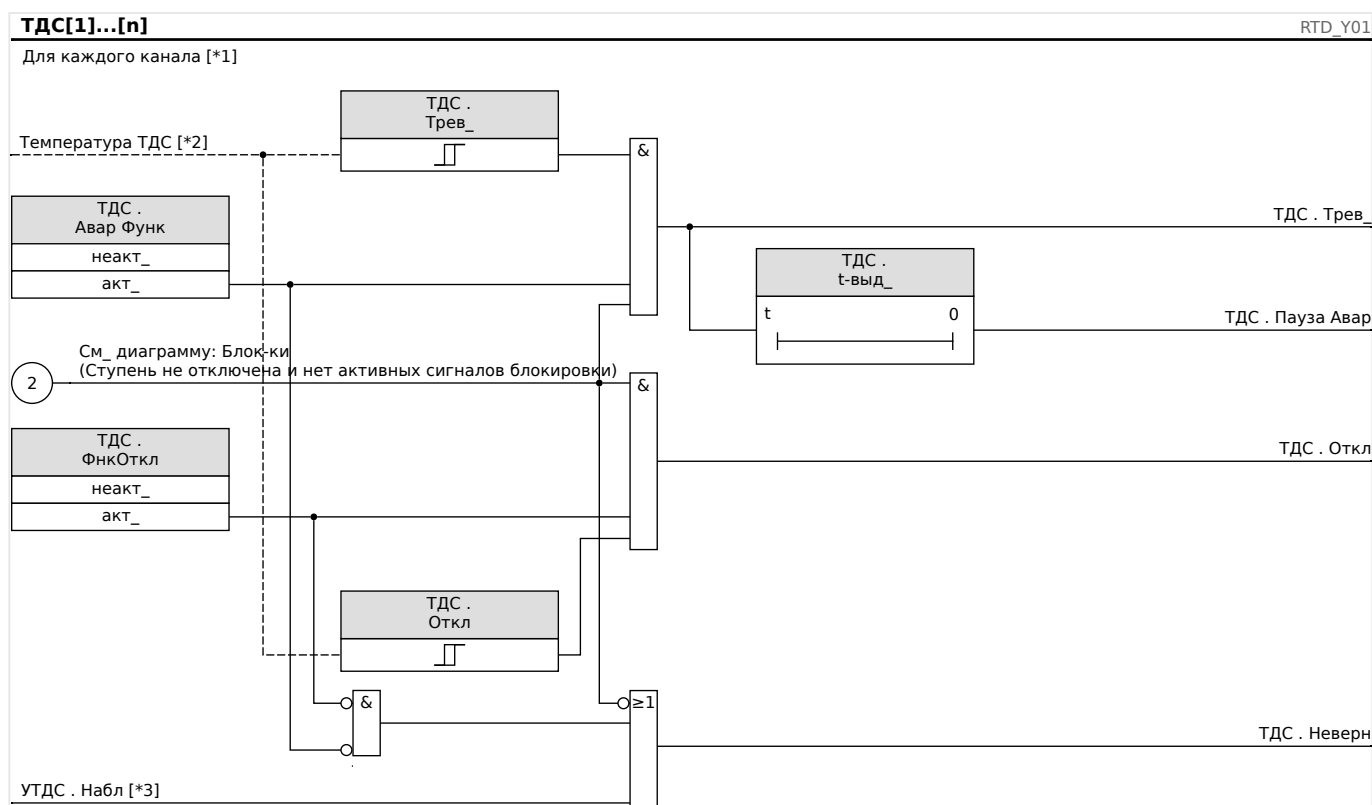
Рис. 83: Общий принцип работы (аварийный сигнал с задержкой, отключение без задержки).
