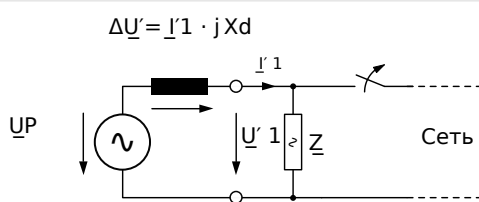
Рис. 77: Эквивалентная цепь при сбое электросети.
