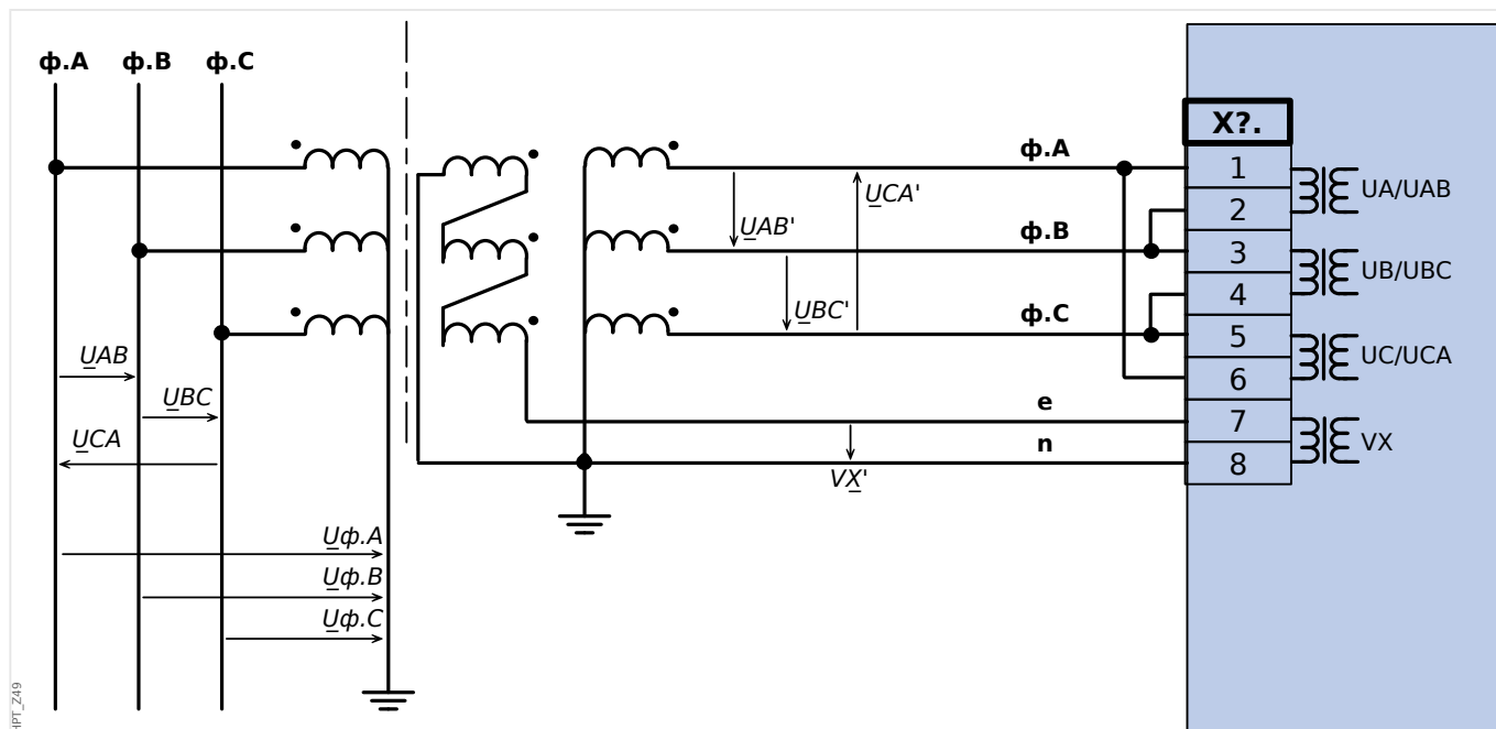
Рис. 31: Измерение трехфазного напряжения - схема измерительных входов: "соединение треугольником" Измерение напряжения нулевой последовательности V_G через вспомогательные обмотки (e-n) («открытый треугольник»)
