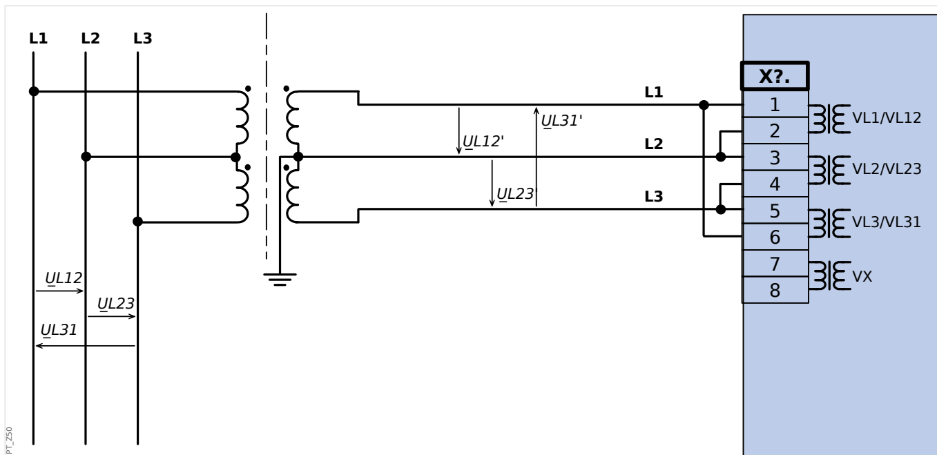
Fig. 32: Mesure de tension biphasée - câblage des entrées de mesure: "Triangle ouvert"
