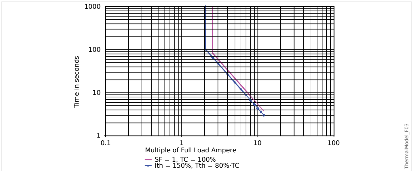
Fig. 63: Limite du modèle img thermique et courbes de déclenchement avec RTD =100°C
