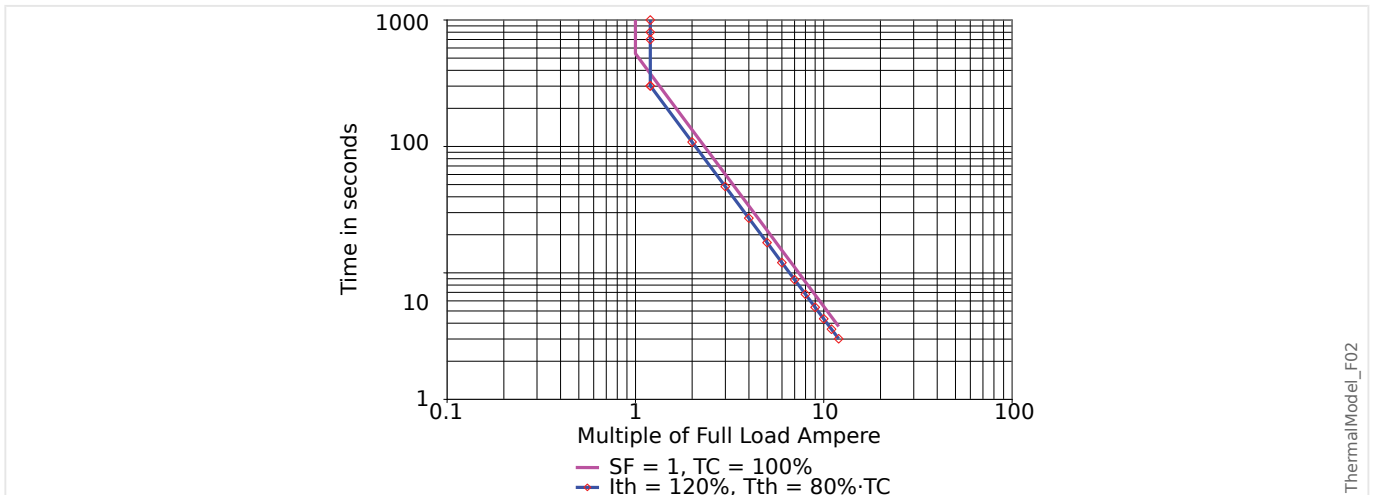
Fig. 62: Limite du modèle Img thermique et courbes de déclenchement sans dét RTD.
