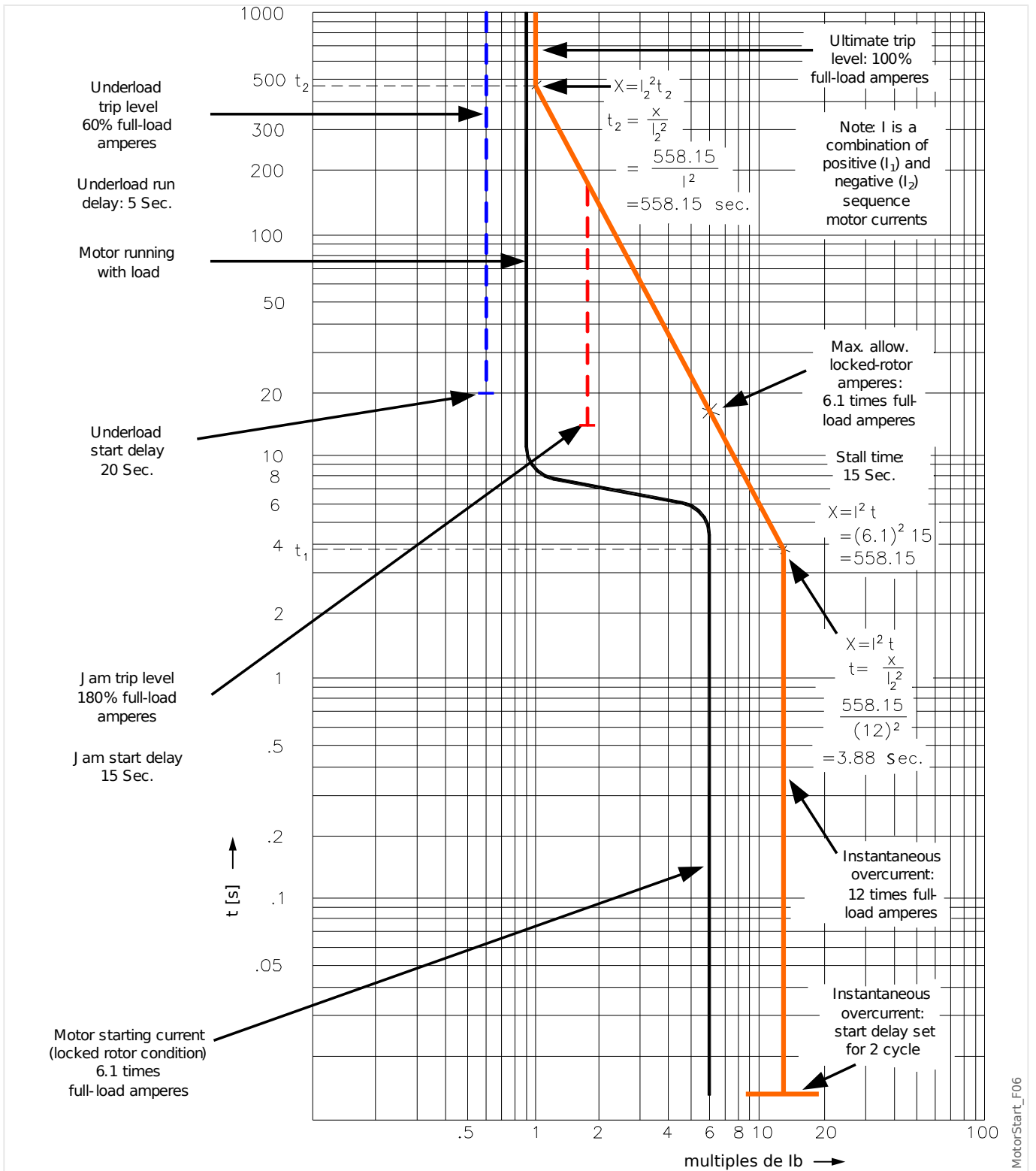
Fig. 65: Courbe de protection du moteur (exemple 2 - sans thermomètres à résistance).
