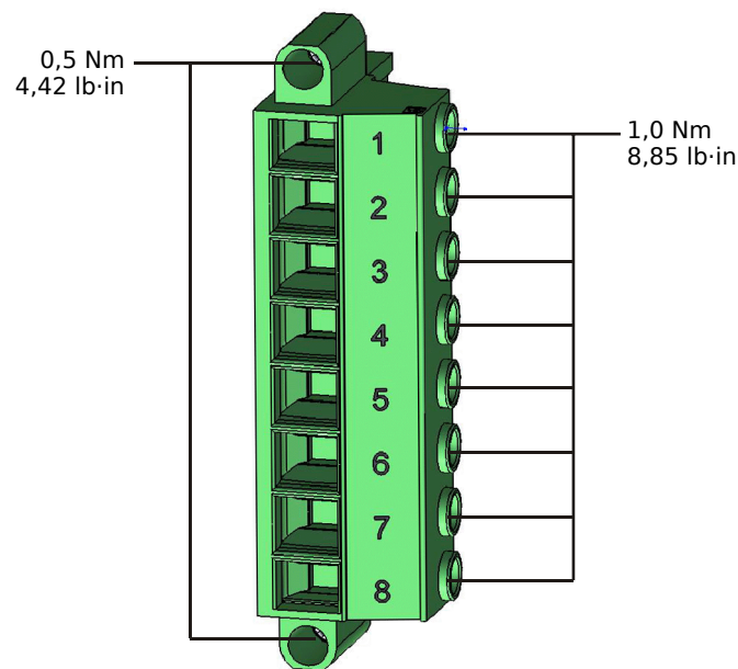
Fig. 109: Bornes de mesure de tension de la carte de mesure « TU » (↳ « TU - Entrées de mesure de tension »).
