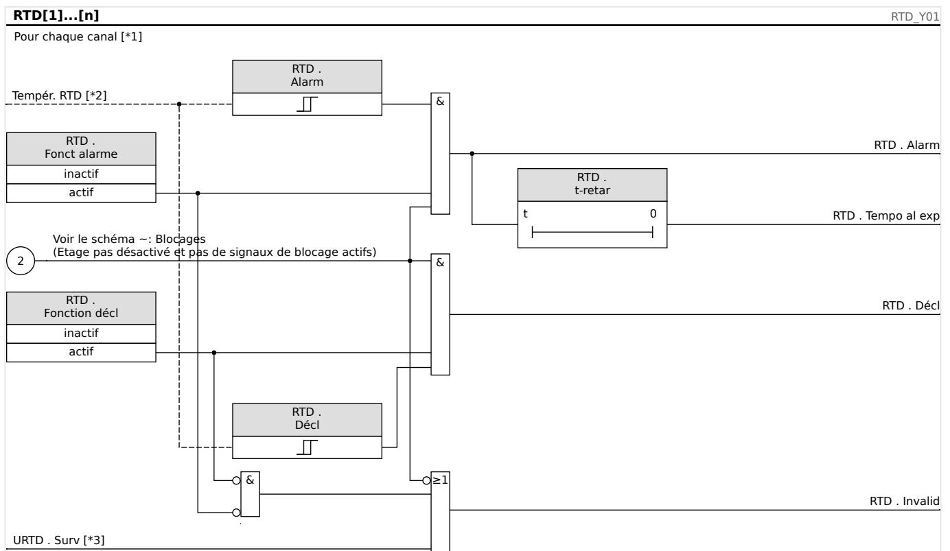
Fig. 83: Principe de fonctionnement général (alarme retardée, déclenchement non retardé).
