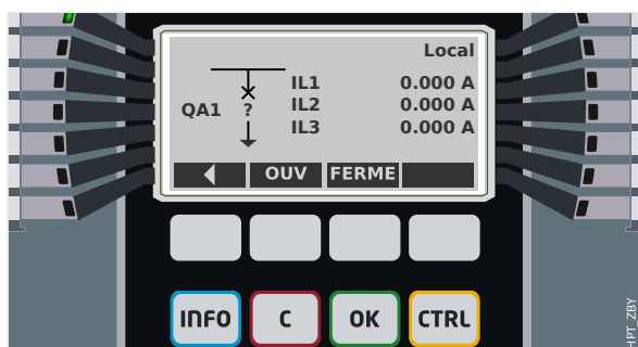
Fig. 89: Exemple de page de contrôle, avec le « disjoncteur » en position de dysfonctionnement (ou invraisemblable).
