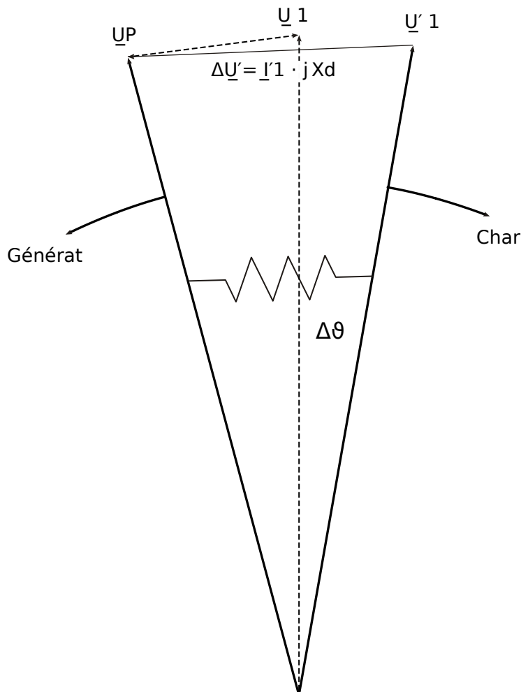
Fig. 78: Vecteurs de tension en cas de coupure de réseau.
