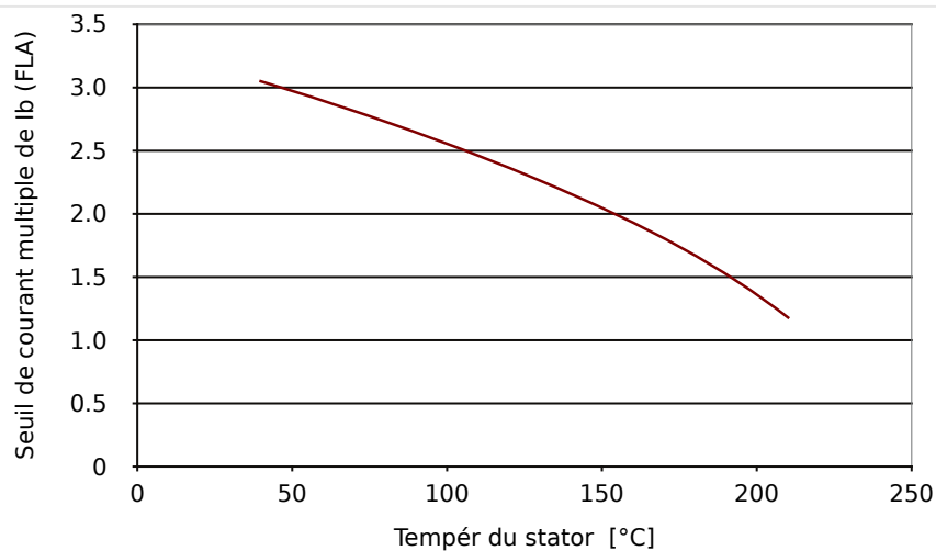
Fig. 61: Seuil de courant efficace / Tempér maxi du stator.
