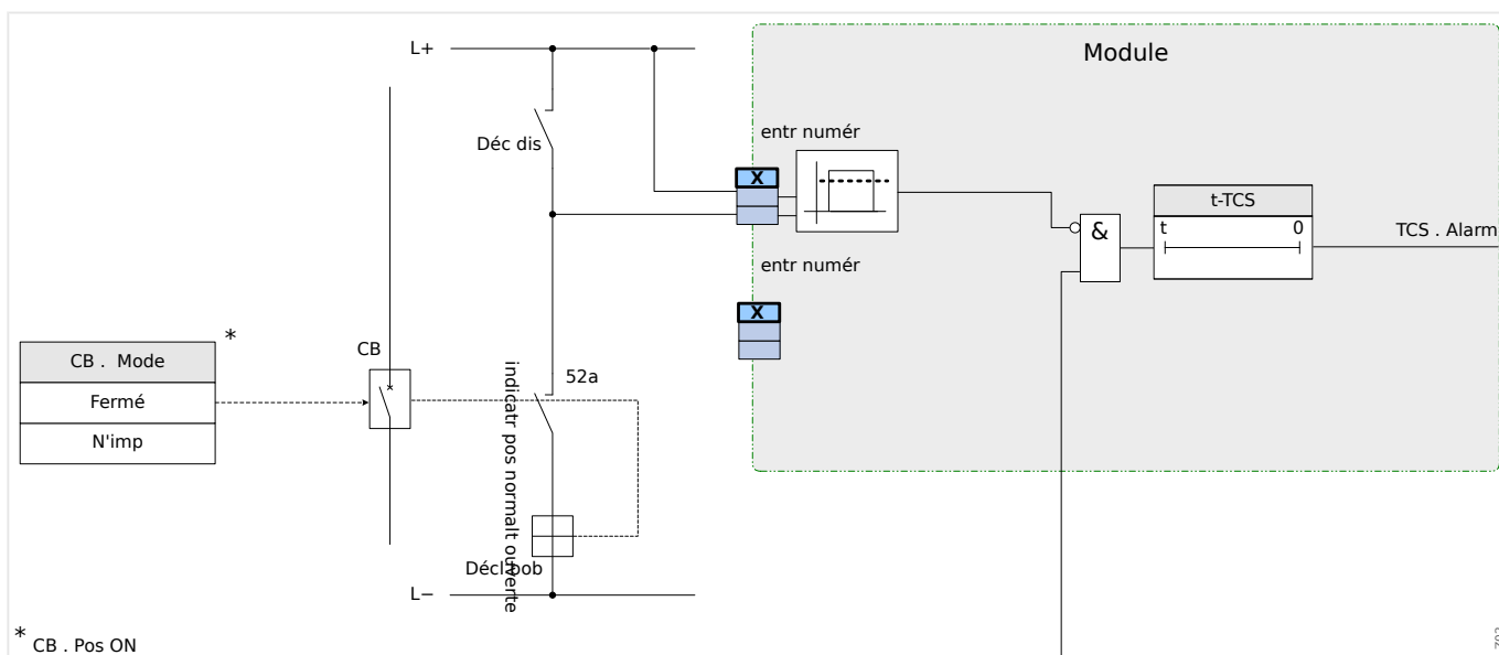
Fig. 85: Exemple de connexion : Surveillance du circuit de déclenchement avec un contact auxiliaire de disjoncteur »Aux ON« (52a).
