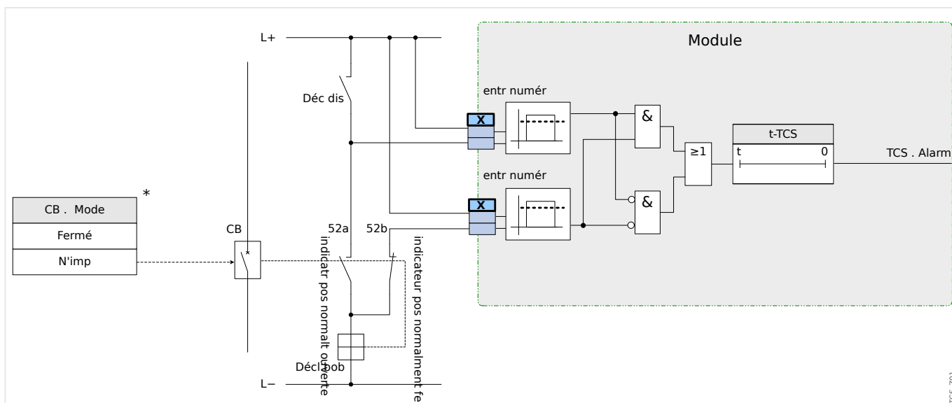
Fig. 84: Exemple de connexion : Surveillance du circuit de déclenchement avec de contacts auxiliaires de disjoncteur »Aux ON« (52a) et »Aux OFF« (52b).
