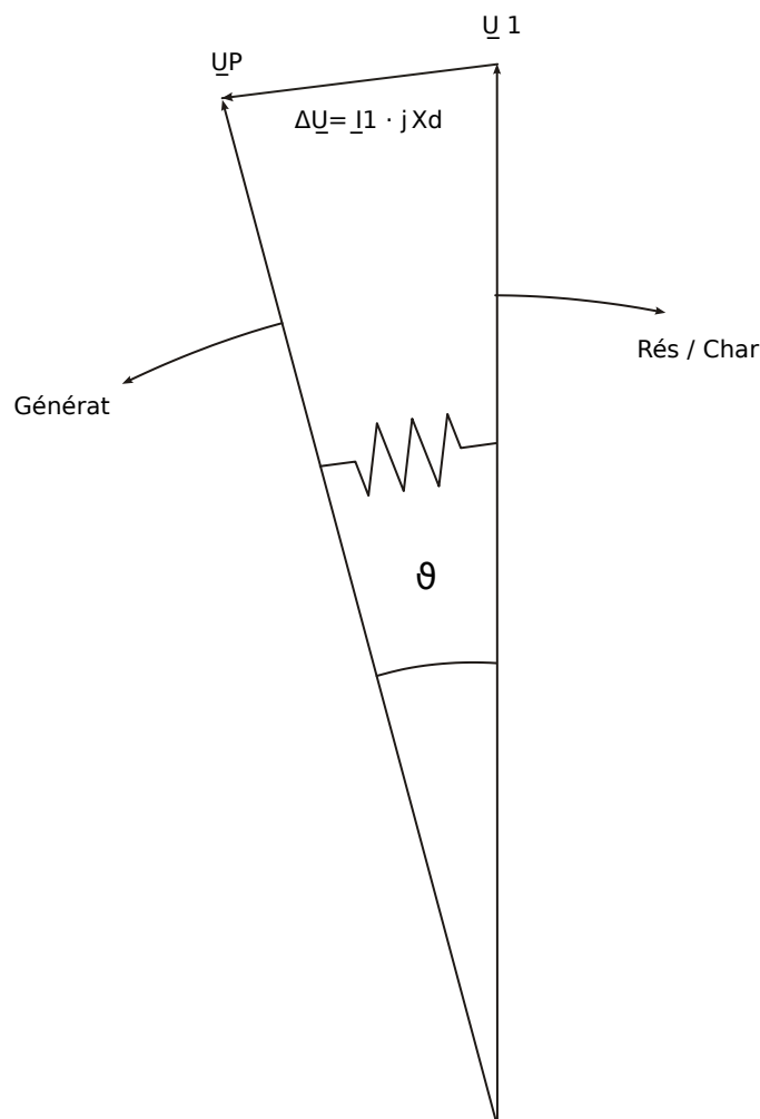
Fig. 76: Vecteurs de tension en fonctionnement parallèle du réseau.
