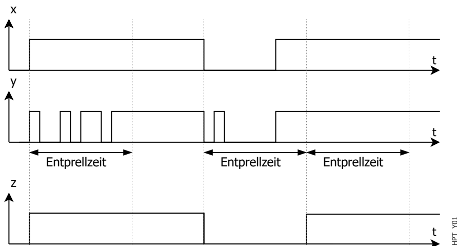
Abb. 56: Entprell-Mechanismus des MRMV4.
