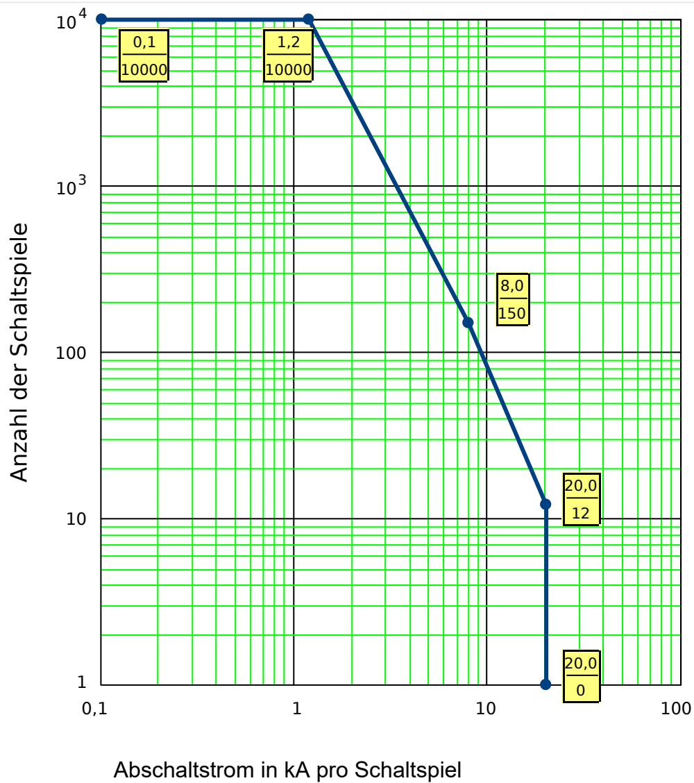
Abb. 129: Wartungskurve für einen typischen 25 kV Leistungsschalter
