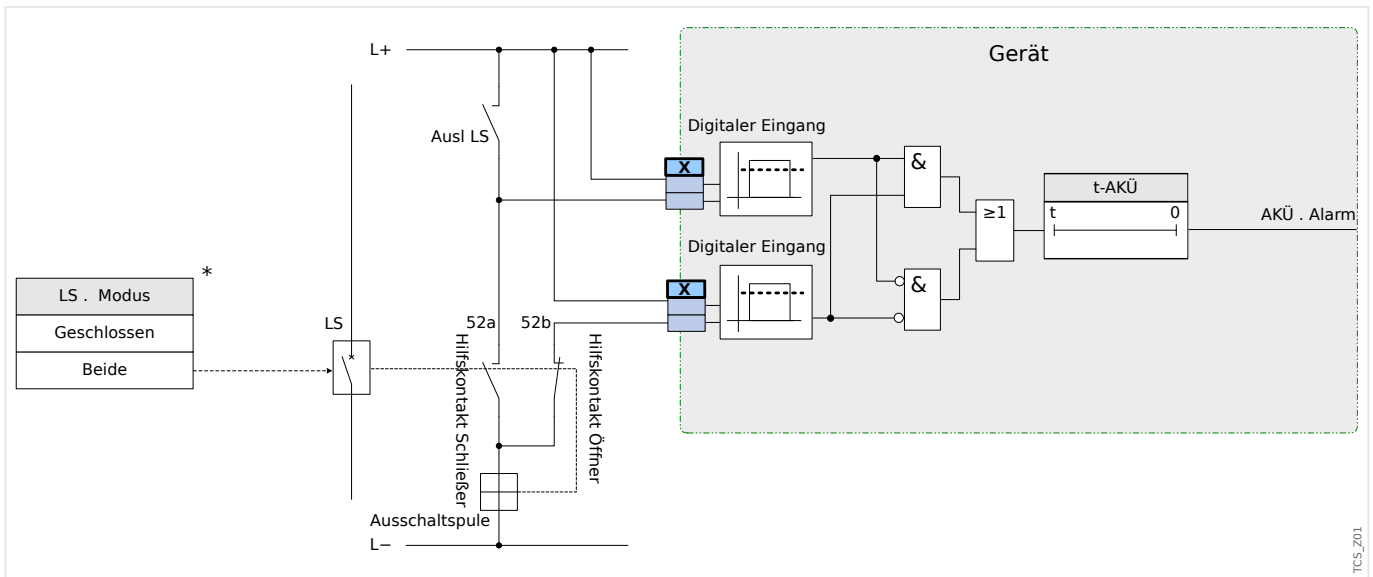
Abb. 119: Anschlussbeispiel (Empfehlung): Auslösekreisüberwachung mit zwei Hilfskontakten »Hiko EIN« (52a) und »Hiko AUS« (52b).
