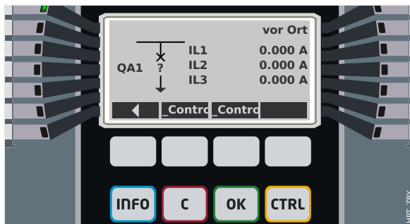
Abb. 125: Beispiel einer Steuer-Seite mit „Leistungsschalter“ in Störstellung (bzw. unplausiblem Zustand).
