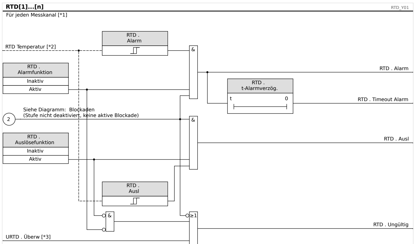
Abb. 118: Generelles RTD-Funktionsprinzip.
