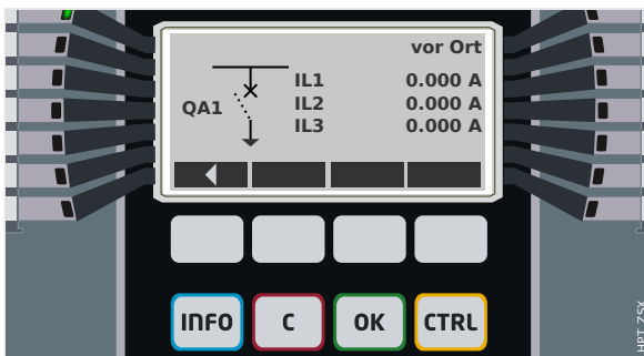
Abb. 123: Beispiel einer Steuer-Seite mit „Leistungsschalter“ in Zwischenposition).
