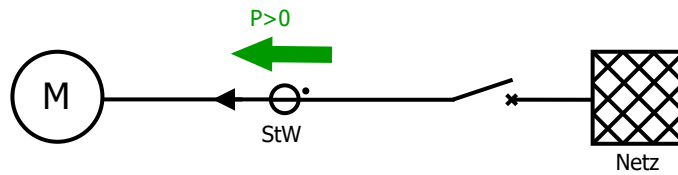
Abb. 115: Richtungsdefinition der Leistung beim MRMV4.
