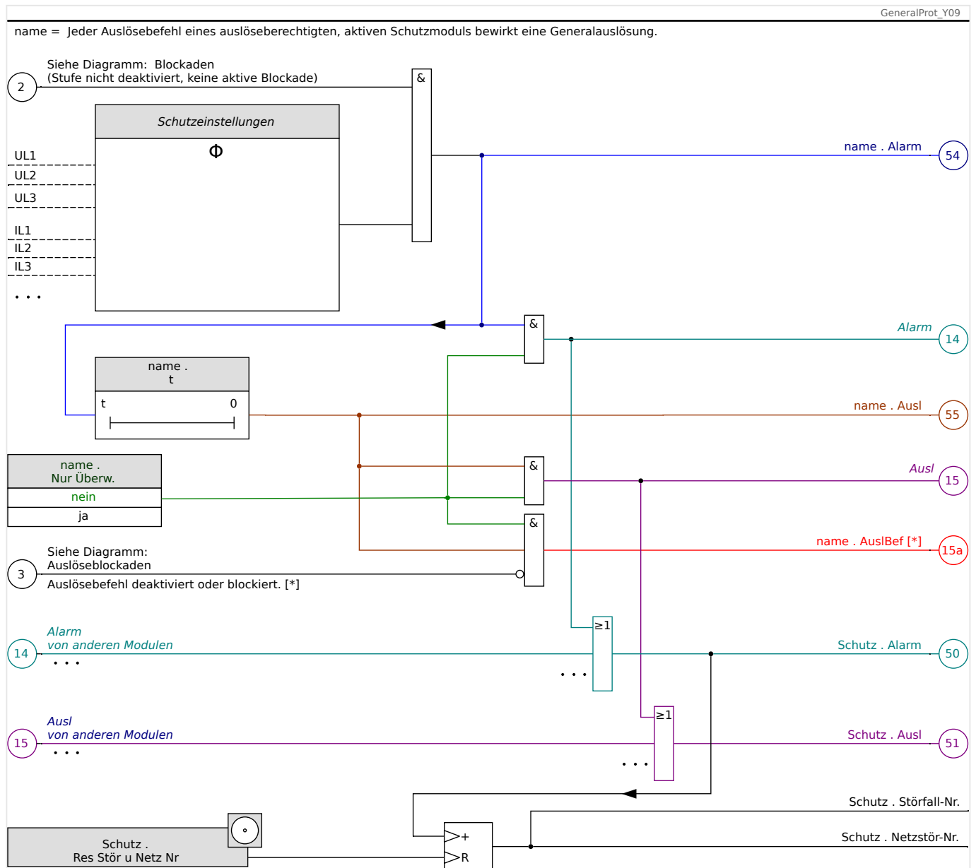
Abb. 64: Grobe Skizze der Funktionalität einer HighPROTEC-Schutzfunktion.
