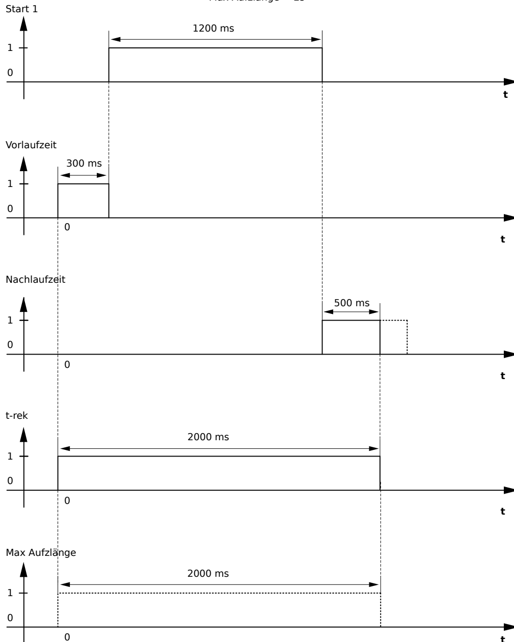
Abb. 132: Beispiel I Störschreiber-Ablaufdiagramm
