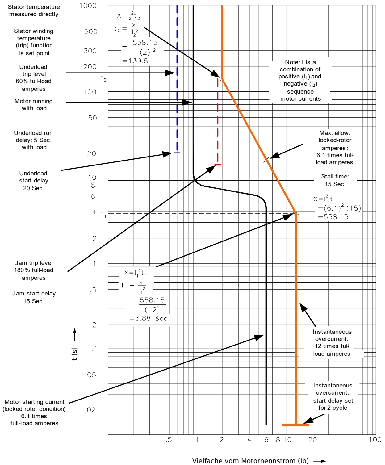
Abb. 75: Auslösekennlinien (Beispiel 3 - mit RTDs).
