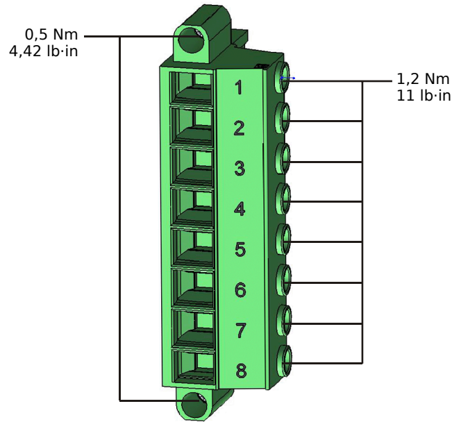
Abb. 144: Spannungsmessstecker der Spannungsmesskarte „TU“ (↔3.6.1 TU - Spannungsmesseingänge).
