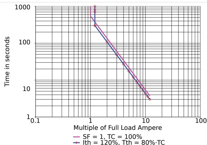
Abb. 71: Thermisches Abbild und Auslösecharakteristik ohne RTD.
