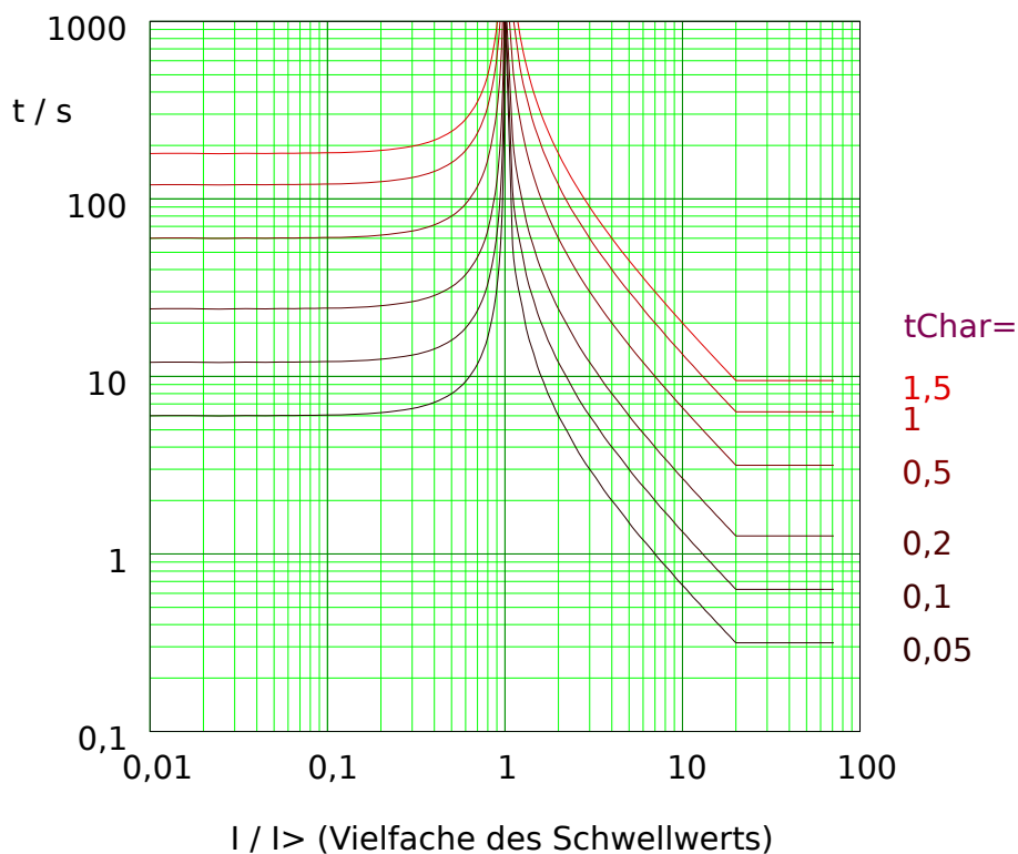
Abb. 81: LINV: Rückfallverzögerung (linke Hälfte, I < I_n ) und Auslöseverzögerung (rechte Hälfte, I > I_n ), Beispieldiagramm für I_{max} = 20 \cdot I_n .
