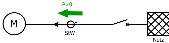
Abb. 110: Richtungsdefinition der Leistung beim MRMV4.
