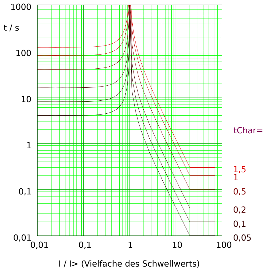
Abb. 75: EINV: Rückfallverzögerung (linke Hälfte, I < I_{>} ) und Auslöseverzögerung (rechte Hälfte, I > I_{>} ), Beispieldiagramm für I_{max} = 20 \cdot I_{>} .
