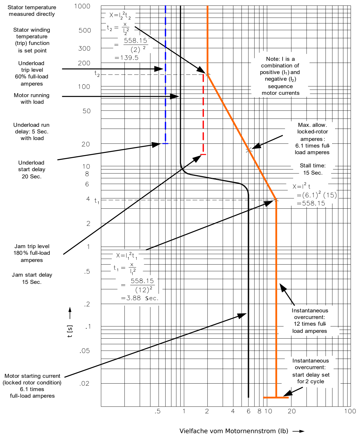
Abb. 70: Auslösekennlinien (Beispiel 3 - mit RTDs).
