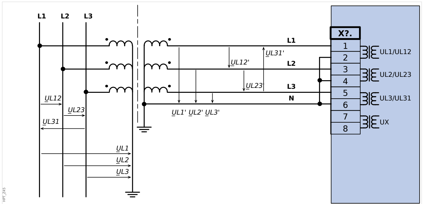
Abb. 28: Drei Spannungswandler mit Geräteanschluss in Sternschaltung
