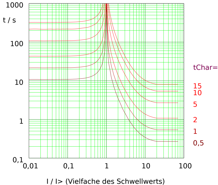
Abb. 79: VINV: Rückfallverzögerung (linke Hälfte, I < I_{>} ) und Auslöseverzögerung (rechte Hälfte, I > I_{>} ), Beispieldiagramm für I_{max} = 20 \cdot I_{>} .
