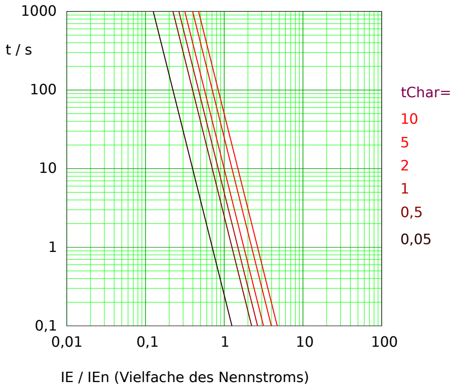
Abb. 97: Auslösekurve „I4T“, wobei nur der Bereich IE > I_{E>} jeweils anwendbar ist. Beispieldiagramm für gemessenen (nicht empfindlichen) Erdstrom.
