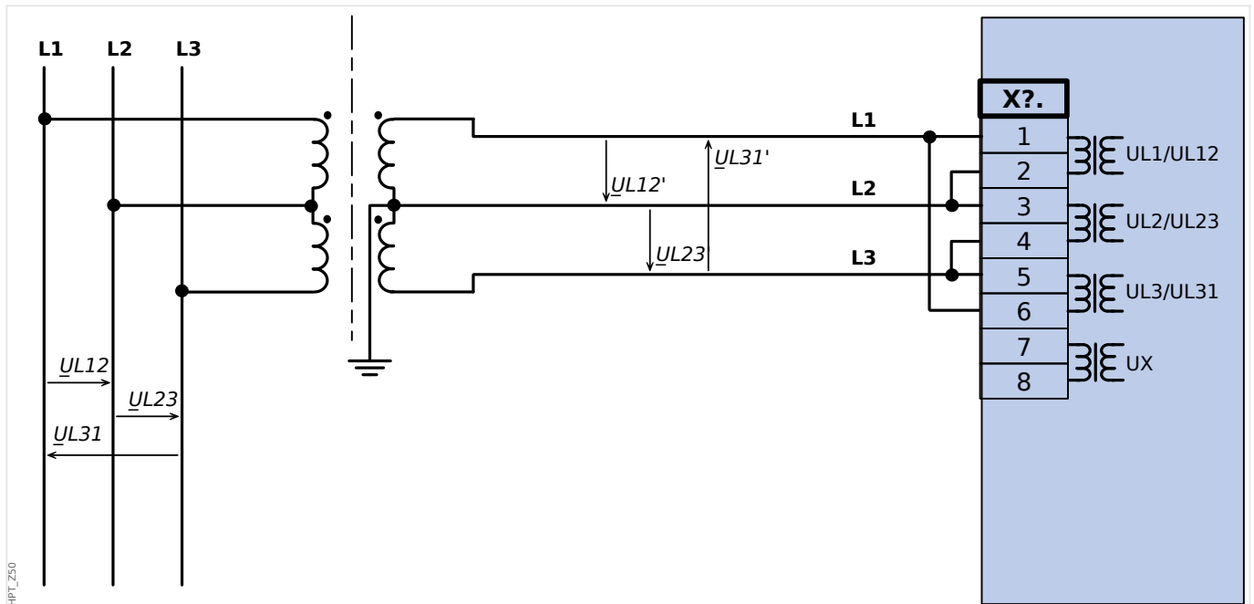
Abb. 32: Zwei Spannungswandler mit Geräteanschluss in V-Schaltung
