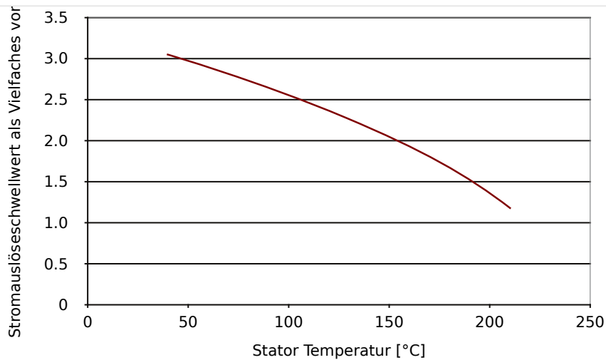
Abb. 65: Stromauslöseschwellwerte (Effektivwerte) über der maximalen Statortemperatur.
