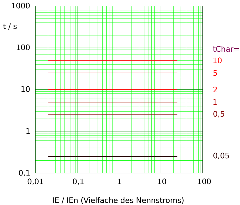
Abb. 94: Auslösekurve „Therm Flat“, wobei nur der Bereich IE > I_{E>} jeweils anwendbar ist. Beispieldiagramm für gemessenen (nicht empfindlichen) Erdstrom.
