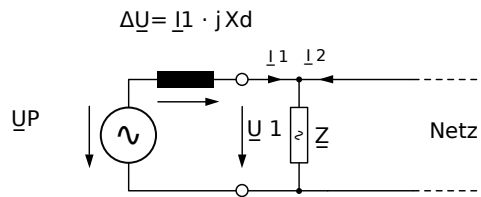
Abb. 104: Ersatzschaltbild netzparalleler Synchrongenerator
