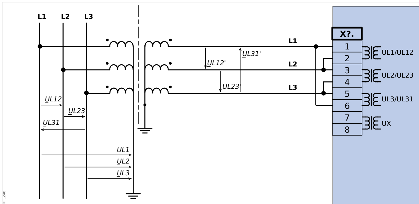
Abb. 30: Drei Spannungswandler mit Geräteanschluss in Dreieckschaltung
