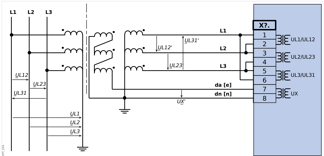
Abb. 31: Drei Spannungswandler mit Geräteanschluss in Dreieckschaltung Erfassung der Verlagerungsspannung UE mit offener Dreieckswicklung e-n
