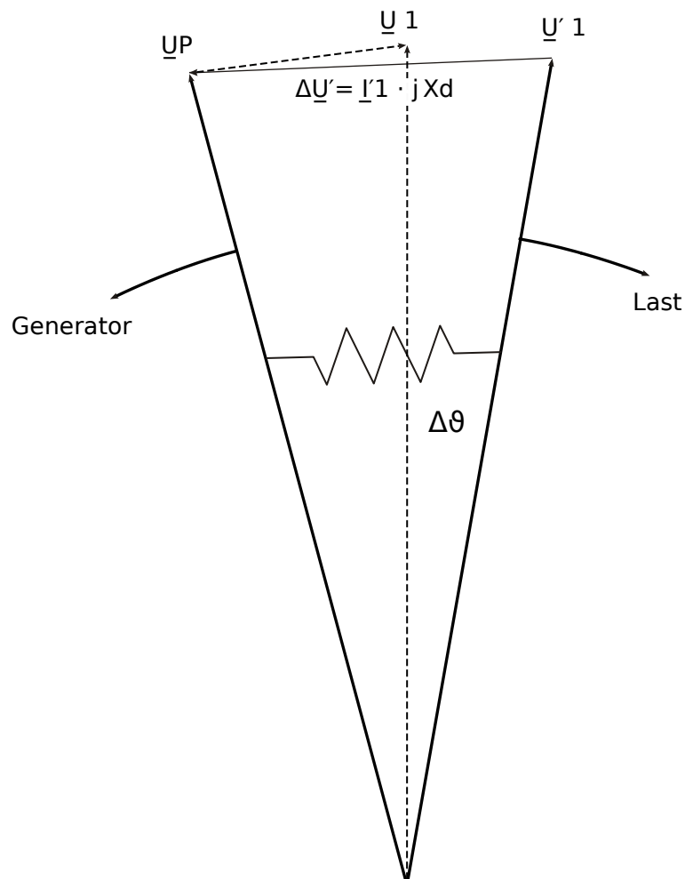
Abb. 107: Änderung des Polradwinkels bei plötzlicher Belastung des Generators.
