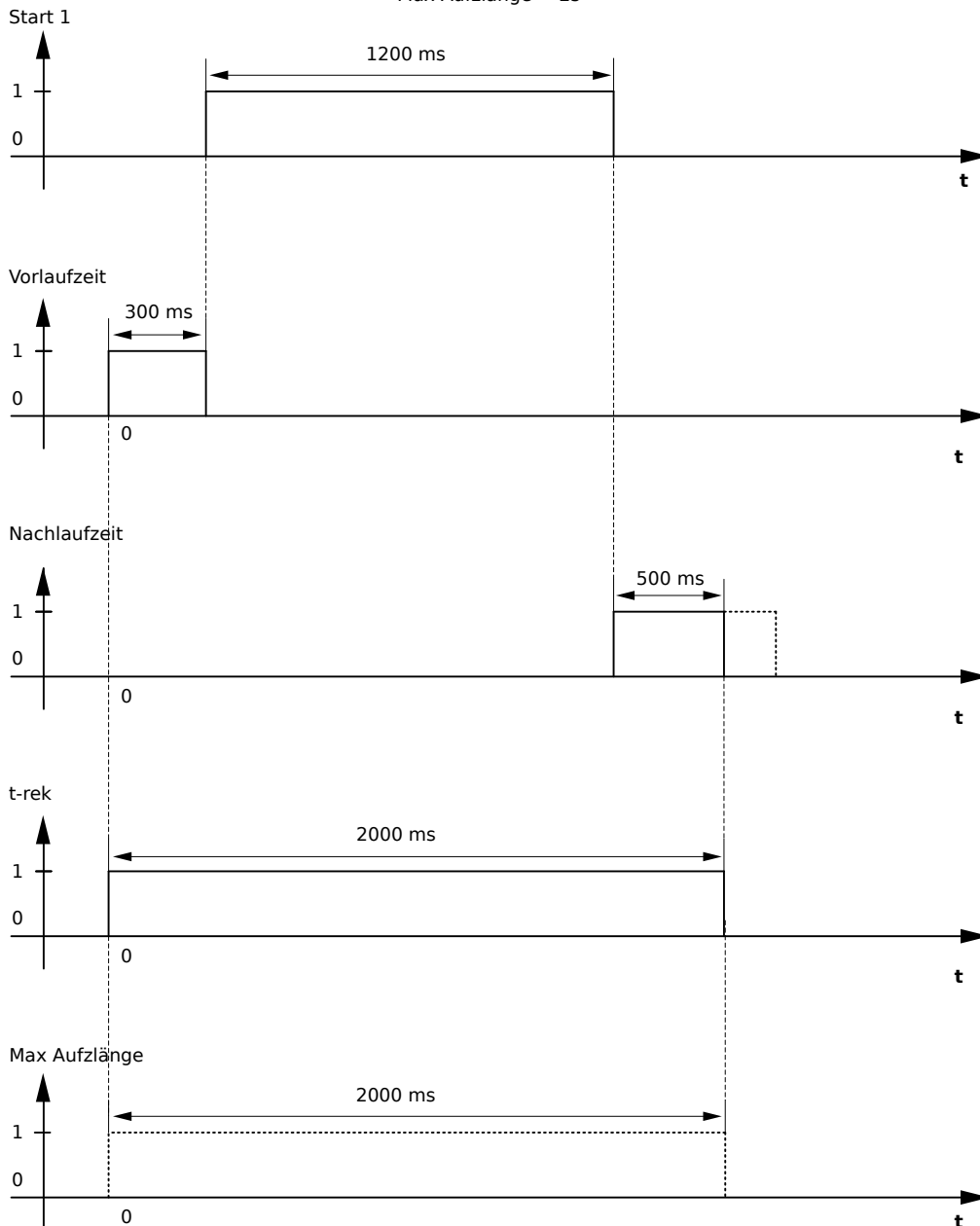
Abb. 127: Beispiel I Störschreiber-Ablaufdiagramm
