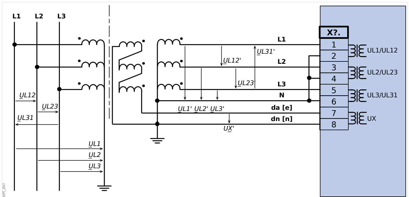
Abb. 29: Spannungswandler mit Geräteanschluss in offener Dreieckschaltung.
