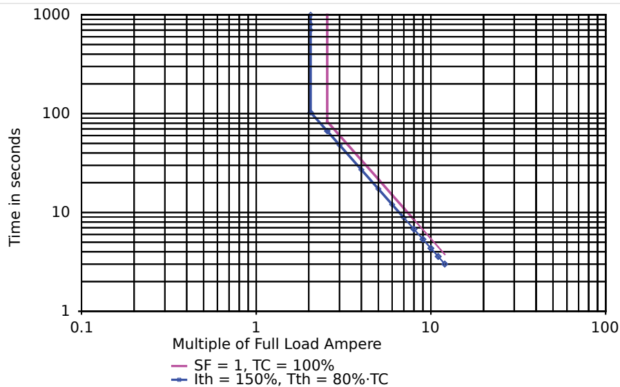
Abb. 67: Thermisches Abbild: Grenzwerte und Auslösecharakteristik mit RTD = 100°C.
