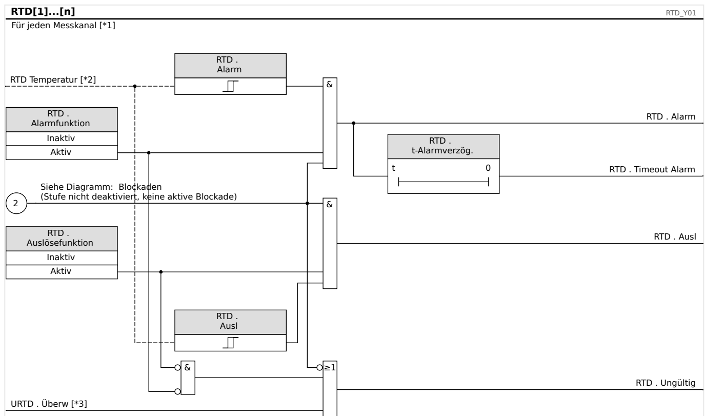
Abb. 113: Generelles RTD-Funktionsprinzip.
