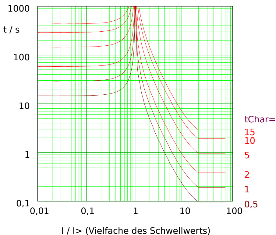
Abb. 80: EINV: Rückfallverzögerung (linke Hälfte, I < I_{>} ) und Auslöseverzögerung (rechte Hälfte, I > I_{>} ), Beispieldiagramm für I_{max} = 20 \cdot I_{>} .
