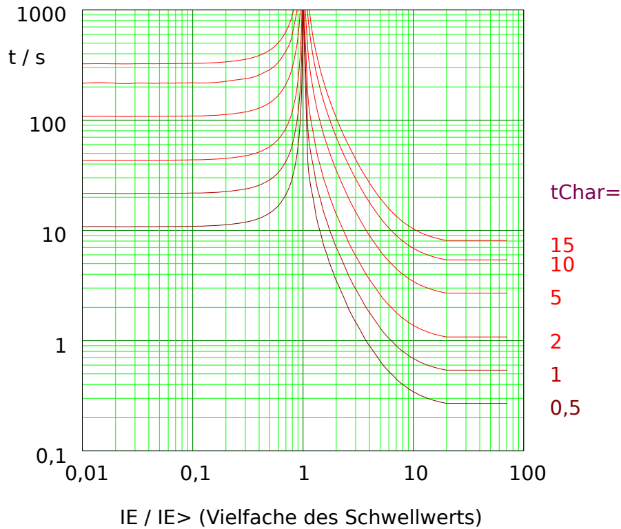
Abb. 91: VINV: Rückfallverzögerung (linke Hälfte, IE < I_{E>} ) und Auslöseverzögerung (rechte Hälfte, IE > I_{E>} ), Beispieldiagramm für I_{max} = 20 \cdot I_{E>} .
