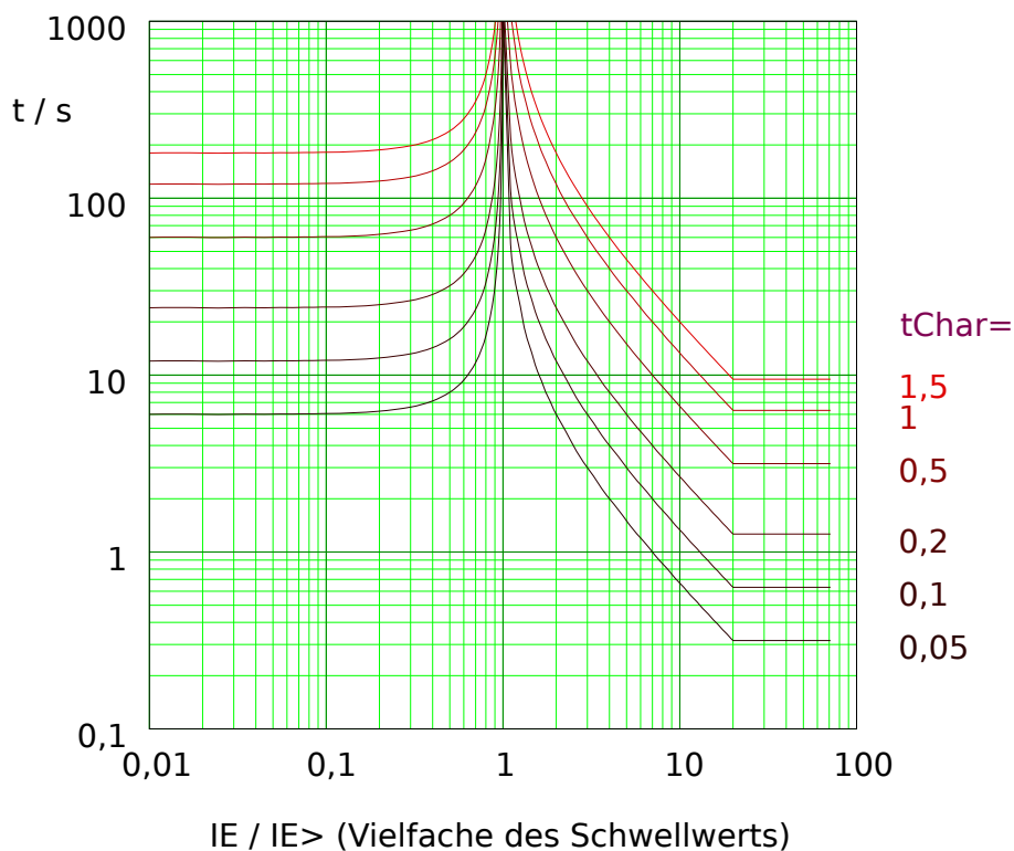
Abb. 88: LINV: Rückfallverzögerung (linke Hälfte, IE < I_{E>} ) und Auslöseverzögerung (rechte Hälfte, IE > I_{E>} ), Beispieldiagramm für I_{max} = 20 \cdot I_{E>} .
