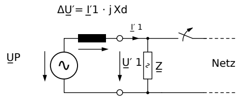
Abb. 106: Ersatzschaltbild Synchrongenerator bei Netzausfall.
