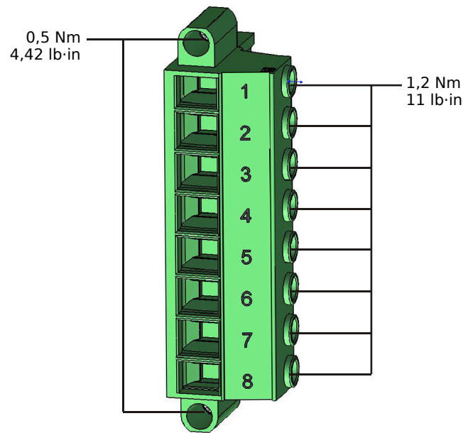
Fig. 118: Terminais de medição de tensão da placa de medição "TU" (↪ "2.6.1 TU - Entradas de Medição de Tensão").
