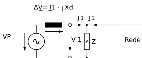
Fig. 86: Circuito equivalente no gerador síncrono em paralelo com a rede.
