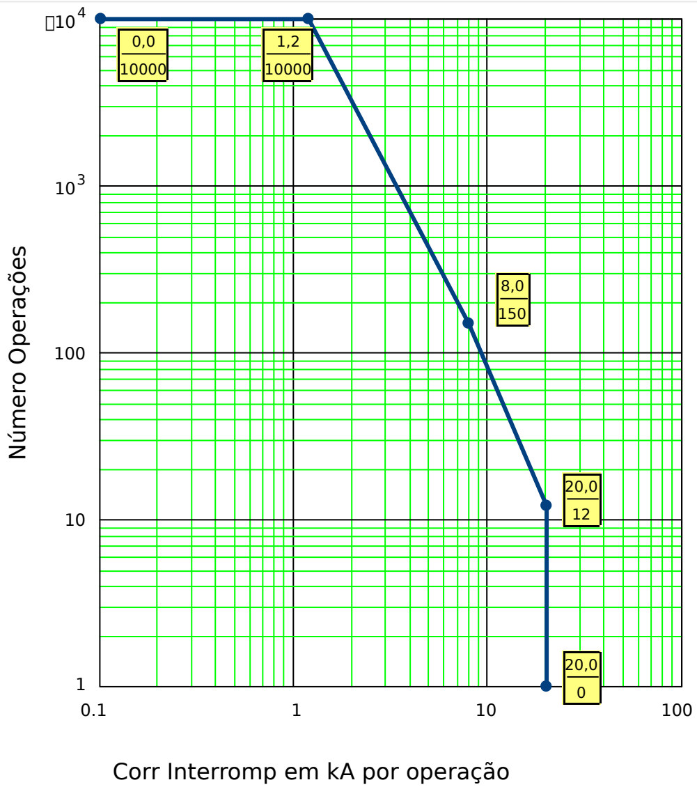
Fig. 104: Curva Manutenção de Disjuntor para Disjuntor normal 25kV
