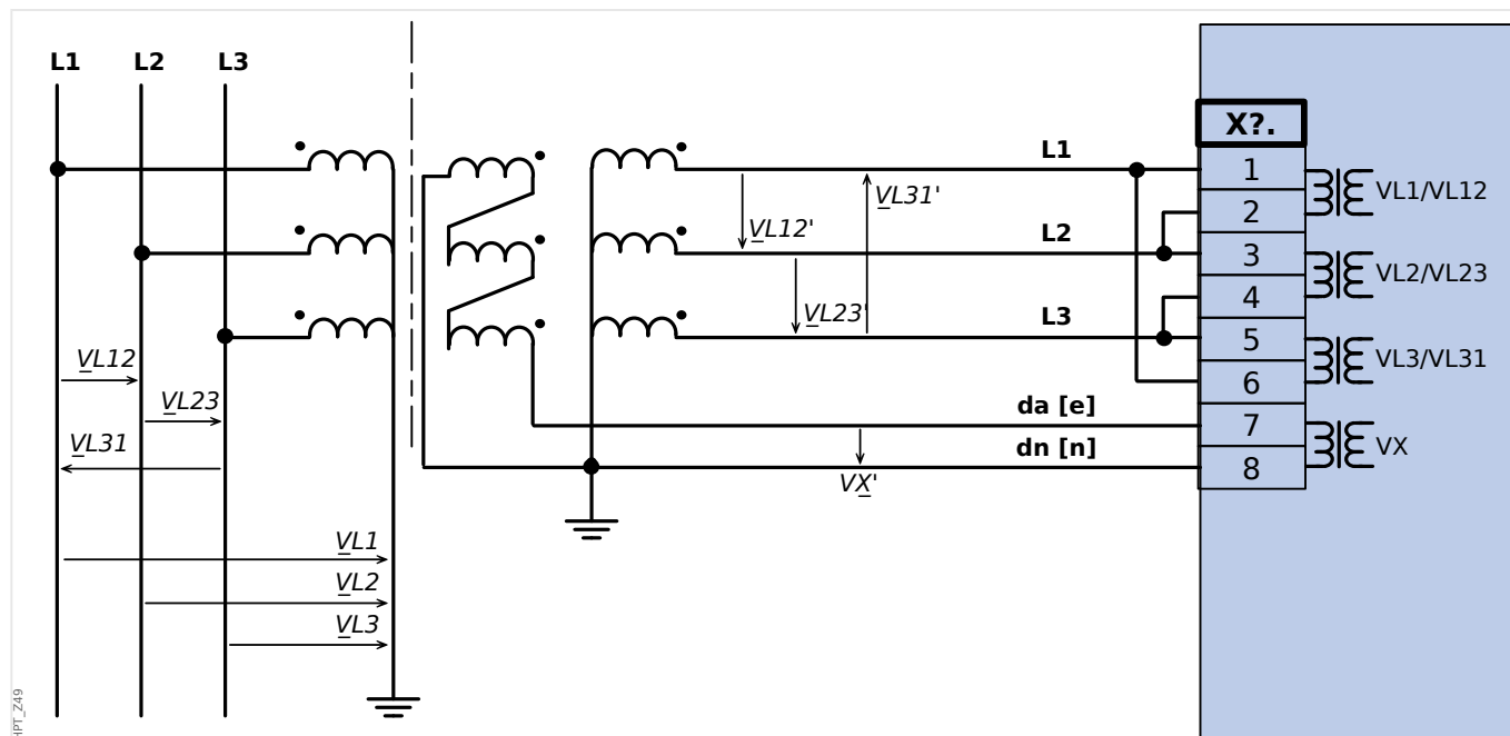
Fig. 31: Medição VG tensão residual por meio de "delta aberto" (e-n) de circuito auxiliar
