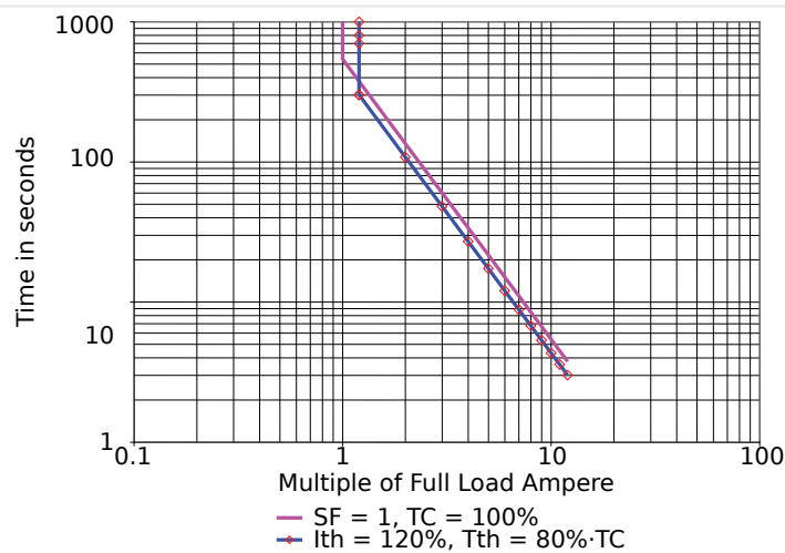
Fig. 65: Limite do modelo de réplica térmica e curvas de disparo sem DTR.
