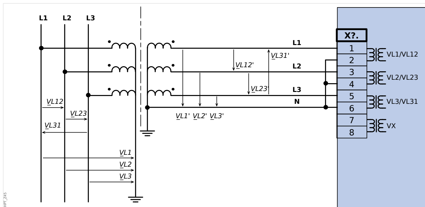
Fig. 28: VT Wye: Medição de voltagem trifásica - fiação das entradas de medição: "conexão estrela"
