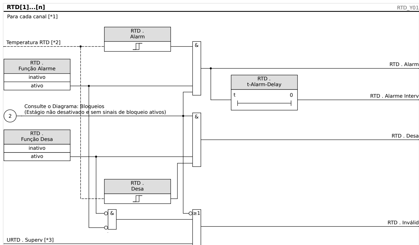
Fig. 94: O princípio geral de funcionamento (alarme atrasado, disparo sem atraso).
