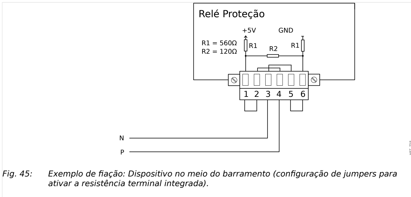
Fig. 44: Exemplo de fiação: Dispositivo no meio do barramento
