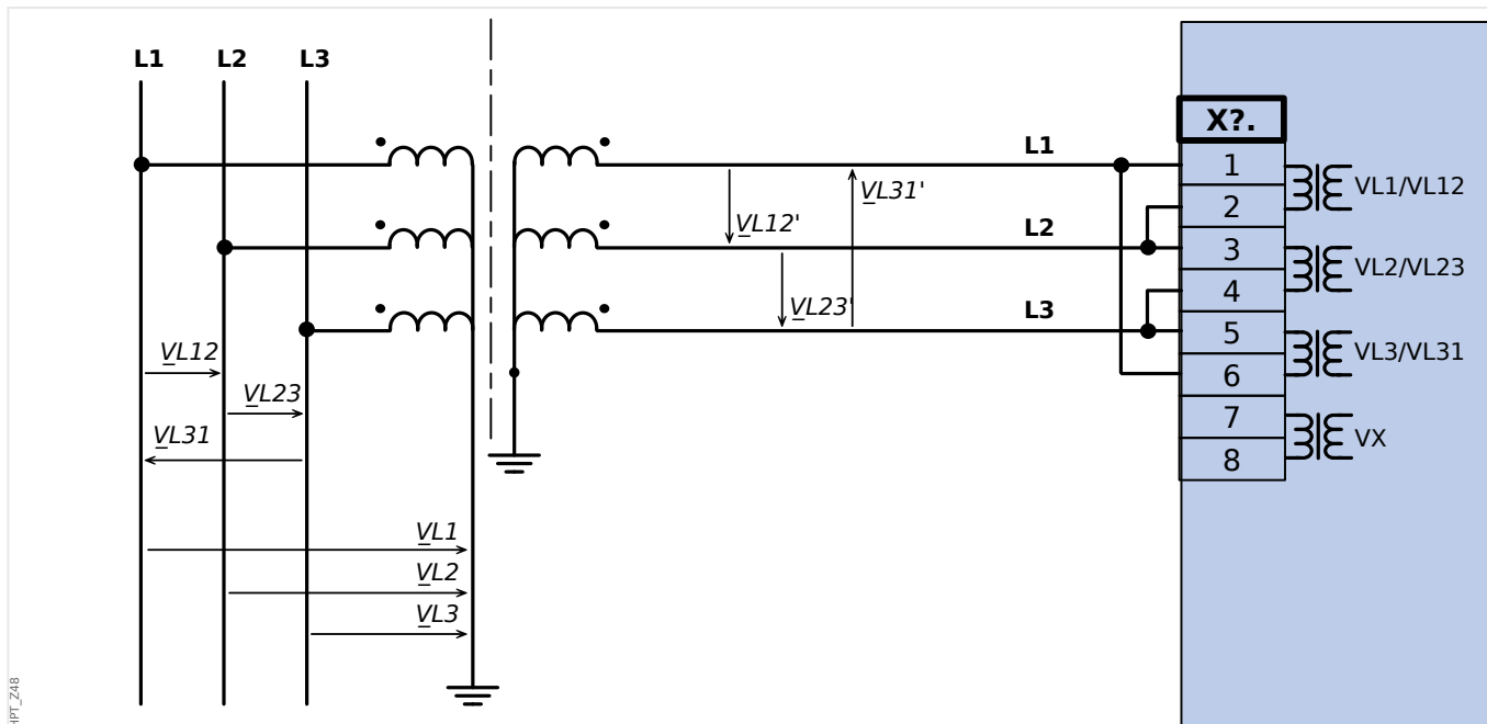
Fig. 30: Medição de tensão trifásica - fiação das entradas de medição: "conexão-delta"
