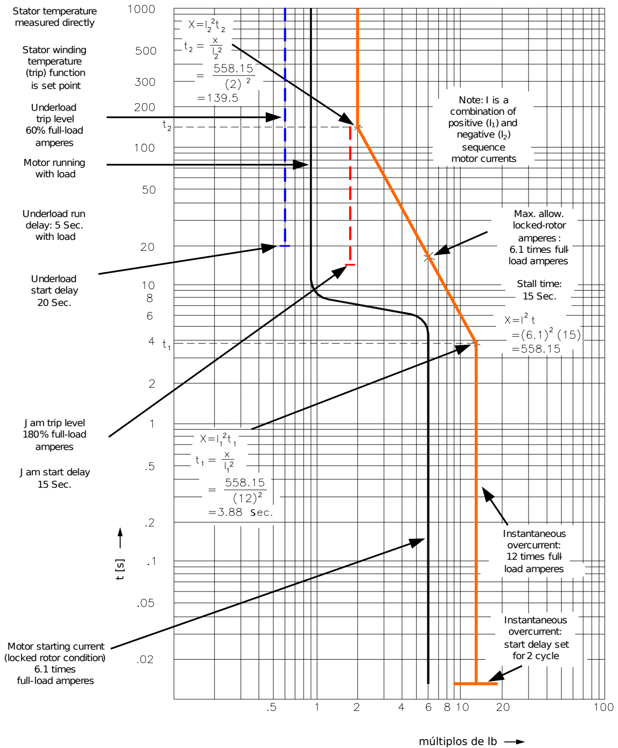
Fig. 69: Curva de Proteção do Motor (Exemplo 3 - com RTDs)
