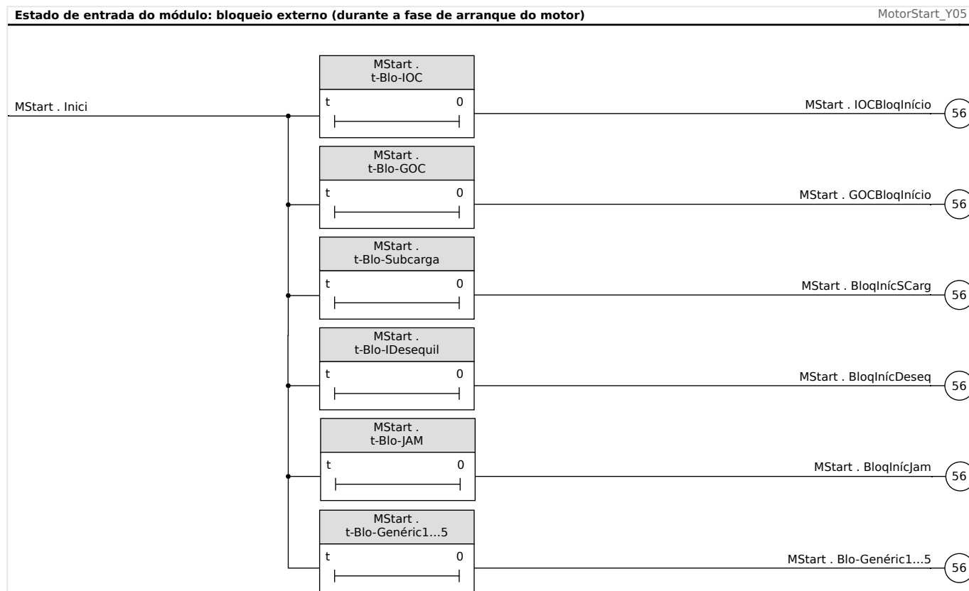
Fig. 60: Bloqueio temporário das funções de proteção de corrente durante a partida do motor.
