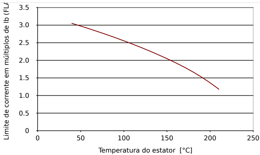
Fig. 64: Limite de corrente real vs. Temperatura máxima do estator.
