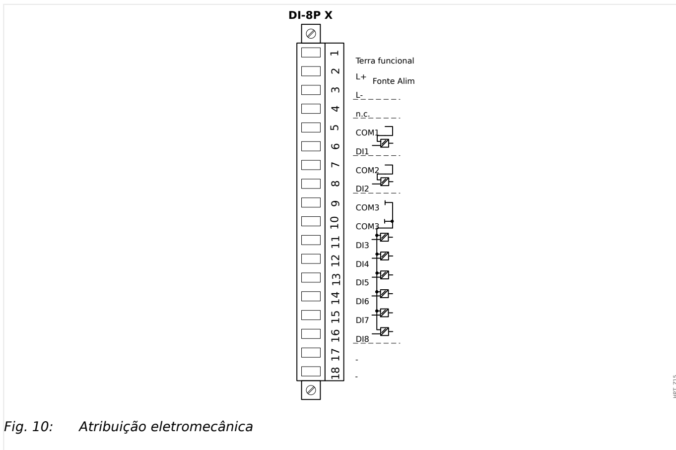
Fig. 9: Terminais
