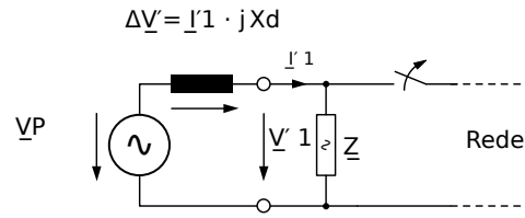
Fig. 88: Circuito equivalente em falha da rede
