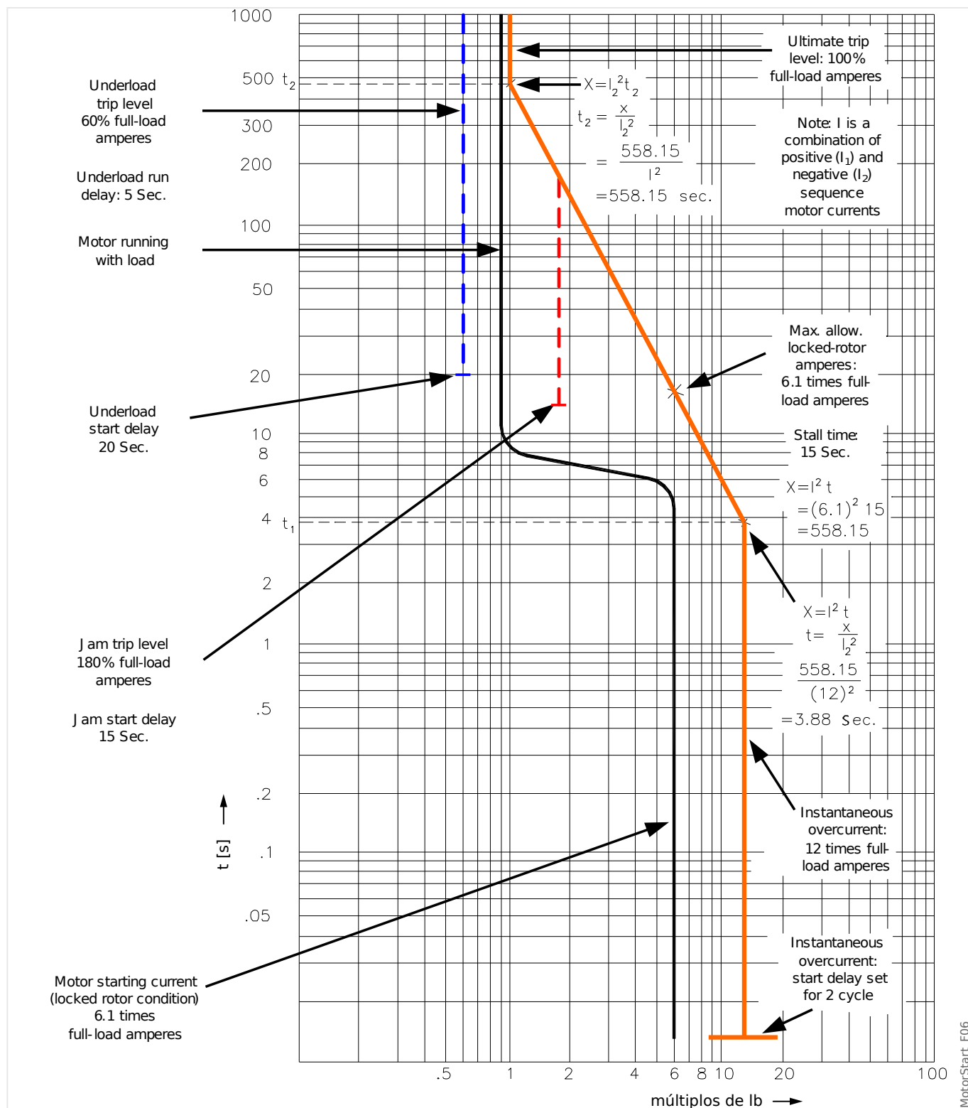
Fig. 68: Curva de Proteção do Motor (Exemplo 2 - sem RTDs)
