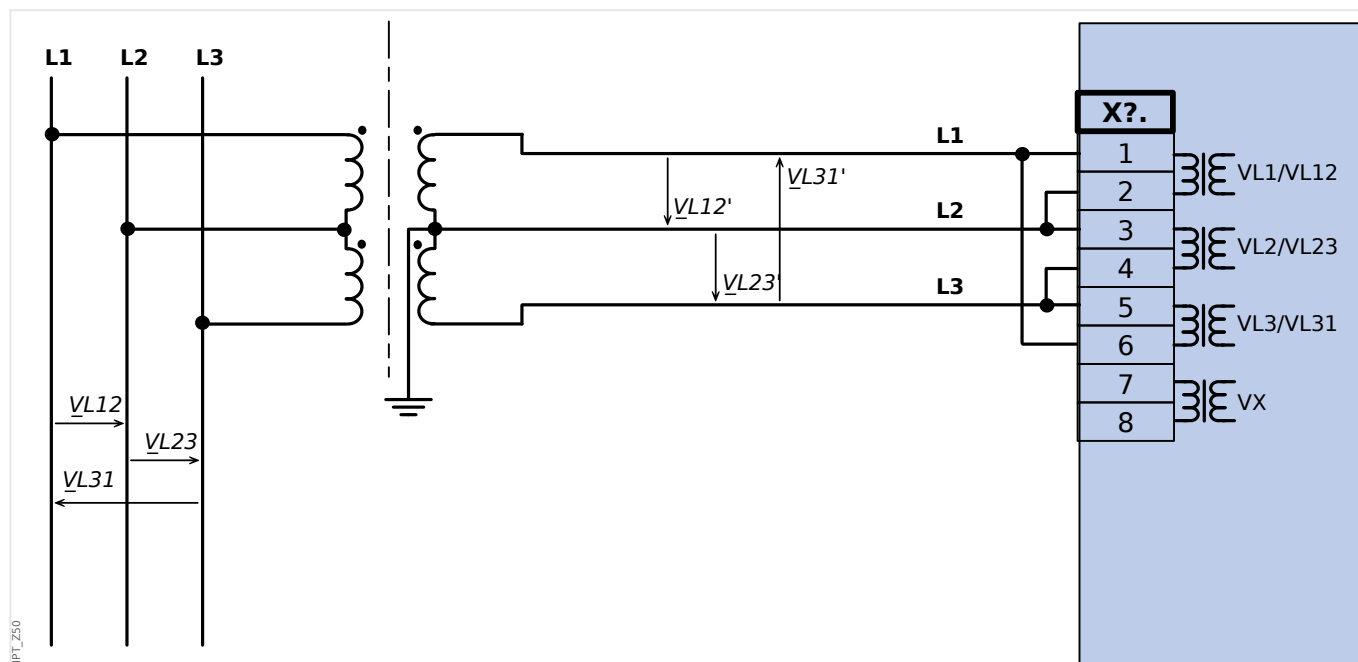
Fig. 32: Medição de tensão bifásica - fiação das entradas de medição: "Delta Aber"
