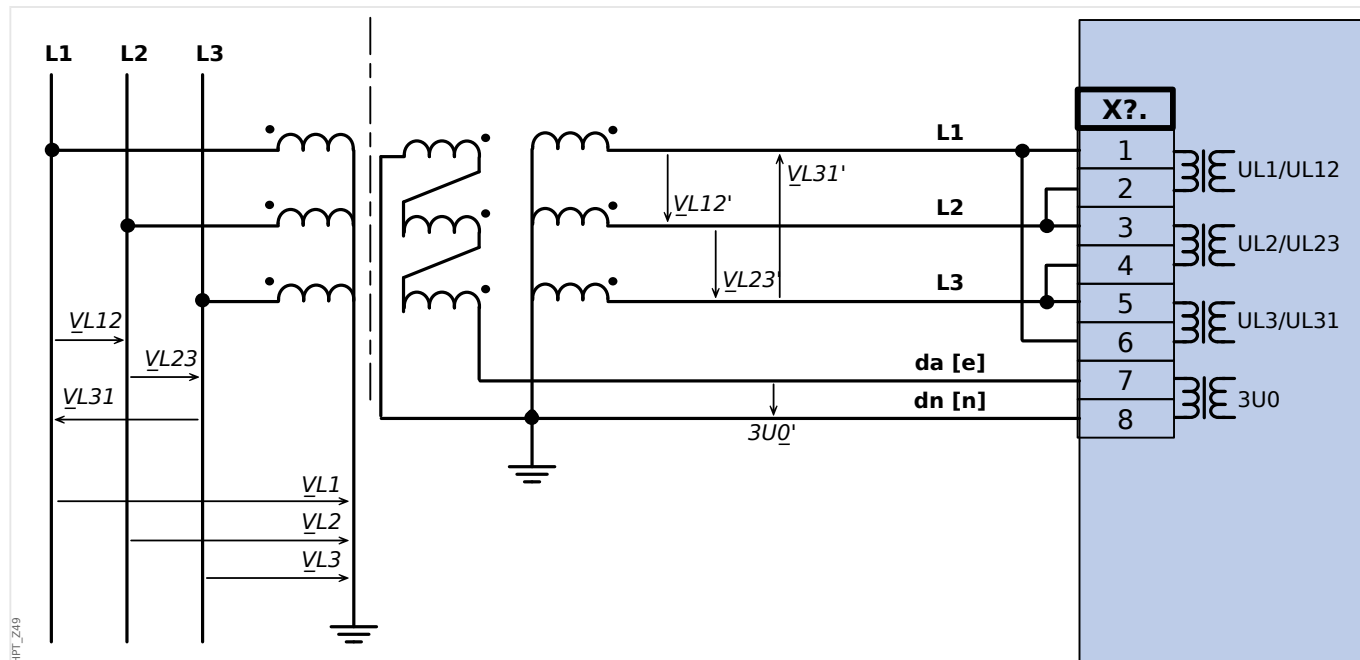
Rys. 31: Trójfazowy pomiar napięcia w układzie trójkąta: połączenie przewodów wejść pomiarowych: "połączenie w trójkąt" Pomiar 3U0 napięcia szczytkowego poprzez dodatkowe uzwojenia (e-n) w układzie otwartego trójkąta
