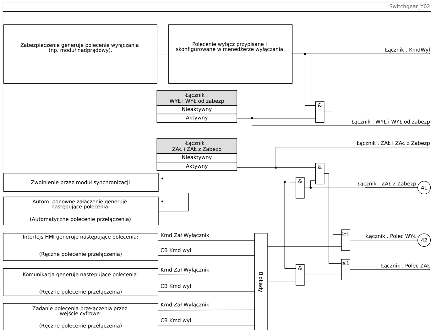
Rys. 102: Blokady. (Podzespoły oznaczone symbolem „*”: dostępność zależy od typu zamówionego urządzenia).
