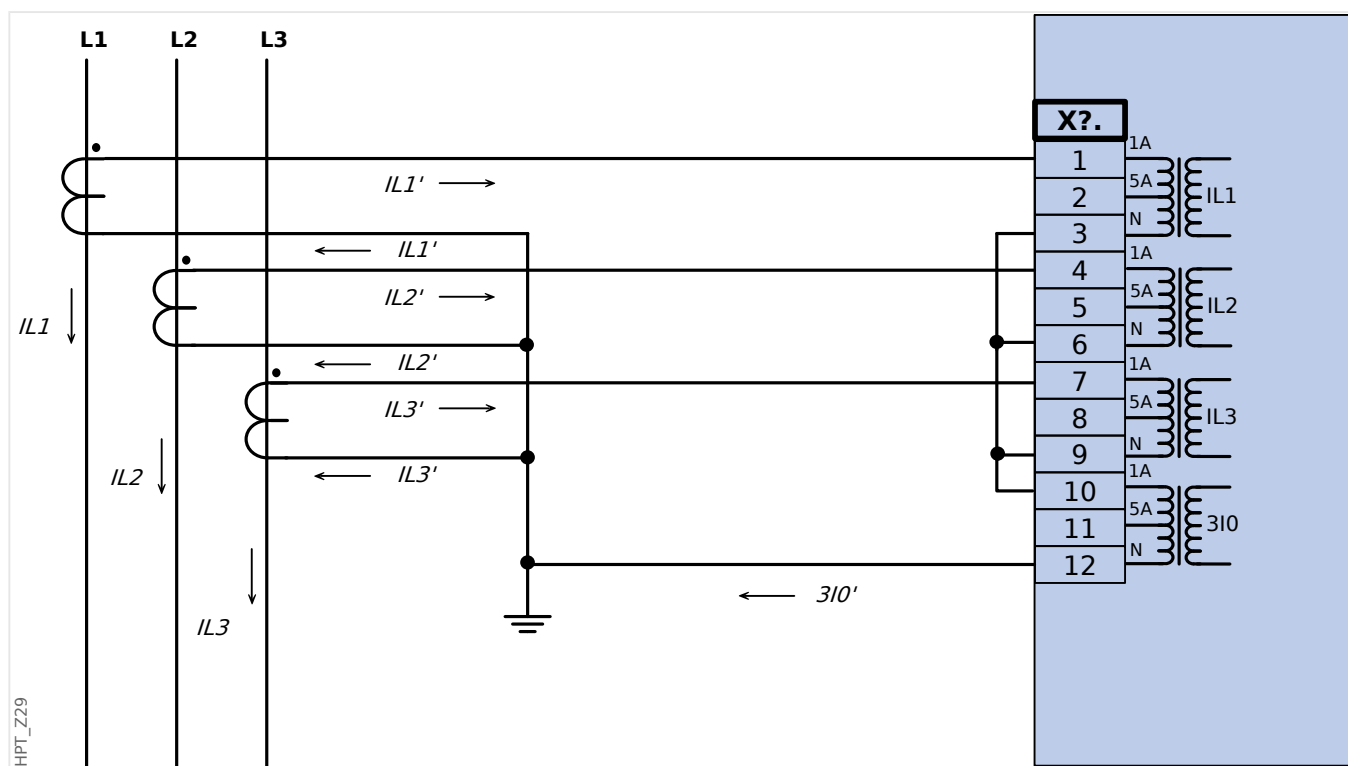
Rys. 22: Trójfazowy pomiar prądu; I_n wtórny = 1 A. Pomiar prądu doziemnego w układzie Holmgrena 310n wtórny = 1 A.
