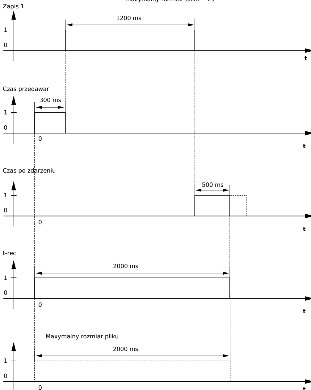
Rys. 107: Przykładowy wykres czasów pracy rejestratora zakłóceń I
