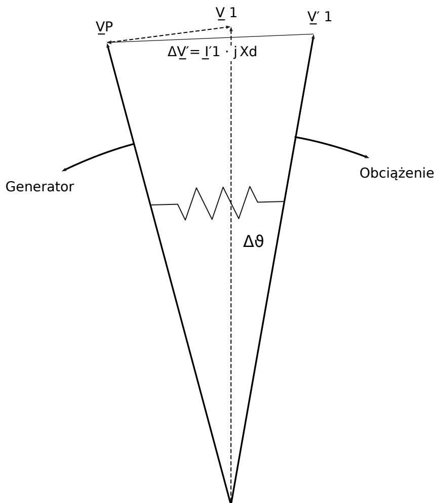
Rys. 89: Wektory napięcia przy awarii sieci.
