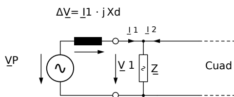
Fig. 86: Circuito equivalente en generador sincrónico en paralelo con la red de suministro eléctrico.
