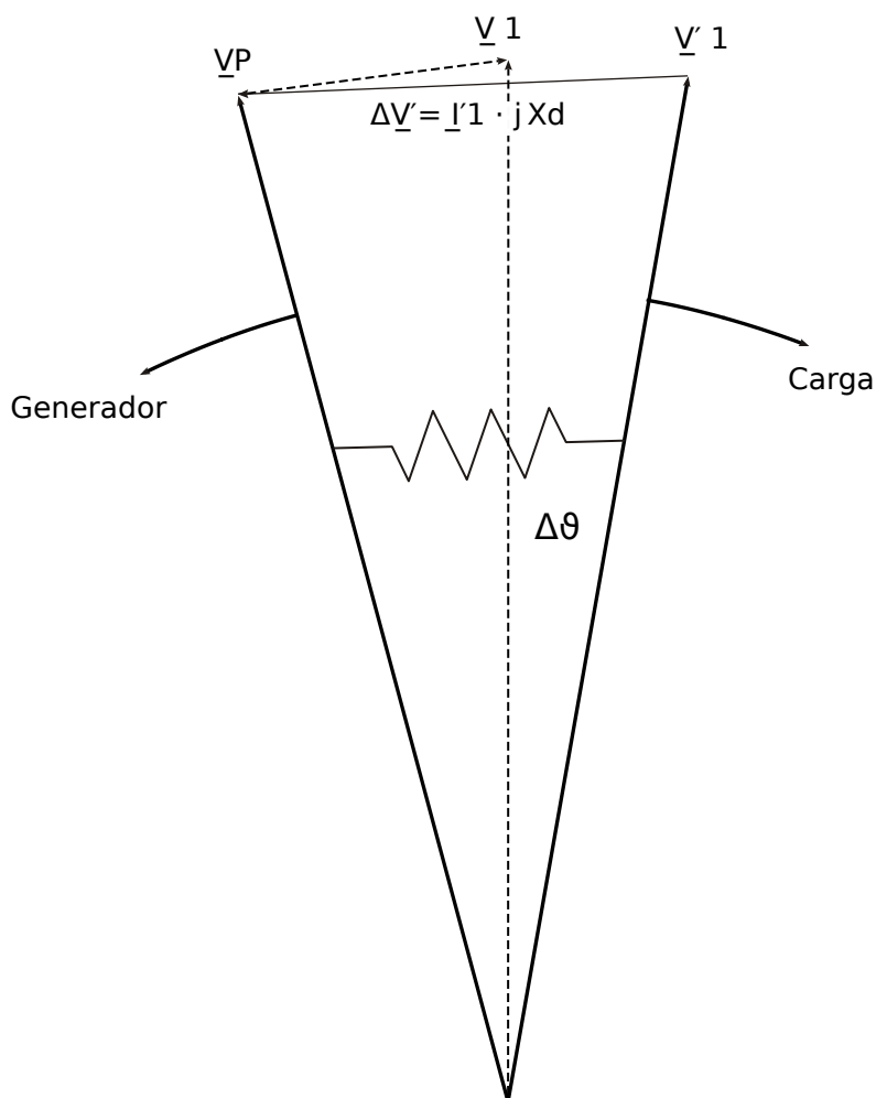
Fig. 89: Fallo de los vectores de tensión en la red.
