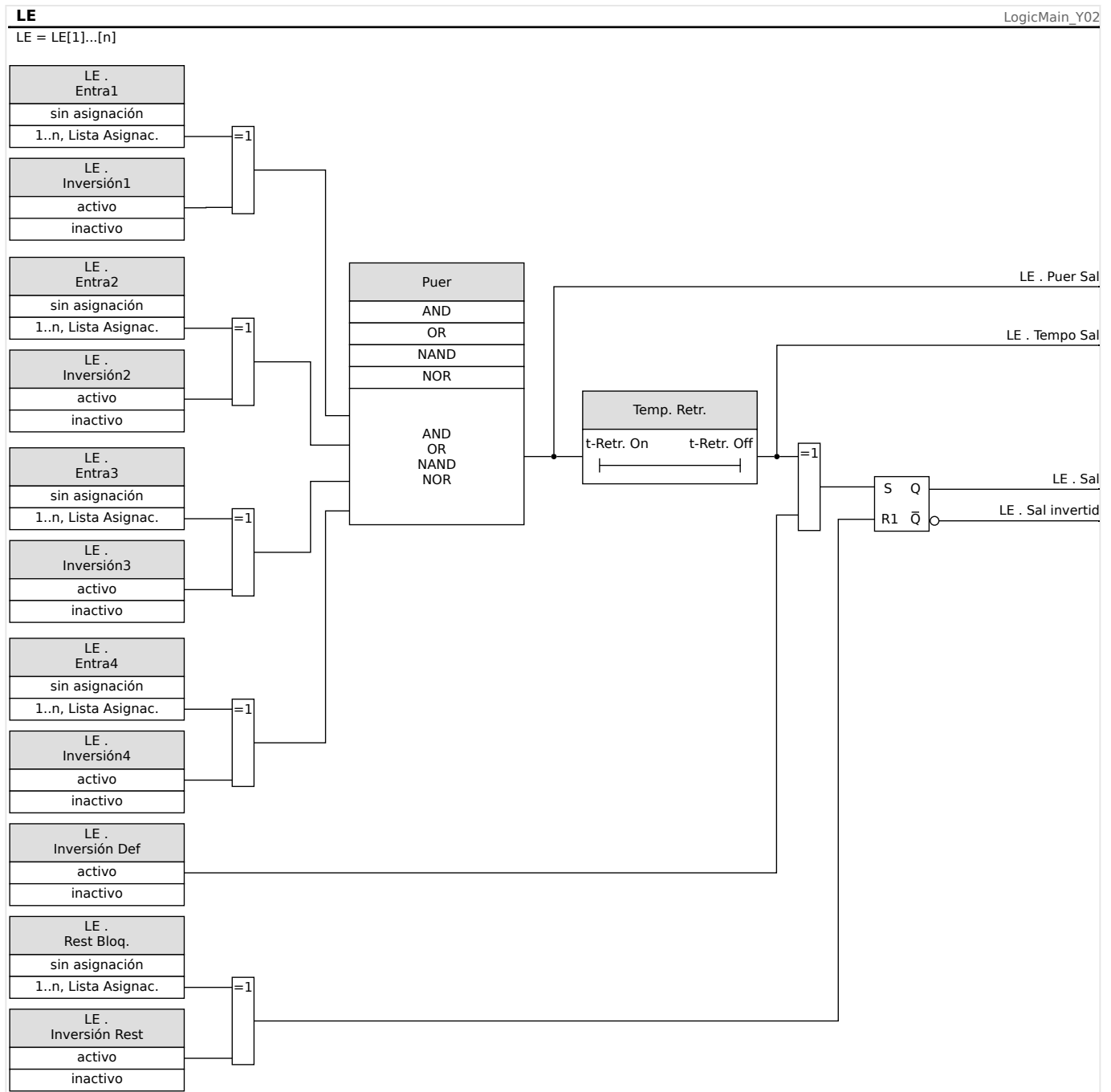
Fig. 111: Descripción detallada - Diagrama de lógica general.
