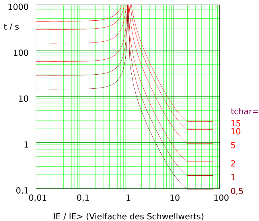
Abb. 90: EINV: Rückfallverzögerung (linke Hälfte, IE < IE> ) und Auslöseverzögerung (rechte Hälfte, IE > IE> ), Beispieldiagramm für I_{E,max} = 20 \cdot IE> .
