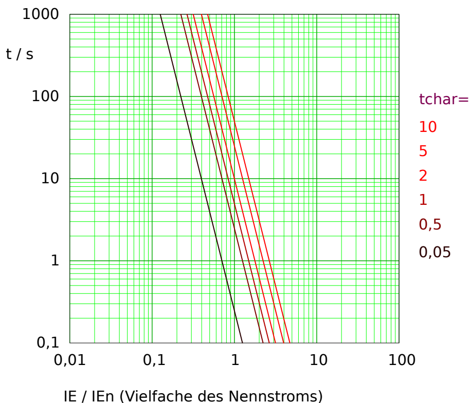
Abb. 96: Auslösekurve „I4T“, wobei nur der Bereich IE > IE_{n> jeweils anwendbar ist. Beispieldiagramm für gemessenen (nicht empfindlichen) Erdstrom.
