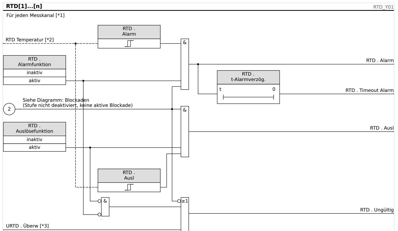
Abb. 111: Generelles RTD-Funktionsprinzip.
