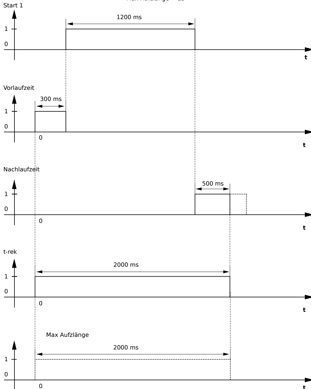
Abb. 124: Beispiel I Störschreiber-Ablaufdiagramm
