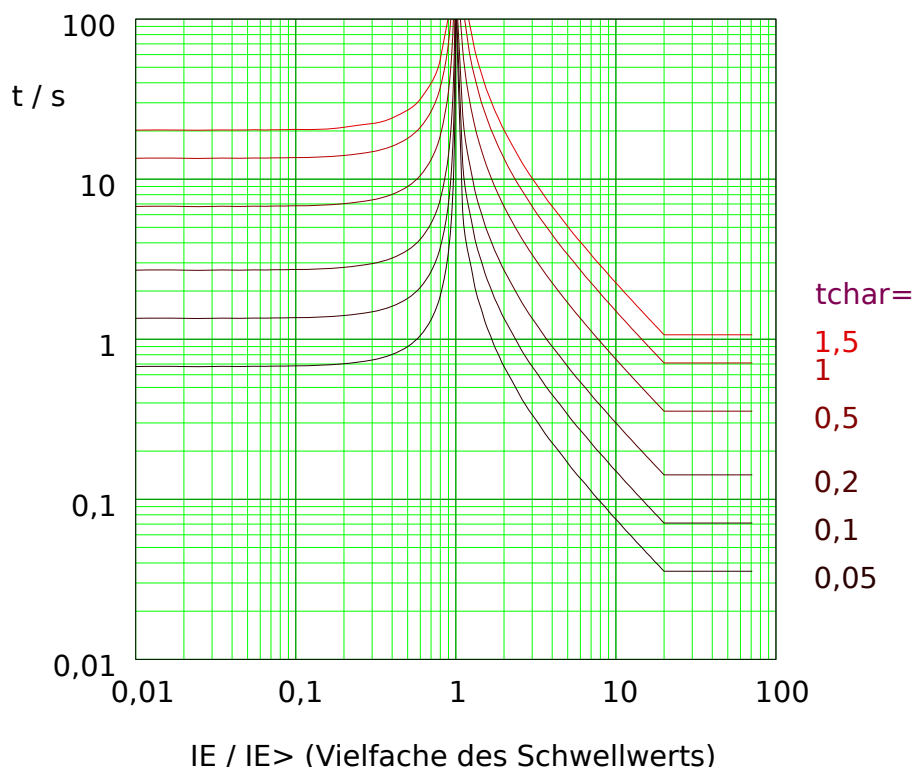
Abb. 85: VINV: Rückfallverzögerung (linke Hälfte, IE < IE_{max} ) und Auslöseverzögerung (rechte Hälfte, IE > IE_{max} ), Beispieldiagramm für IE_{max} = 20 \cdot IE_{nom} .
