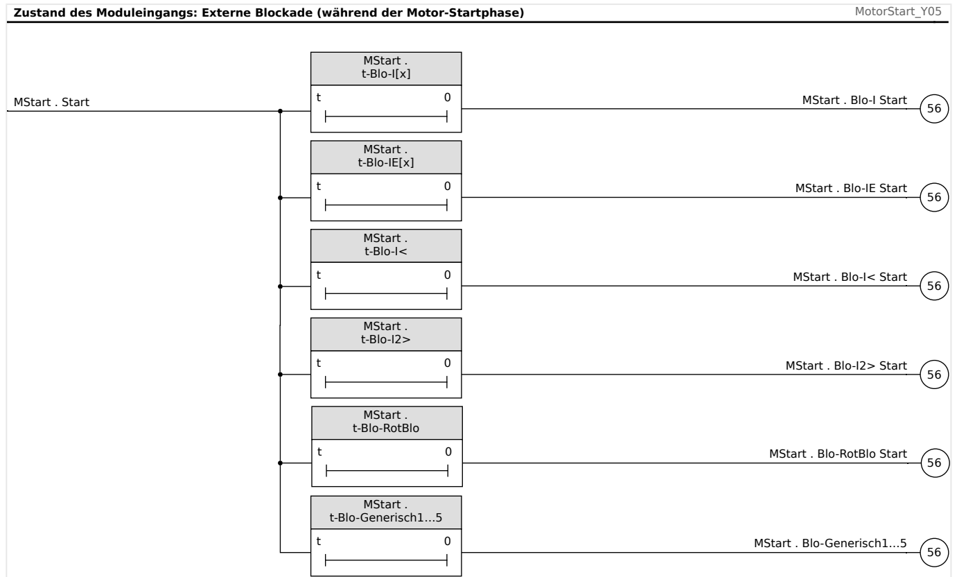
Abb. 60: Temporäre Blockade von Stromschutzfunktionen während Motorstarts.
