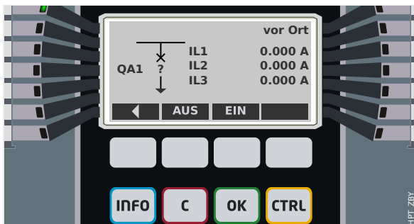
Abb. 117: Beispiel einer Steuer-Seite mit „Leistungsschalter“ in Störstellung (bzw. unplausiblem Zustand).
