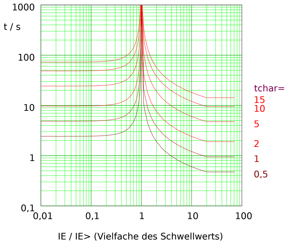
Abb. 88: MINV: Rückfallverzögerung (linke Hälfte, IE < IE> ) und Auslöseverzögerung (rechte Hälfte, IE > IE> ), Beispieldiagramm für I_{E,max} = 20 \cdot IE> .
