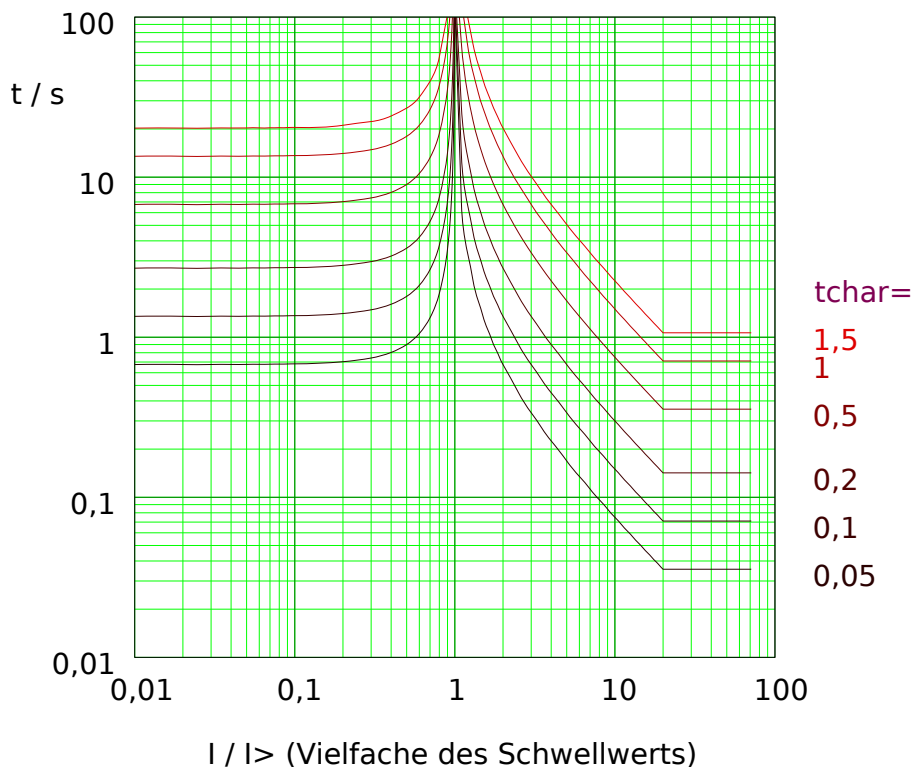
Abb. 73: VINV: Rückfallverzögerung (linke Hälfte, I < I> ) und Auslöseverzögerung (rechte Hälfte, I > I> ), Beispieldiagramm für I_{max} = 20 \cdot I> .
