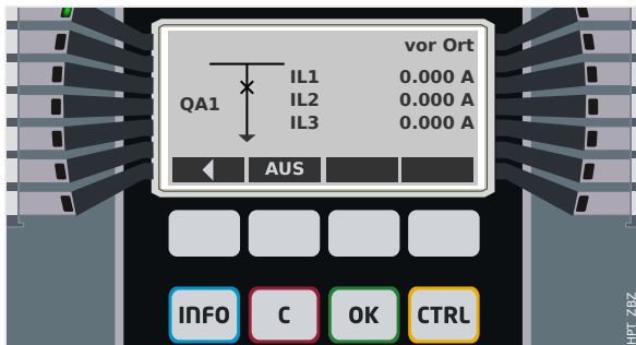
Abb. 116: Beispiel einer Steuer-Seite mit geschlossenem „Leistungsschalter“.
