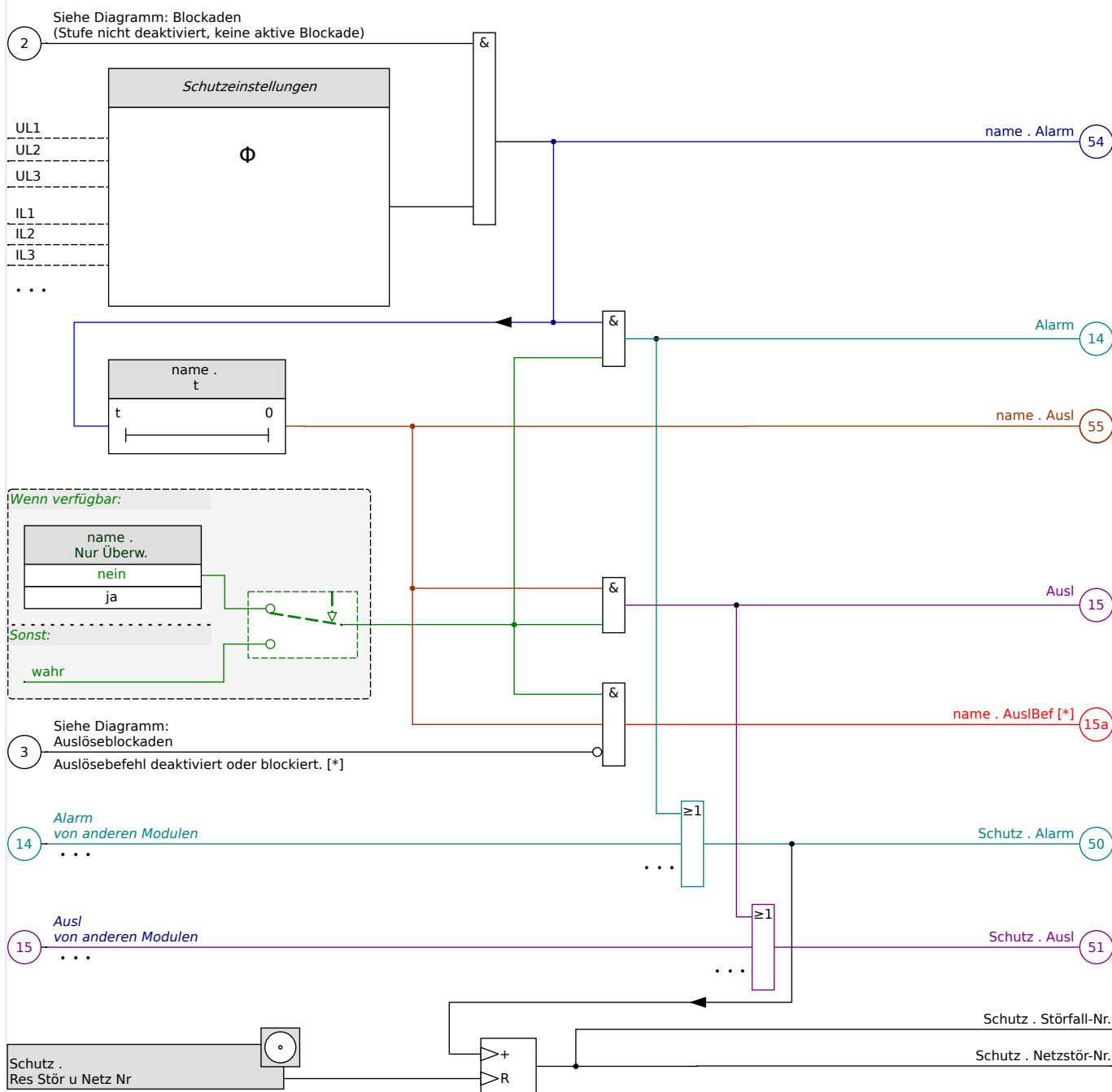
Abb. 58: Grobe Skizze der Funktionalität einer HighPROTEC-Schutzfunktion.
