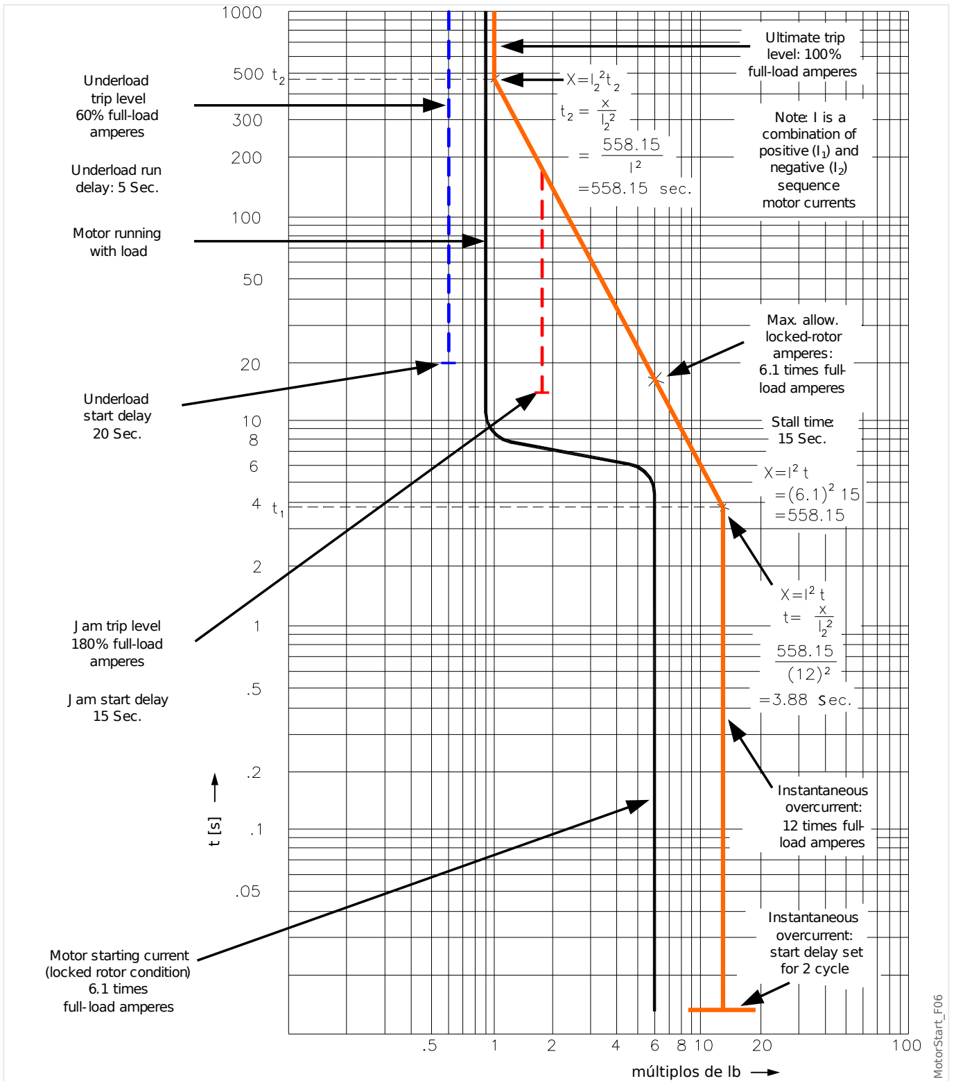
Fig. 56: Curva de Proteção do Motor (Exemplo 2 - sem RTDs)
