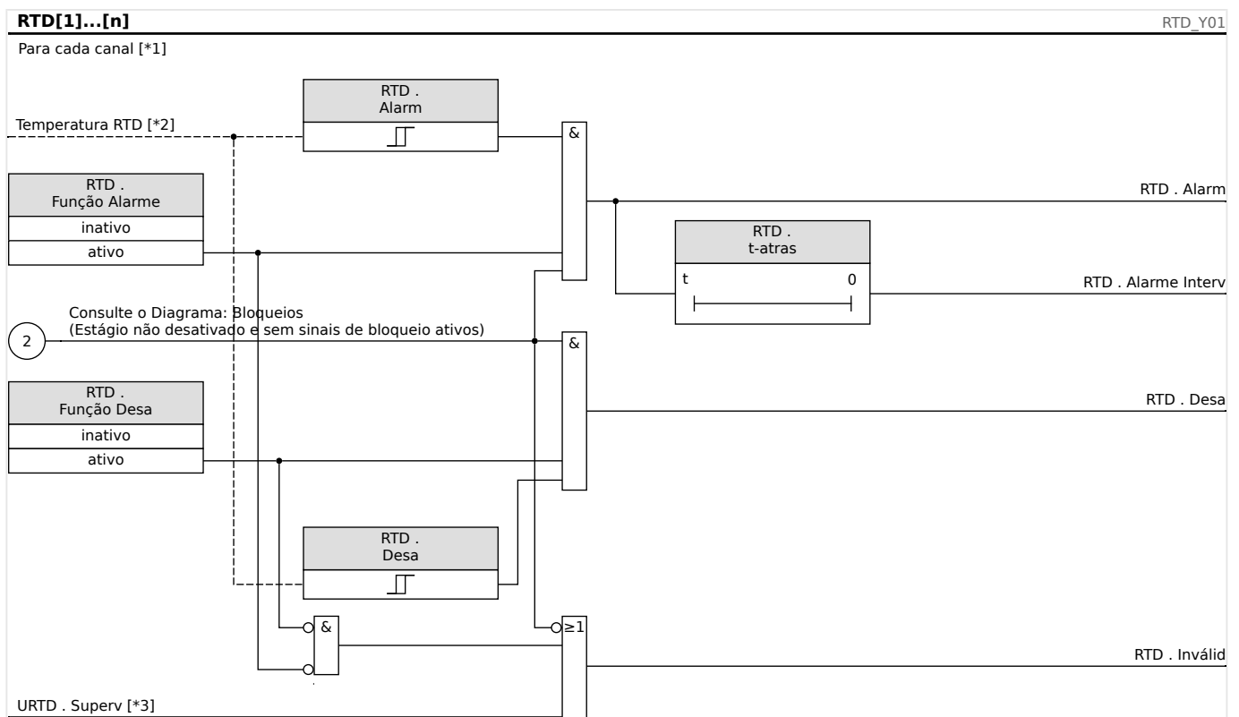
Fig. 63: O princípio geral de funcionamento (alarme atrasado, disparo sem atraso).
