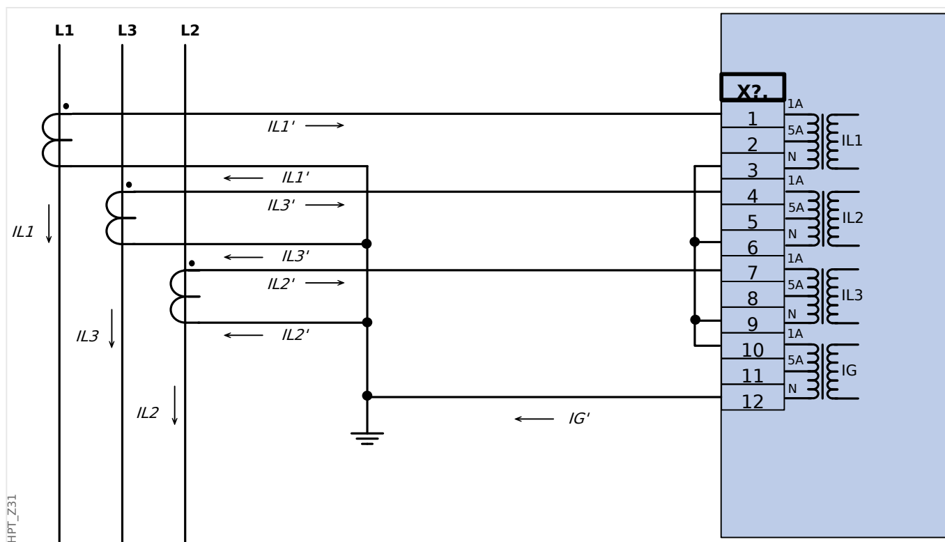
Fig. 28: Medição de corrente de trifásica; I_n secundário = 1 A. Medição corrente terra via conexão Holmgreen; I_{Gnom} secundário = 1 A.
