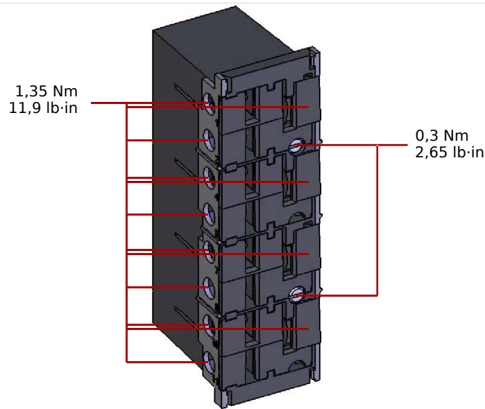
Fig. 87: Conector plug-in com acionador de curto-circuito integrado (entradas de corrente convencionais)
