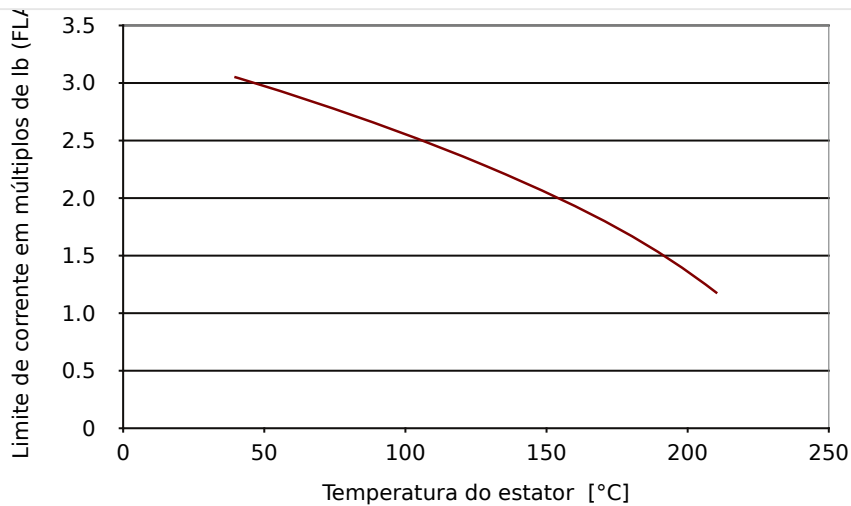
Fig. 52: Limite de corrente real vs. Temperatura máxima do estator.
