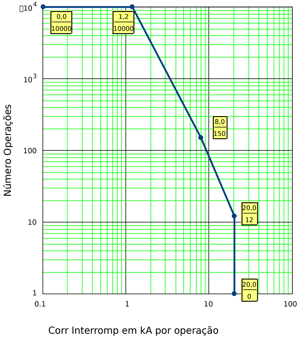
Fig. 72: Curva Manutenção de Disjuntor para Disjuntor normal 25kV
