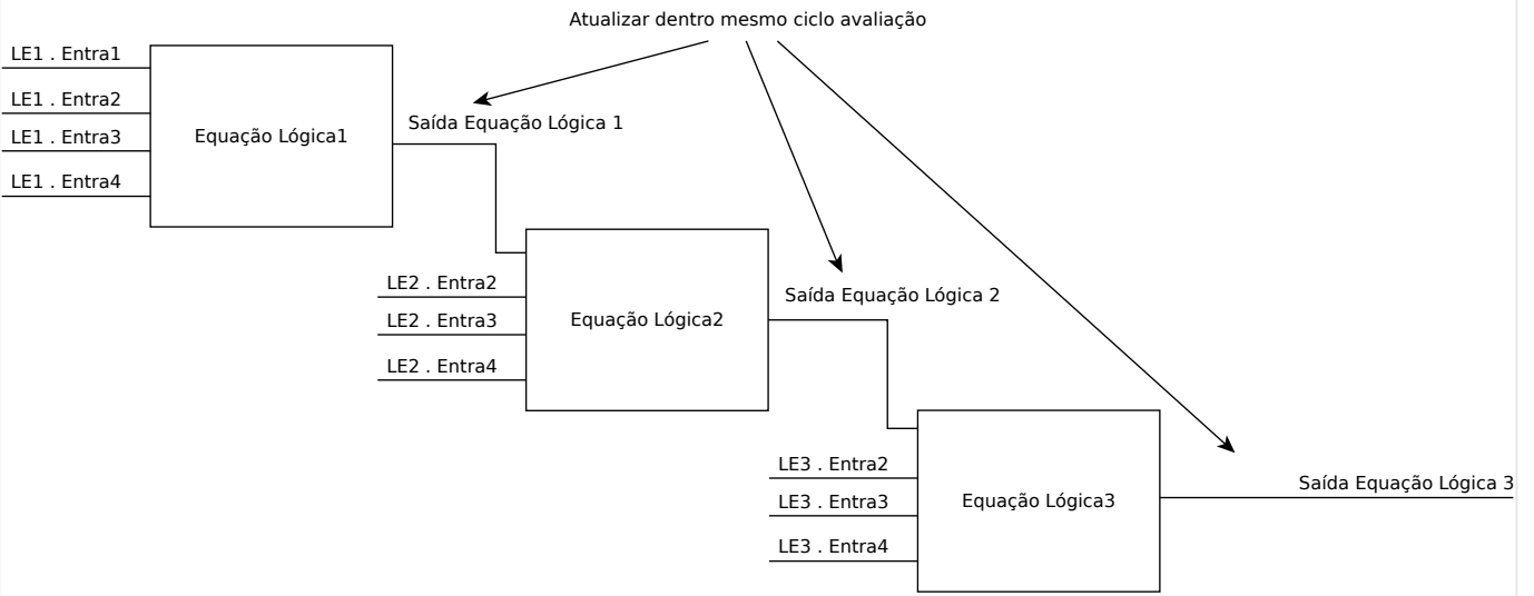
Fig. 82: Em cascata crescente
