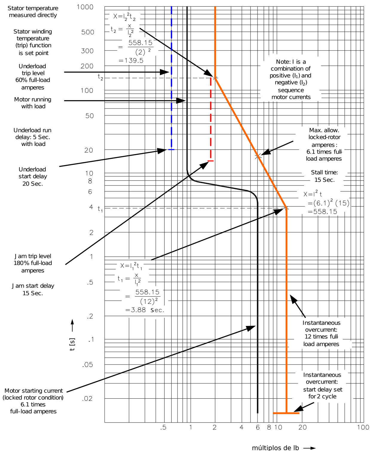
Fig. 57: Curva de Proteção do Motor (Exemplo 3 - com RTDs)
