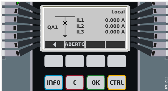
Fig. 67: Exemplo de página de controle, com o "Disjuntor" na posição fechada.
