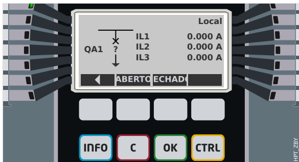
Fig. 68: Exemplo de página de controle, com o "Disjuntor" na posição de falha (ou implausível).
