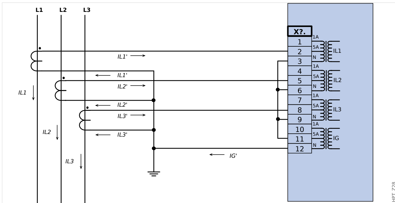
Fig. 25: Medição de corrente de trifásica; I_n secundário = 5 A. Medição corrente terra via conexão Holmgreen; I_{Gnom} secundário = 5 A.
