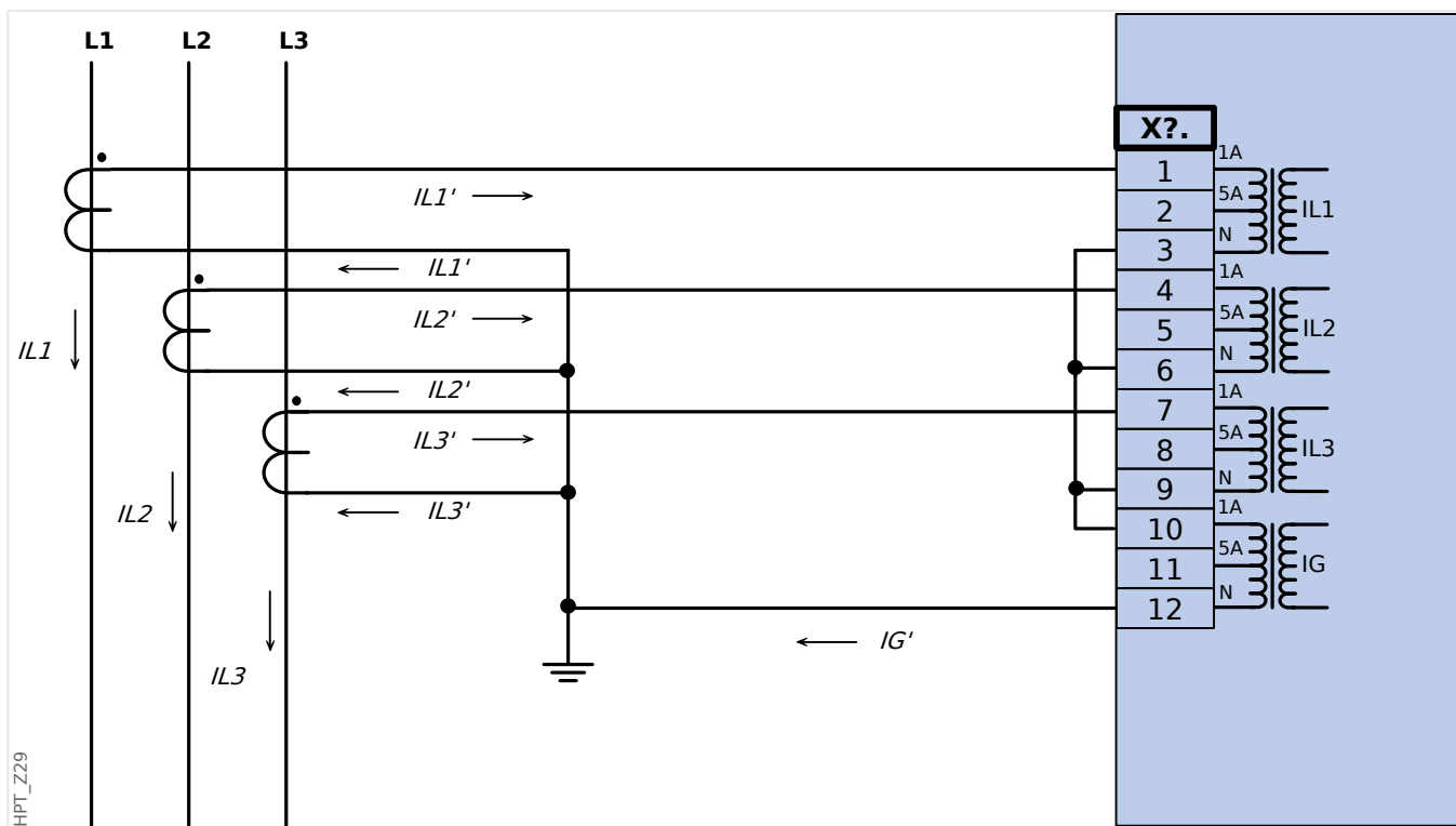
Fig. 26: Medição de corrente de trifásica; I_n secundário = 1 A. Medição corrente terra via conexão Holmgreen; I_{Gnom} secundário = 1 A.
