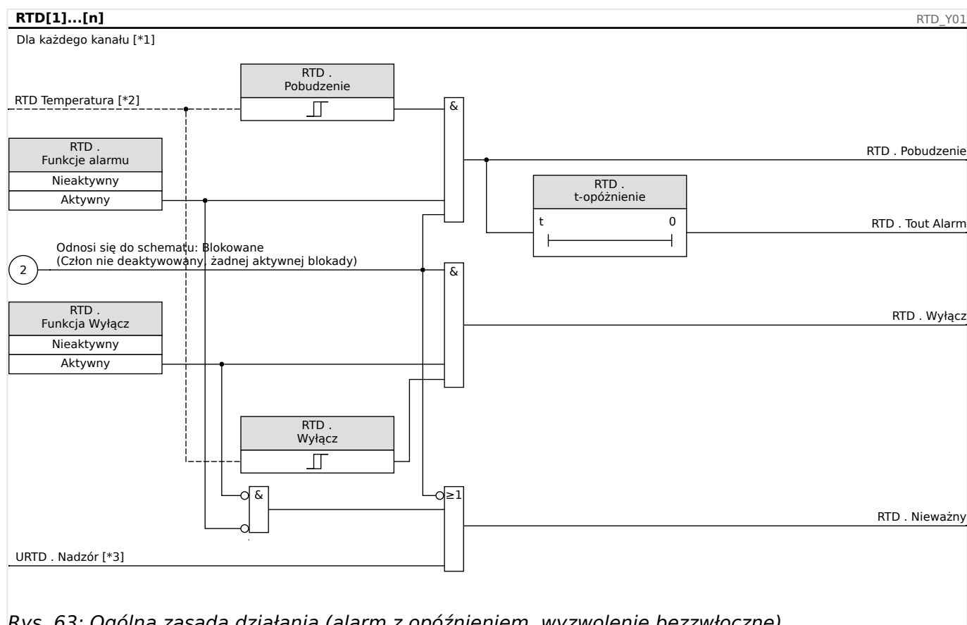
Rys. 63: Ogólna zasada działania (alarm z opóźnieniem, wyzwolenie bezzwłoczne).
