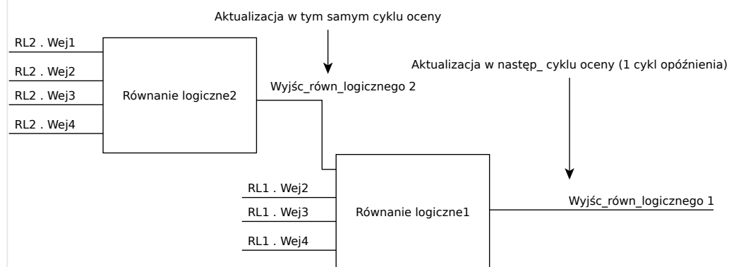
Rys. 83: Ukł. kaskadowy w porządku malejącym
