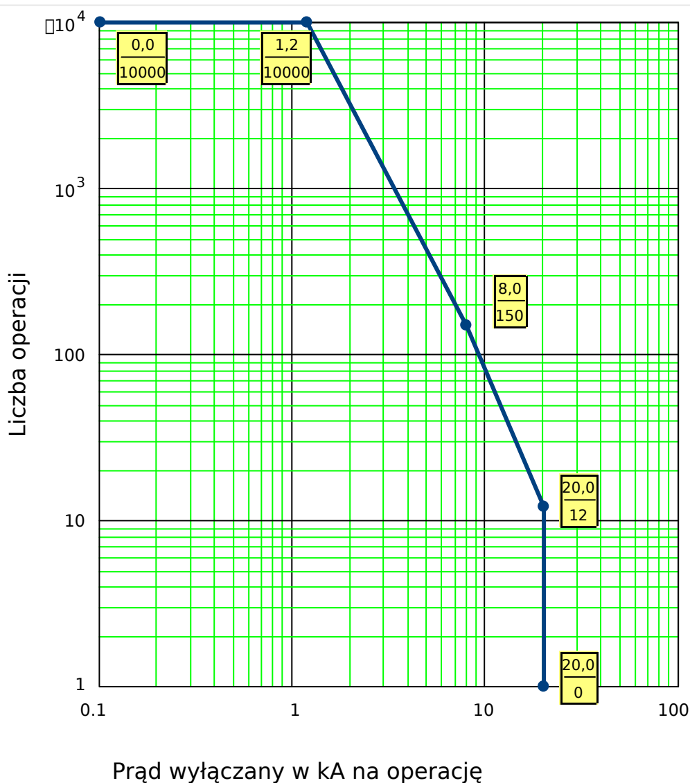
Rys. 72: Krzywa konserwacji wyłącznika typowego wyłącznika 25 kV
