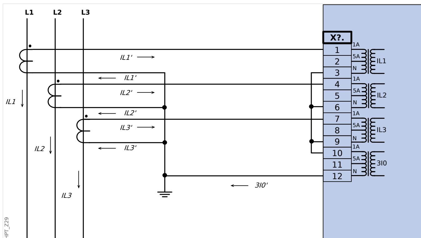
Rys. 26: Trójfazowy pomiar prądu; I_n wtórny = 1 A. Pomiar prądu doziemnego w układzie Holmgreena 3I_0 wtórny = 1 A.
