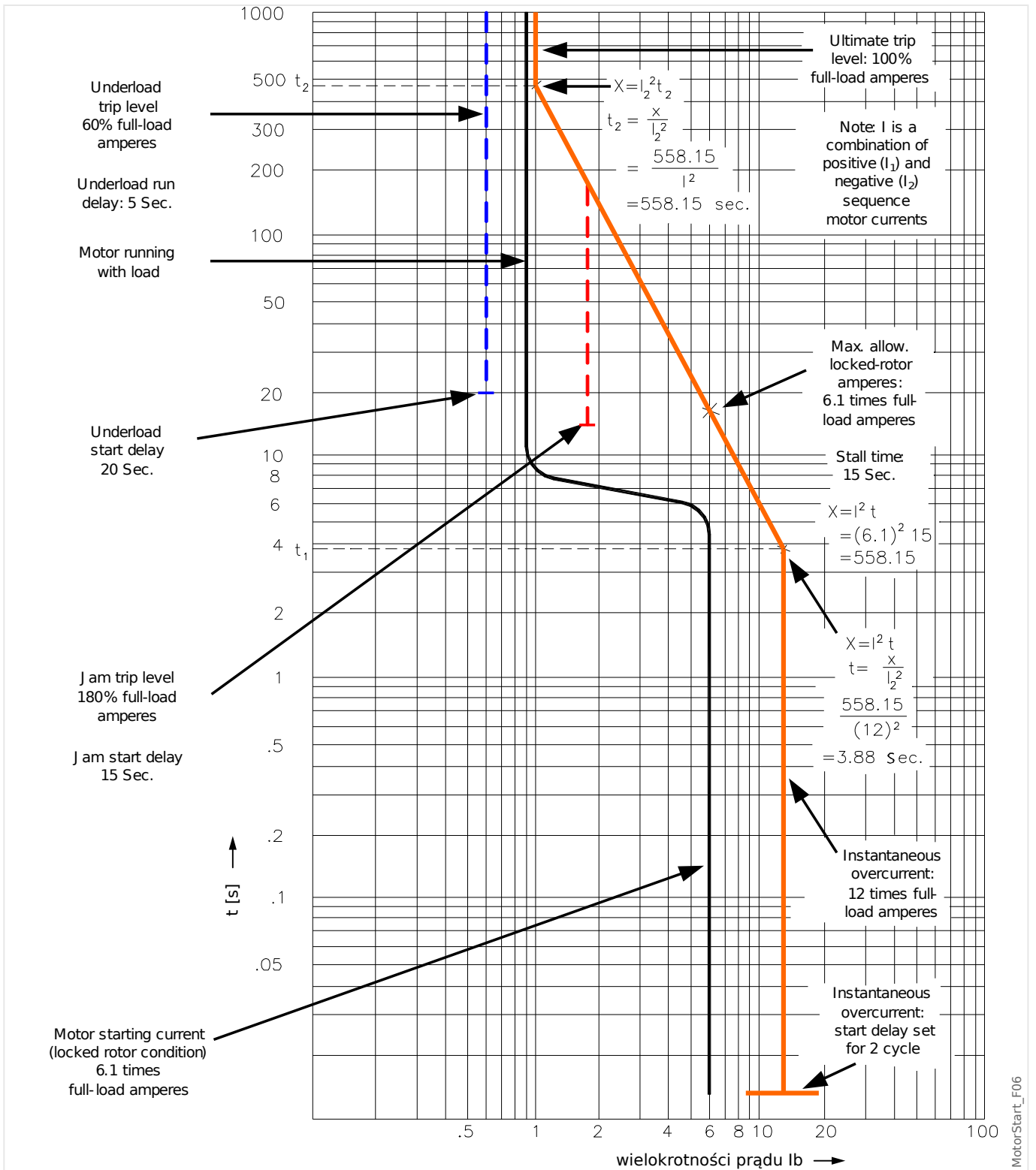
Rys. 56: Krzywa zabezpieczenia silnika (przykład 2 — bez RCT).
