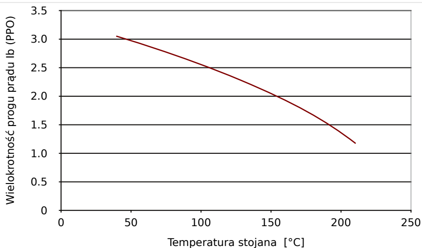
Rys. 52: Próg prądu skutecznego w stosunku do maksymalnej temperatury stojana.
