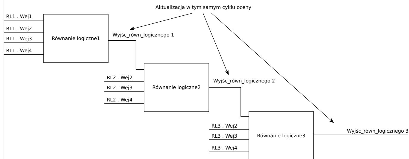
Rys. 82: Ukł. kaskadowy w porządku rosnącym
