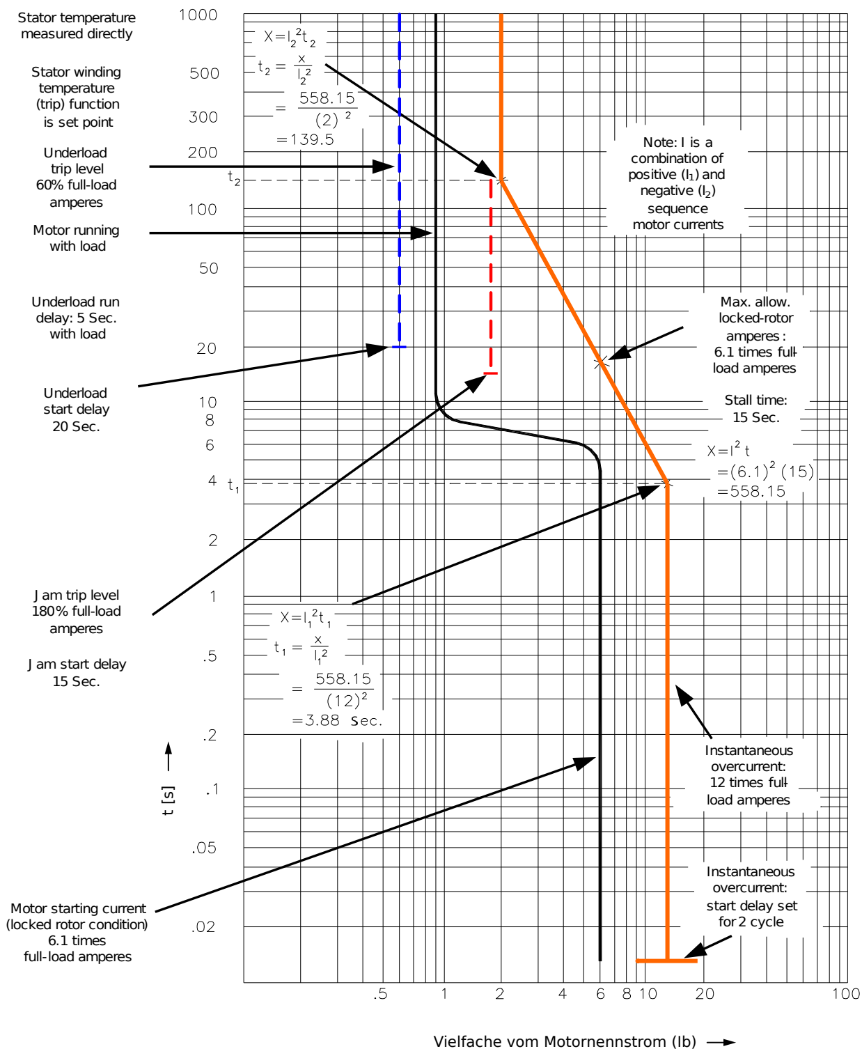
Abb. 58: Auslösekennlinien (Beispiel 3 - mit RTDs).
