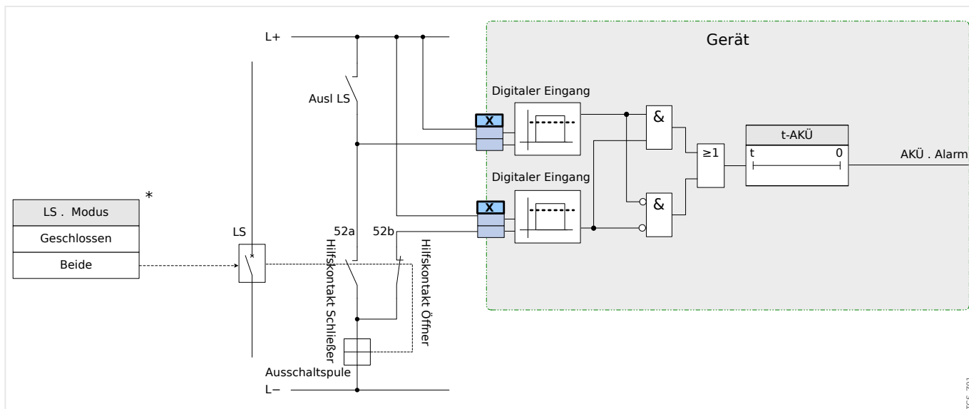
Abb. 65: Anschlussbeispiel (Empfehlung): Auslösekreisüberwachung mit zwei Hilfskontakten »Hiko EIN« (52a) und »Hiko AUS« (52b).
