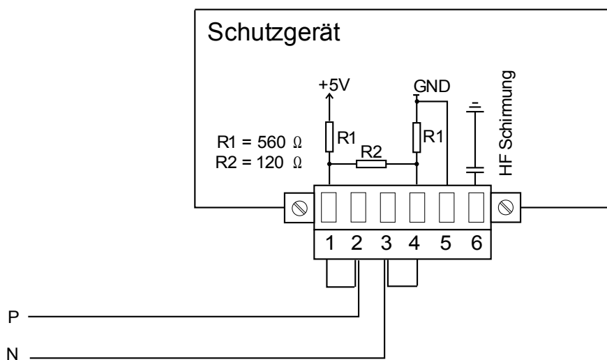
Typ 2 Verdrahtungsbeispiel, Gerät am Ende des Busses (Benutzen des integrierten Abschlusswiderstands)
