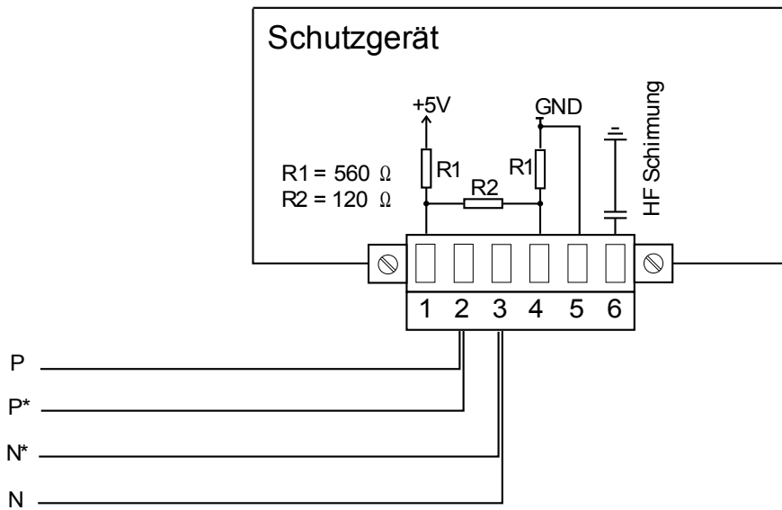
Typ 2 Verdrahtungsbeispiel, Gerät in der Mitte des Busses
