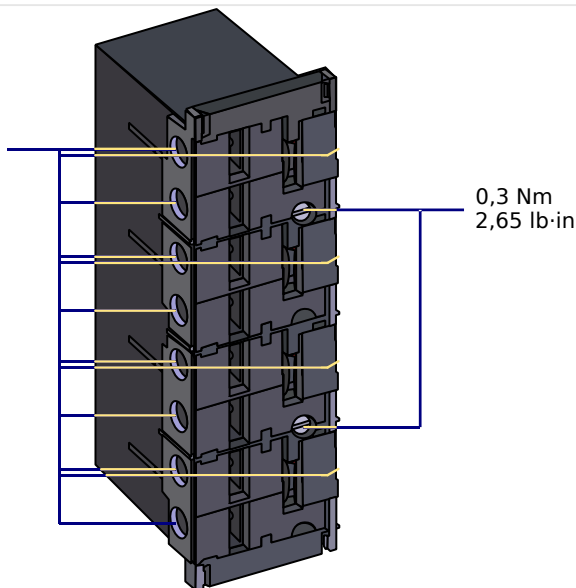
Рис. 95: Штепсельные соединения со встроенными закорачивающими перемычками (стандартные токовые входы)
