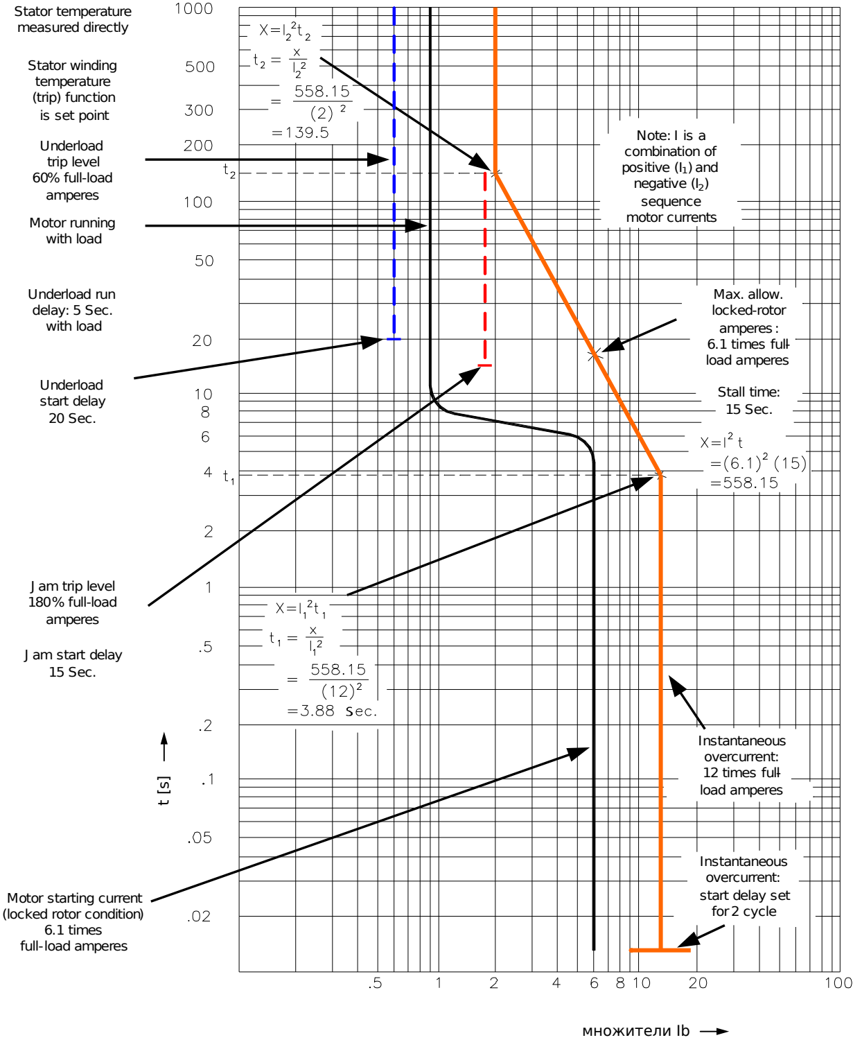
Рис. 59: Кривая защиты двигателя (пример 3 — с ТДС).
