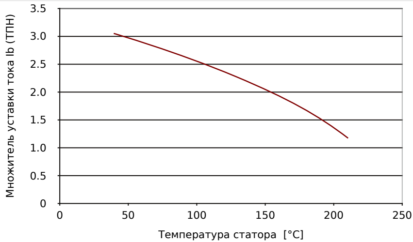
Рис. 54: Эффективная уставка тока по ср. с максимальной температурой статора.
