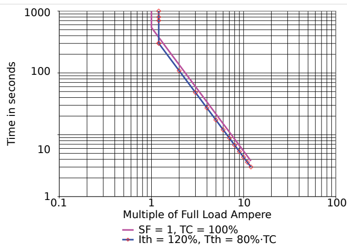
Рис. 55: Кривые ограничений и отключения тепловой модели без ТДС.
