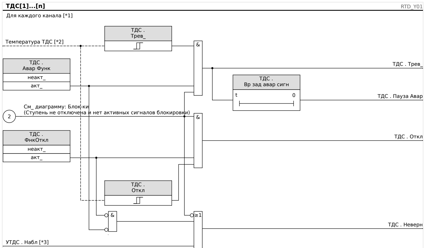
Рис. 73: Общий принцип работы (аварийный сигнал с задержкой, отключение без задержки).
