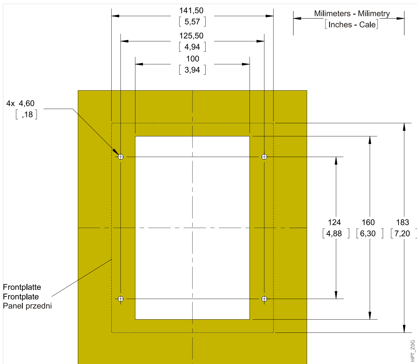
Рис. 6: Вырез дверцы в корпусе V1 (версия с 8 кнопками). (Все размеры указаны в миллиметрах, за исключением размеров в квадратных скобках — [дюймы].)
