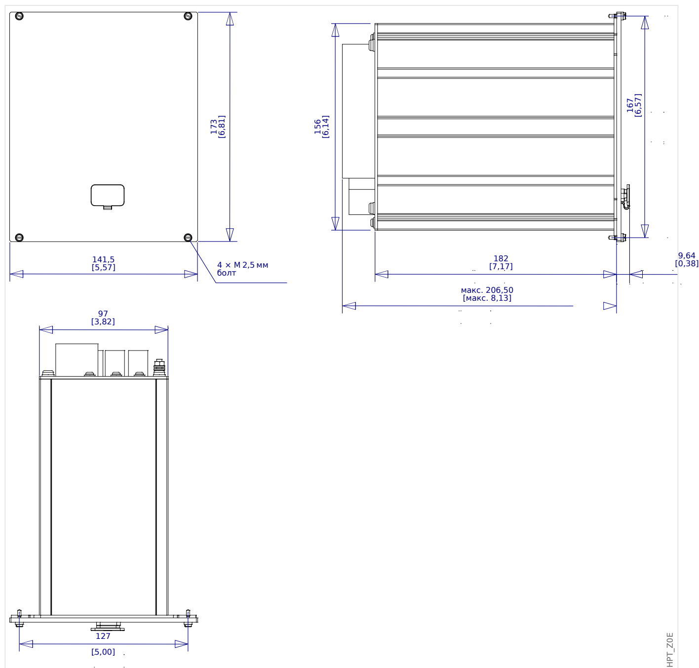
Рис. 4: Корпус V1: внешний вид (19-дюймовые устройства). (Все размеры указаны в миллиметрах, за исключением размеров в квадратных скобках — [дюймы].)
