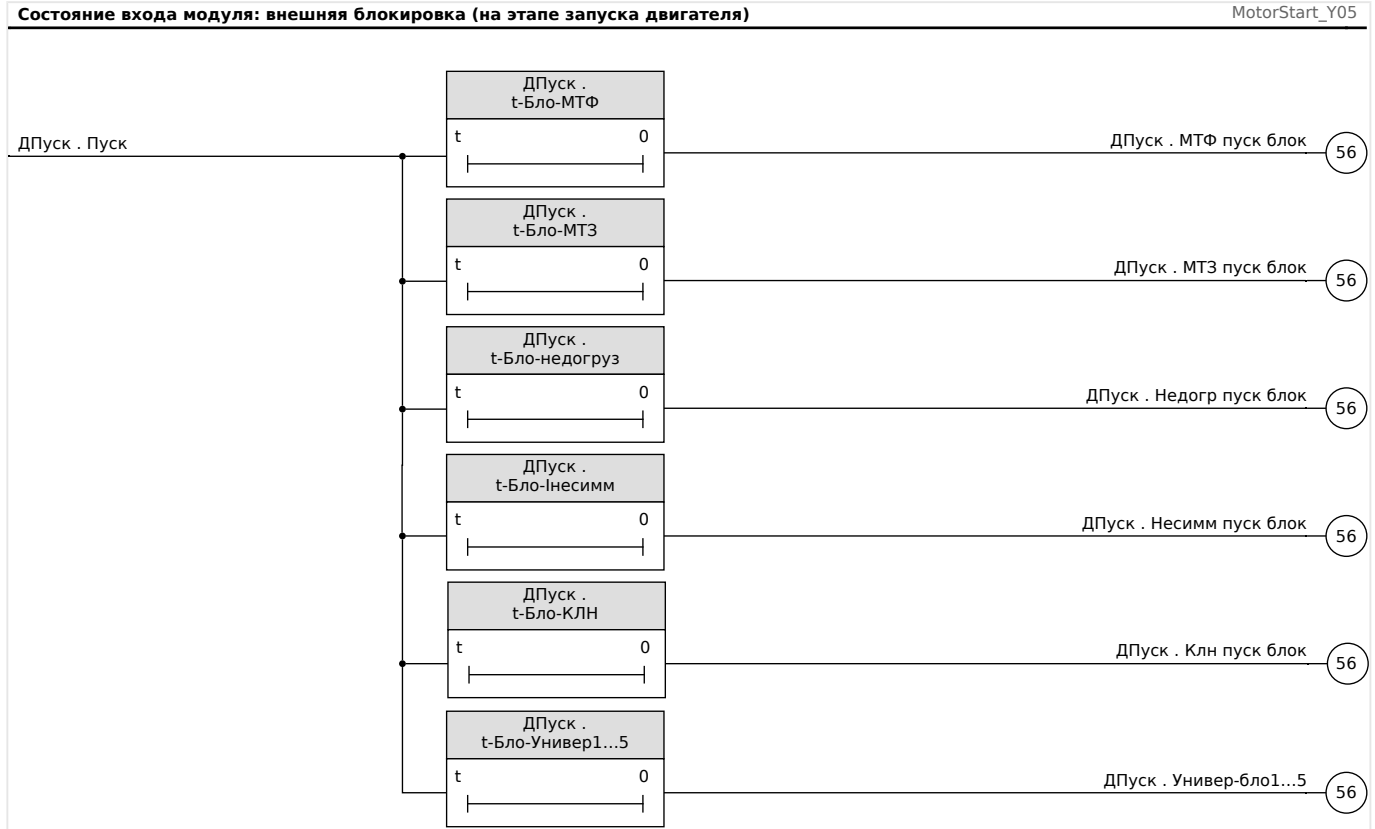
Рис. 51: Временная блокировка токовых защитных функций во время запуска двигателя.
