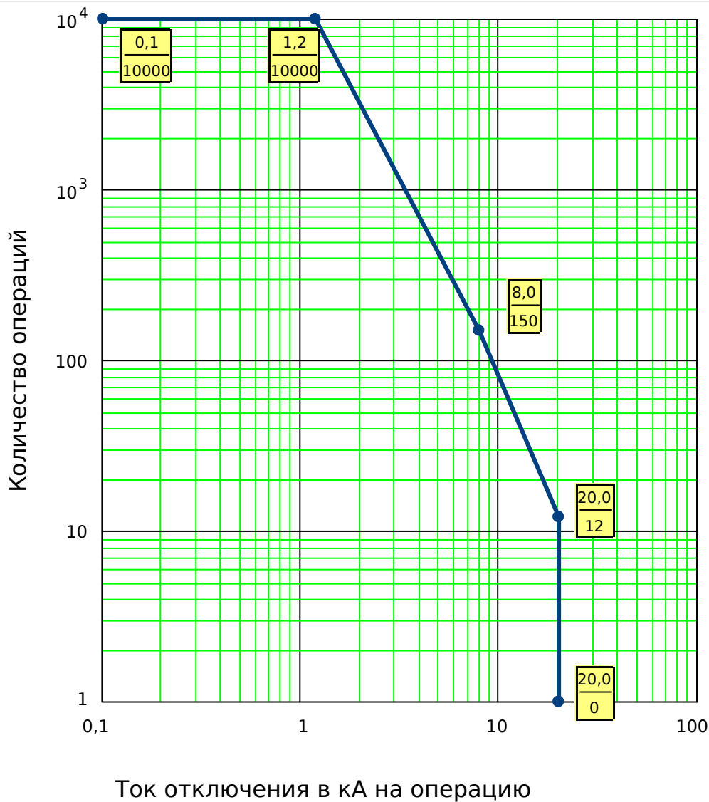
Рис. 82: Эксплуатационная кривая выключателя для типичного выключателя 25кВ
