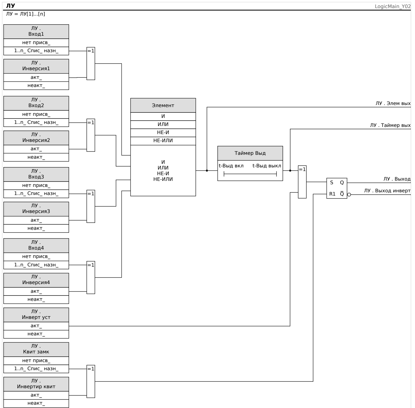
Рис. 89: Подробный обзор — общая логическая схема.
