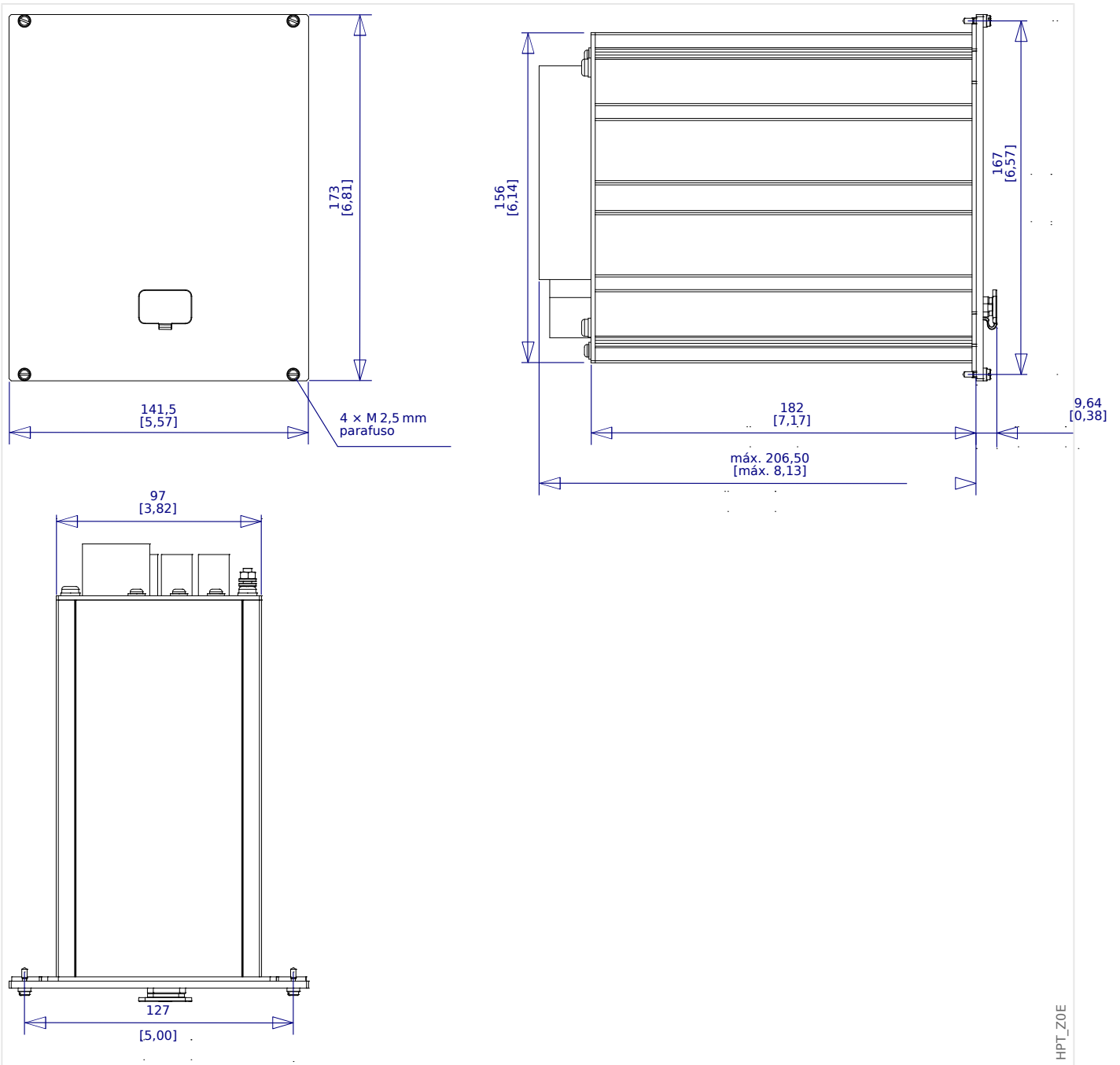
Fig. 4: Vista de 3 lados, carcasa B1 (dispositivos de 19 pulg.) Todas las dimensiones se expresan en mm, excepto las dimensiones entre paréntesis [pulg.]
