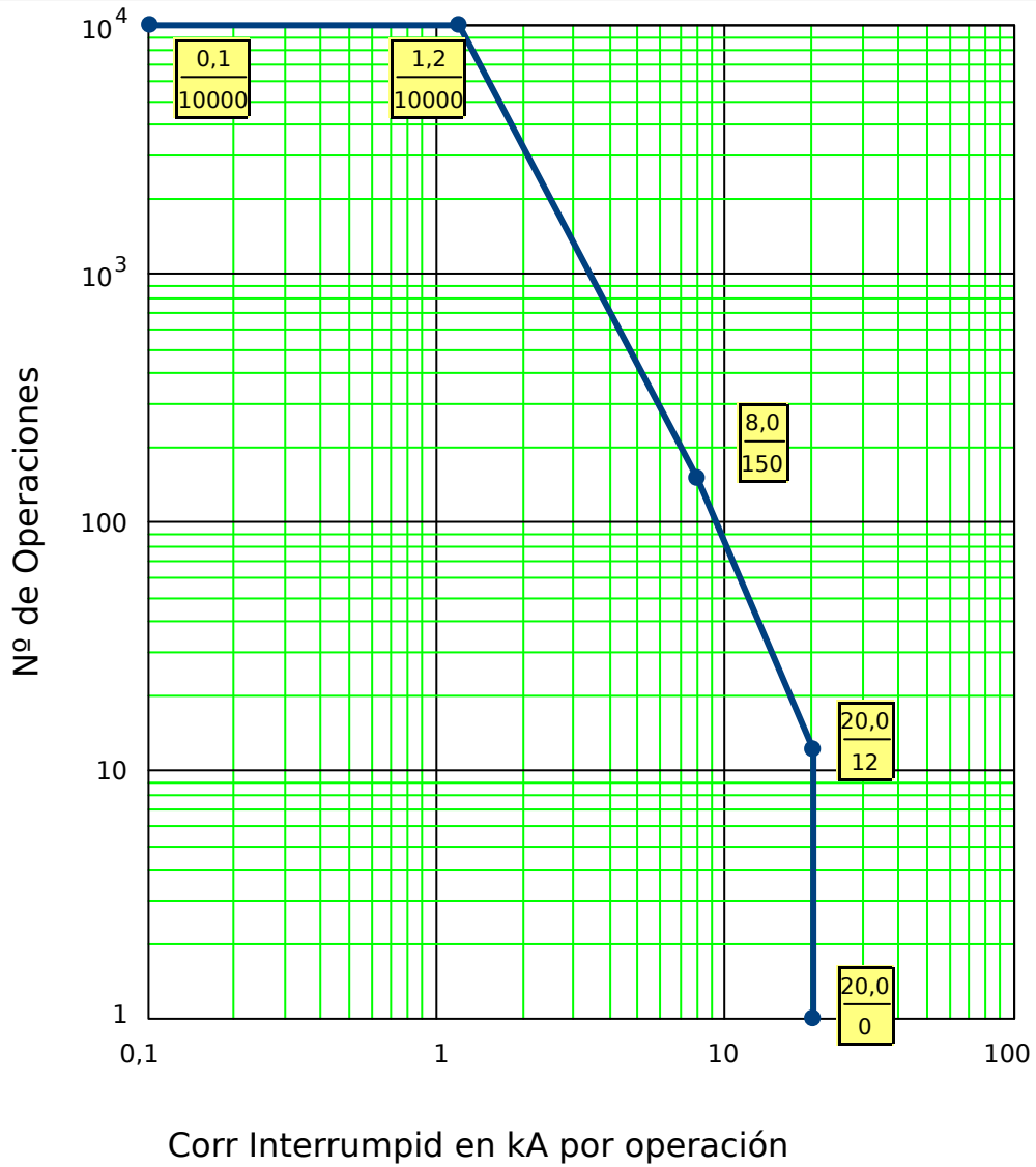
Fig. 82: Curva Mantenim Interruptor para Interrupt Circuito típico 25kV
