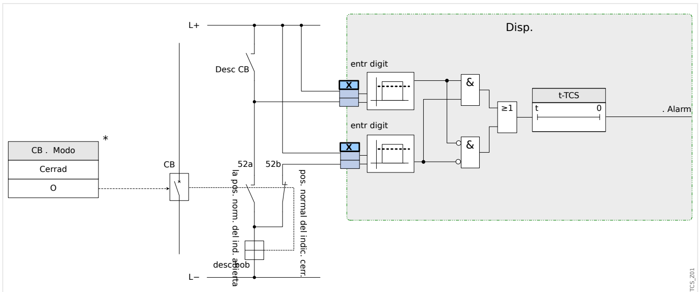
Fig. 74: Ejemplo de conexión: Supervisión del circuito de desconexión con dos contactos auxiliares CB »Aux ON« (52a) and »Aux OFF« (52b).
