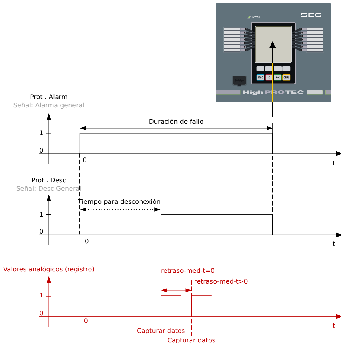
Fig. 87: Registrador de fallos: tiempos y duraciones.
