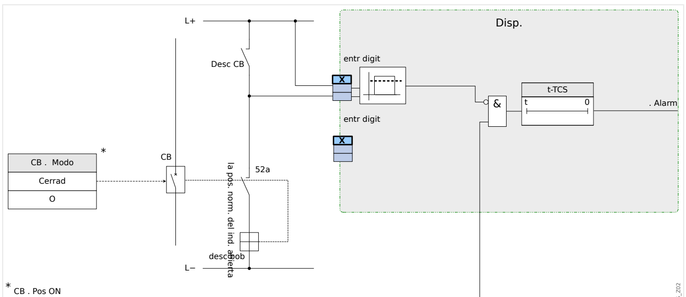
Fig. 75: Ejemplo de conexión: Supervisión del circuito de desconexión solo con un contacto auxiliar CB »Aux ON« (52a).
