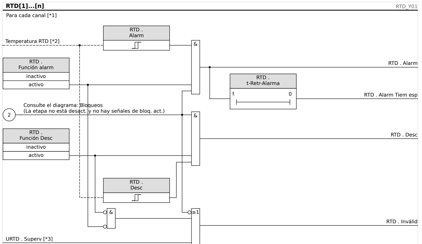
Fig. 73: El principio de funcionamiento general (alarma retrasada, desconexión sin retraso).
