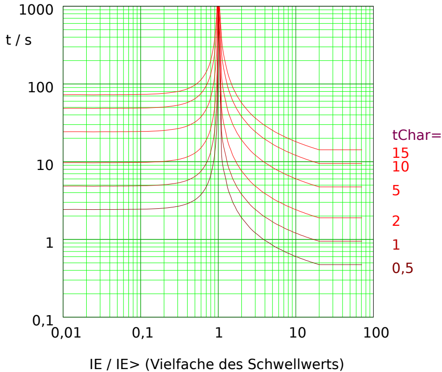
Abb. 79: MINV: Rückfallverzögerung (linke Hälfte, IE < I_{E>} ) und Auslöseverzögerung (rechte Hälfte, IE > I_{E>} ), Beispieldiagramm für I_{max} = 20 \cdot I_{E>} .
