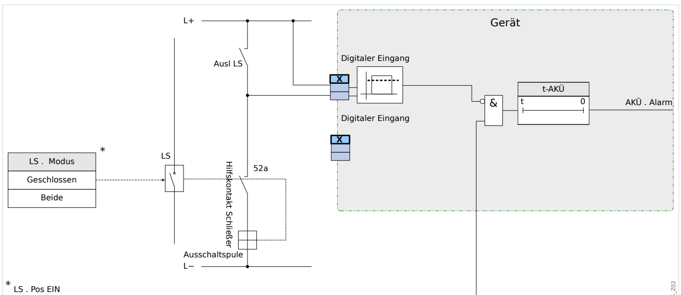
Abb. 92: Anschlussbeispiel: Auslösekreisüberwachung mit einem Hilfskontakt »Hiko EIN« (52a).
