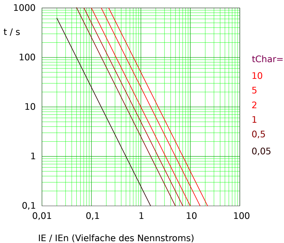
Abb. 85: Auslösekurve „I2T“, wobei nur der Bereich IE > I_{E>} jeweils anwendbar ist. Beispieldiagramm für gemessenen (nicht empfindlichen) Erdstrom.
