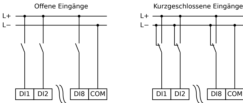
Abb. 114: Sicherer Zustand der digitalen Eingänge
