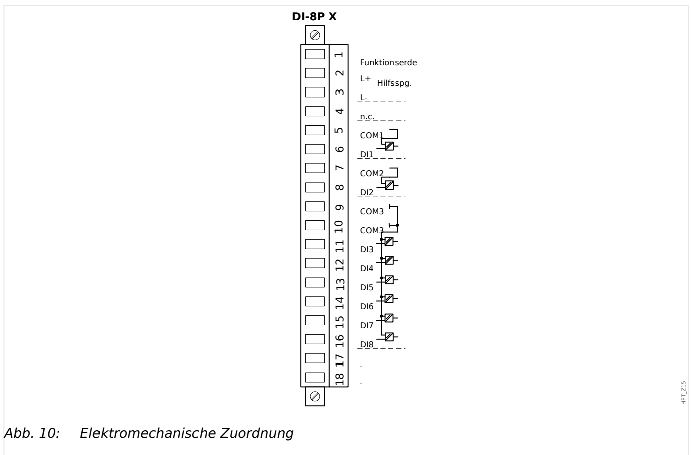
Abb. 9: Klemmenbelegung
