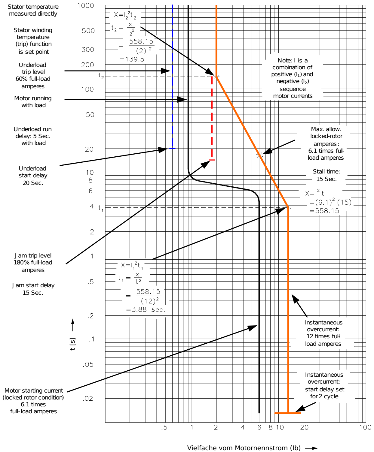
Abb. 59: Auslösekennlinien (Beispiel 3 - mit RTDs).
