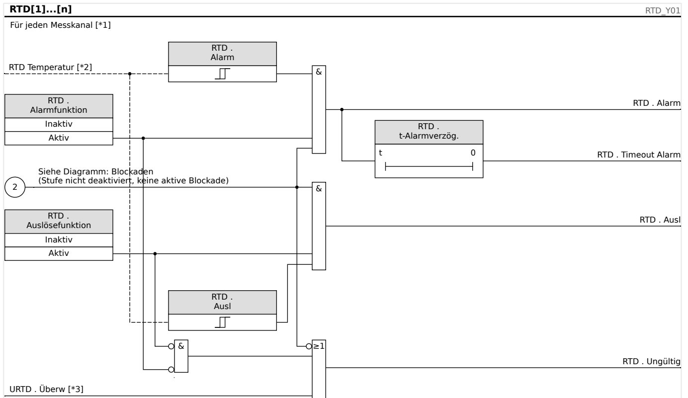
Abb. 90: Generelles RTD-Funktionsprinzip.
