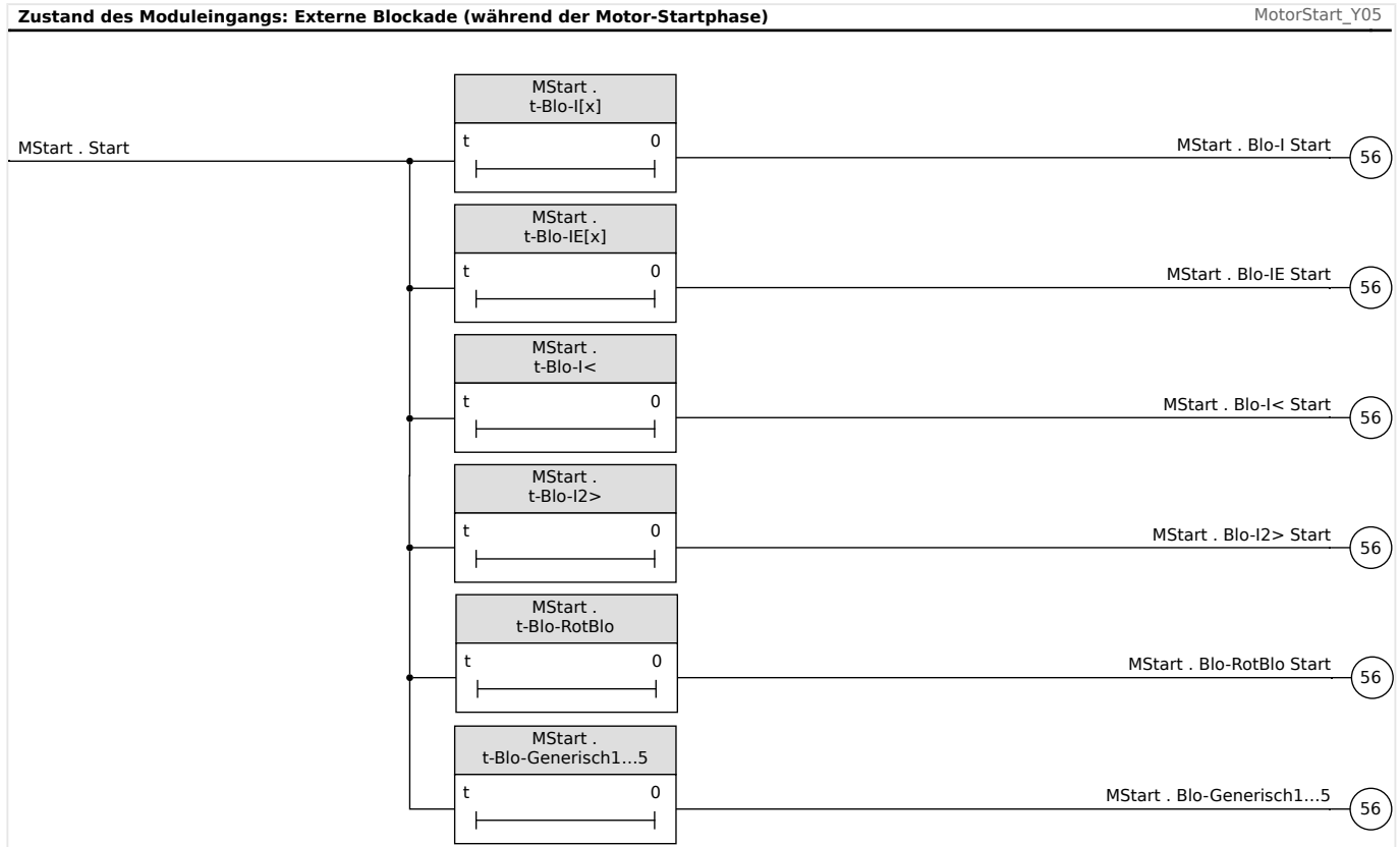
Abb. 51: Temporäre Blockade von Stromschutzfunktionen während Motorstarts.
