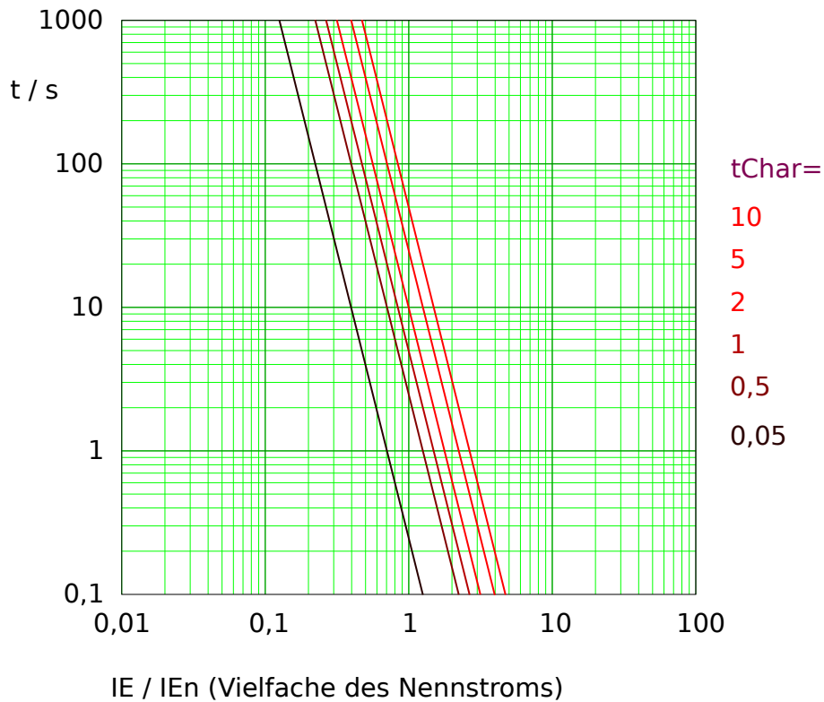
Abb. 86: Auslösekurve „I4T“, wobei nur der Bereich IE > I_{E>} jeweils anwendbar ist. Beispieldiagramm für gemessenen (nicht empfindlichen) Erdstrom.
