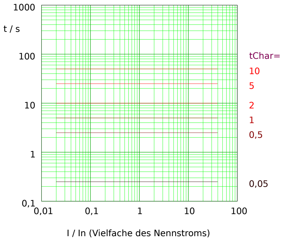
Abb. 70: Auslösekurve „Therm Flat“, wobei nur der Bereich I > I_{>} jeweils anwendbar ist.
