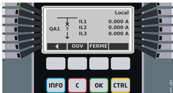
Fig. 68: Exemple de page de contrôle, avec le « disjoncteur » en position de dysfonctionnement (ou invraisemblable).
