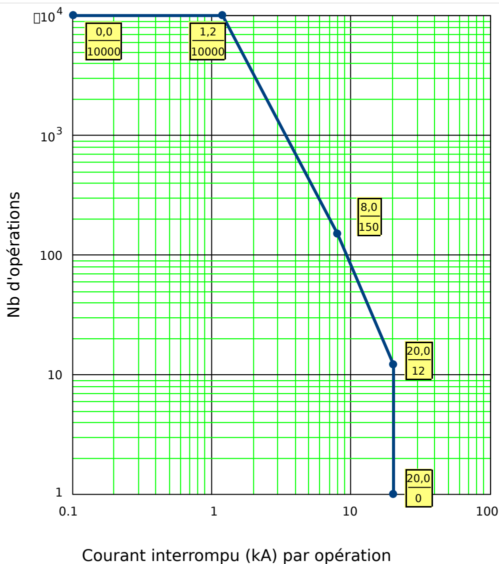
Fig. 72: Courbe de maintenance du disj pour un disj 25 ~kV typique
