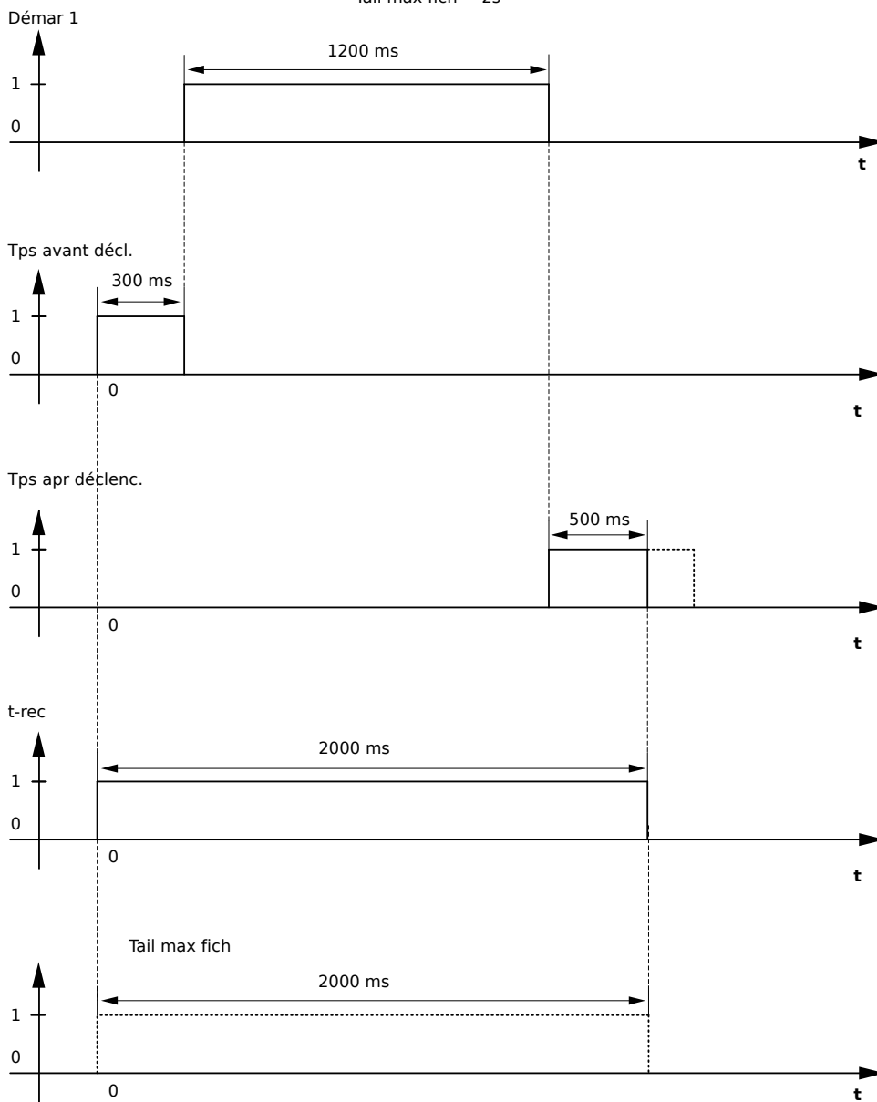
Fig. 75: Exemple de diagramme des temps de l'enregistreur de perturbations I
