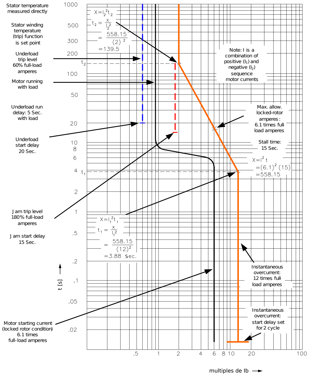
Fig. 57: Courbe de protection du moteur (exemple 3 - avec thermomètres à résistance).
