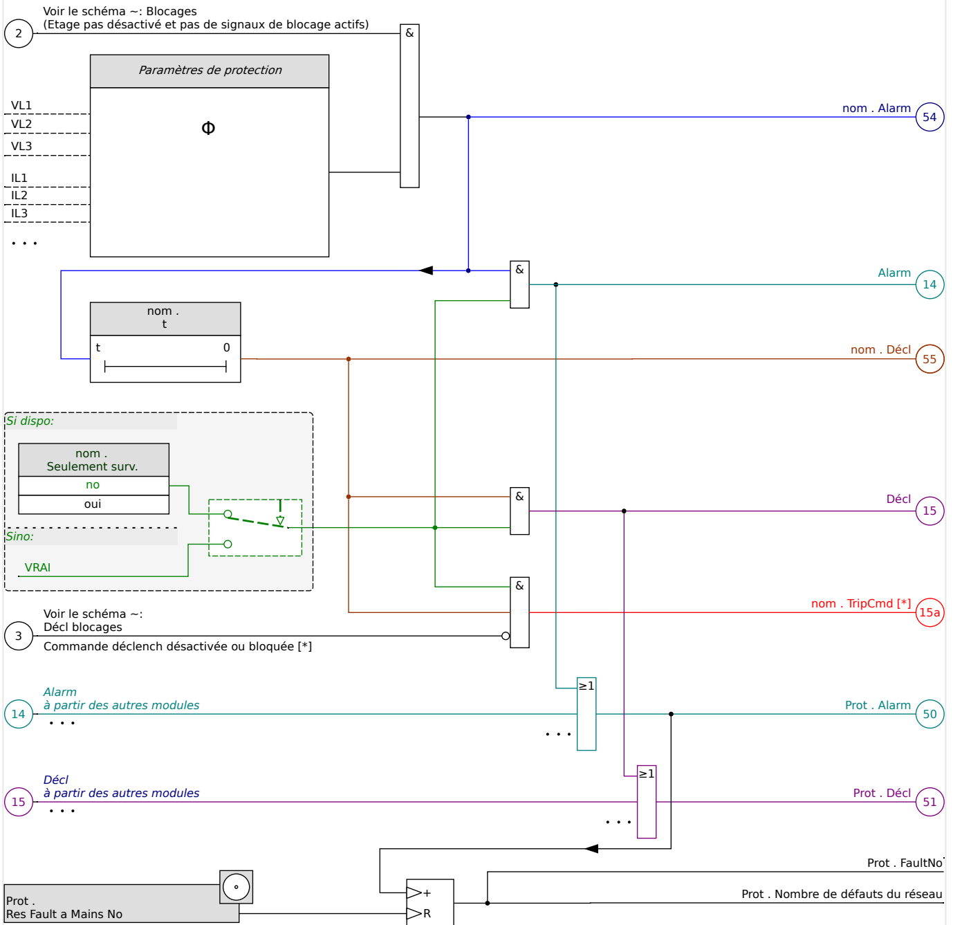
Fig. 48: Schéma de fonctionnalité des éléments de protection HighPROTEC.
