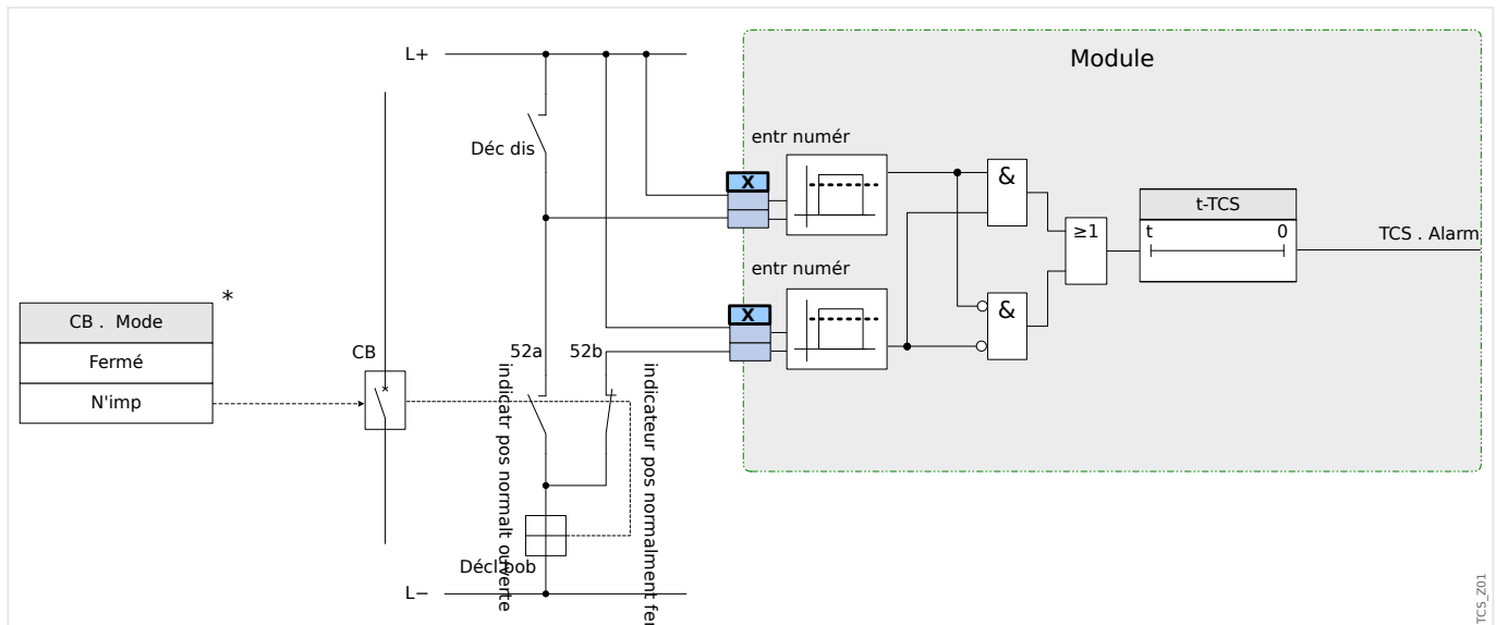
Fig. 64: Exemple de connexion : Surveillance du circuit de déclenchement avec de contacts auxiliaires de disjoncteur «Aux ON» (52a) et «Aux OFF» (52b).
