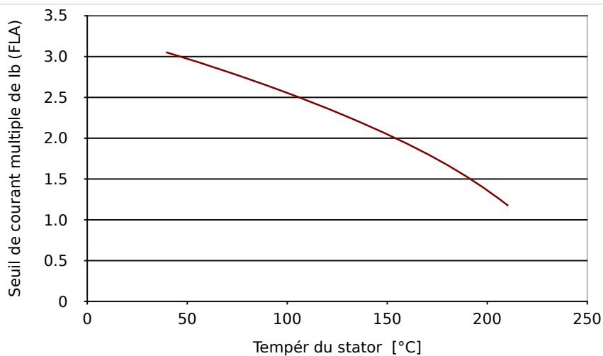
Fig. 52: Seuil de courant efficace / Tempér maxi du stator.
