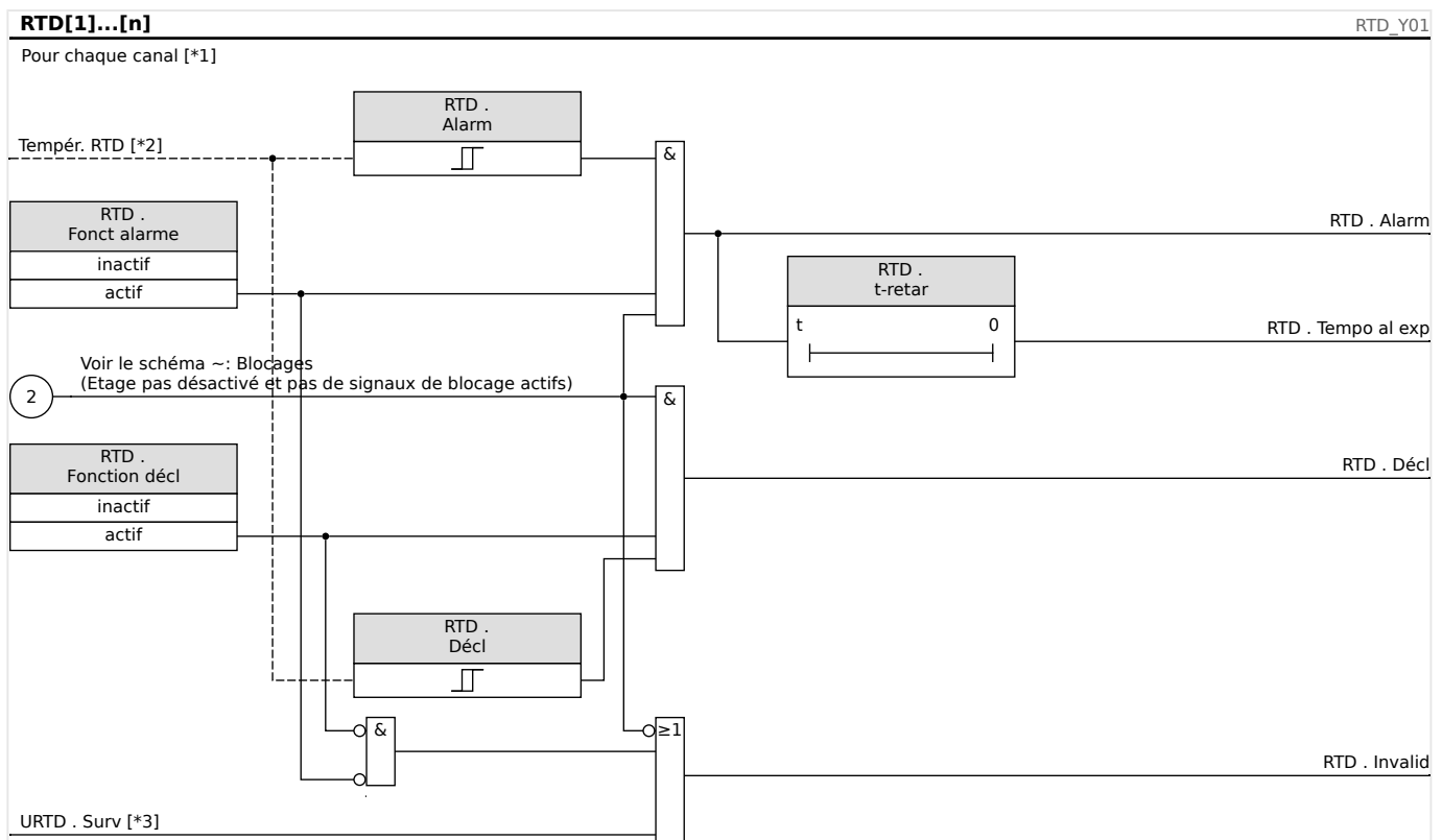
Fig. 63: Principe de fonctionnement général (alarme retardée, déclenchement non retardé).
