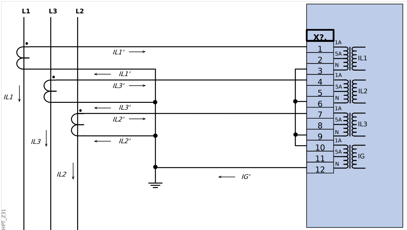
Fig. 28: Mesure de courant triphasé; I_n \text{ sec} = 1 \text{ A} Mesure courant via connexion de Holmgreen; I_{Gnom} \text{ sec} = 1 \text{ A}
