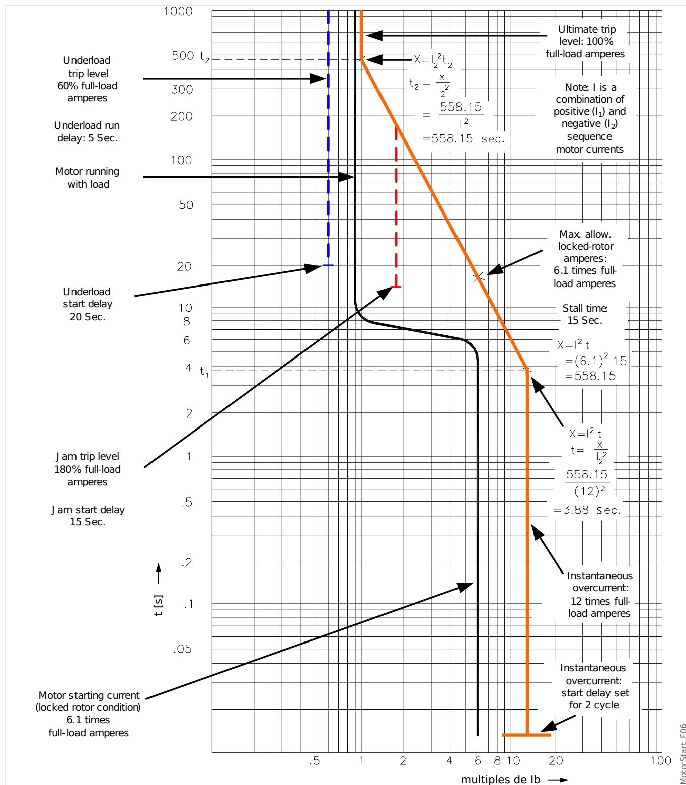
Fig. 56: Courbe de protection du moteur (exemple 2 - sans thermomètres à résistance).
