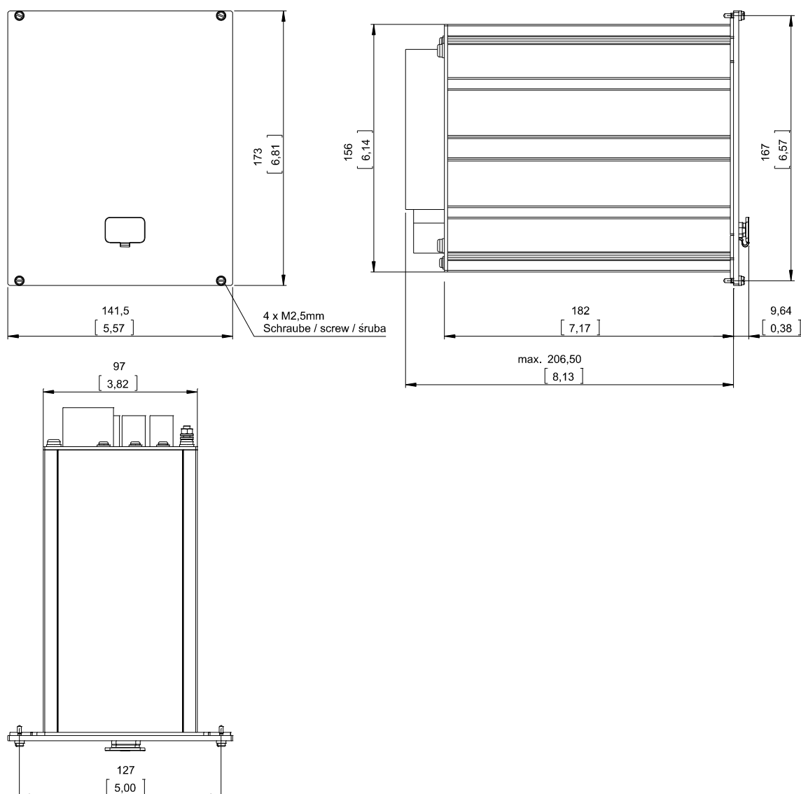
Obudowa B1 — widok z trzech stron (urządzenia 19-calowe) (Wszystkie wymiary podano w mm [calach]).
