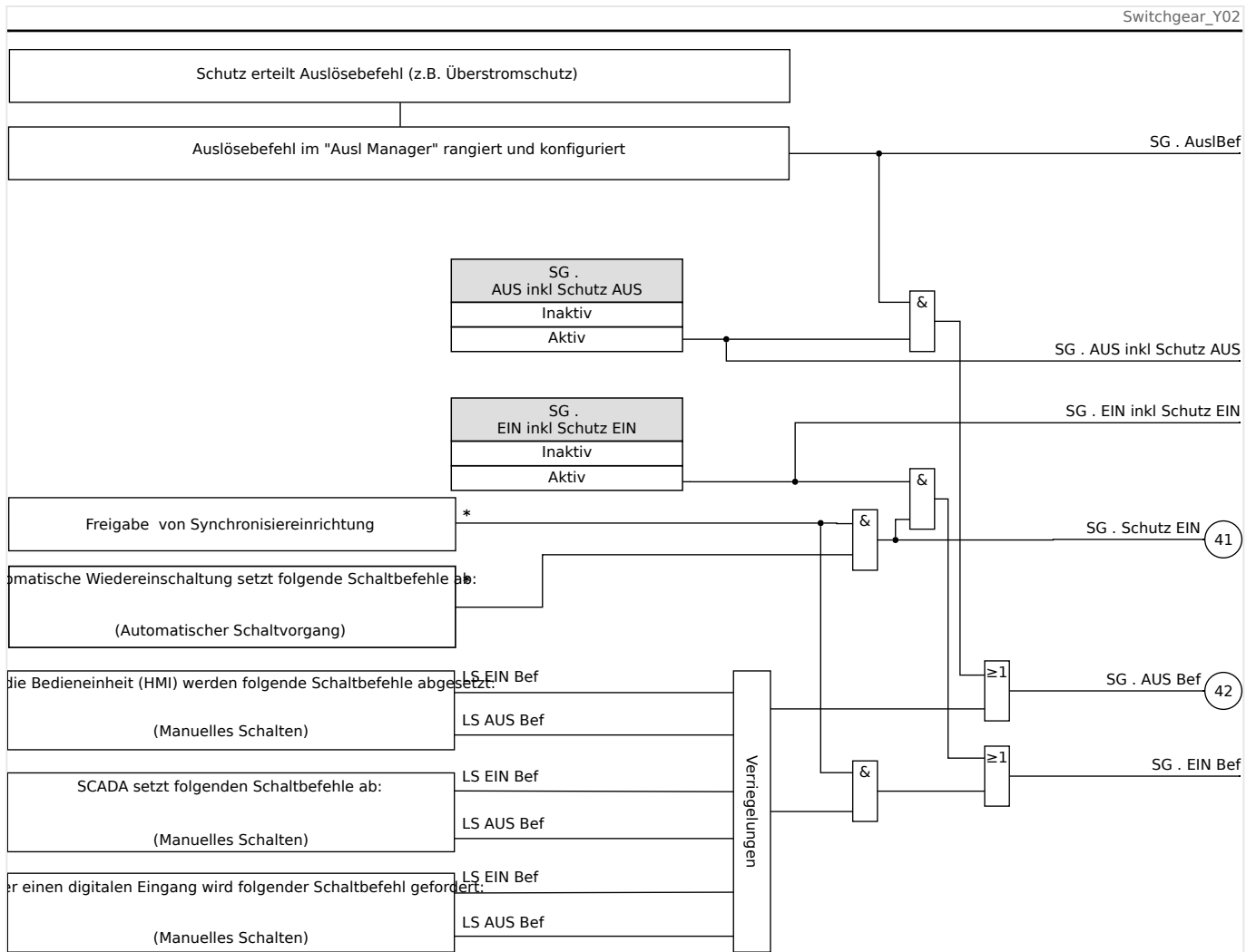
Abb. 98: Verriegelungen. (Für die mit „*“ markierten Teile gilt: Verfügbarkeit hängt von der bestellten Gerätevariante ab.)
