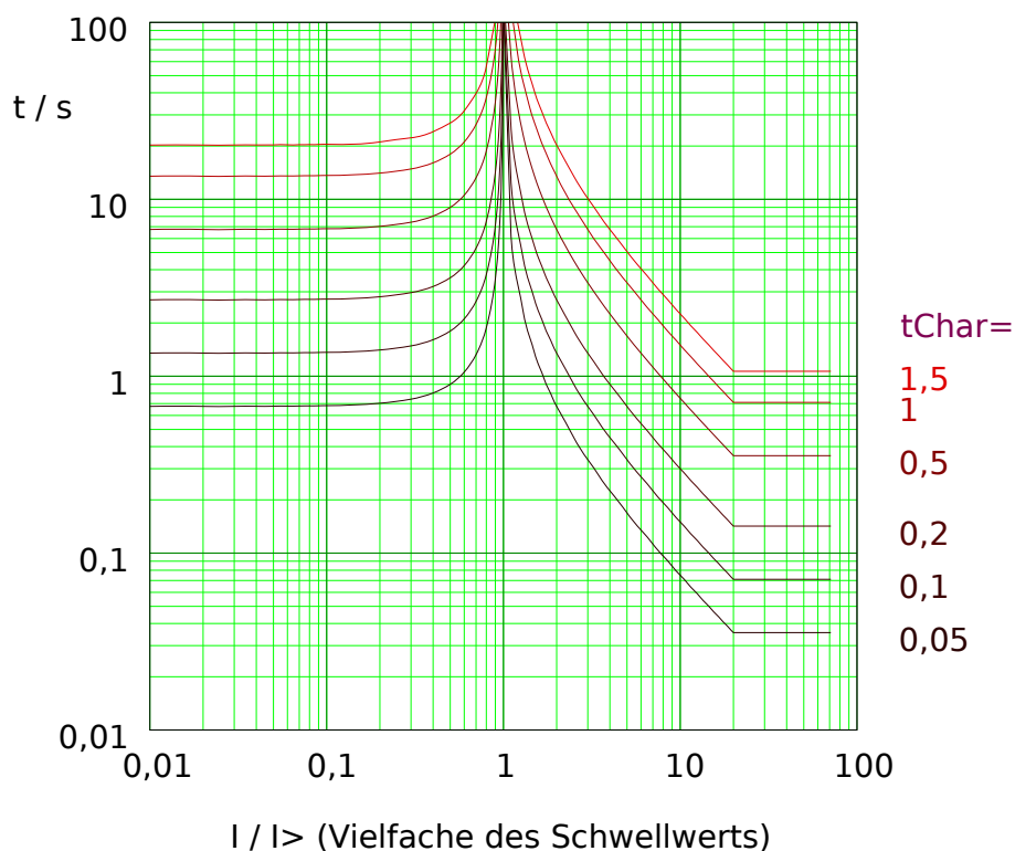
Abb. 63: VINV: Rückfallverzögerung (linke Hälfte, I < I_{>} ) und Auslöseverzögerung (rechte Hälfte, I > I_{>} ), Beispieldiagramm für I_{max} = 20 \cdot I_{>} .
