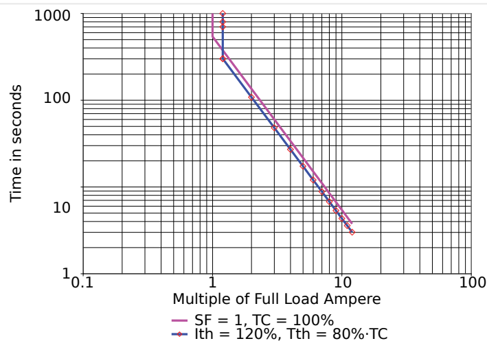
Abb. 55: Thermisches Abbild und Auslösecharakteristik ohne RTD.
