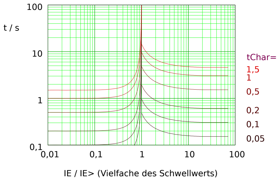
Abb. 78: RINV: Rückfallverzögerung (linke Hälfte, IE < I_{E>} ) und Auslöseverzögerung (rechte Hälfte, IE > I_{E>} ), Beispieldiagramm für I_{max} = 20 \cdot I_{E>} .
