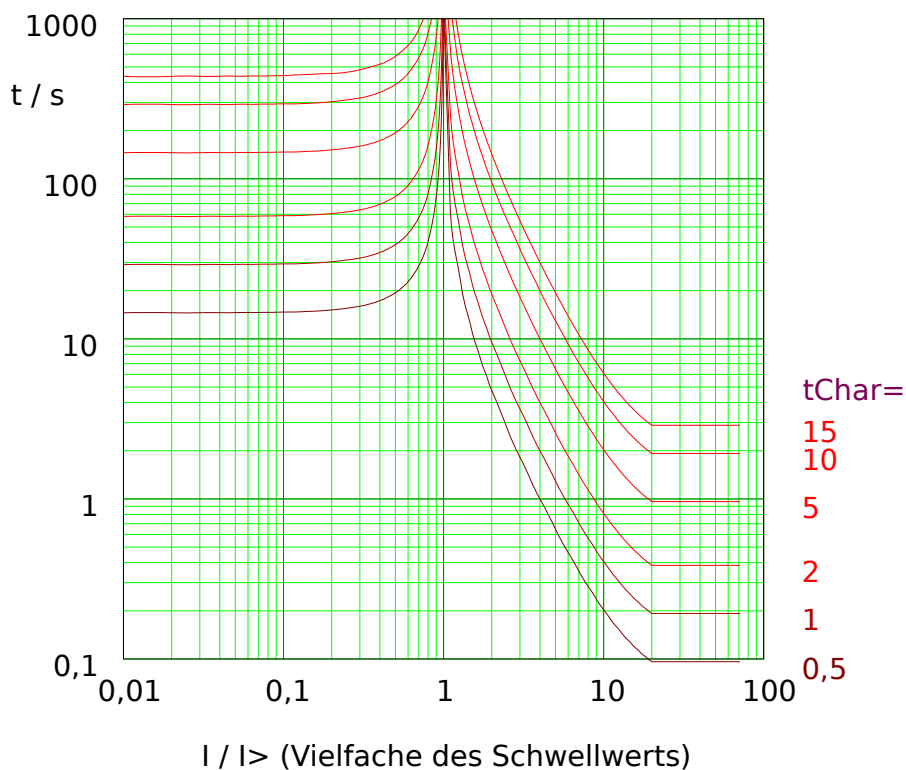
Abb. 69: EINV: Rückfallverzögerung (linke Hälfte, I < I_{>} ) und Auslöseverzögerung (rechte Hälfte, I > I_{>} ), Beispieldiagramm für I_{max} = 20 \cdot I_{>} .
