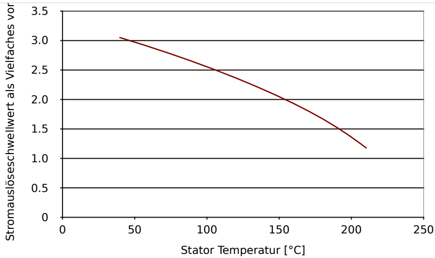
Abb. 54: Stromauslöseschwellwerte (Effektivwerte) über der maximalen Statortemperatur.
