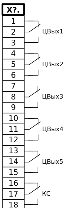
Рис. 14: RO-5 — обозначение разъемов
