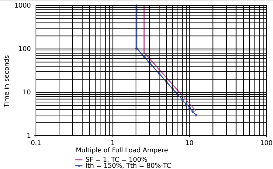
Рис. 56: Кривые ограничений и отключения тепловой модели при ТДС = 100 °С.
