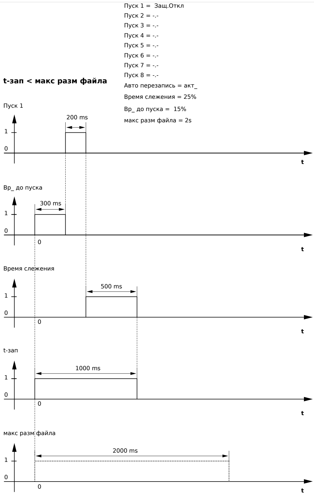
Рис. 86: Пример временной диаграммы регистратора аварийных нарушений II
