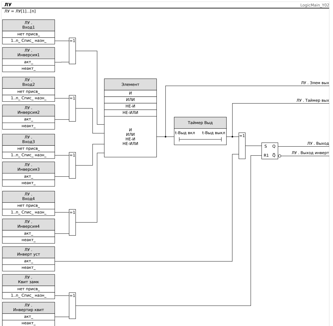
Рис. 89: Подробный обзор — общая логическая схема.
